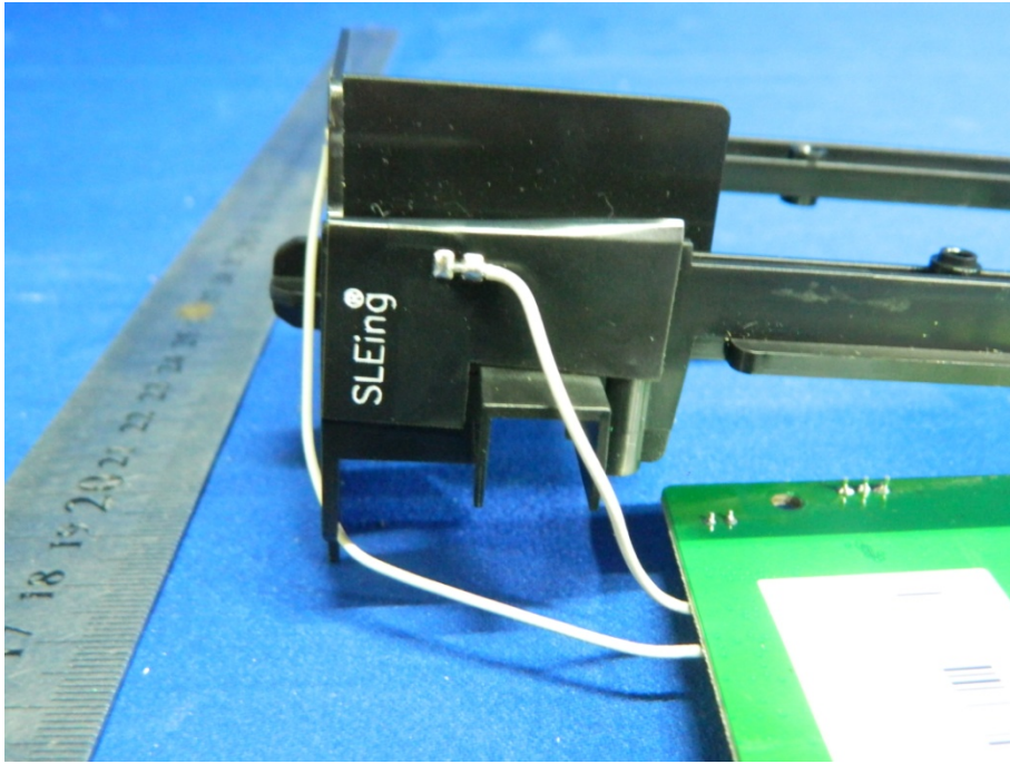
WIFI&BT ANTENNA
