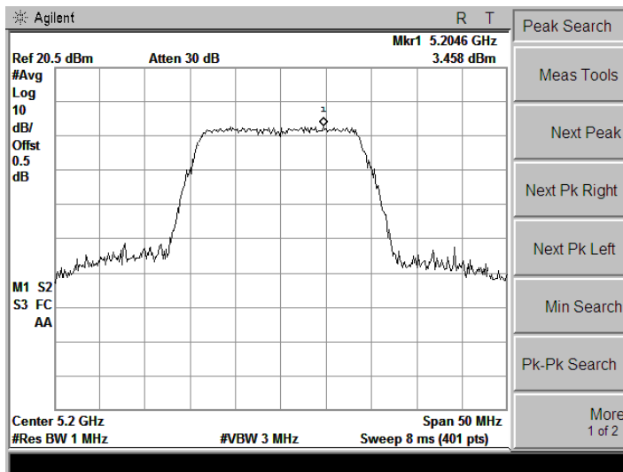
5200 MHz
