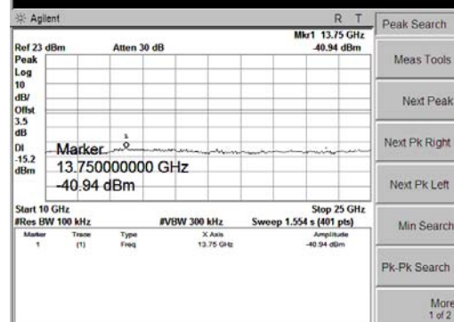
802.11b Mode, Ch6
