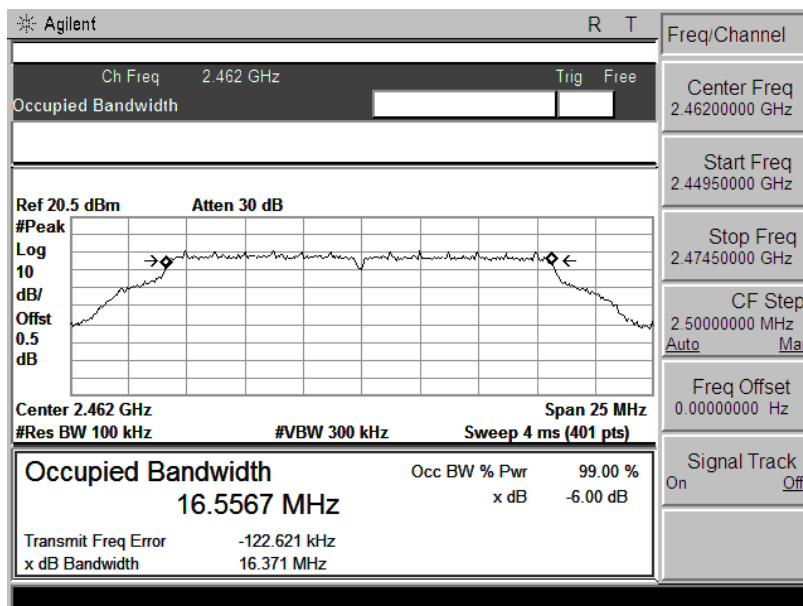
Ch 11 802.11 n(20M) Mode
