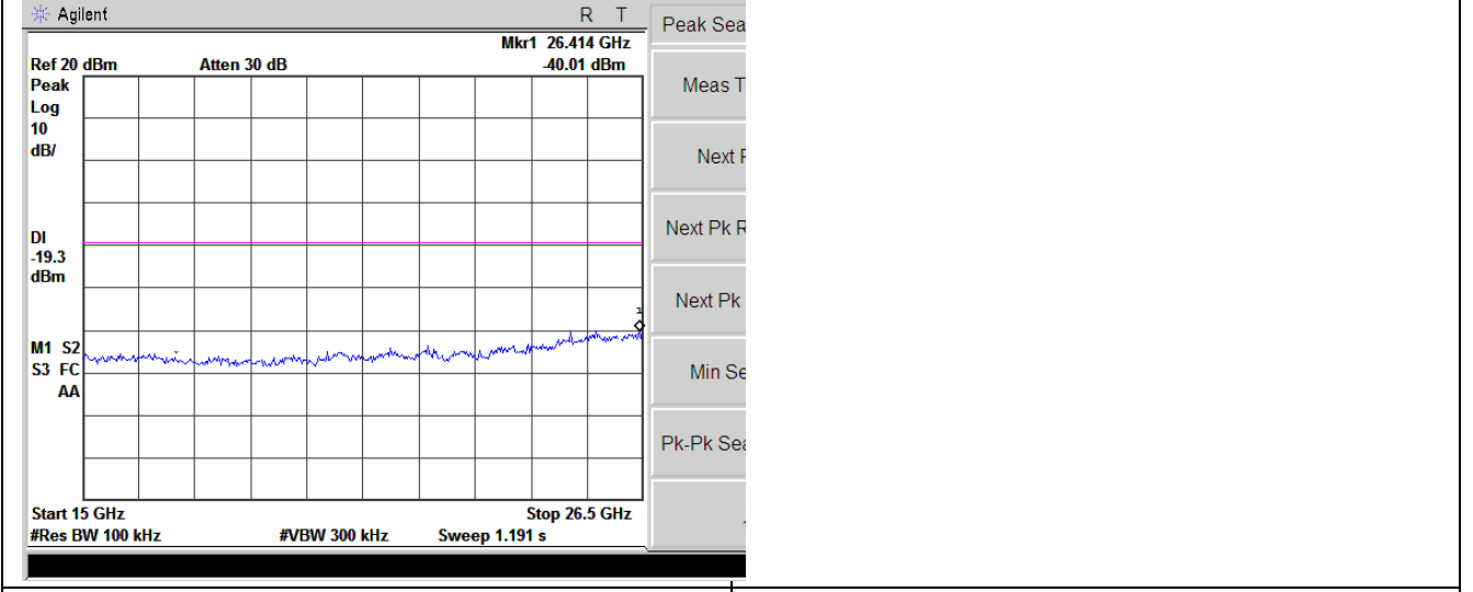
15GHz~26.5GHz Modulaiton: π/4DQPSK Test channel: 39
