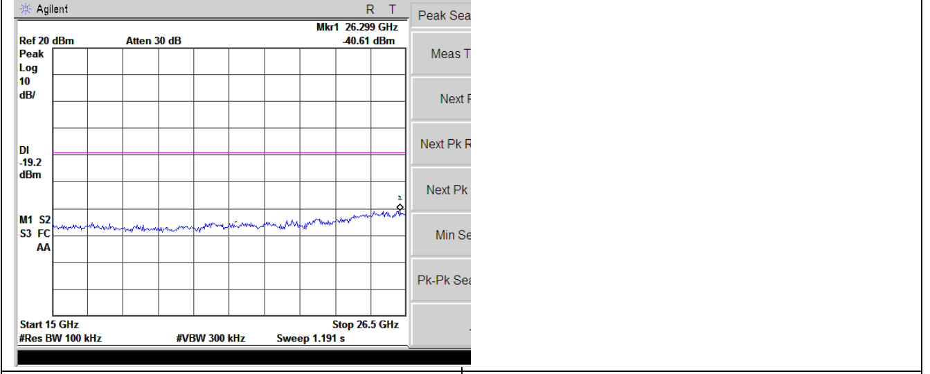
15GHz~26.5GHz Modulaiton: 8DPSK Test channel: 39
