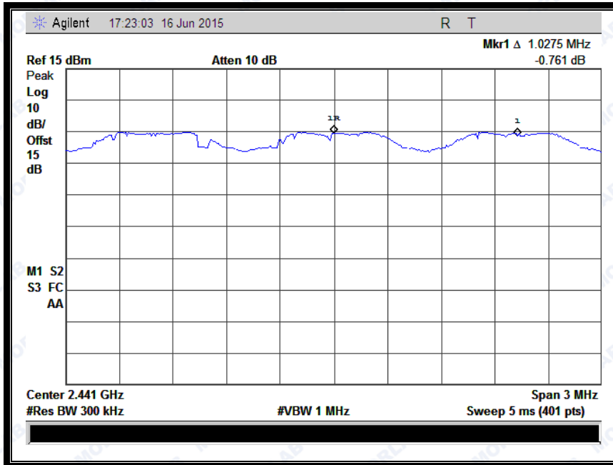
(Plot B: □/4-DQPSK)
