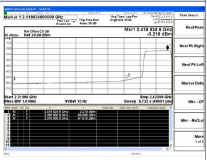
802.11n(HT20)-Low channel(Average)
