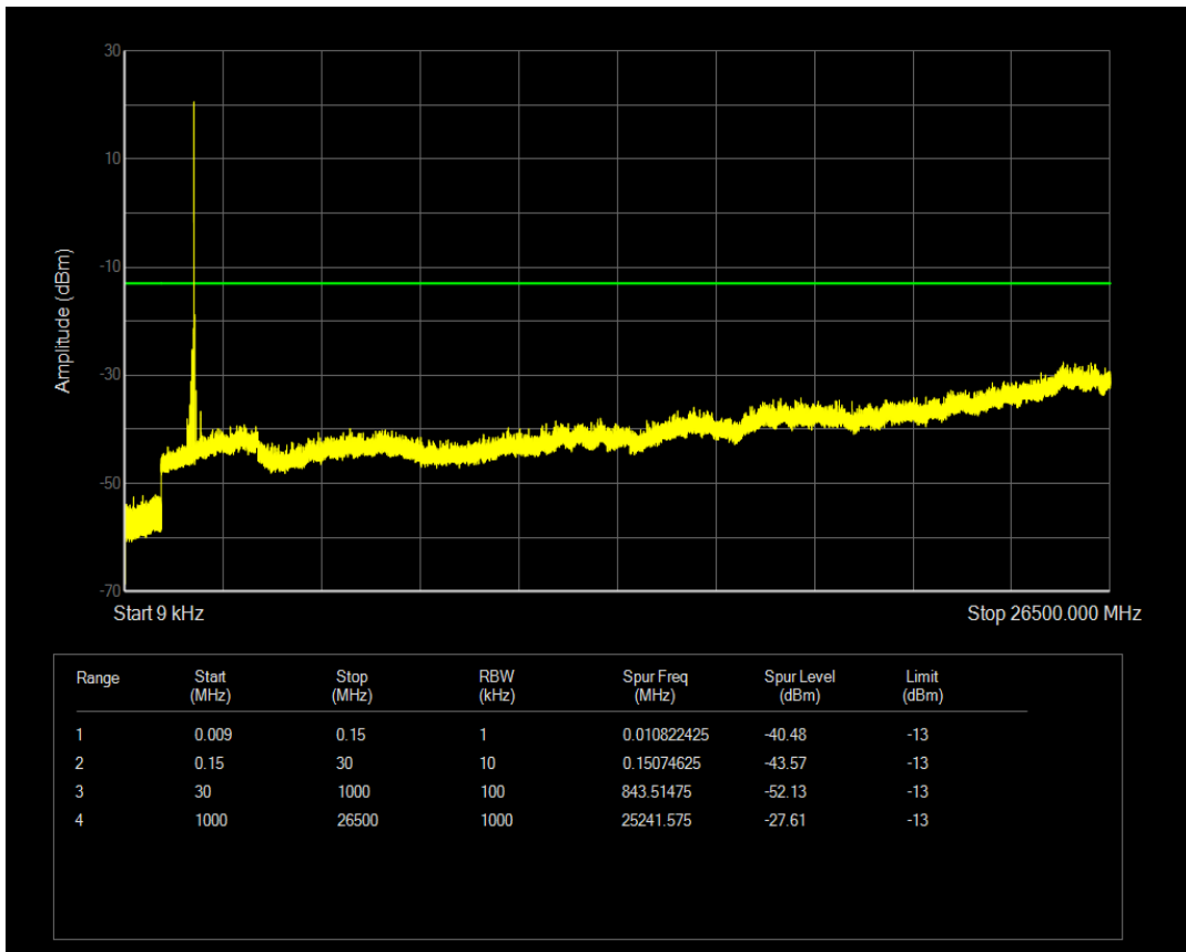
Band2 QPSK Channel=18900 nTones=1@0 Spacing=15kHz
