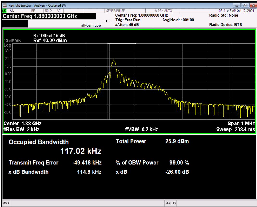
Band2 QPSK Channel=18900 nTones=12@0 Spacing=15kHz
