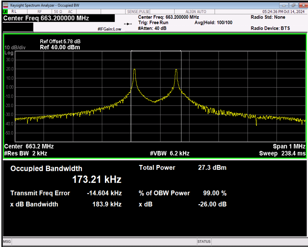
Band71 QPSK Channel=133124 nTones=1@0 Spacing=3.75kHz
