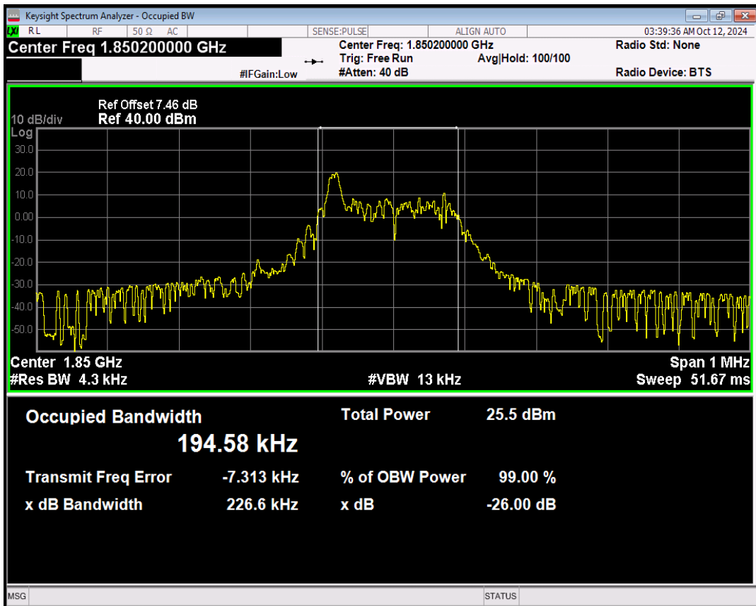
Band2 QPSK Channel=18900 nTones=1@0 Spacing=3.75kHz
