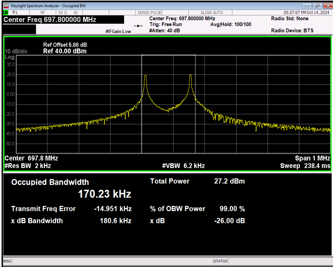
Band71 QPSK Channel=133470 nTones=1@0 Spacing=3.75kHz
