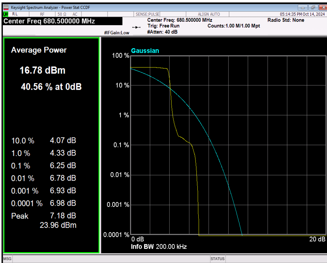
Band71 QPSK Channel=133297 nTones=1@0 Spacing=3.75kHz
