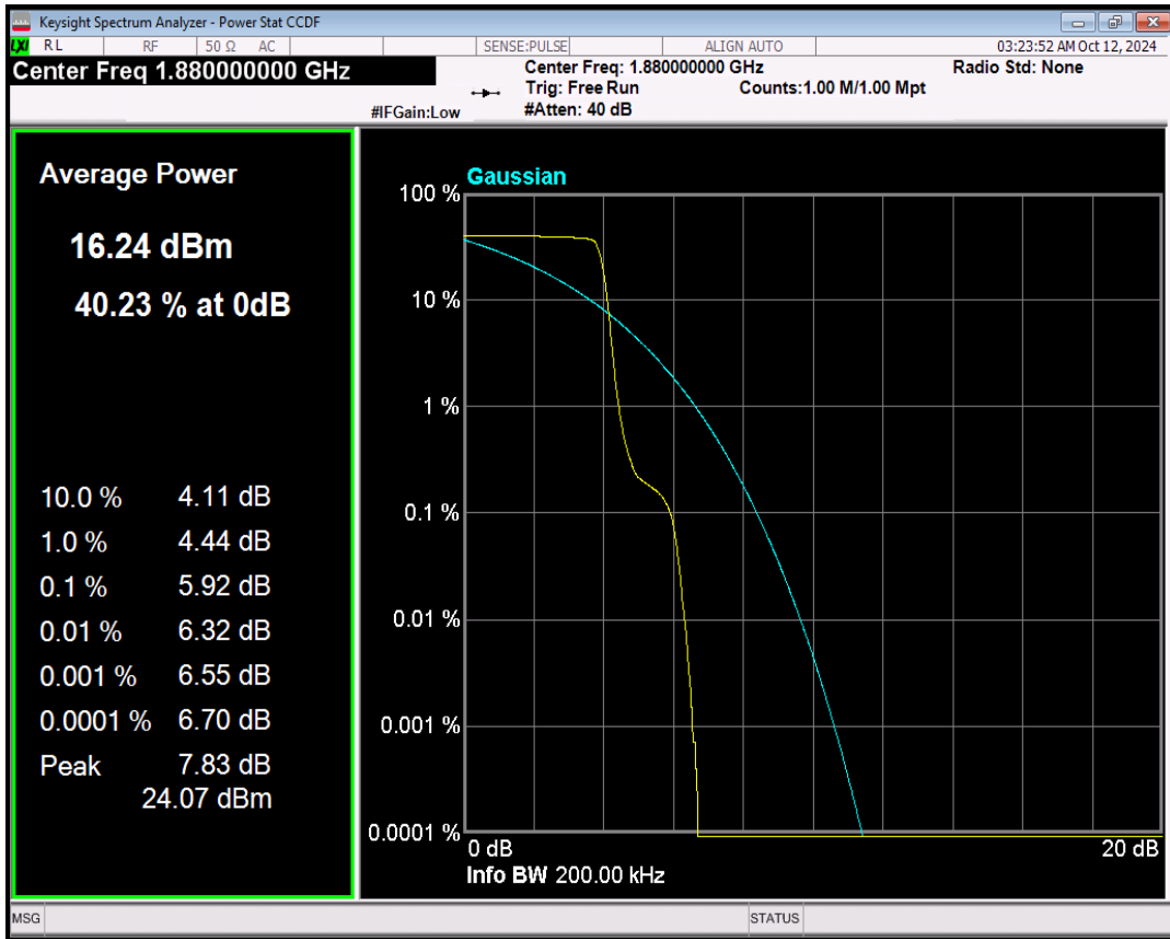
Band2 BPSK Channel=18900 nTones=1@0 Spacing=15kHz
