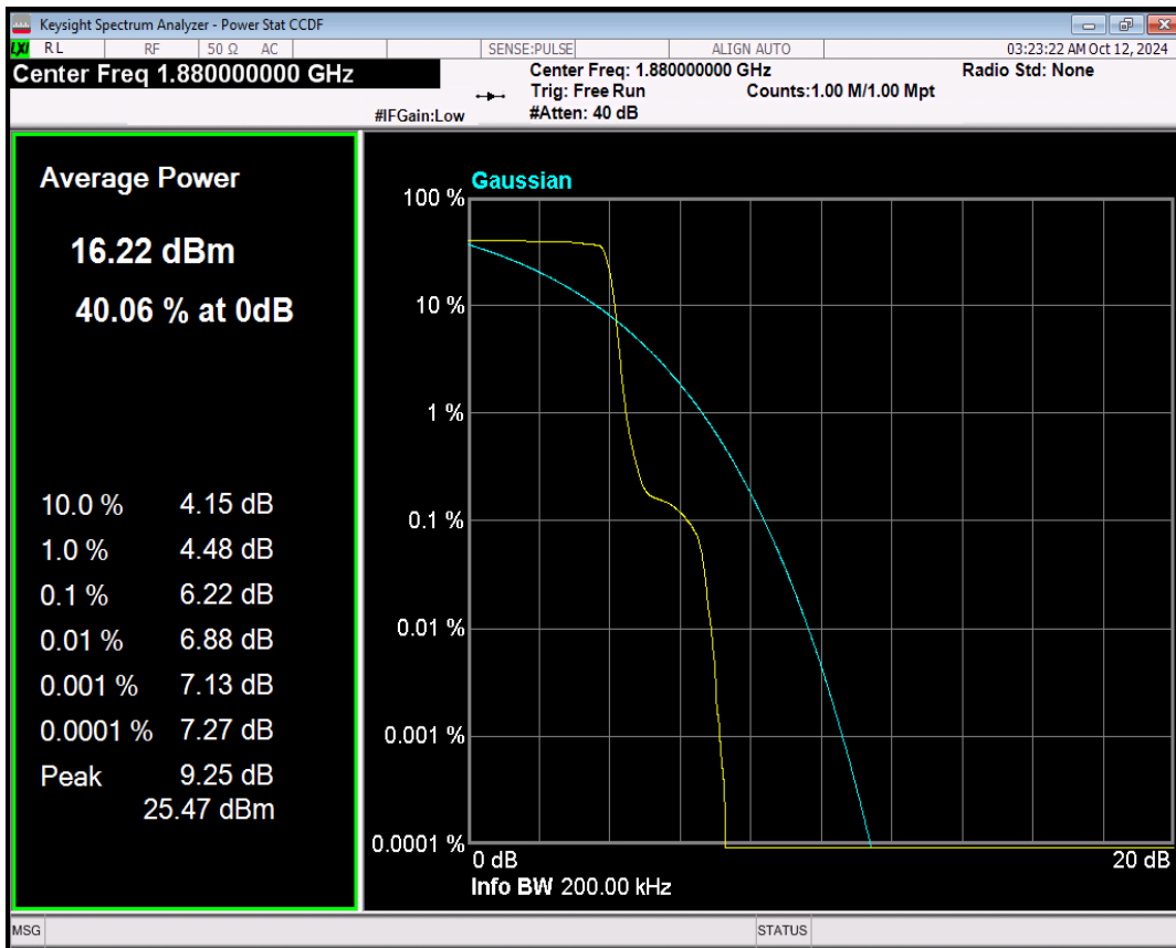
Band2 QPSK Channel=18900 nTones=1@0 Spacing=3.75kHz
