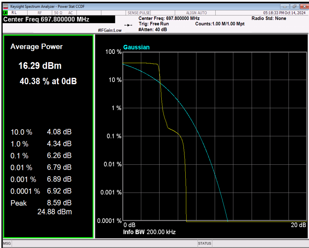
Band71 QPSK Channel=133470 nTones=1@0 Spacing=3.75kHz
