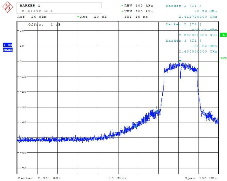
(Plot 4.5.2.2 A: Channel 01: 2412MHz @ 802.11 g)
