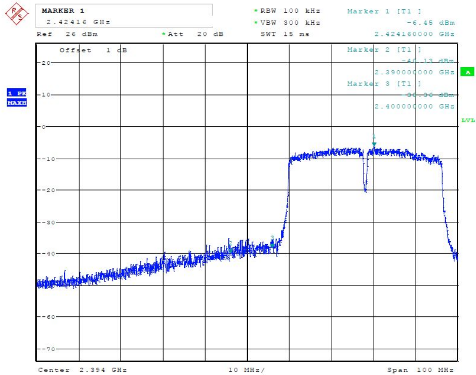
(Plot 4.5.2.4 A: Channel 3: 2422MHz@ 802.11n HT40)
