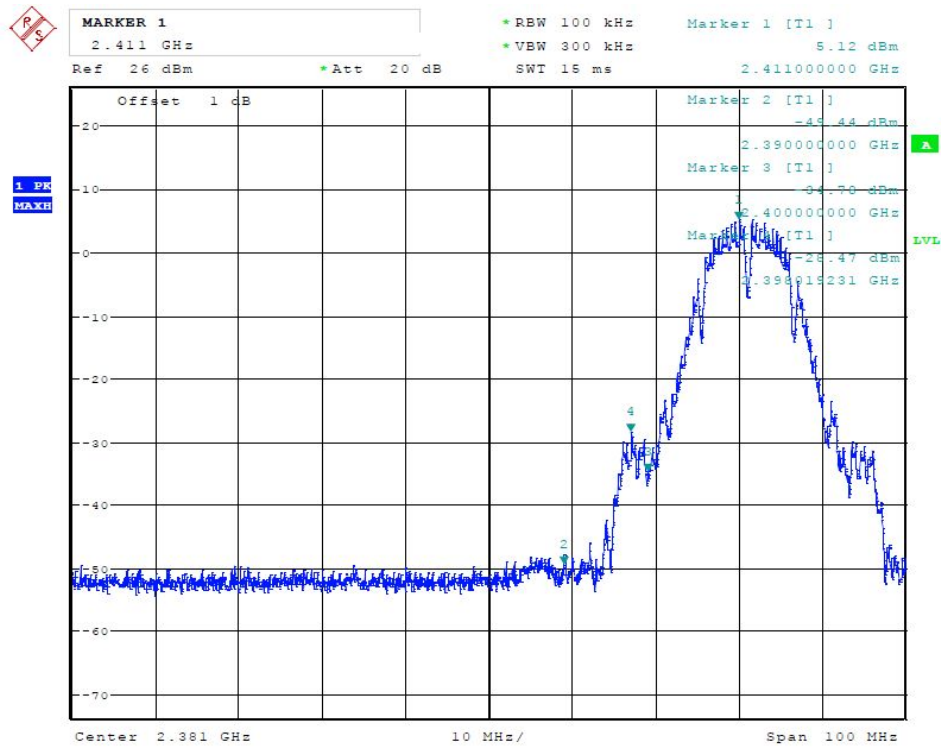
(Plot 4.5.2.1 A: Channel 01: 2412MHz @ 802.11 b )
