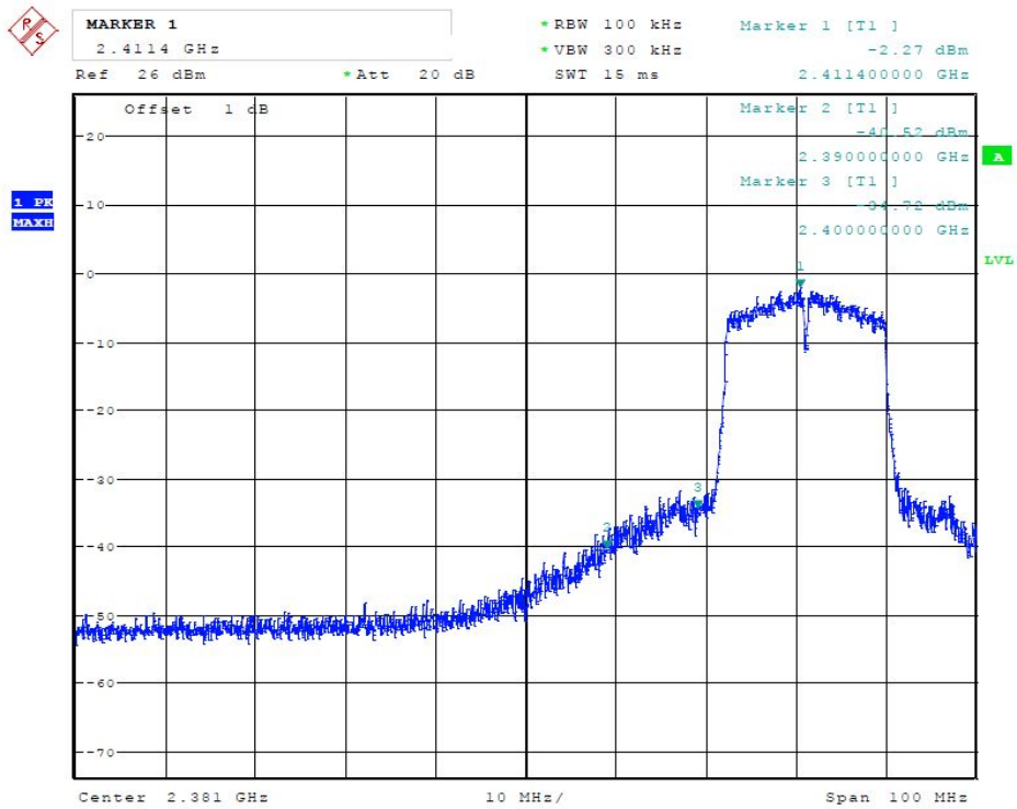
Plot 4.5.2.3 A: Channel 01: 2412MHz @ 802.11n HT20)
