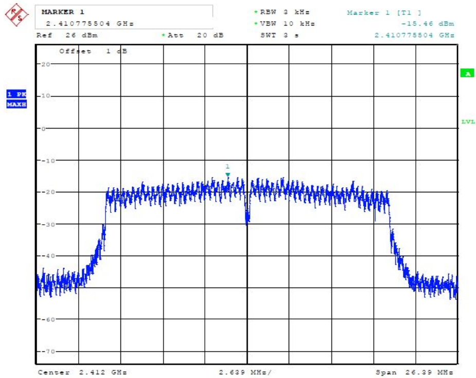
(Plot 4.4.3 A: Channel 1: 2412MHz @ 802.11n HT20)
