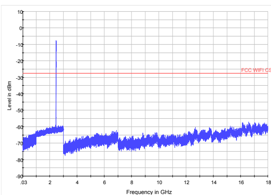
802.11b CH11 30MHz to 18GHz
