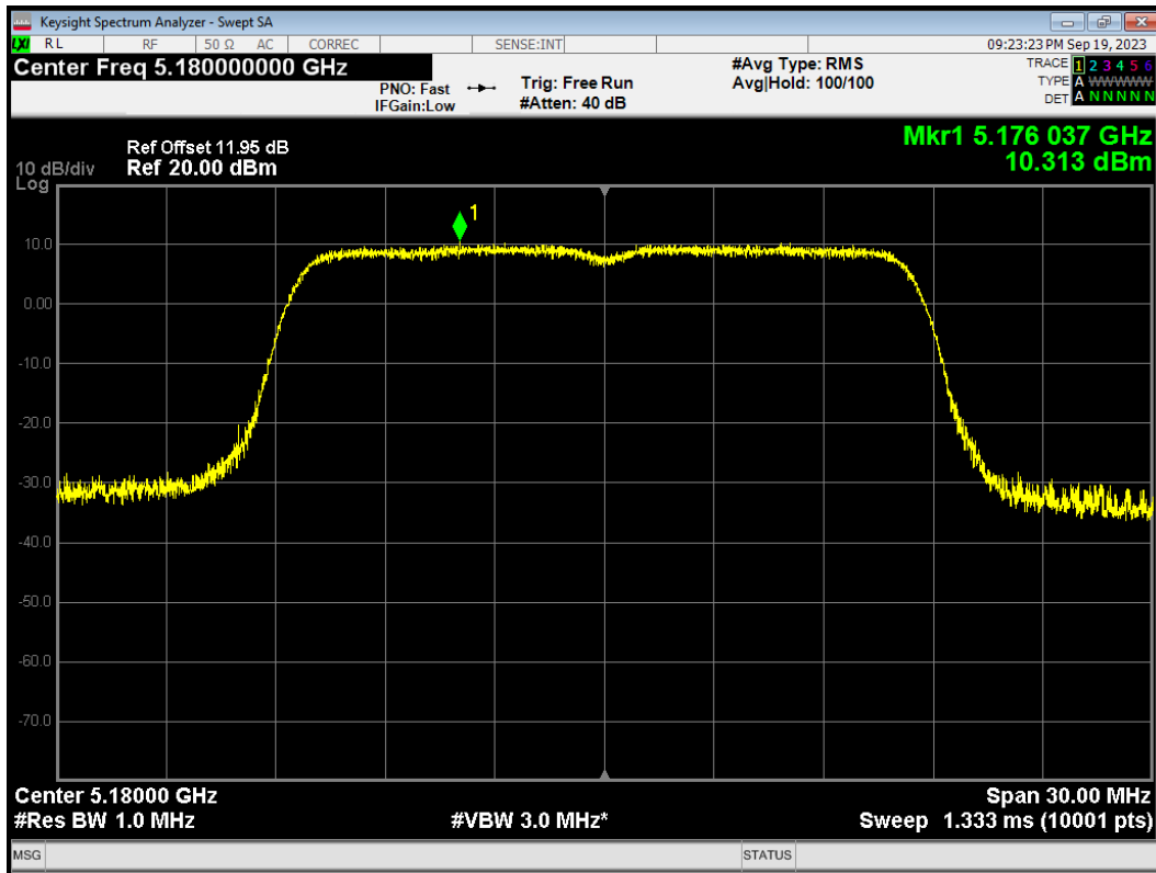
PSD 802.11a 5180MHz Ant1
