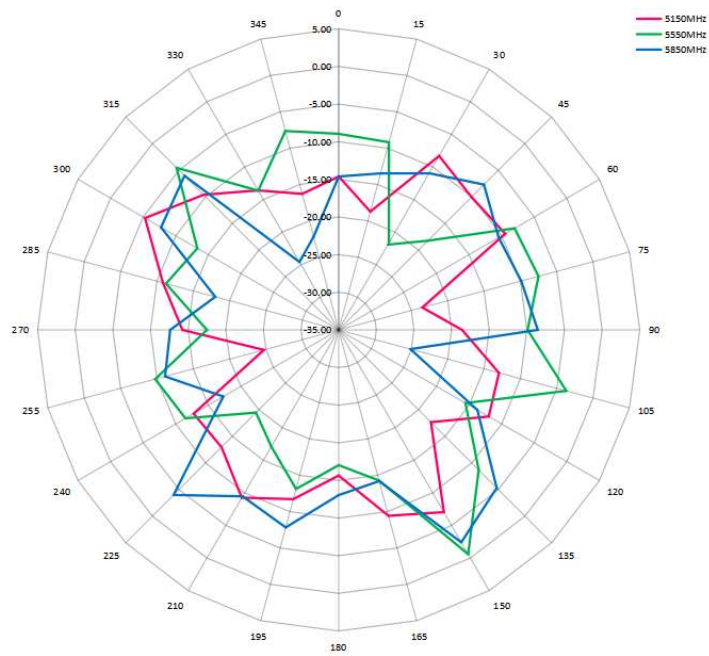
XZ_Pol_Phi_Ant.5
