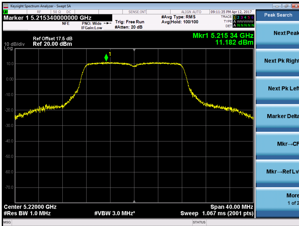
802.11a-5220MHz
