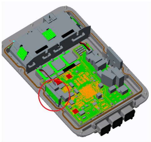
WPON AP-Pole
