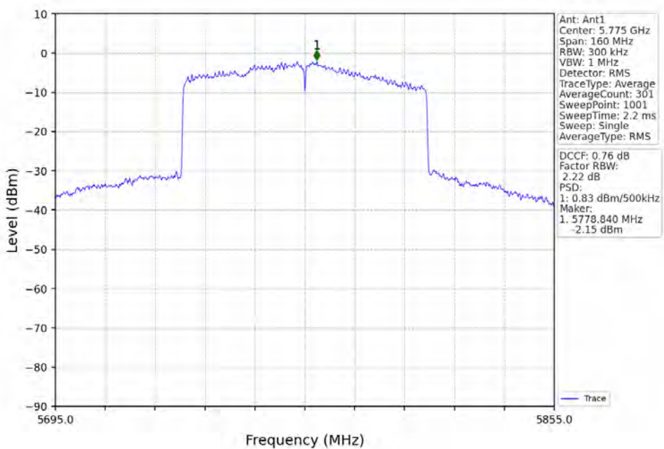
802.11ax(HEW80)_MCH_5775MHz_RU996_Left_Ant1_NTNV
