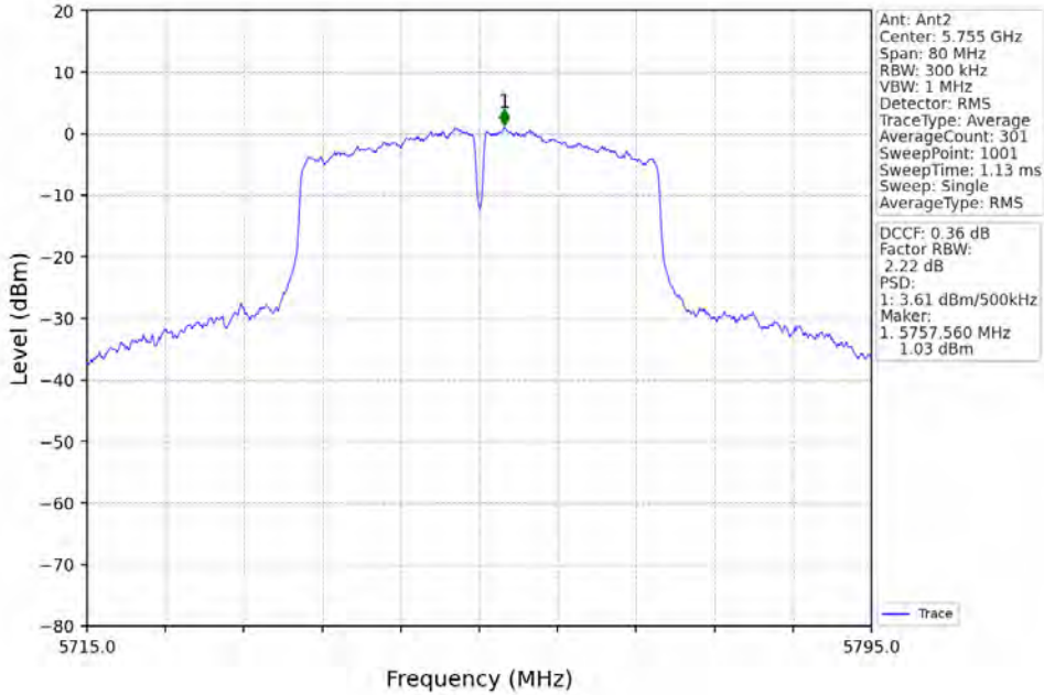
802.11ac(VHT40)_LCH_5755MHz_MIMO_NTNV
