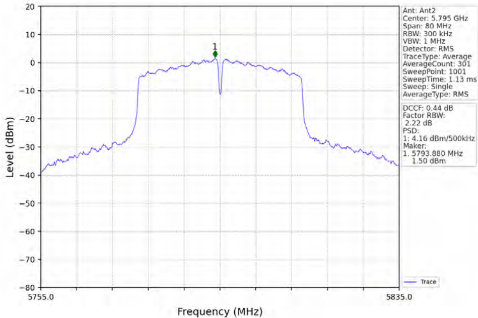
802.11n(HT40)_HCH_5795MHz_MIMO_NTNV
