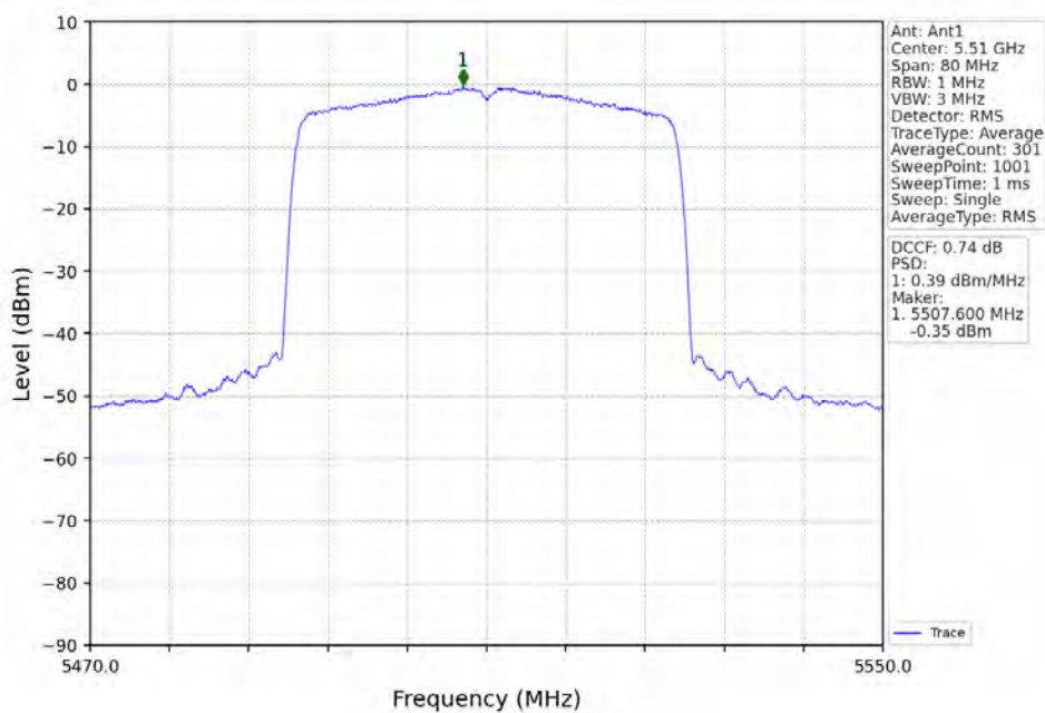
802.11ax(HEW40)_LCH_5510MHz_RU484_Left_Ant1_NTNV
