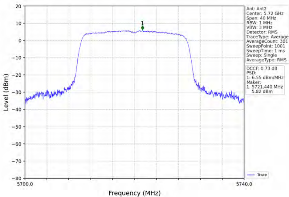
802.11ax(HEW20)_HCH_5720MHz_RU242_Left_Ant2_NTNV
