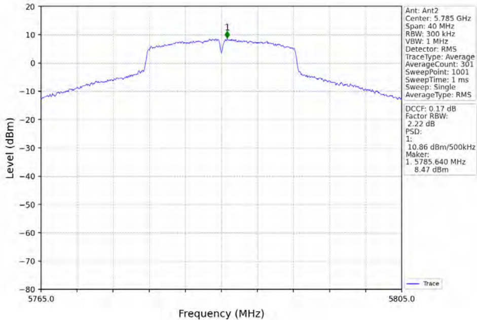
802.11a_MCH_5785MHz_MIMO_NTNV
