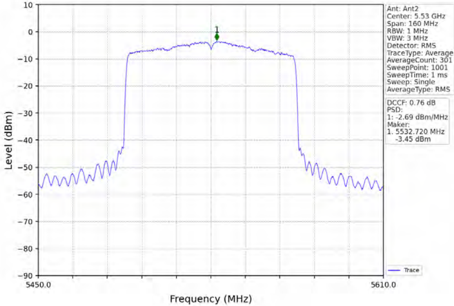
802.11ax(HEW80)_LCH_5530MHz_RU996_Left_MIMO_NTNV
