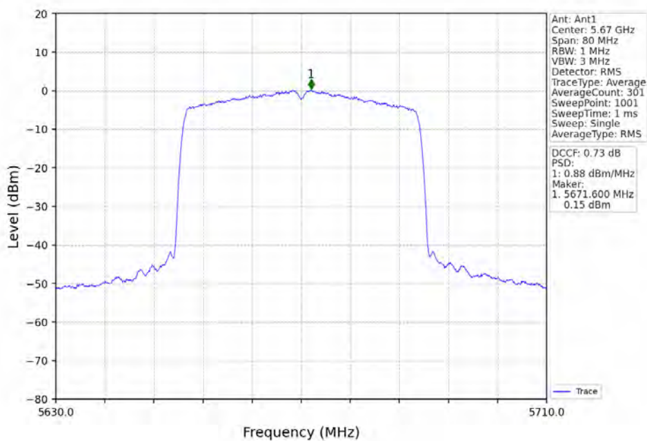
802.11ax(HEW40)_HCH_5670MHz_RU484_Left_Ant1_NTNV
