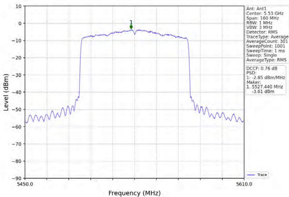
802.11ax(HEW80)_LCH_5530MHz_RU996_Left_Ant1_NTNV
