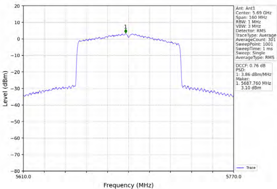
802.11ax(HEW80)_HCH_5690MHz_RU996_Left_Ant1_NTNV
