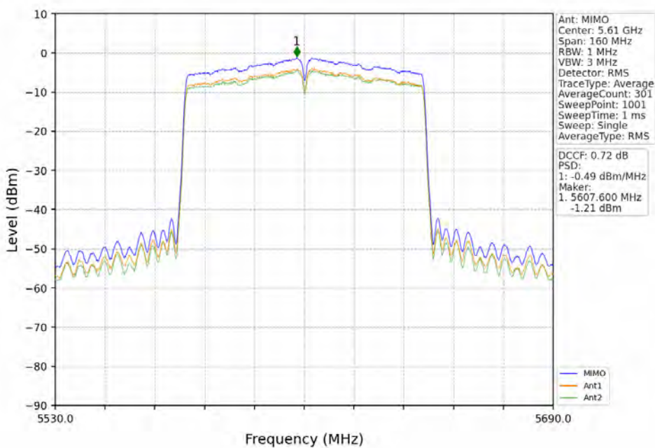
802.11ac(VHT80)_HCH_5610MHz_MIMO_NTNV
