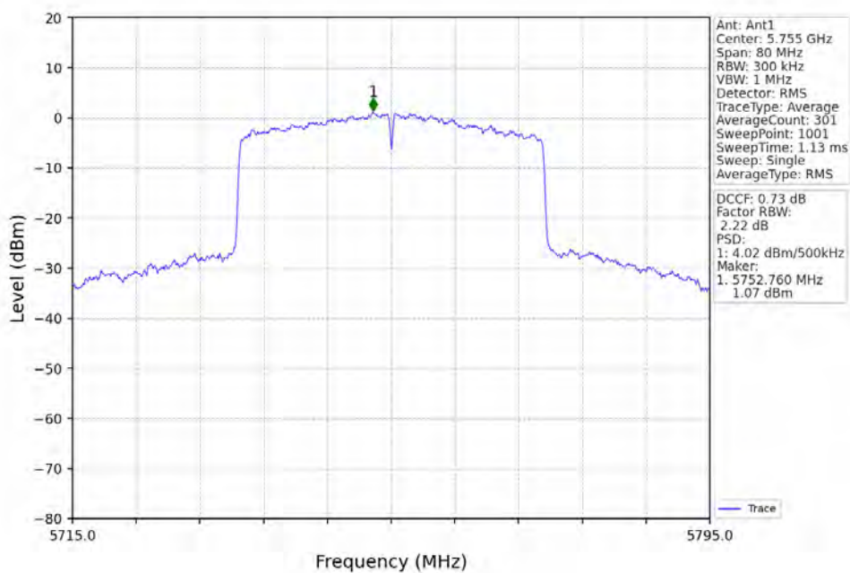
802.11ax(HEW40)_LCH_5755MHz_RU484_Left_Ant1_NTNV
