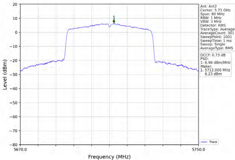
802.11ax(HEW40)_HCH_5710MHz_RU484_Left_Ant2_NTNV
