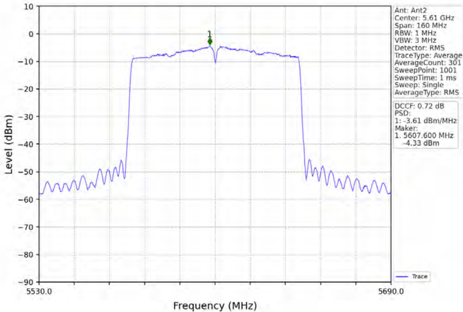
802.11ac(VHT80)_HCH_5610MHz_MIMO_NTNV
