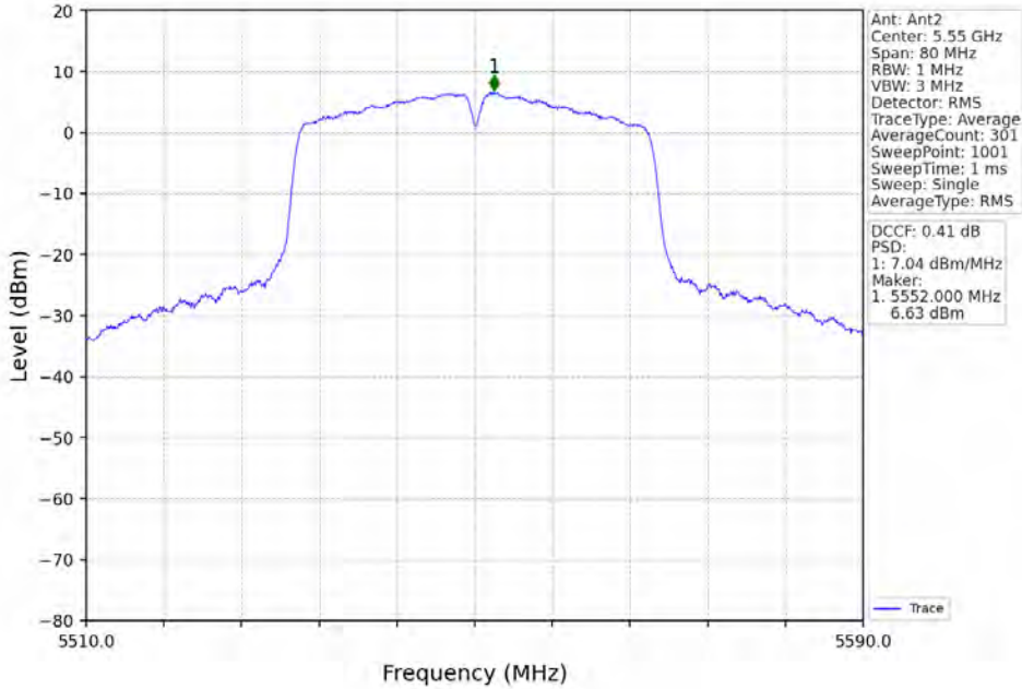
802.11n(HT40)_MCH_5550MHz_MIMO_NTNV
