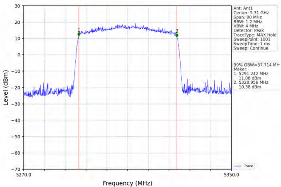
802.11ax(HEW40)_HCH_5310MHz_RU484_Left_Ant1_NTNV
