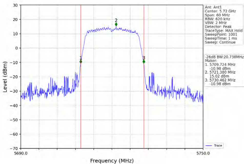
802.11ac(VHT20)_HCH_5720MHz_Ant1_NTNV
