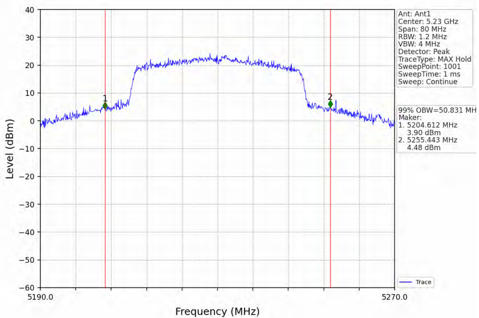
802.11ax(HEW40)_HCH_5230MHz_RU484_Left_Ant1_NTNV
