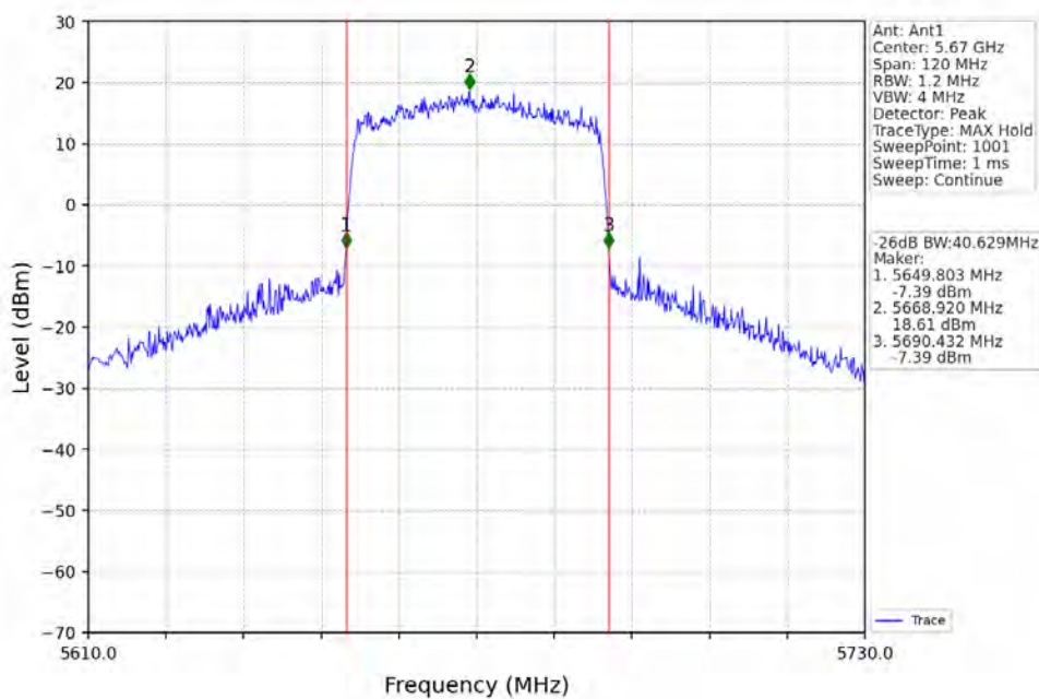
802.11ax(HEW40)_HCH_5670MHz_RU484_Left_Ant1_NTNV
