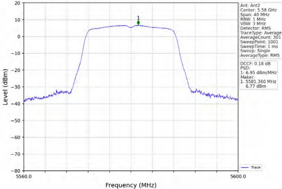
802.11a_MCH_5580MHz_MIMO_NTNV
