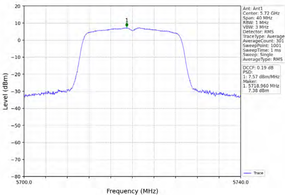
802.11n(HT20)_HCH_5720MHz_Ant1_NTNV
