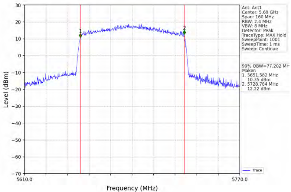
802.11ax(HEW80)_HCH_5690MHz_RU996_Left_Ant1_NTNV
