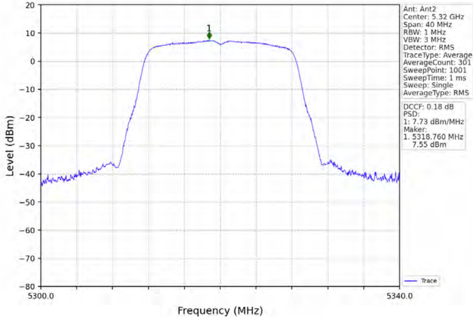
802.11a_HCH_5320MHz_MIMO_NTNV
