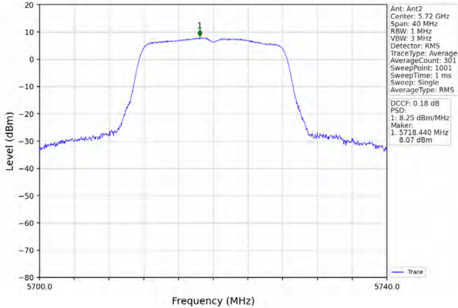
802.11a_HCH_5720MHz_MIMO_NTNV
