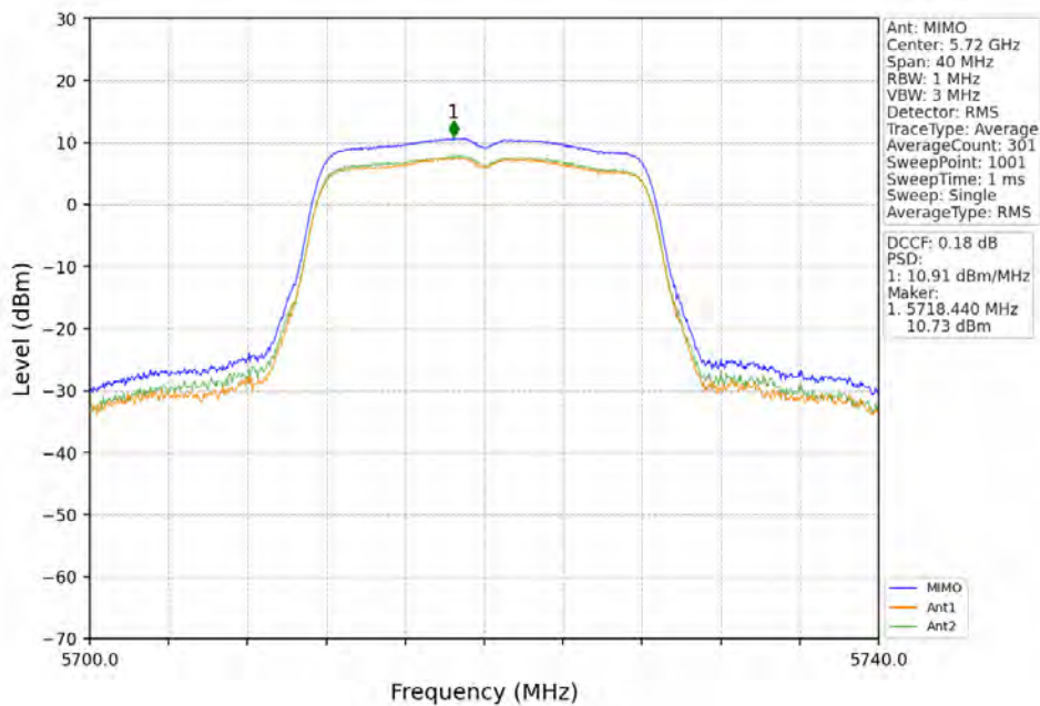
802.11a_HCH_5720MHz_MIMO_NTNV
