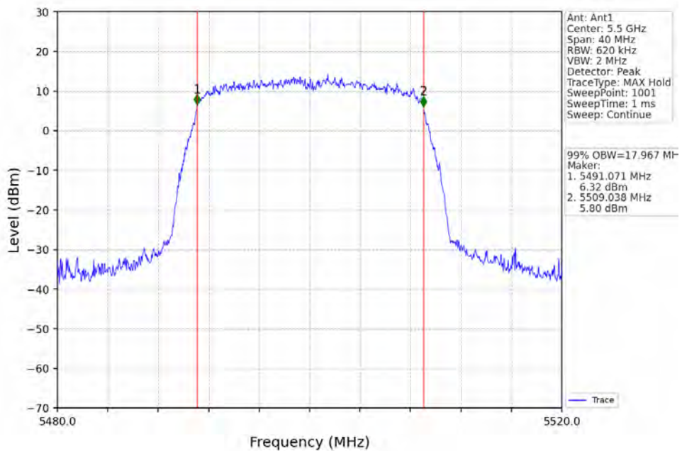
802.11n(HT20)_LCH_5500MHz_Ant1_NTNV
