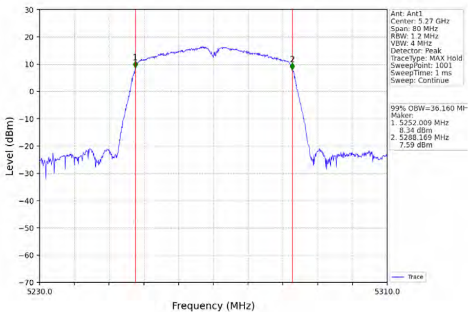
802.11ac(VHT40)_LCH_5270MHz_Ant1_NTNV
