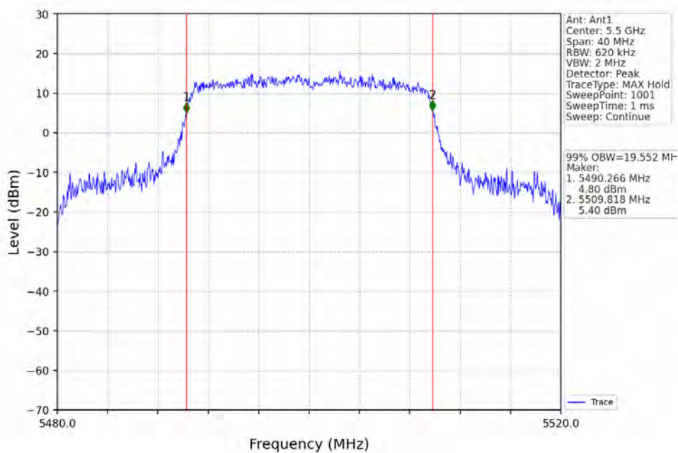
802.11ax(HEW20)_LCH_5500MHz_RU242_Left_Ant1_NTNV
