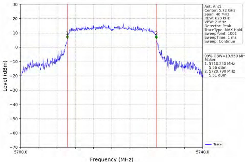
802.11ax(HEW20)_HCH_5720MHz_RU242_Left_Ant1_NTNV
