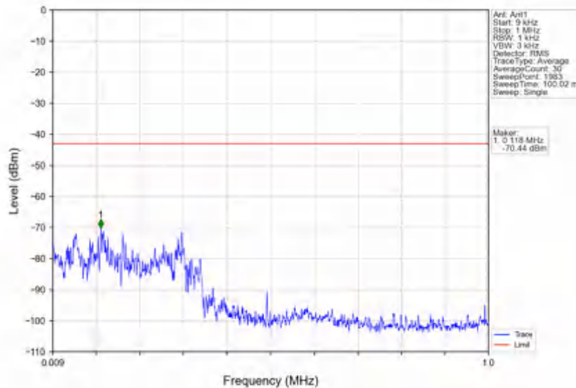
n78e_30kHz_SISO_NTNV_30MHz_DFT-s-OFDM PI/2 BPSK_3465MHz_Inner_1RB_Left
