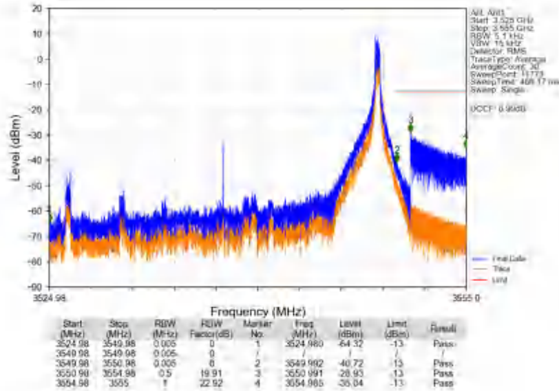
n78e_30kHz_SISO_NTV_25MHz_DFT-s-OFDM PI/2 BPSK_3537.48MHz_Inner_1RB_Right
