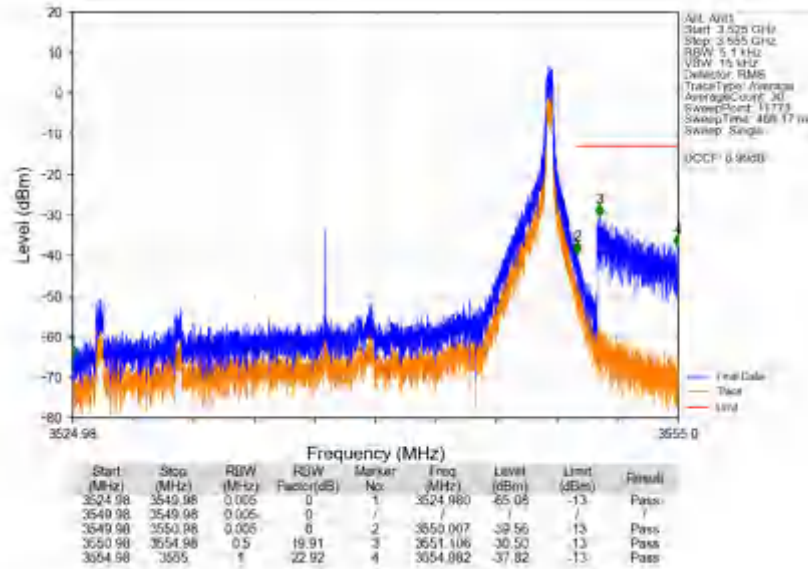
n78e_30kHz_SISO_NTV_25MHz_CP-OFDM QPSK_3537.48MHz_Inner_1RB_Right
