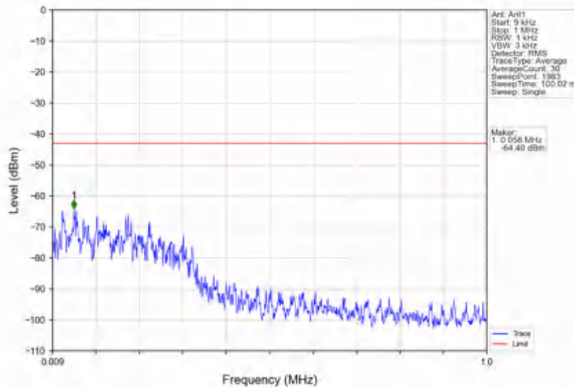
n78e_30kHz_SISO_NTV_30MHz_CP-OFDM QPSK_3465MHz_Inner_1RB_Left
