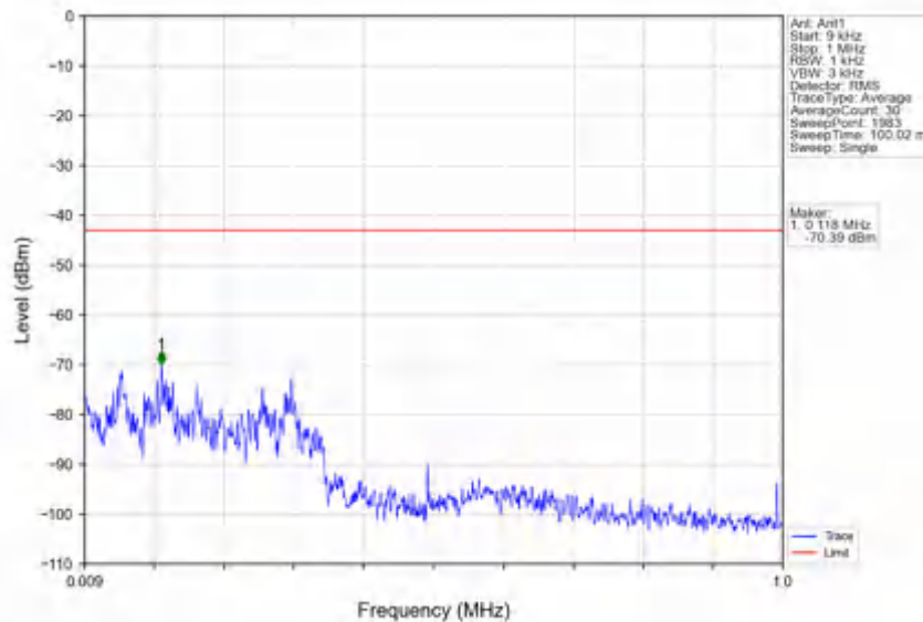
n78e_30kHz_SISO_NTV_25MHz_DFT-s-OFDM PI/2 BPSK_3537.48MHz_Inner_1RB_Right
