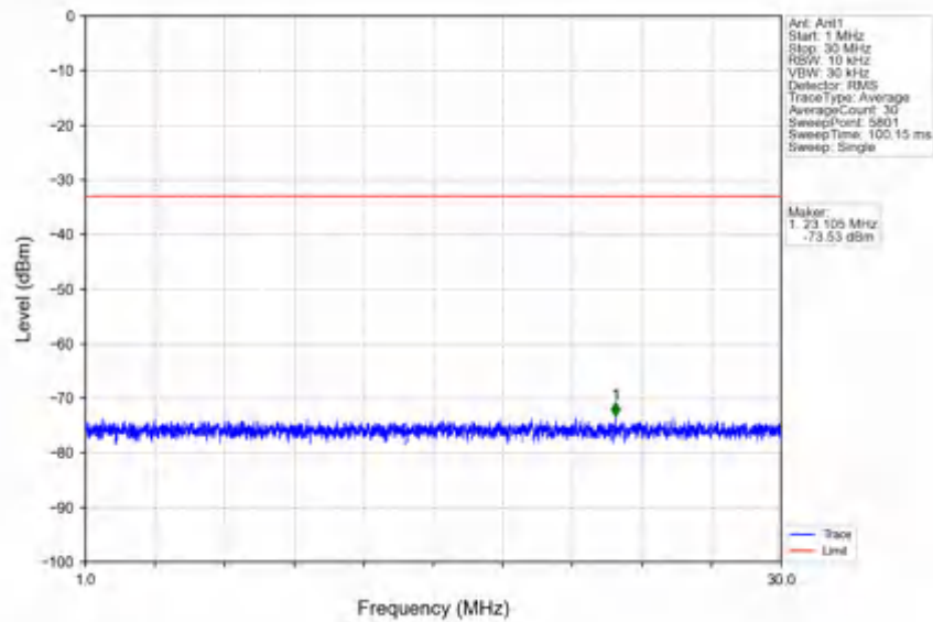
n78e_30kHz_SISO_NTV_25MHz_CP-OFDM QPSK_3537.48MHz_Inner_1RB_Right
