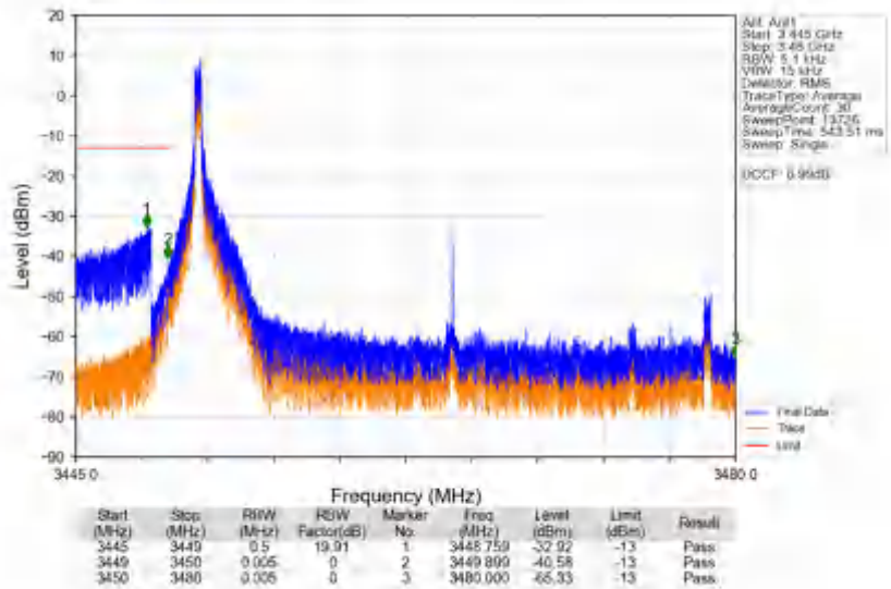
n78e_30kHz_SISO_NTNV_30MHz_DFT-s-OFDM QPSK_3465MHz_Inner_1RB_Left
