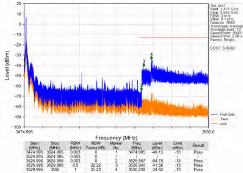
n78e_15kHz_SISO_NTNV_50MHz_DFT-s-OFDM QPSK_3499.995MHz_Edge_1RB_Left
