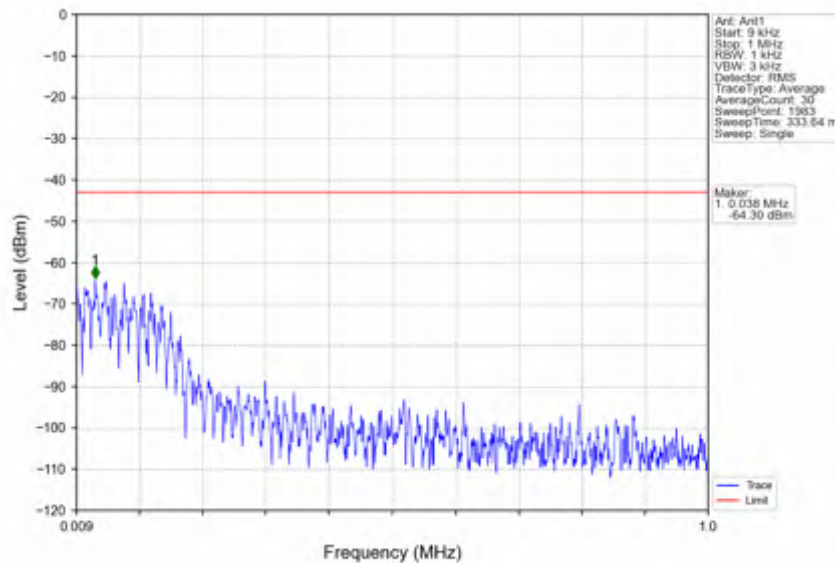
n78e_15kHz_SISO_NTVV_40MHz_CP-OFDM_QPSK_3470.01MHz_Inner_1RB_Left
