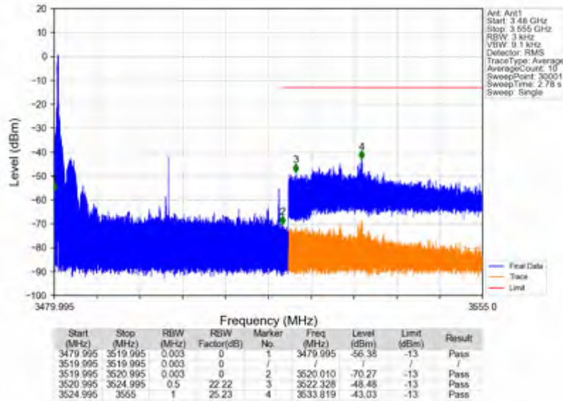
n78e_15kHz_SISO_NTV_40MHz_CP-OFDM QPSK_3499.995MHz_Edge_1RB_Left
