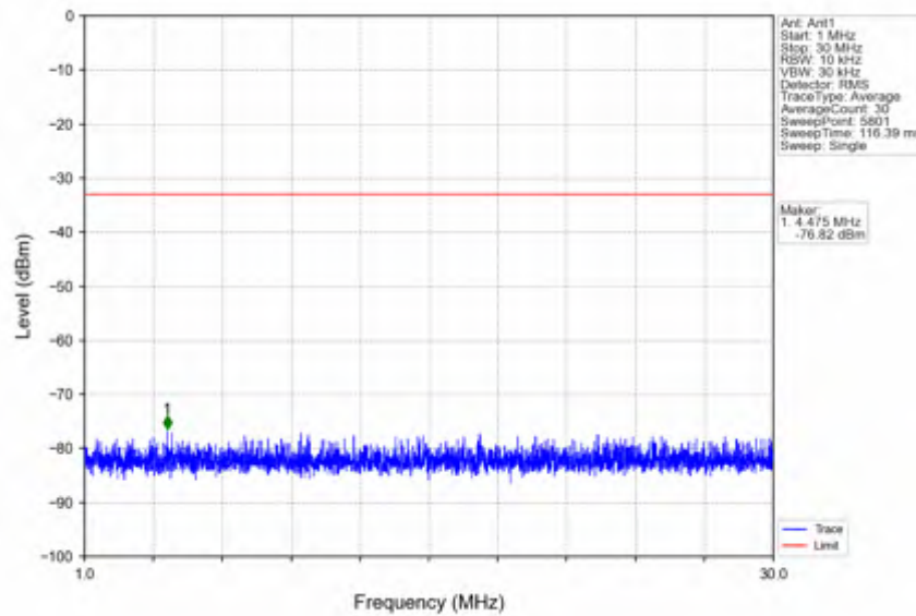
n78e_30kHz_SISO_NTNV_10MHz_CP-OFDM QPSK_3455.01MHz_Inner_1RB_Left
