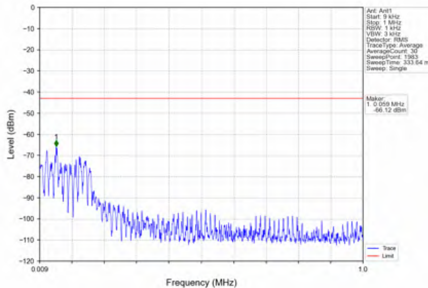
n78e_15kHz_SISO_NTV_50MHz_DFT-s-OFDM PI/2 BPSK_3475.005MHz_Inner_1RB_Left
