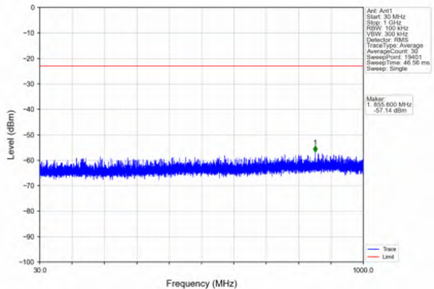
n78e_15kHz_SISO_NTNV_50MHz_DFT-s-OFDM QPSK_3499.995MHz_Edge_1RB_Left
