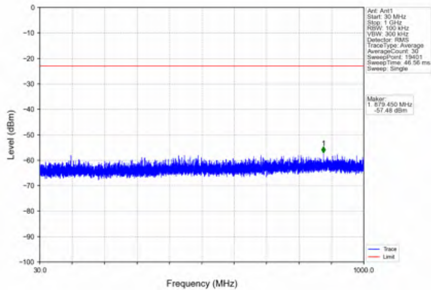
n78e_15kHz_SISO_NTNV_40MHz_CP-OFDM QPSK_3499.995MHz_Edge_1RB_Left
