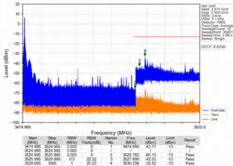
n78e_15kHz_SISO_NTNV_50MHz_DFT-s-OFDM PI/2 BPSK_3499.995MHz_Edge_1RB_Left
