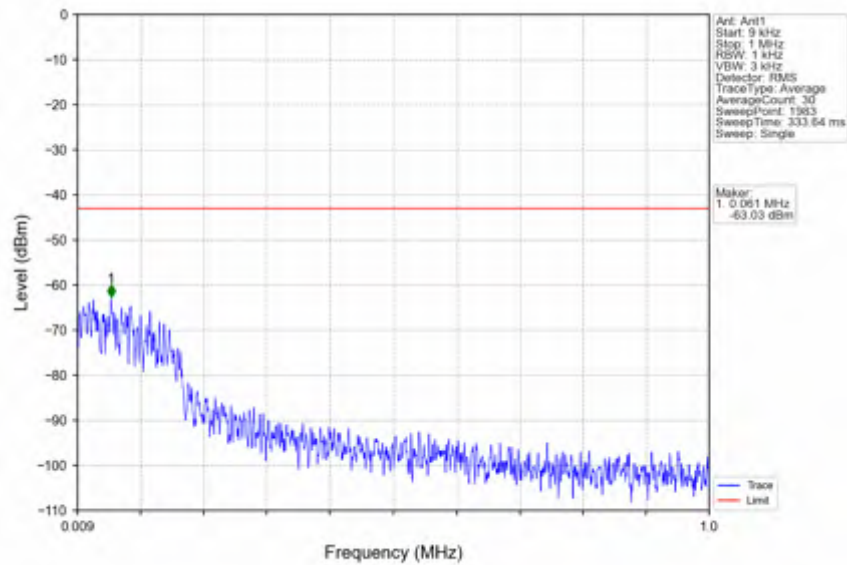
n78e_15kHz_SISO_NTNV_50MHz_CP-OFDM QPSK_3499.995MHz_Edge_1RB_Left
