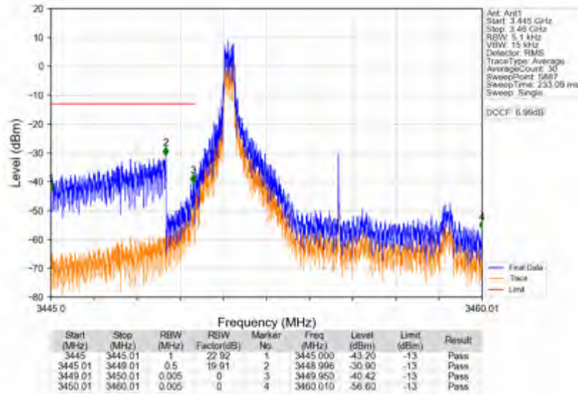
n78e_30kHz_SISO_NTNV_10MHz_CP-OFDM QPSK_3455.01MHz_Inner_1RB_Left
