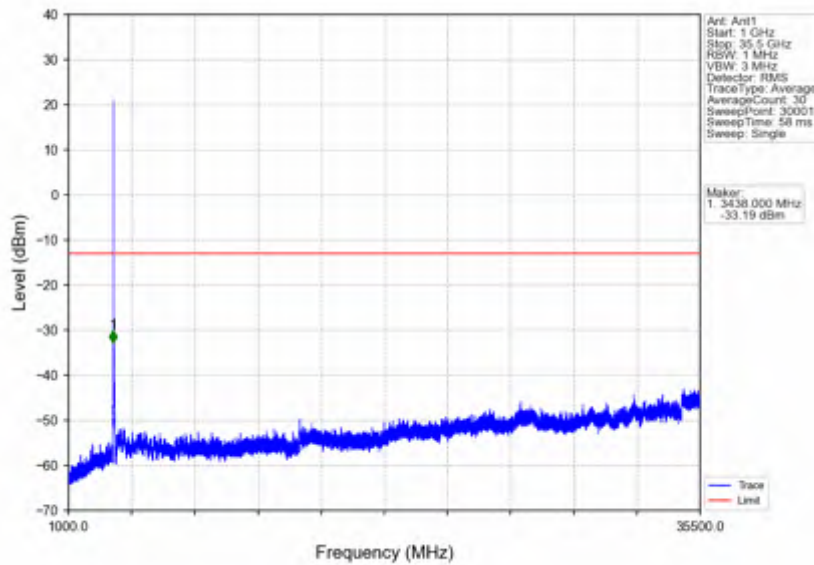
n78e_15kHz_SISO_NTV_40MHz_CP-OFDM QPSK_3499.995MHz_Edge_1RB_Left
