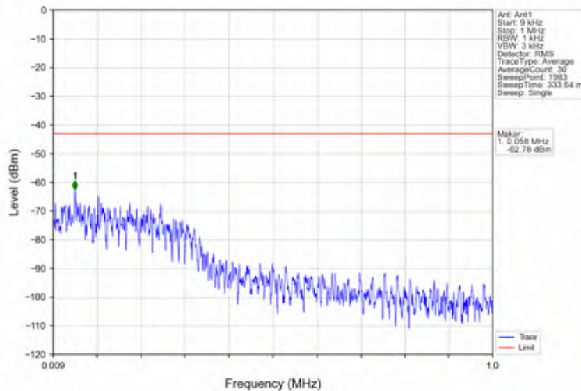
n78e_30kHz_SISO_NTNV_10MHz_CP-OFDM QPSK_3455.01MHz_Inner_1RB_Left
