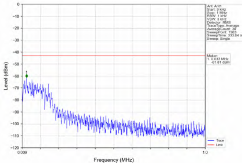
n78e_15kHz_SISO_NTNV_50MHz_CP-OFDM QPSK_3475.005MHz_Inner_1RB_Left
