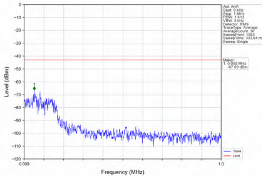
n78e_15kHz_SISO_NTNV_50MHz_DFT-s-OFDM PI/2 BPSK_3499.995MHz_Edge_1RB_Left
