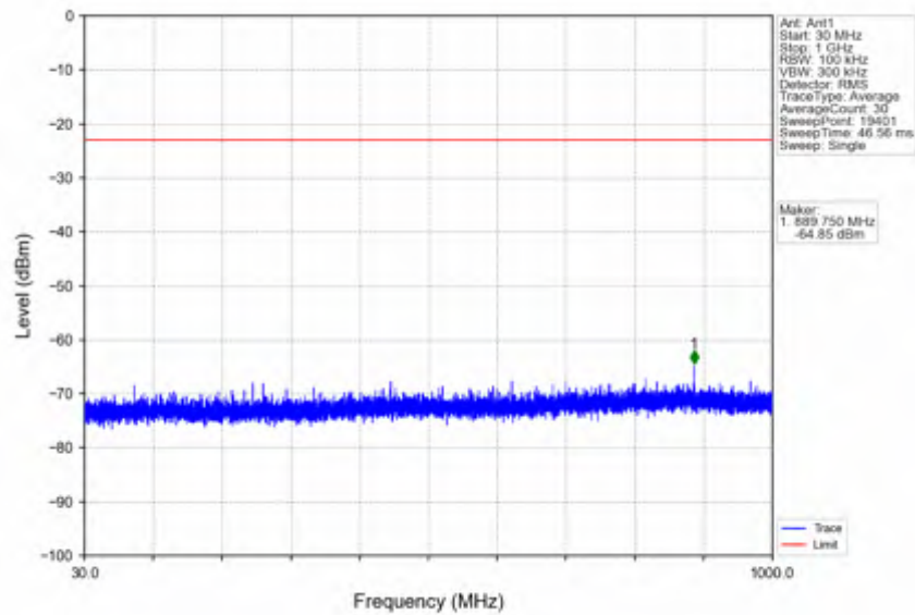
n78e_15kHz_SISO_NTNV_50MHz_DFT-s-OFDM QPSK_3475.005MHz_Inner_1RB_Left
