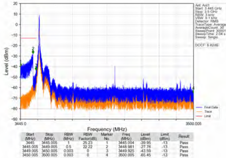
n78e_15kHz_SISO_NTNV_50MHz_CP-OFDM QPSK_3475.005MHz_Inner_1RB_Left
