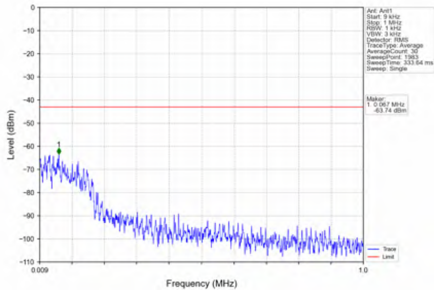
n78e_15kHz_SISO_NTNV_40MHz_CP-OFDM QPSK_3499.995MHz_Edge_1RB_Left
