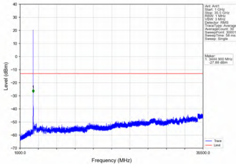
n78e_15kHz_SISO_NTNV_50MHz_DFT-s-OFDM PI/2 BPSK_3499.995MHz_Edge_1RB_Left
