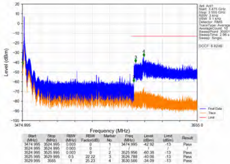
n78e_15kHz_SISO_NTNV_50MHz_CP-OFDM QPSK_3499.995MHz_Edge_1RB_Left
