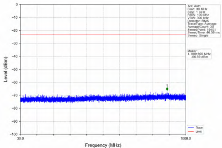
n78e_15kHz_SISO_NTNV_40MHz_CP-OFDM QPSK_3470.01MHz_Inner_1RB_Left
