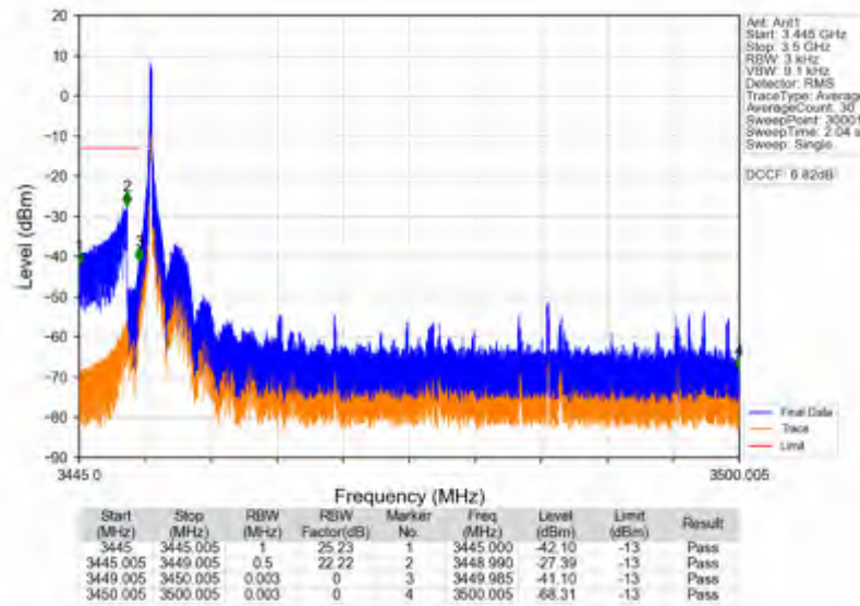
n78e_15kHz_SISO_NTV_50MHz_DFT-s-OFDM PI/2 BPSK_3475.005MHz_Inner_1RB_Left
