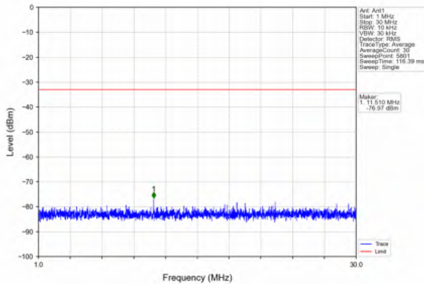
n78e_15kHz_SISO_NTNV_50MHz_CP-OFDM QPSK_3475.005MHz_Inner_1RB_Left
