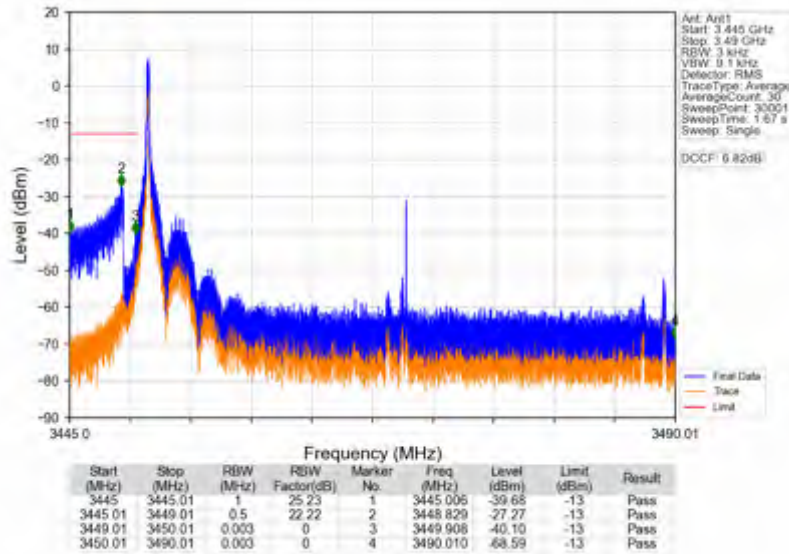
n78e_15kHz_SISO_NTVV_40MHz_CP-OFDM_QPSK_3470.01MHz_Inner_1RB_Left
