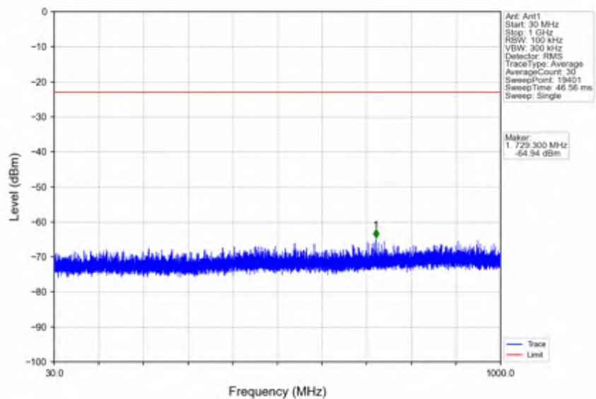
n78e_30kHz_SISO_NTNV_10MHz_DFT-s-OFDM PI/2 BPSK_3455.01MHz_Inner_1RB_Left
