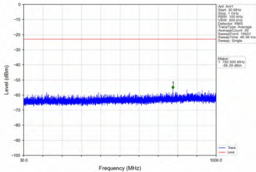
n78e_15kHz_SISO_NTNV_50MHz_CP-OFDM QPSK_3499.995MHz_Edge_1RB_Left
