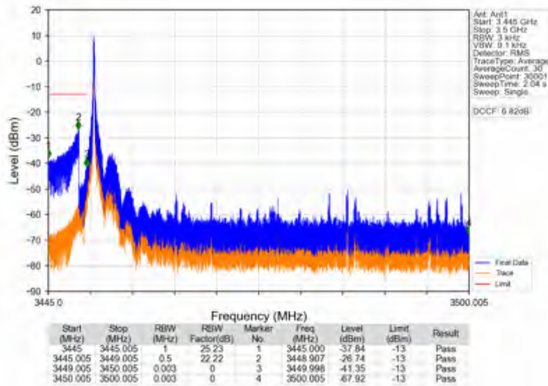
n78e_15kHz_SISO_NTNV_50MHz_DFT-s-OFDM QPSK_3475.005MHz_Inner_1RB_Left
