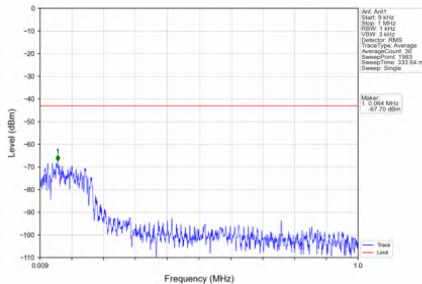
n78e_15kHz_SISO_NTNV_50MHz_DFT-s-OFDM QPSK_3499.995MHz_Edge_1RB_Left
