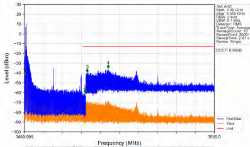
n78e_15kHz_SISO_NTNV_20MHz_CP-OFDM QPSK_3499.995MHz_Edge_1RB_Left
