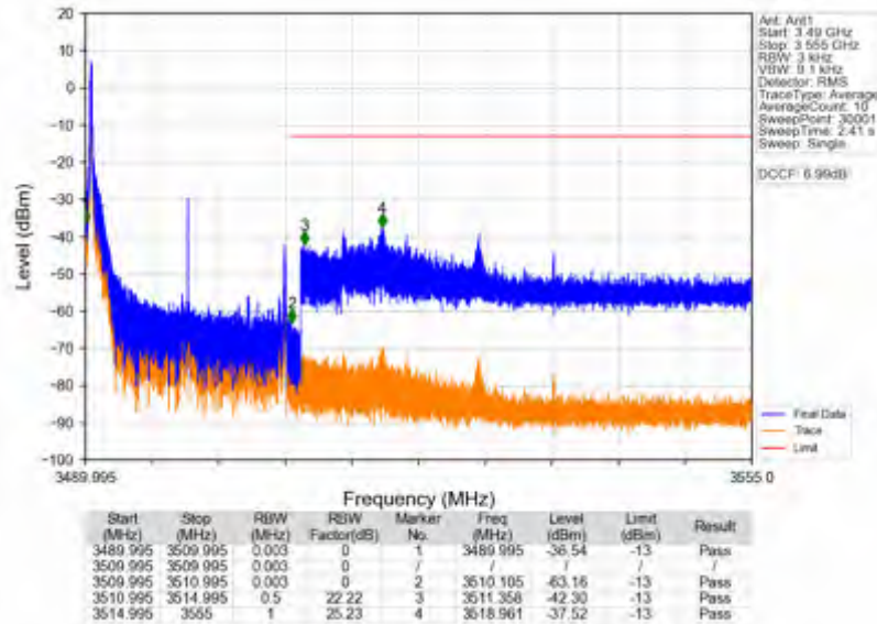
n78e_15kHz_SISO_NTNV_20MHz_DFT-s-OFDM QPSK_3499.995MHz_Edge_1RB_Left
