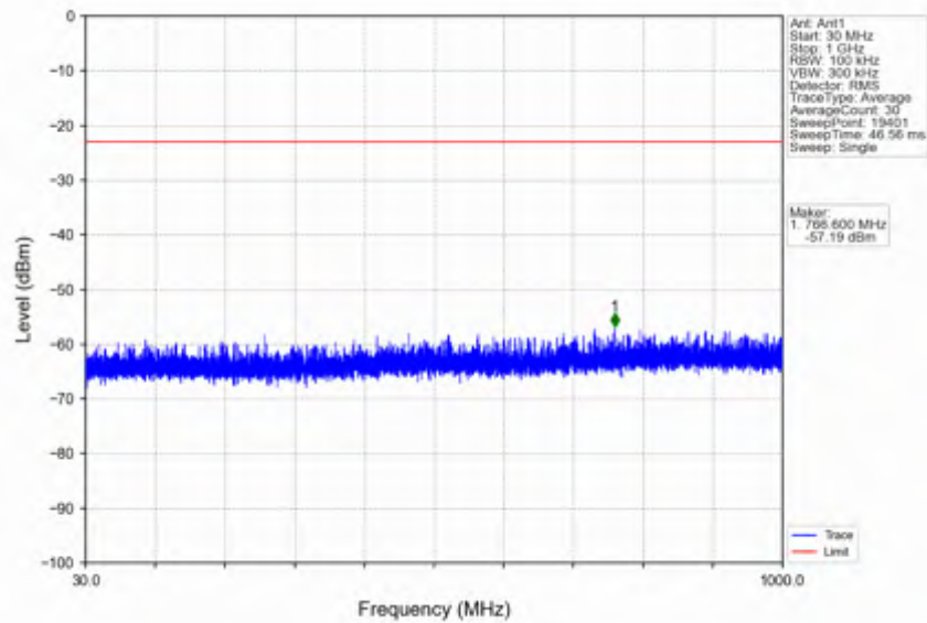
n78e_15kHz_SISO_NTNV_40MHz_DFT-s-OFDM PI/2 BPSK_3499.995MHz_Edge_1RB_Left
