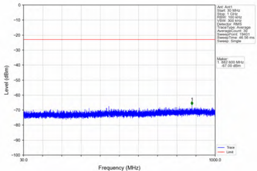
n78e_15kHz_SISO_NTNV_20MHz_DFT-s-OFDM_PI/2_BPSK_3540MHz_Inner_1RB_Right
