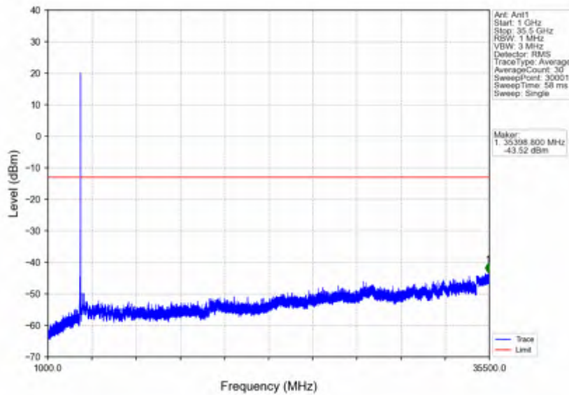
n78e_15kHz_SISO_NTV_30MHz_DFT-s-OFDM QPSK_3465MHz_Edge_1RB_Left
