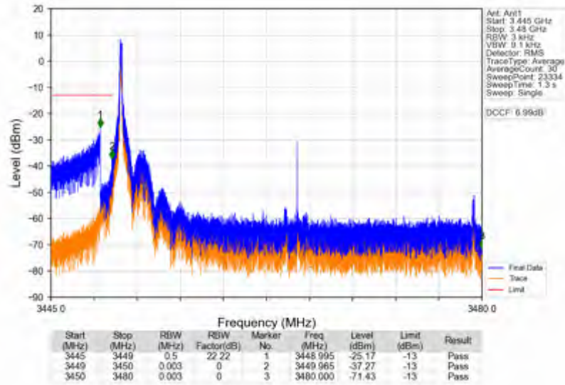
n78e_15kHz_SISO_NTNV_30MHz_CP-OFDM QPSK_3465MHz_Edge_1RB_Left
