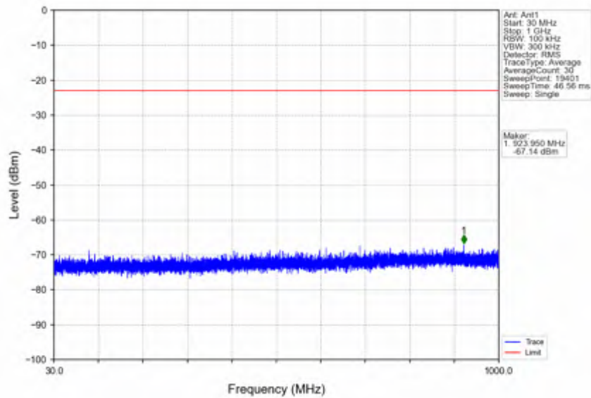
n78e_15kHz_SISO_NTV_30MHz_DFT-s-OFDM QPSK_3465MHz_Inner_1RB_Left
