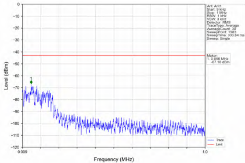
n78e_15kHz_SISO_NTNV_20MHz_DFT-s-OFDM PI/2 BPSK_3499.995MHz_Edge_1RB_Left
