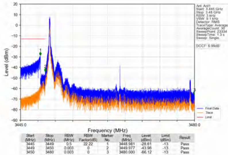
n78e_15kHz_SISO_NTV_30MHz_CP-OFDM_QPSK_3465MHz_Inner_1RB_Left
