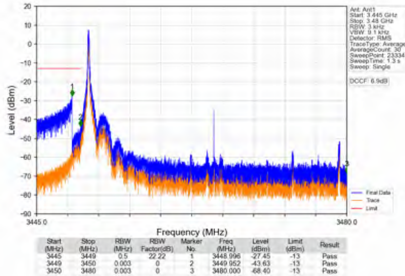
n78e_15kHz_SISO_NTNV_30MHz_DFT-s-OFDM PI/2 BPSK_3465MHz_Inner_1RB_Left
