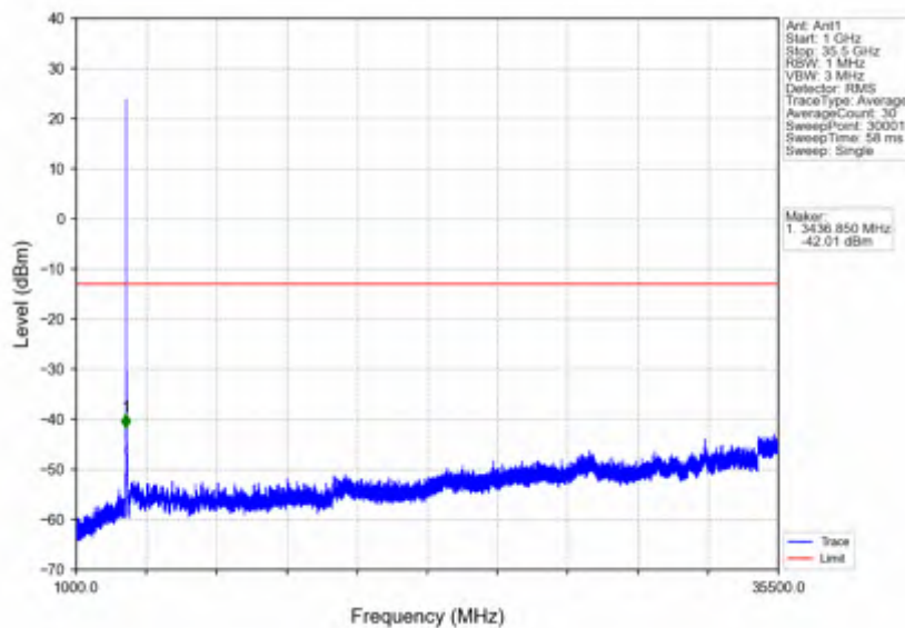
n78e_15kHz_SISO_NTV_30MHz_DFT-s-OFDM QPSK_3465MHz_Inner_1RB_Left
