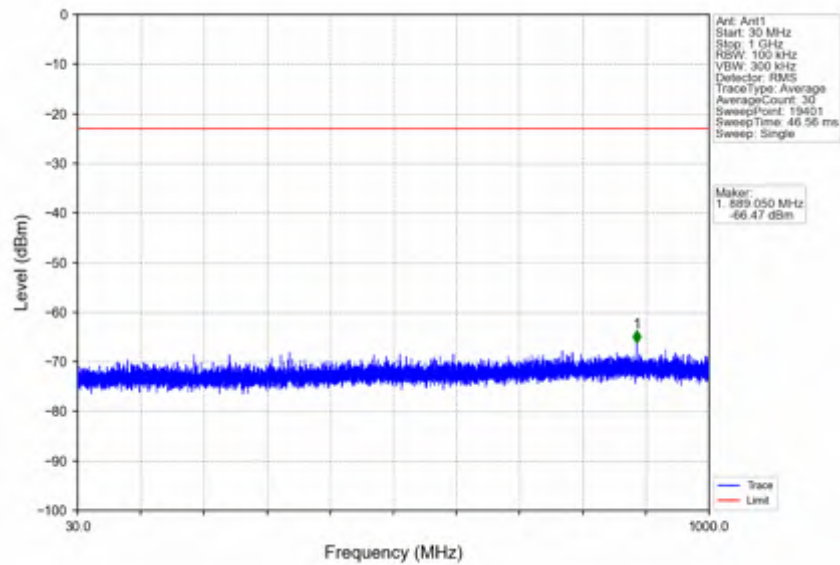
n78e_15kHz_SISO_NTNV_20MHz_DFT-s-OFDM QPSK_3460.005MHz_Inner_1RB_Left
