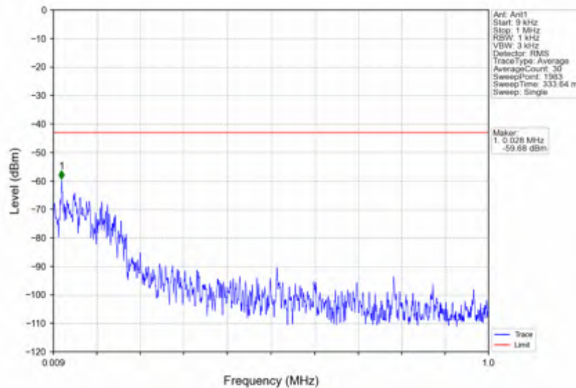
n78e_15kHz_SISO_NTV_30MHz_CP-OFDM_QPSK_3465MHz_Inner_1RB_Left
