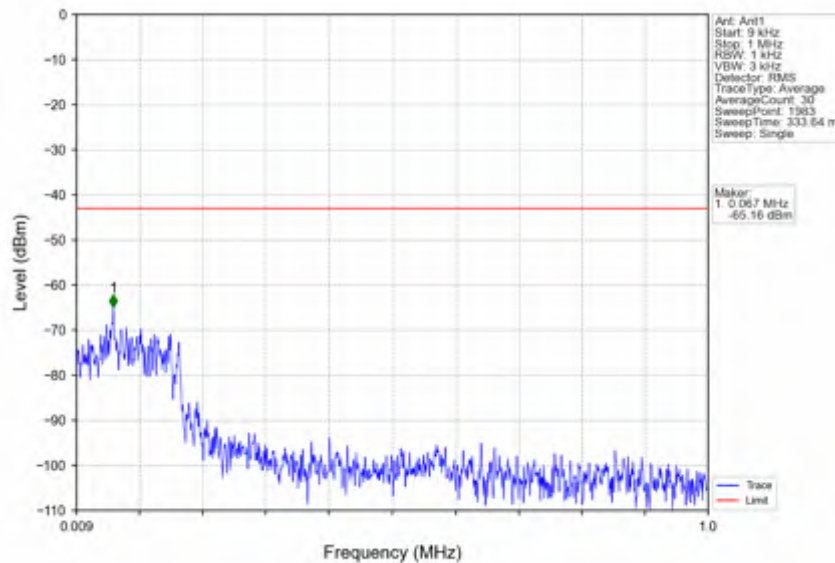
n78e_15kHz_SISO_NTNV_40MHz_DFT-s-OFDM QPSK_3499.995MHz_Edge_1RB_Left
