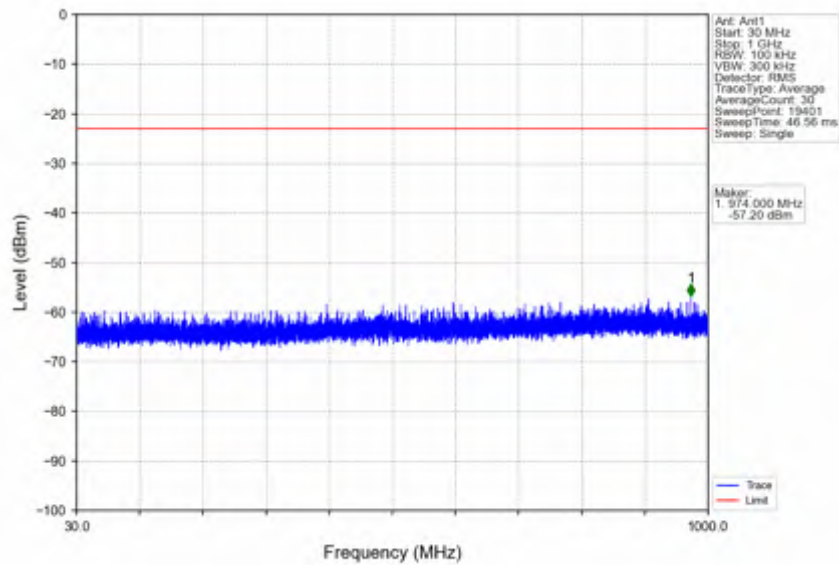
n78e_15kHz_SISO_NTV_30MHz_DFT-s-OFDM QPSK_3465MHz_Edge_1RB_Left
