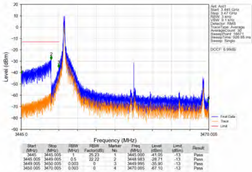
n78e_15kHz_SISO_NTNV_20MHz_DFT-s-OFDM QPSK_3460.005MHz_Inner_1RB_Left
