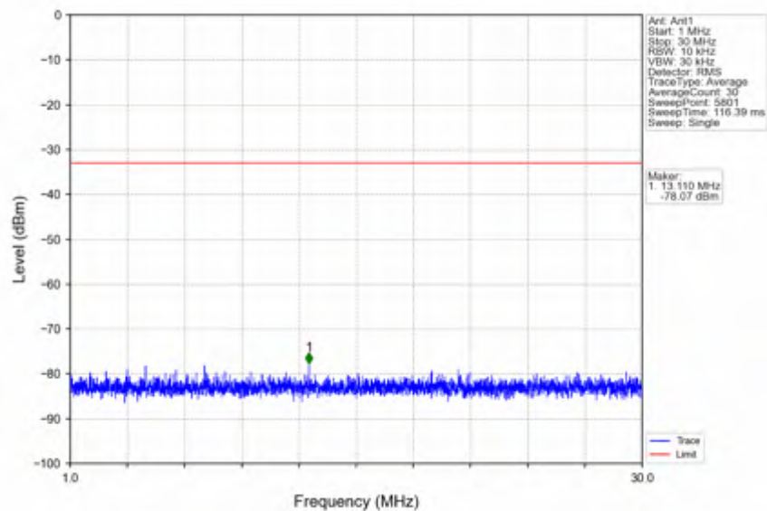
n78e_15kHz_SISO_NTNV_20MHz_DFT-s-OFDM QPSK_3460.005MHz_Inner_1RB_Left
