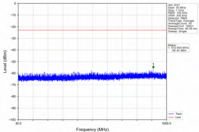
n78e_15kHz_SISO_NTNV_40MHz_DFT-s-OFDM QPSK_3499.995MHz_Edge_1RB_Left
