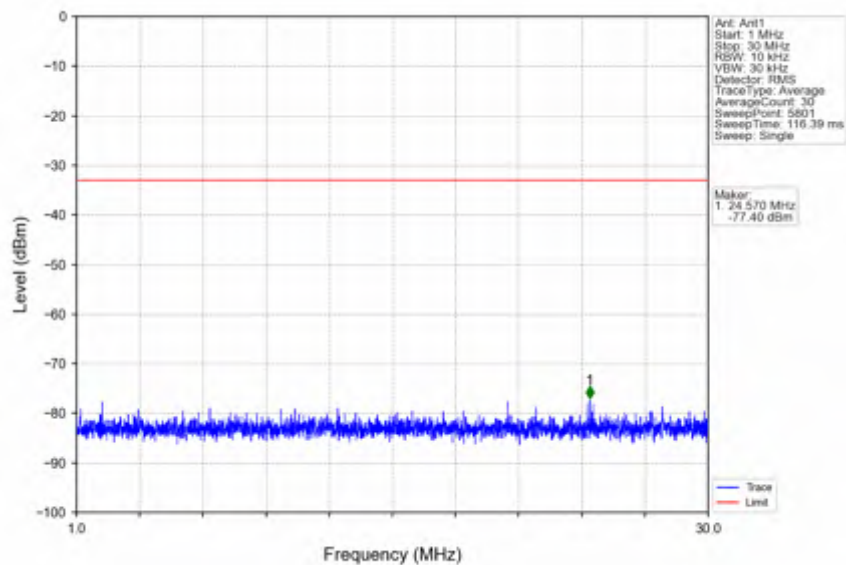
n78e_15kHz_SISO_NTV_30MHz_DFT-s-OFDM QPSK_3465MHz_Inner_1RB_Left
