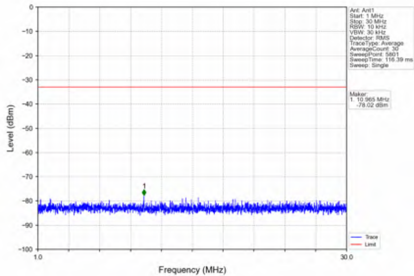
n78e_15kHz_SISO_NTNV_40MHz_DFT-s-OFDM PI/2 BPSK_3470.01MHz_Inner_1RB_Left
