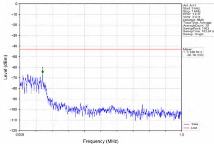
n78e_15kHz_SISO_NTNV_20MHz_DFT-s-OFDM QPSK_3499.995MHz_Edge_1RB_Left
