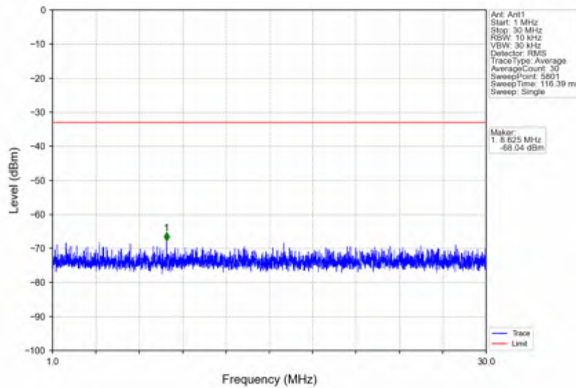
n78e_15kHz_SISO_NTNV_20MHz_DFT-s-OFDM_PI/2_BPSK_3460.005MHz_Edge_1RB_Left
