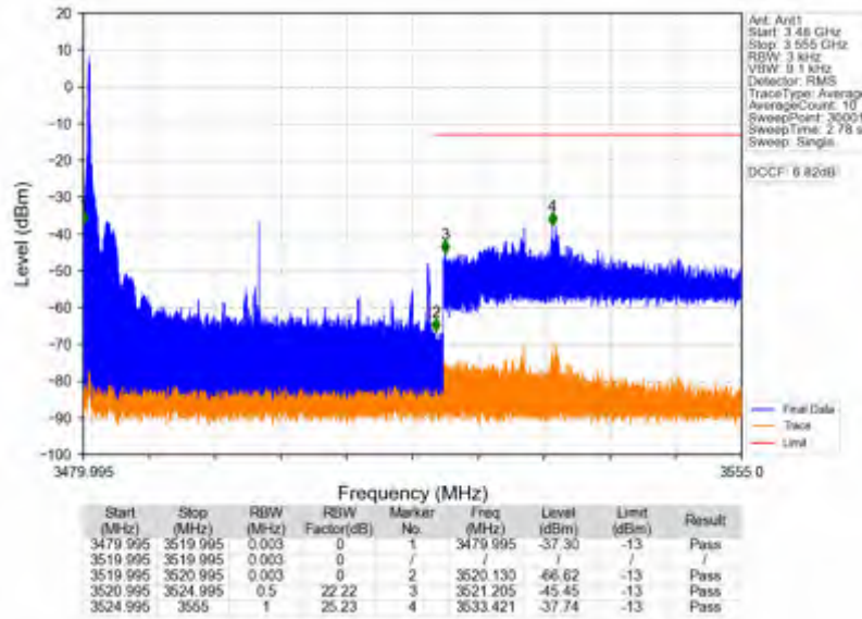
n78e_15kHz_SISO_NTNV_40MHz_DFT-s-OFDM QPSK_3499.995MHz_Edge_1RB_Left
