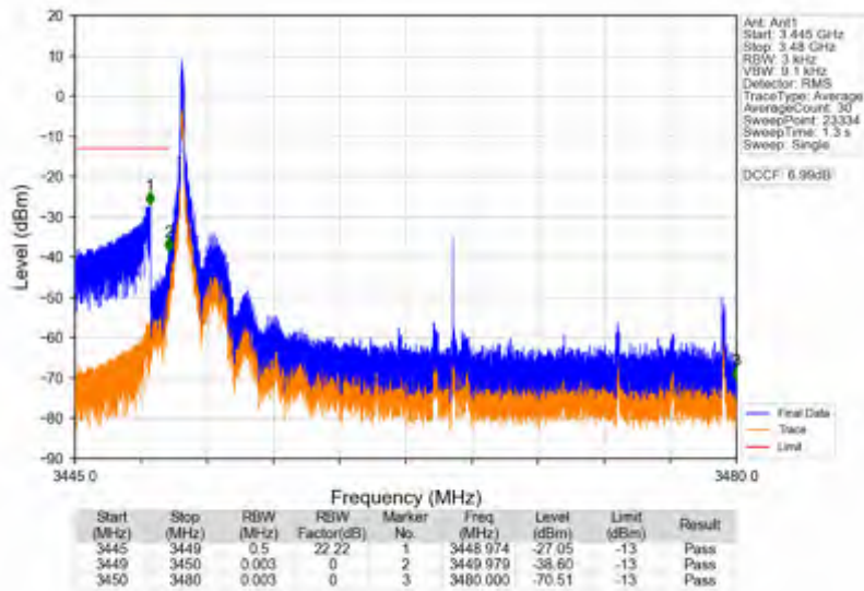
n78e_15kHz_SISO_NTV_30MHz_DFT-s-OFDM QPSK_3465MHz_Edge_1RB_Left
