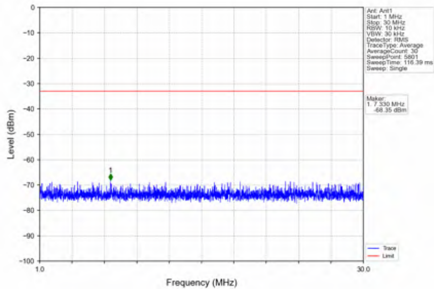
n78e_15kHz_SISO_NTNV_30MHz_CP-OFDM QPSK_3465MHz_Edge_1RB_Left
