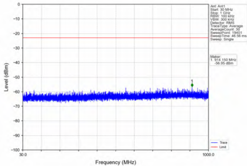
n78e_15kHz_SISO_NTNV_30MHz_CP-OFDM QPSK_3499.995MHz_Edge_1RB_Left
