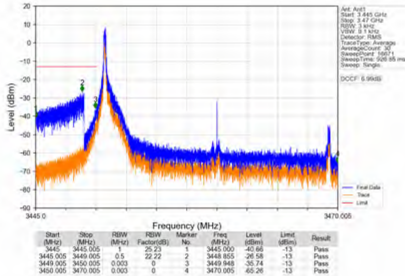
n78e_15kHz_SISO_NTNV_20MHz_CP-OFDM QPSK_3460.005MHz_Inner_1RB_Left
