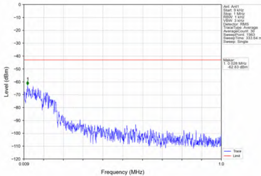
n78e_15kHz_SISO_NTNV_20MHz_CP-OFDM QPSK_3460.005MHz_Inner_1RB_Left
