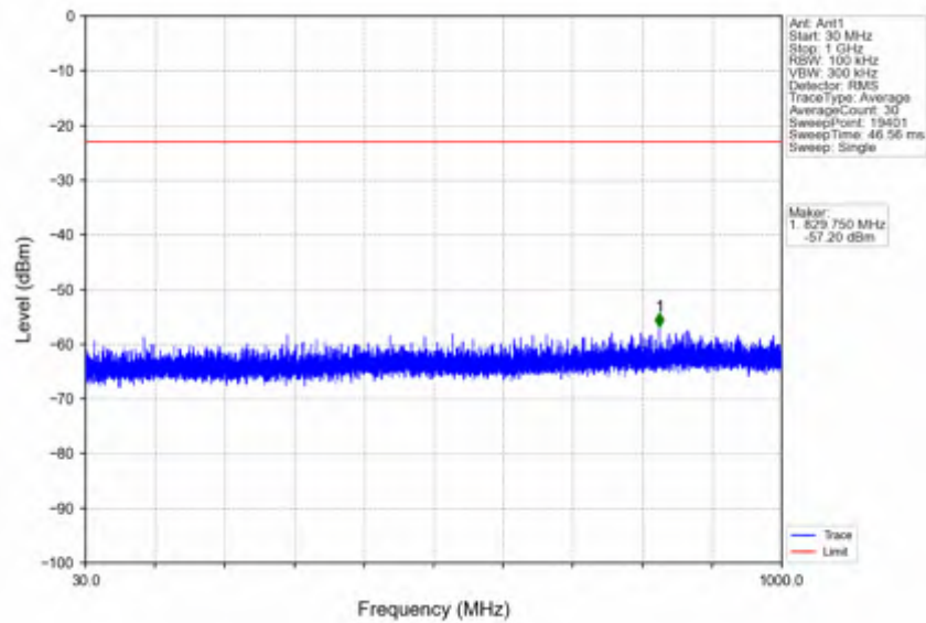
n78e_15kHz_SISO_NTNV_20MHz_CP-OFDM QPSK_3499.995MHz_Edge_1RB_Left
