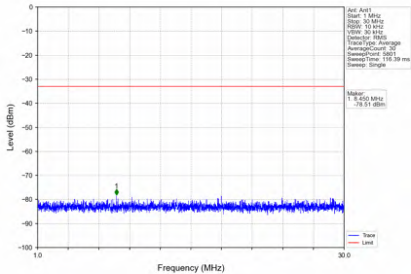
n78e_15kHz_SISO_NTNV_10MHz_CP-OFDM QPSK_3455.01MHz_Inner_1RB_Left
