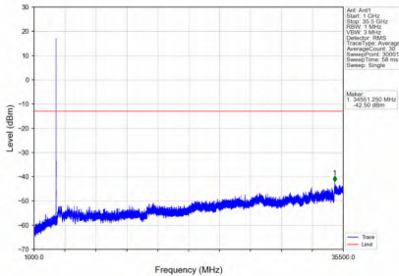
n78e_15kHz_SISO_NTNV_10MHz_DFT-s-OFDM PI/2 BPSK_3499.995MHz_Edge_1RB_Left
