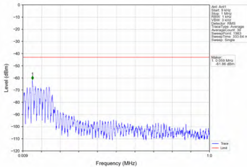
n78e_15kHz_SISO_NTNV_10MHz_DFT-s-OFDM QPSK_3499.995MHz_Edge_1RB_Left
