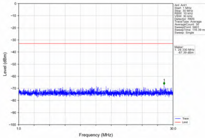
n78e_15kHz_SISO_NTNV_10MHz_DFT-s-OFDM QPSK_3499.995MHz_Edge_1RB_Left
