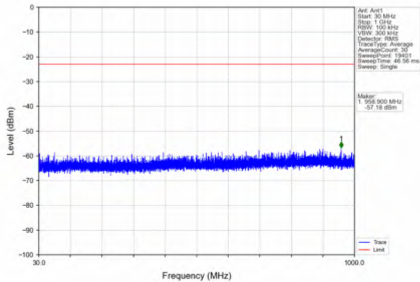
n78e_15kHz_SISO_NTNV_10MHz_CP-OFDM QPSK_3499.995MHz_Edge_1RB_Left
