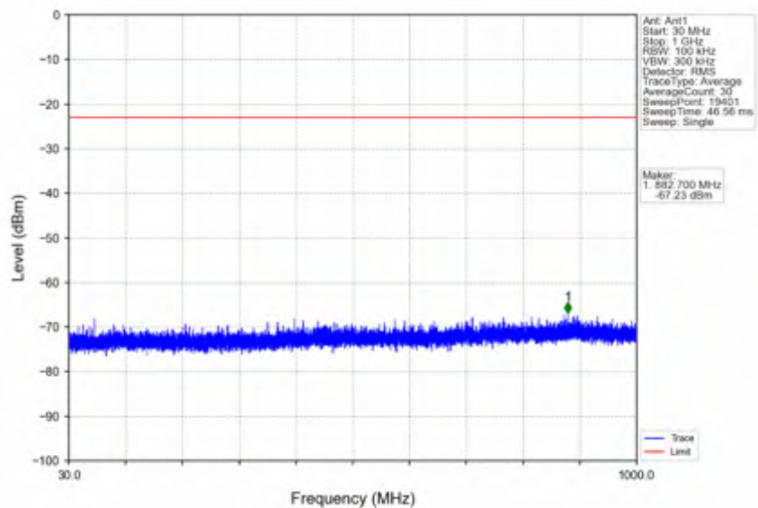
n78e_15kHz_SISO_NTNV_15MHz_DFT-s-OFDM_PI/2_BPSK_3457.5MHz_Inner_1RB_Left
