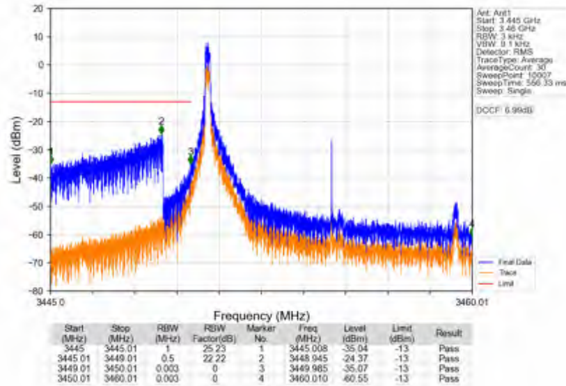
n78e_15kHz_SISO_NTNV_10MHz_CP-OFDM QPSK_3455.01MHz_Inner_1RB_Left
