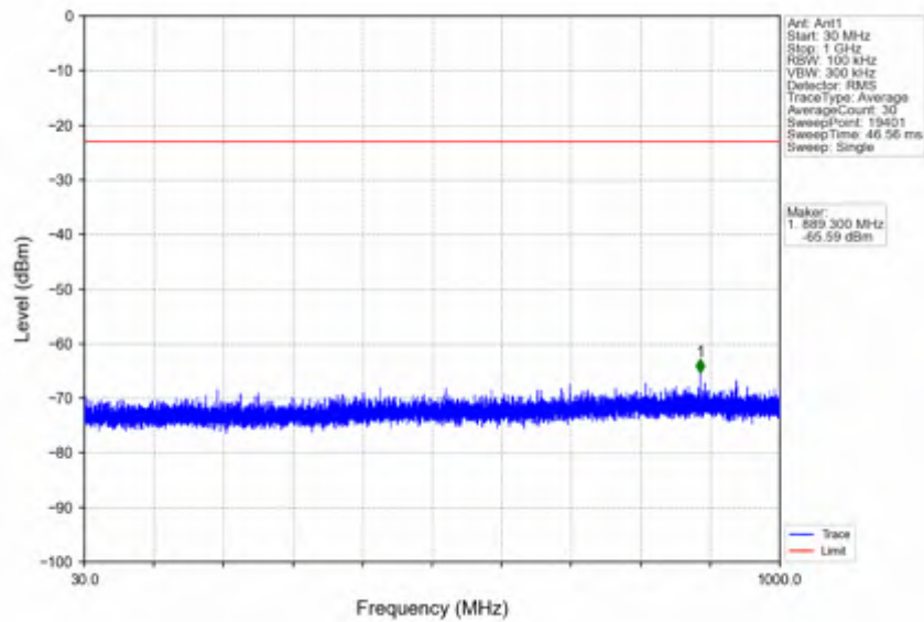
n78e_15kHz_SISO_NTNV_10MHz_DFT-s-OFDM QPSK_3455.01MHz_Inner_1RB_Left
