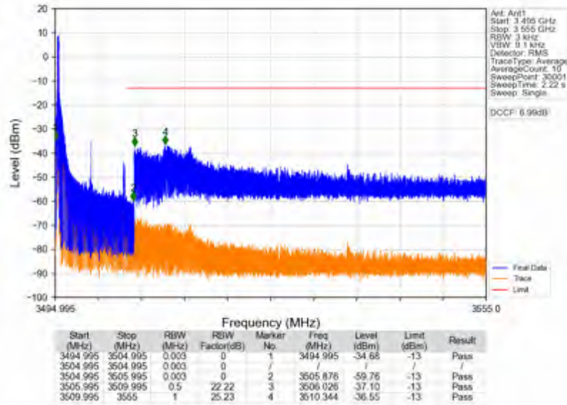
n78e_15kHz_SISO_NTNV_10MHz_DFT-s-OFDM QPSK_3499.995MHz_Edge_1RB_Left
