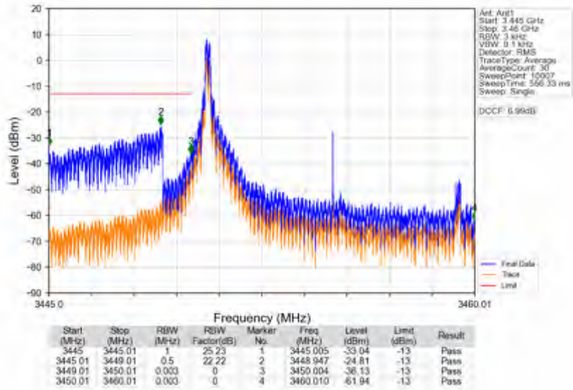
n78e_15kHz_SISO_NTNV_10MHz_DFT-s-OFDM_QPSK_3455.01MHz_Inner_1RB_Left
