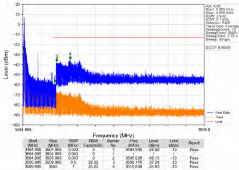
n78e_15kHz_SISO_NTV_10MHz_CP-OFDM QPSK_3499.995MHz_Edge_1RB_Left
