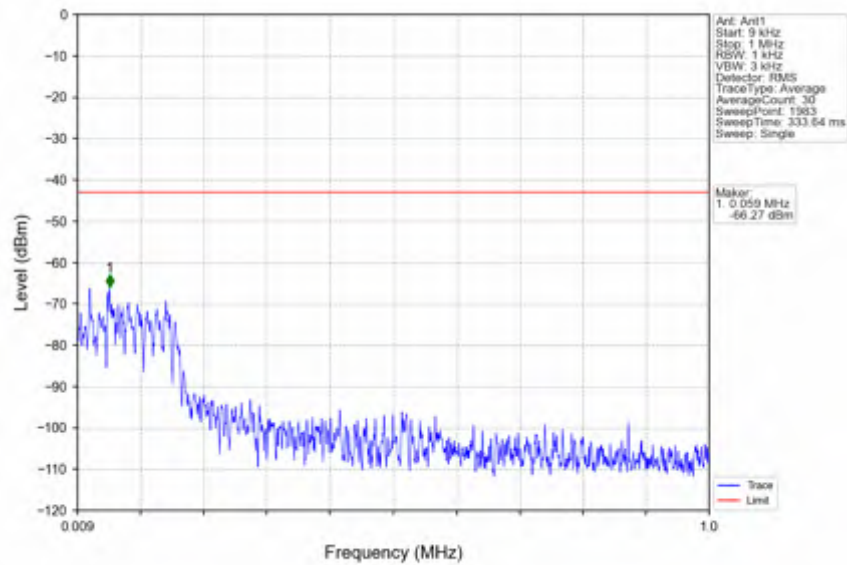
n78e_15kHz_SISO_NTNV_10MHz_DFT-s-OFDM_QPSK_3455.01MHz_Inner_1RB_Left
