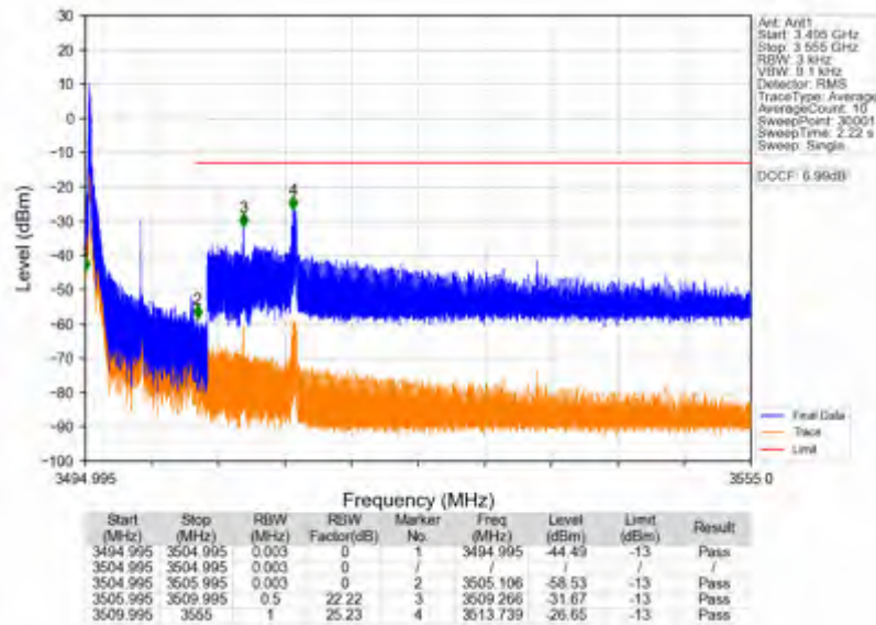
n78e_15kHz_SISO_NTNV_10MHz_DFT-s-OFDM PI/2 BPSK_3499.995MHz_Edge_1RB_Left
