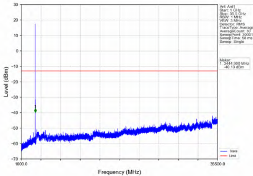
n78e_15kHz_SISO_NTV_10MHz_CP-OFDM QPSK_3499.995MHz_Edge_1RB_Left
