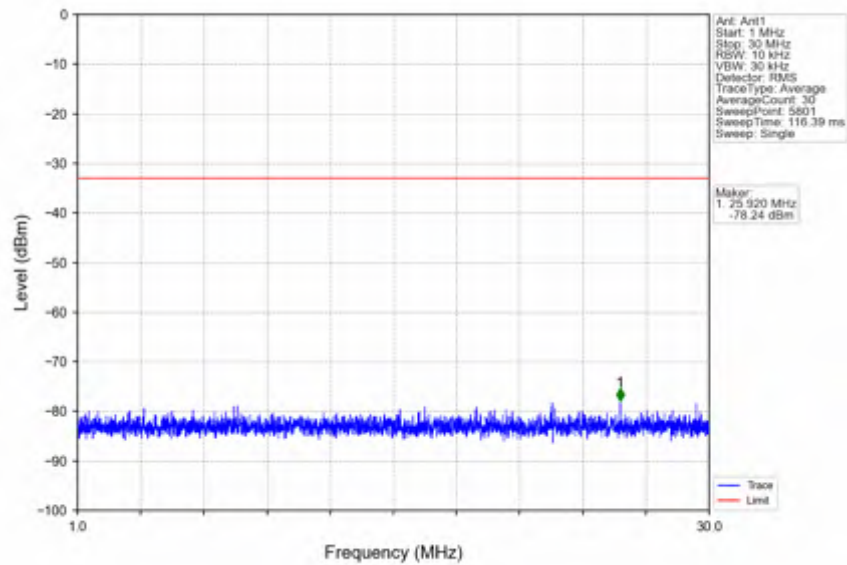
n78e_15kHz_SISO_NTNV_10MHz_DFT-s-OFDM PI/2 BPSK_3455.01MHz_Inner_1RB_Left
