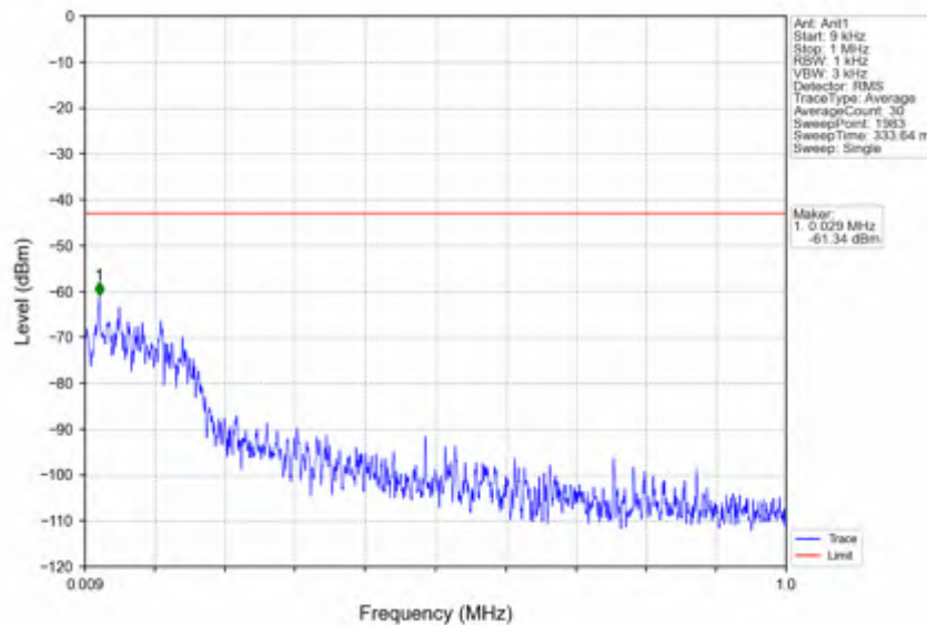
n78e_15kHz_SISO_NTNV_10MHz_CP-OFDM QPSK_3455.01MHz_Inner_1RB_Left
