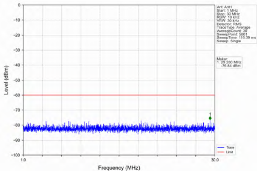
n78d_30kHz_SISO_NTV_70MHz_DFT-s-OFDM QPSK_3585MHz_Inner_1RB_Left
