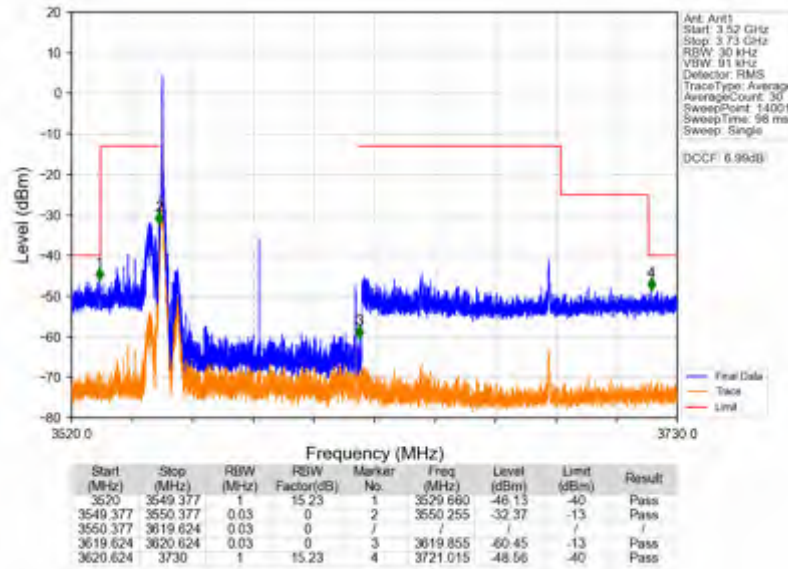
n78d_30kHz_SISO_NTNV_70MHz_CP-OFDM QPSK_3585MHz_Inner_1RB_Left
