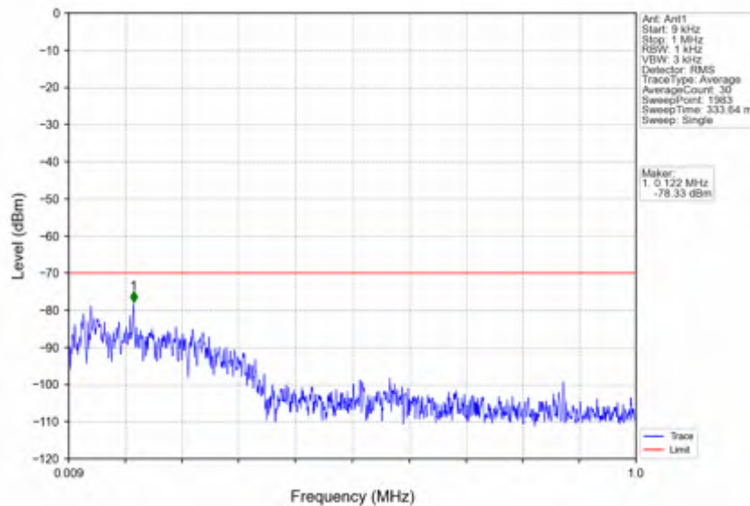
n78d_30kHz_SISO_NTNV_70MHz_CP-OFDM QPSK_3585MHz_Inner_1RB_Left
