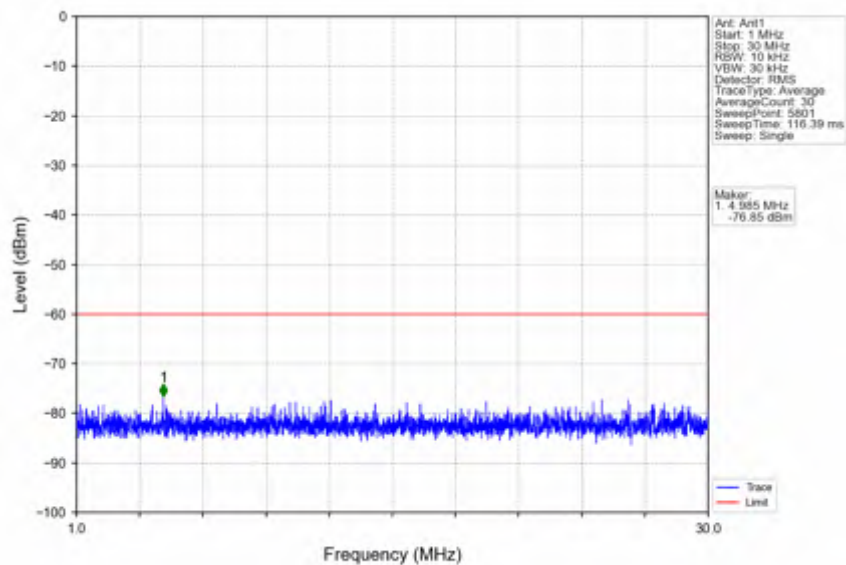
n78d_30kHz_SISO_NTV_40MHz_DFT-s-OFDM QPSK_3570MHz_Inner_1RB_Left
