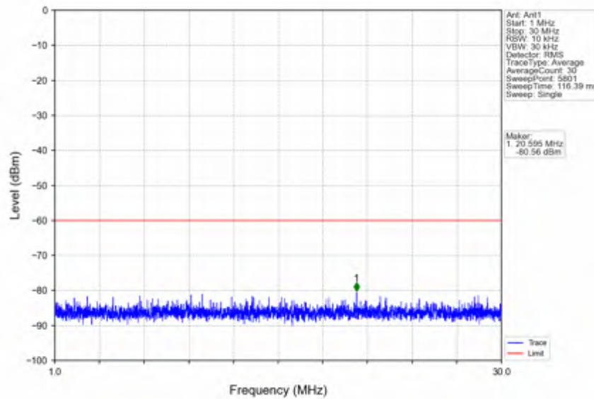
n78d_30kHz_SISO_NTNV_10MHz_CP-OFDM QPSK_3555MHz_Inner_1RB_Left
