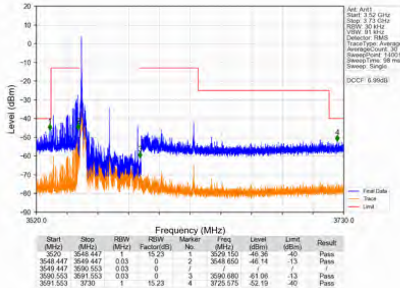
n78d_15kHz_SISO_NTNV_40MHz_CP-OFDM QPSK_3570MHz_Inner_1RB_Left
