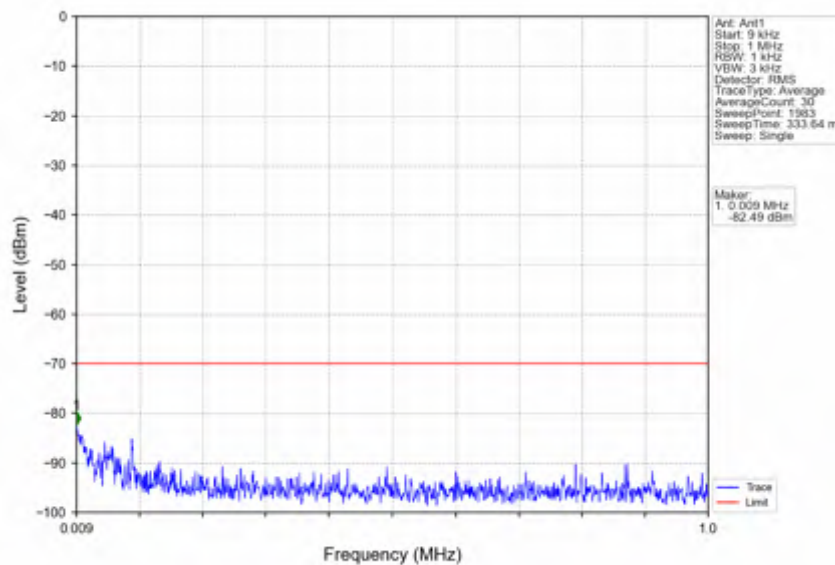
n78d_15kHz_SISO_NTNV_40MHz_CP-OFDM QPSK_3570MHz_Inner_1RB_Left
