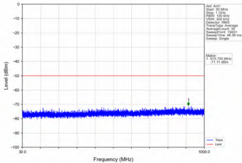
n78d_15kHz_SISO_NTVV_10MHz_DFT-s-OFDM QPSK_3555MHz_Inner_1RB_Left
