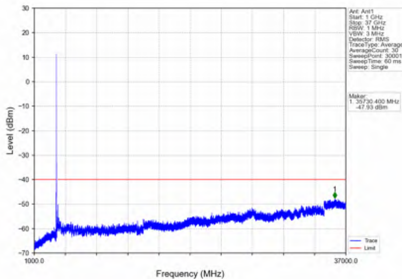
n78d_15kHz_SISO_NTVV_10MHz_DFT-s-OFDM QPSK_3555MHz_Inner_1RB_Left
