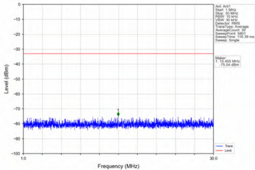
n66_30kHz_SISO_NTNV_40MHz_CP-OFDM QPSK_1760MHz_Inner_1RB_Right
