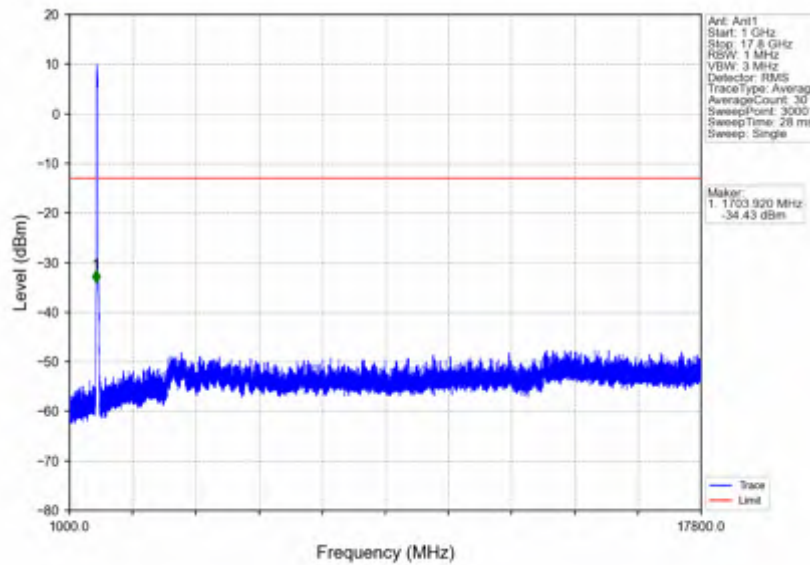
n66_30kHz_SISO_NTNV_40MHz_DFT-s-OFDM QPSK_1730MHz_Inner_1RB_Left
