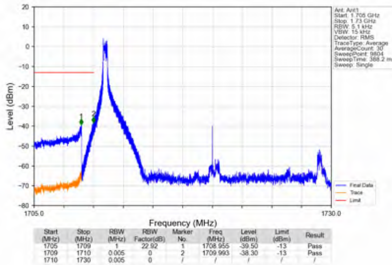
n66_30kHz_SISO_NTNV_20MHz_DFT-s-OFDM QPSK_1720MHz_Edge_1RB_Left
