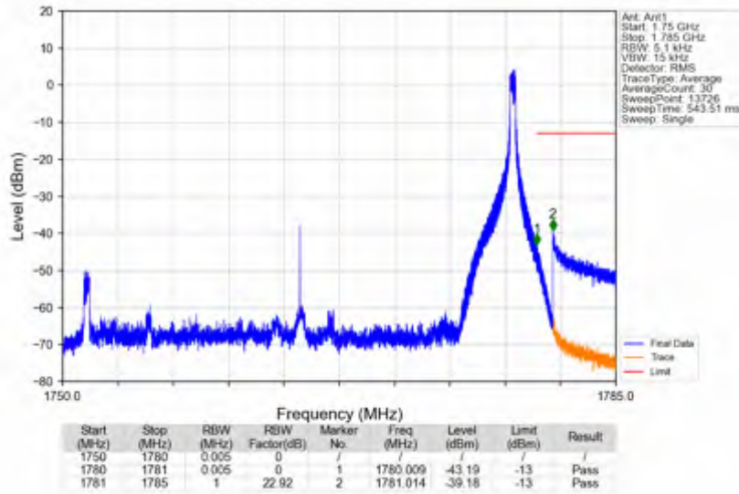
n66_30kHz_SISO_NTNV_30MHz_DFT-s-OFDM QPSK_1765MHz_Inner_1RB_Right
