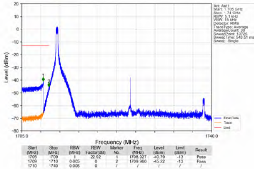
n66_30kHz_SISO_NTNV_30MHz_CP-OFDM QPSK_1725MHz_Inner_1RB_Left
