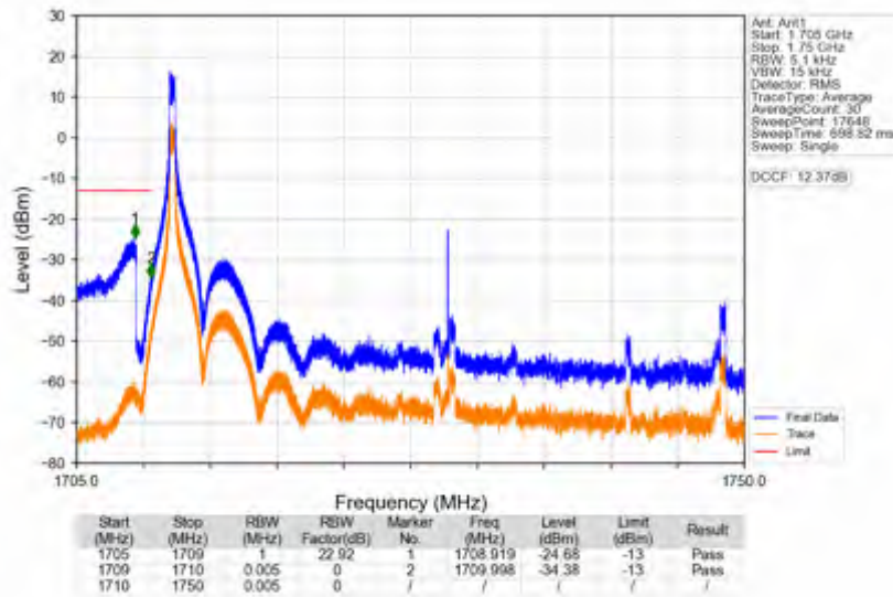
n66_30kHz_SISO_NTNV_40MHz_DFT-s-OFDM QPSK_1730MHz_Inner_1RB_Left
