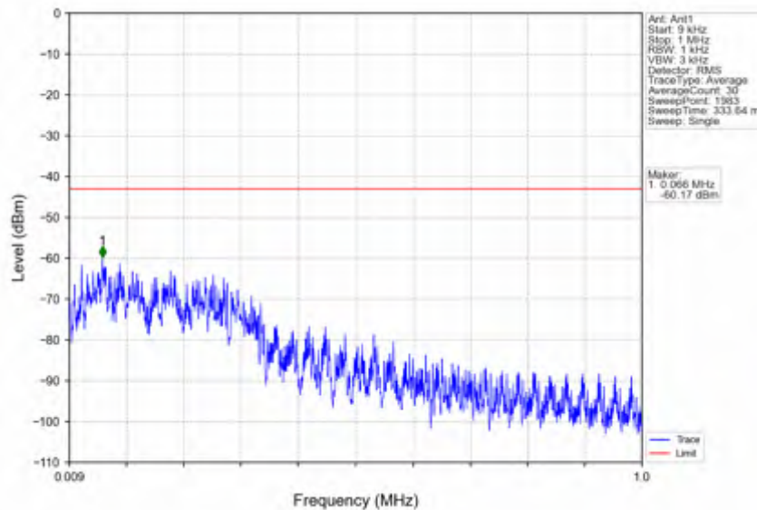
n66_30kHz_SISO_NTNV_40MHz_CP-OFDM QPSK_1730MHz_Inner_1RB_Left
