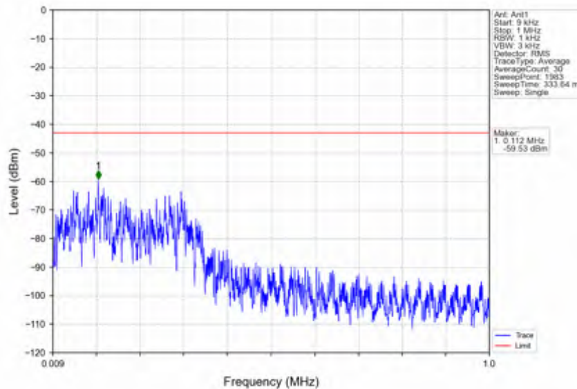
n66_30kHz_SISO_NTNV_40MHz_DFT-s-OFDM PI/2 BPSK_1730MHz_Inner_1RB_Left
