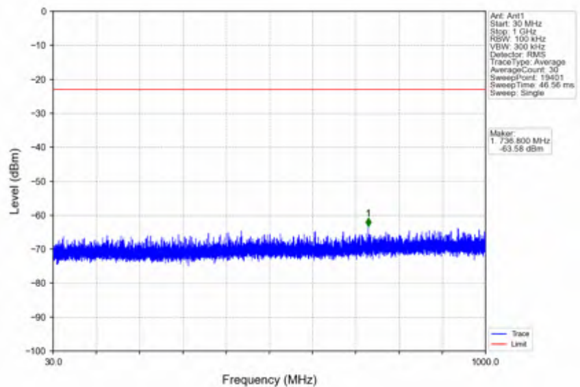
n66_30kHz_SISO_NTNV_30MHz_CP-OFDM QPSK_1725MHz_Inner_1RB_Left
