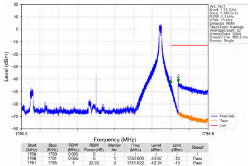
n66_30kHz_SISO_NTNV_20MHz_DFT-s-OFDM QPSK_1770MHz_Inner_1RB_Right
