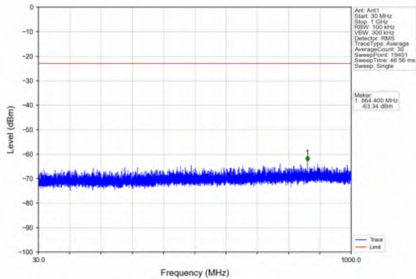
n66_30kHz_SISO_NTNV_20MHz_DFT-s-OFDM QPSK_1720MHz_Edge_1RB_Left
