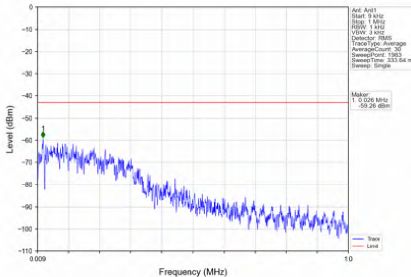
n66_30kHz_SISO_NTNV_20MHz_CP-OFDM QPSK_1770MHz_Inner_1RB_Right
