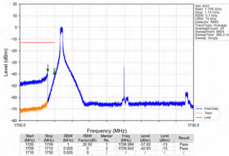
n66_30kHz_SISO_NTNV_20MHz_CP-OFDM QPSK_1720MHz_Edge_1RB_Left
