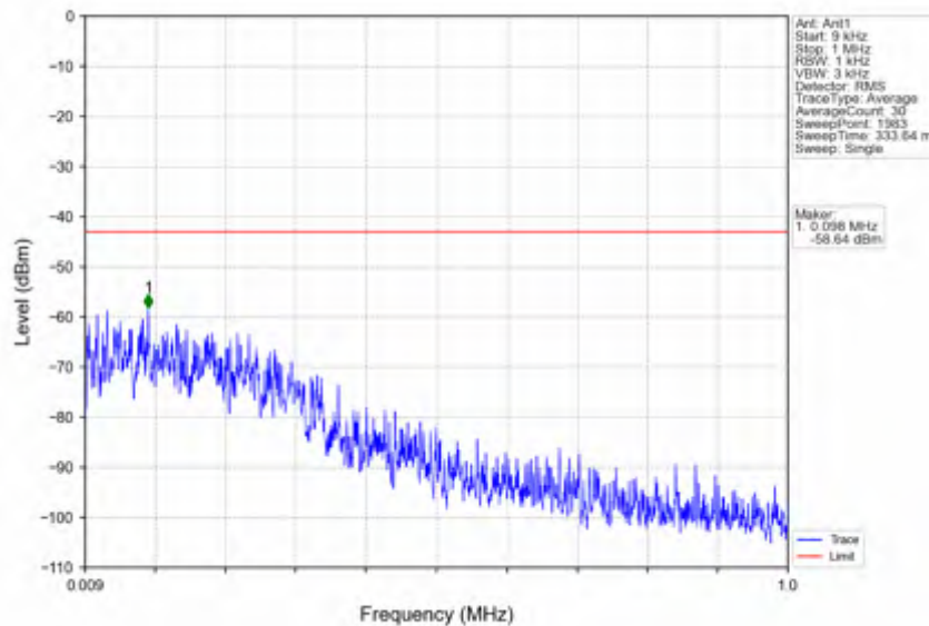
n66_30kHz_SISO_NTNV_20MHz_CP-OFDM QPSK_1720MHz_Inner_1RB_Left
