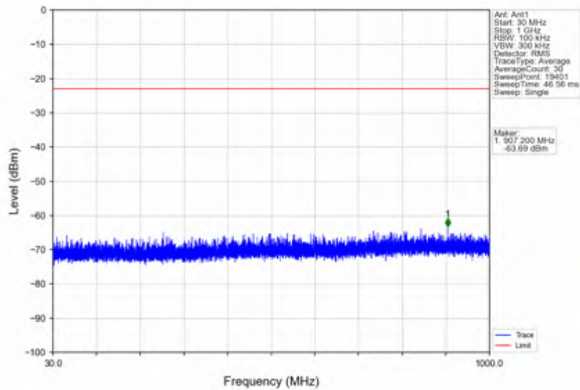
n66_30kHz_SISO_NTNV_40MHz_DFT-s-OFDM QPSK_1730MHz_Inner_1RB_Left
