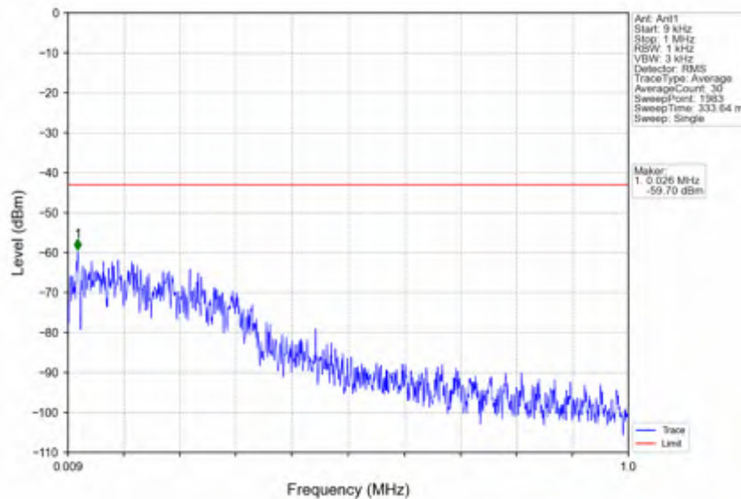
n66_30kHz_SISO_NTNV_30MHz_CP-OFDM QPSK_1725MHz_Inner_1RB_Left
