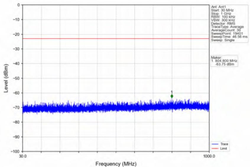
n66_30kHz_SISO_NTNV_30MHz_CP-OFDM QPSK_1765MHz_Inner_1RB_Right
