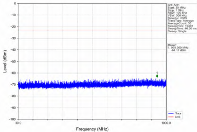
n66_30kHz_SISO_NTNV_20MHz_DFT-s-OFDM_QPSK_1770MHz_Inner_1RB_Right
