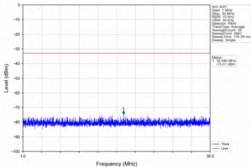
n66_30kHz_SISO_NTNV_20MHz_DFT-s-OFDM QPSK_1720MHz_Inner_1RB_Left
