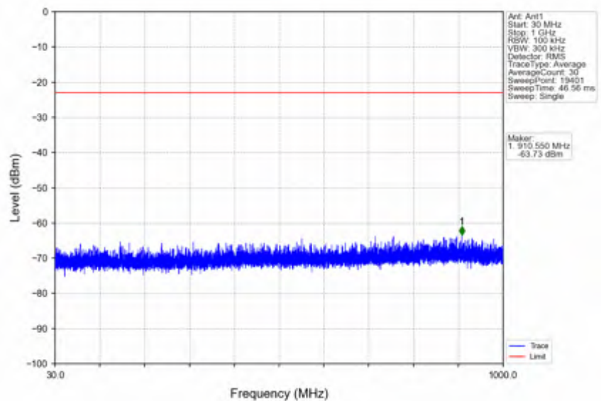
n66_30kHz_SISO_NTNV_20MHz_CP-OFDM QPSK_1720MHz_Edge_1RB_Left
