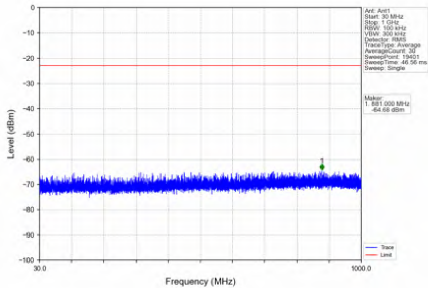
n66_30kHz_SISO_NTNV_40MHz_DFT-s-OFDM QPSK_1760MHz_Inner_1RB_Right
