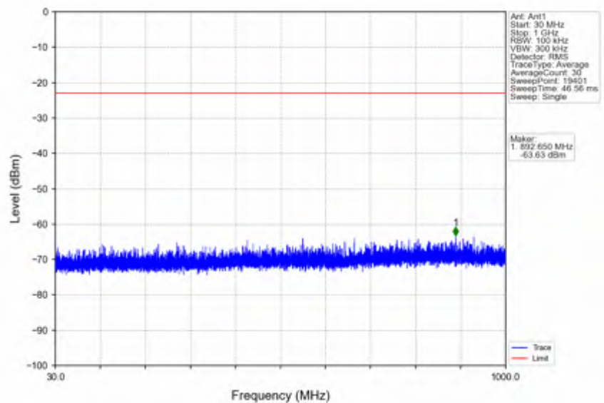
n66_30kHz_SISO_NTNV_40MHz_CP-OFDM QPSK_1730MHz_Inner_1RB_Left
