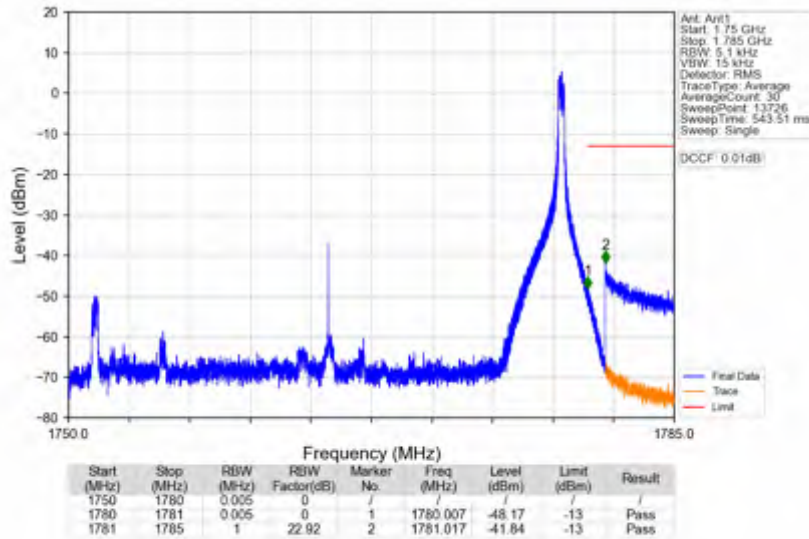
n66_30kHz_SISO_NTNV_30MHz_DFT-s-OFDM PI/2 BPSK_1765MHz_Inner_1RB_Right
