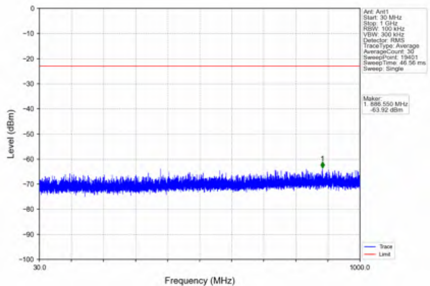
n66_30kHz_SISO_NTNV_20MHz_CP-OFDM QPSK_1770MHz_Inner_1RB_Right
