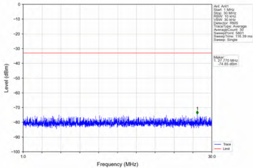
n66_30kHz_SISO_NTNV_20MHz_CP-OFDM QPSK_1720MHz_Inner_1RB_Left
