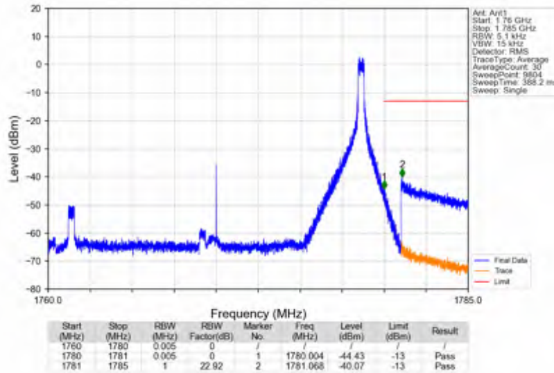
n66_30kHz_SISO_NTNV_20MHz_CP-OFDM QPSK_1770MHz_Inner_1RB_Right
