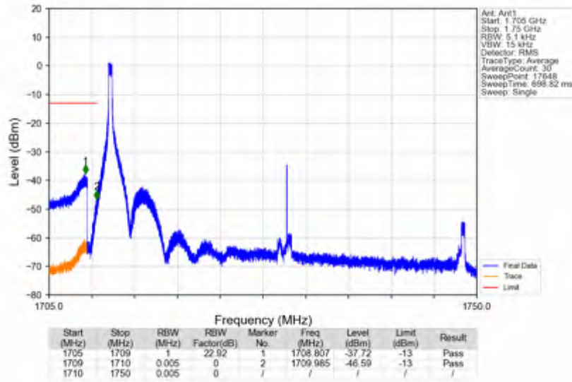
n66_30kHz_SISO_NTNV_40MHz_CP-OFDM QPSK_1730MHz_Inner_1RB_Left
