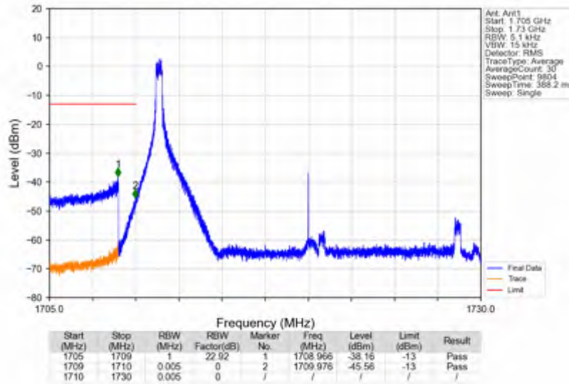
n66_30kHz_SISO_NTNV_20MHz_CP-OFDM QPSK_1720MHz_Inner_1RB_Left
