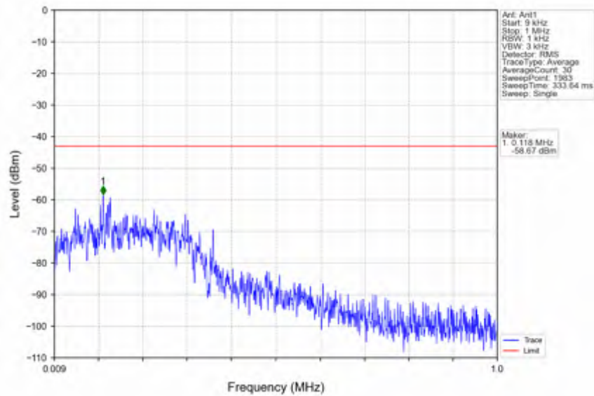
n66_30kHz_SISO_NTNV_40MHz_DFT-s-OFDM QPSK_1760MHz_Inner_1RB_Right
