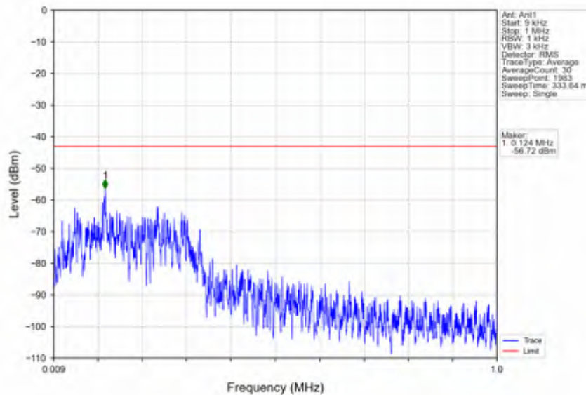
n66_30kHz_SISO_NTNV_10MHz_DFT-s-OFDM PI/2 BPSK_1715MHz_Inner_1RB_Left
