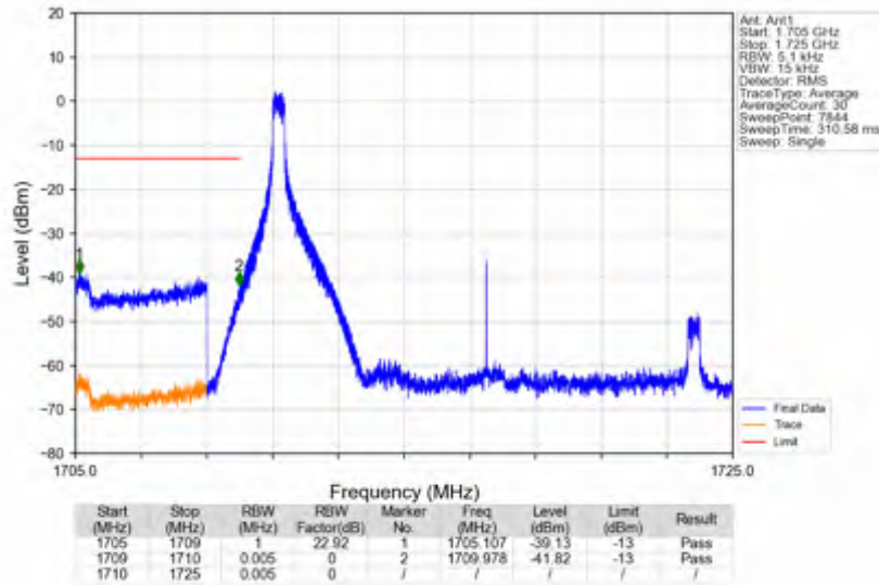
n66_30kHz_SISO_NTV_15MHz_CP-OFDM QPSK_1717.5MHz_Inner_1RB_Left
