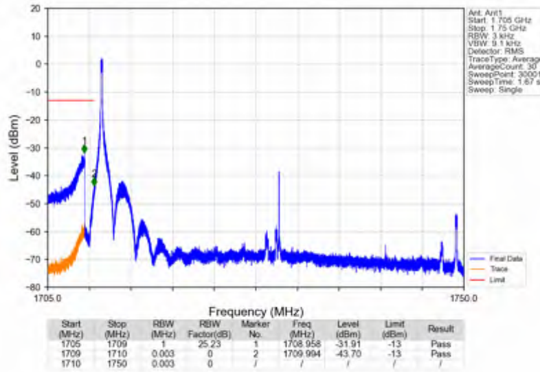
n66_15kHz_SISO_NTNV_40MHz_CP-OFDM QPSK_1730MHz_Inner_1RB_Left
