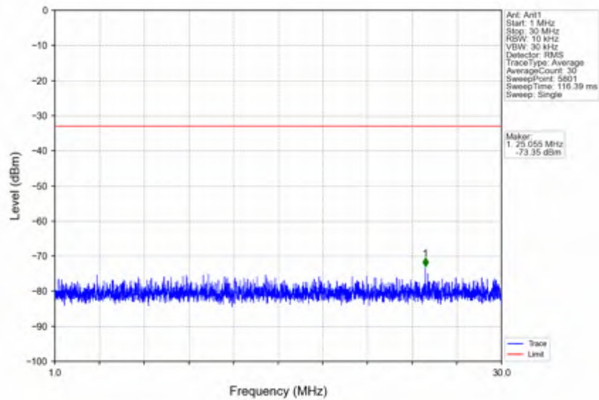
n66_30kHz_SISO_NTNV_10MHz_CP-OFDM QPSK_1715MHz_Inner_1RB_Left
