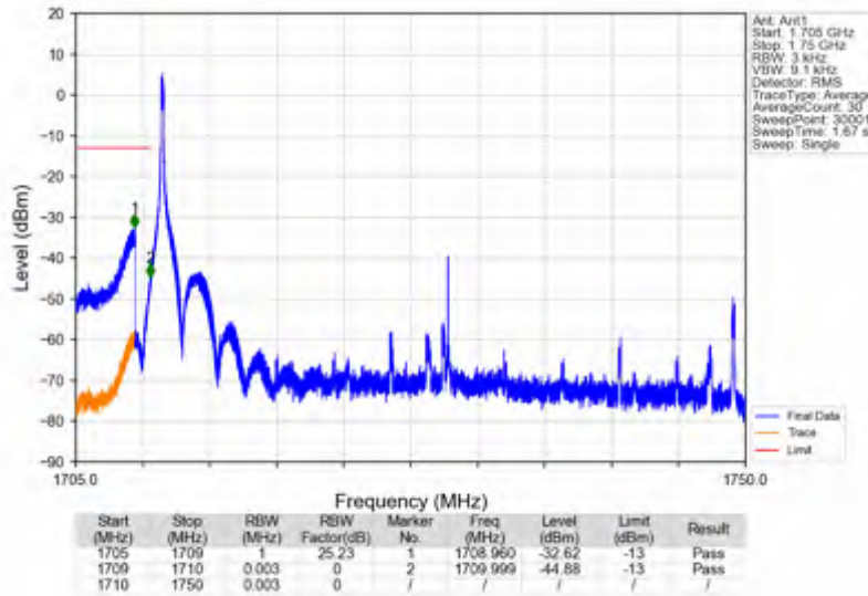
n66_15kHz_SISO_NTNV_40MHz_DFT-s-OFDM PI/2 BPSK_1730MHz_Inner_1RB_Left
