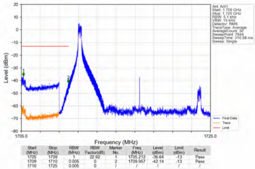
n66_30kHz_SISO_NTNV_15MHz_DFT-s-OFDM QPSK_1717.5MHz_Inner_1RB_Left
