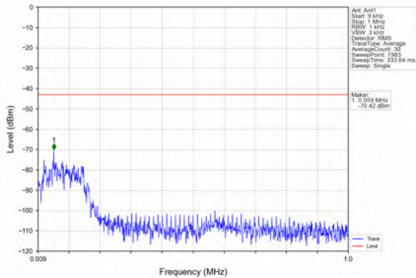
n66_15kHz_SISO_NTNV_40MHz_DFT-s-OFDM QPSK_1760MHz_Inner_1RB_Right
