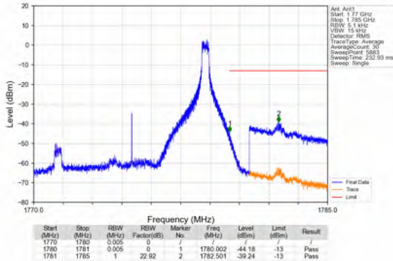
n66_30kHz_SISO_NTNV_10MHz_CP-OFDM QPSK_1775MHz_Inner_1RB_Right
