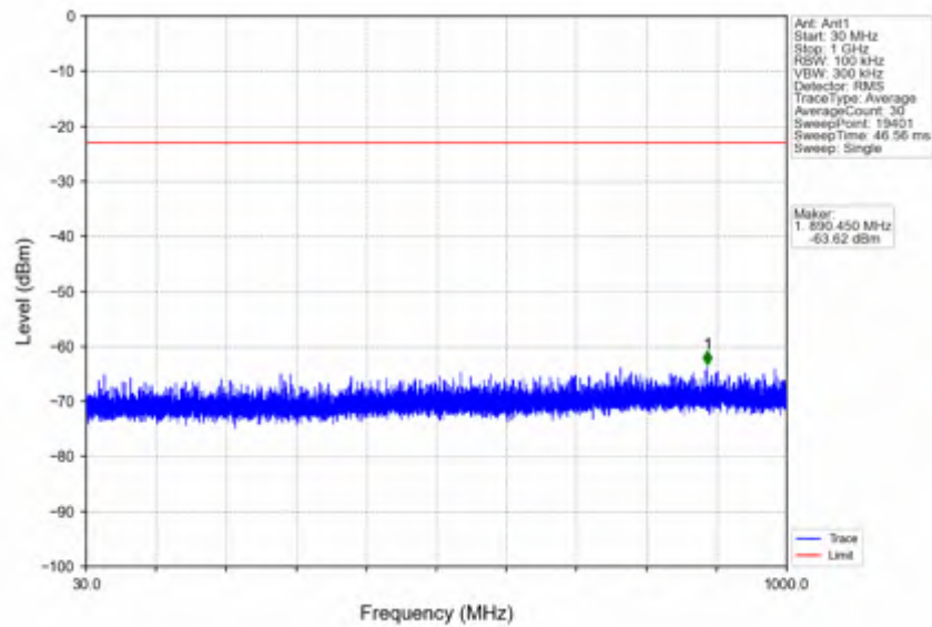
n66_30kHz_SISO_NTNV_15MHz_DFT-s-OFDM QPSK_1717.5MHz_Inner_1RB_Left
