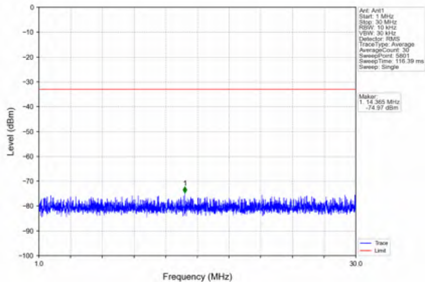
n66_30kHz_SISO_NTNV_15MHz_DFT-s-OFDM QPSK_1717.5MHz_Inner_1RB_Left
