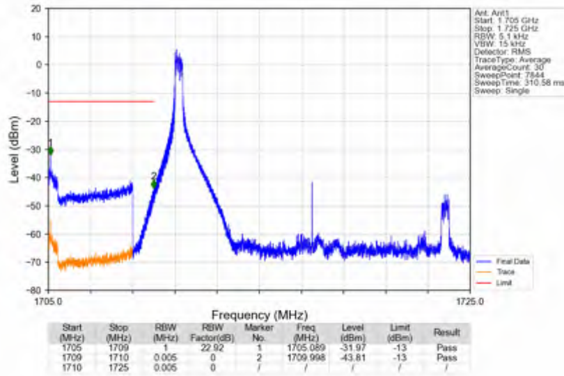
n66_30kHz_SISO_NTNV_15MHz_DFT-s-OFDM PI/2 BPSK_1717.5MHz_Inner_1RB_Left
