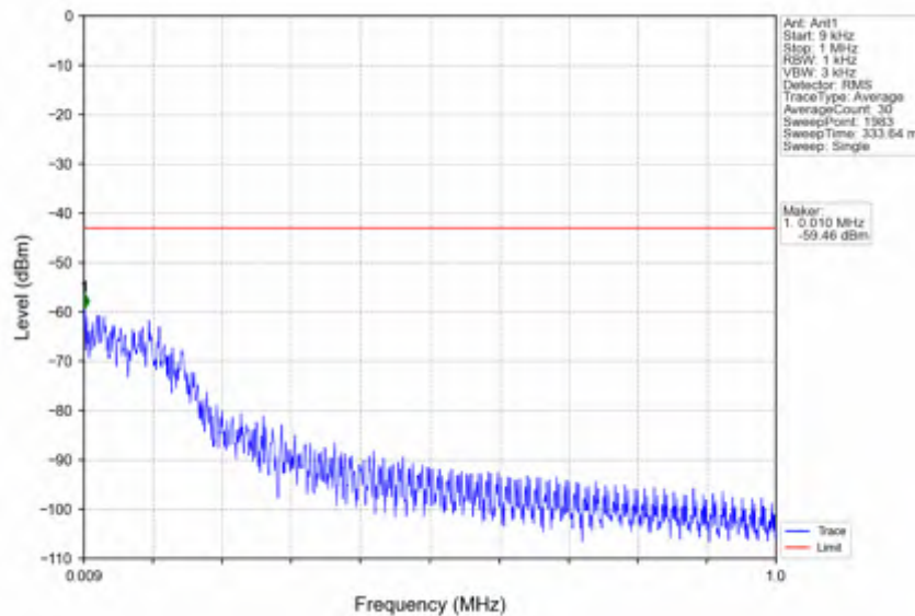
n66_15kHz_SISO_NTNV_30MHz_CP-OFDM QPSK_1725MHz_Inner_1RB_Left
