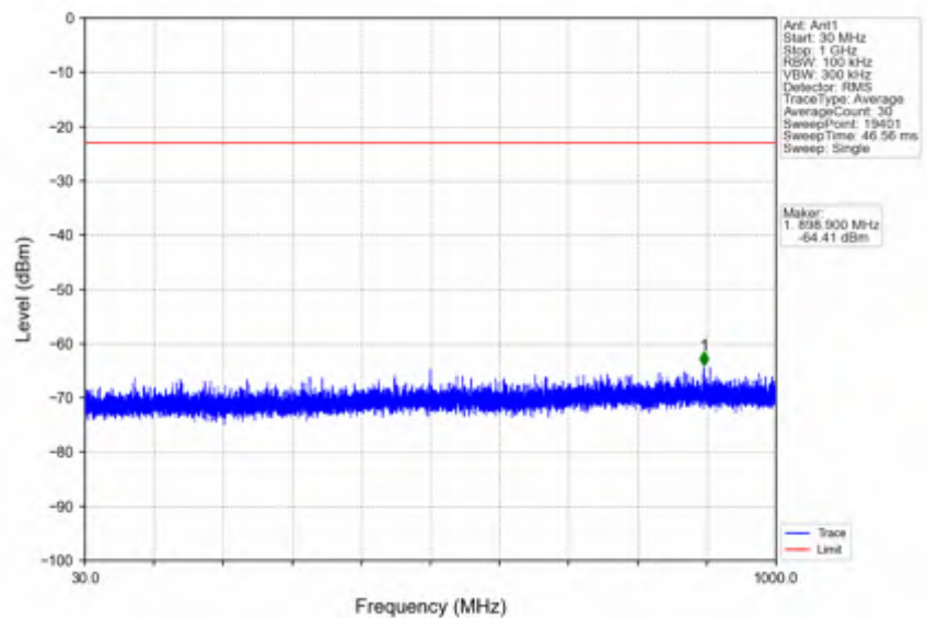
n66_15kHz_SISO_NTNV_30MHz_CP-OFDM QPSK_1725MHz_Inner_1RB_Left
