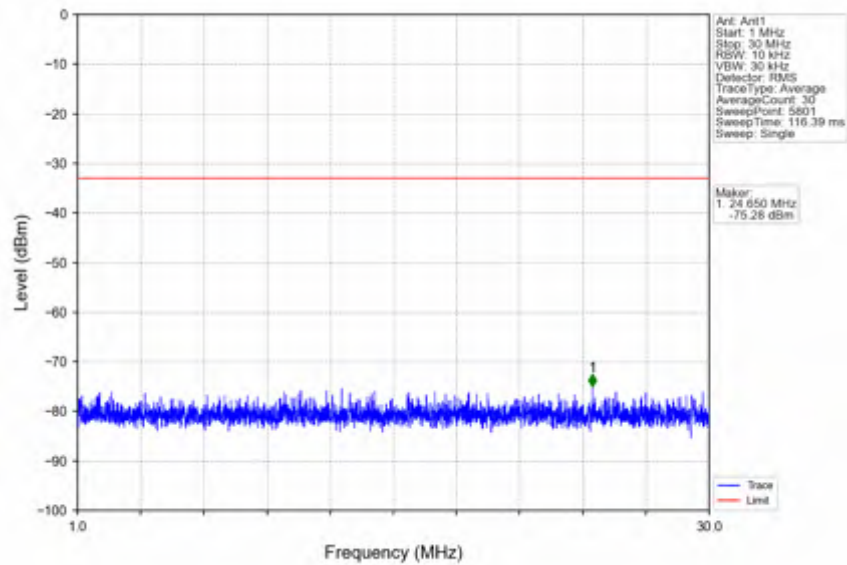
n66_15kHz_SISO_NTNV_30MHz_CP-OFDM QPSK_1765MHz_Inner_1RB_Right
