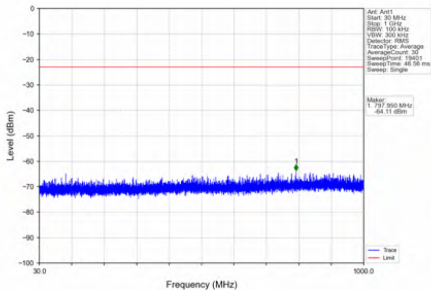
n66_15kHz_SISO_NTNV_40MHz_CP-OFDM QPSK_1760MHz_Inner_1RB_Right
