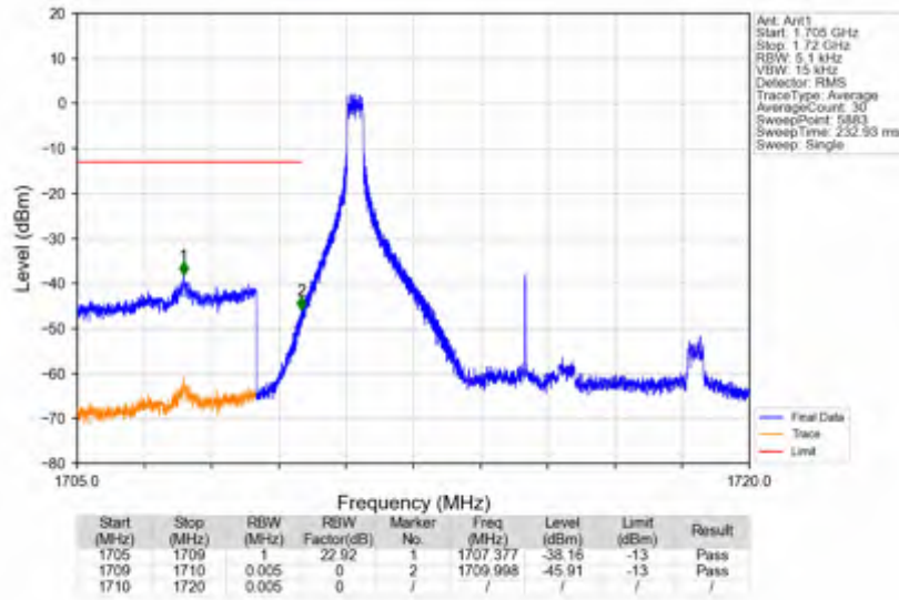
n66_30kHz_SISO_NTNV_10MHz_CP-OFDM QPSK_1715MHz_Inner_1RB_Left
