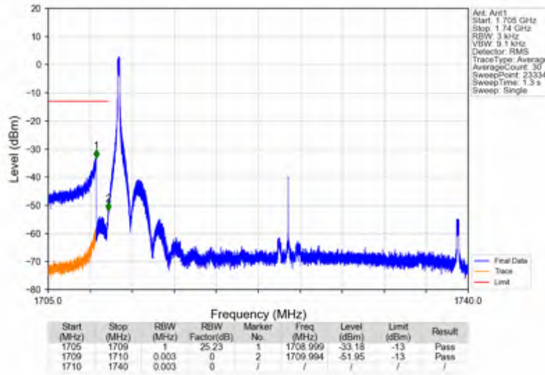
n66_15kHz_SISO_NTNV_30MHz_CP-OFDM QPSK_1725MHz_Inner_1RB_Left
