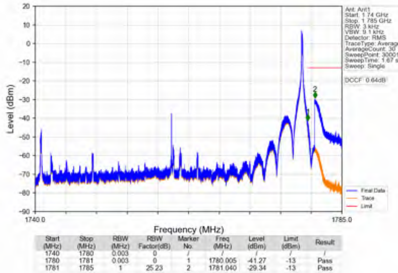
n66_15kHz_SISO_NTNV_40MHz_DFT-s-OFDM PI/2 BPSK_1760MHz_Inner_1RB_Right
