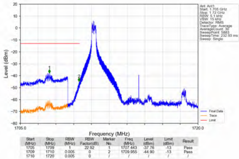
n66_30kHz_SISO_NTNV_10MHz_DFT-s-OFDM QPSK_1715MHz_Inner_1RB_Left
