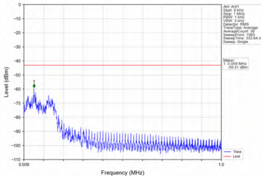
n66_15kHz_SISO_NTNV_40MHz_DFT-s-OFDM PI/2 BPSK_1760MHz_Inner_1RB_Right
