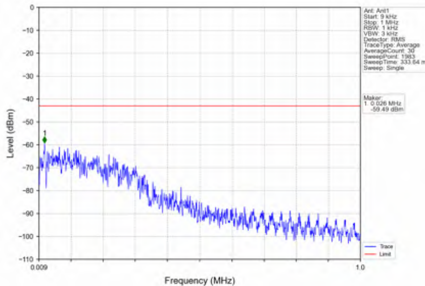
n66_30kHz_SISO_NTV_15MHz_CP-OFDM QPSK_1717.5MHz_Inner_1RB_Left
