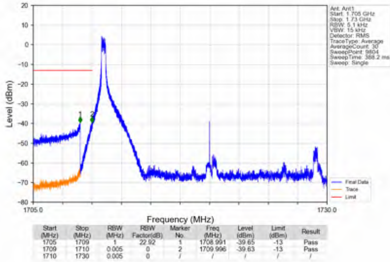
n66_30kHz_SISO_NTNV_20MHz_DFT-s-OFDM_PI/2_BPSK_1720MHz_Edge_1RB_Left
