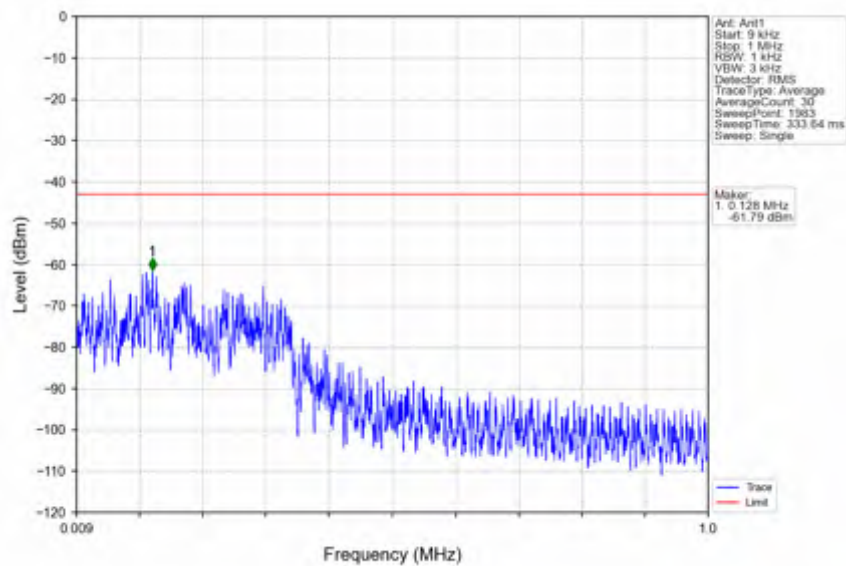
n66_30kHz_SISO_NTNV_20MHz_DFT-s-OFDM_PI/2_BPSK_1720MHz_Edge_1RB_Left
