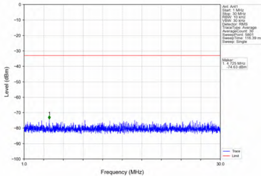
n66_30kHz_SISO_NTV_15MHz_CP-OFDM QPSK_1717.5MHz_Inner_1RB_Left
