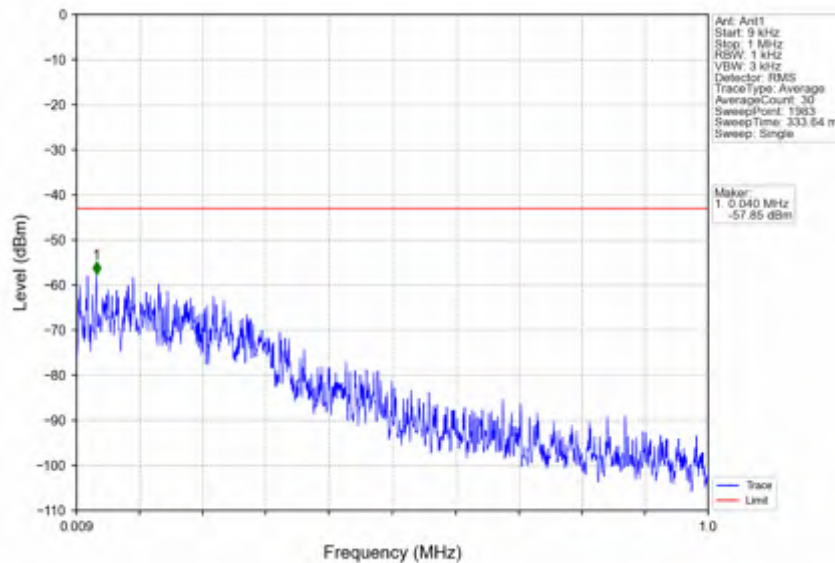
n66_30kHz_SISO_NTNV_10MHz_CP-OFDM QPSK_1775MHz_Inner_1RB_Right
