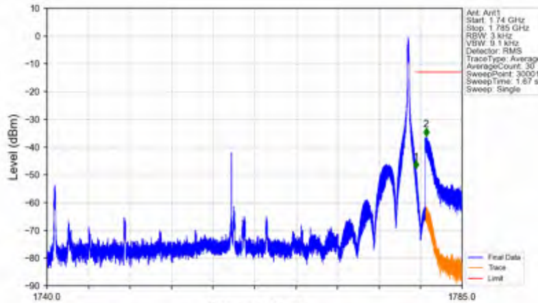
n66_15kHz_SISO_NTNV_40MHz_DFT-s-OFDM QPSK_1760MHz_Inner_1RB_Right
