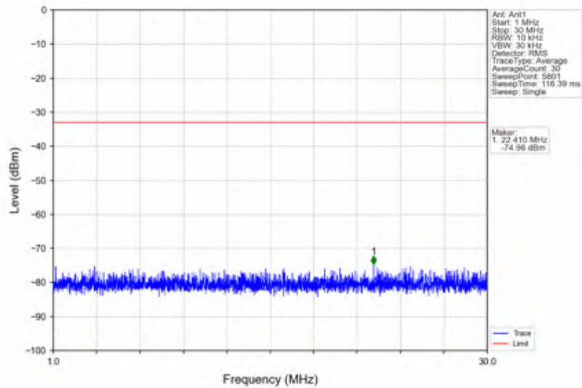
n66_30kHz_SISO_NTNV_10MHz_CP-OFDM QPSK_1775MHz_Inner_1RB_Right
