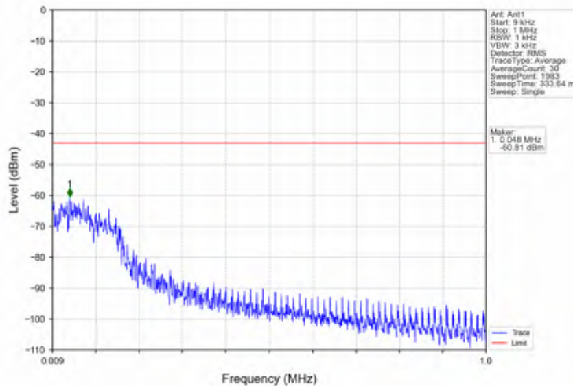
n66_15kHz_SISO_NTNV_40MHz_CP-OFDM QPSK_1730MHz_Inner_1RB_Left
