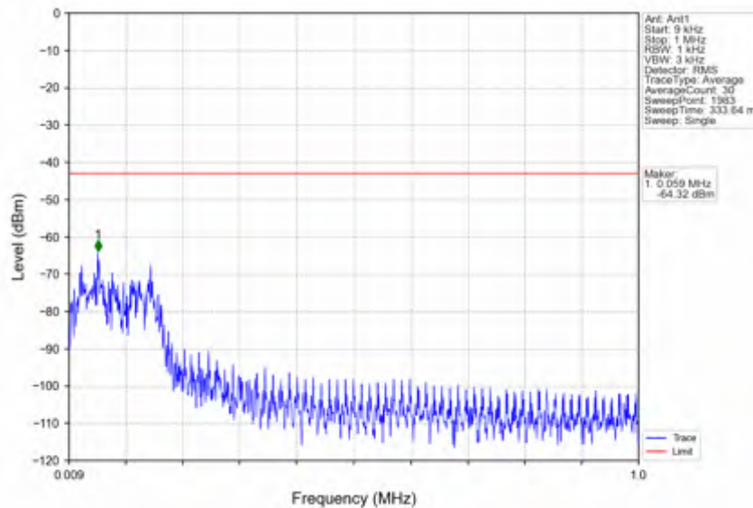
n66_15kHz_SISO_NTNV_40MHz_DFT-s-OFDM PI/2 BPSK_1730MHz_Inner_1RB_Left
