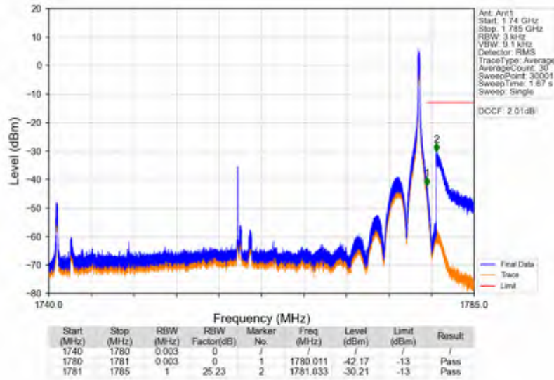
n66_15kHz_SISO_NTNV_40MHz_CP-OFDM QPSK_1760MHz_Inner_1RB_Right
