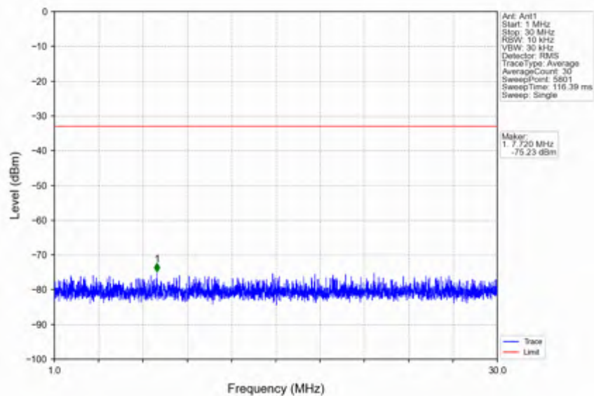
n66_30kHz_SISO_NTNV_10MHz_DFT-s-OFDM QPSK_1715MHz_Inner_1RB_Left
