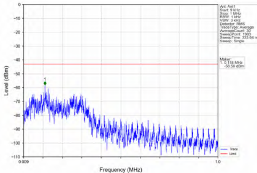
n66_30kHz_SISO_NTNV_10MHz_DFT-s-OFDM PI/2 BPSK_1775MHz_Inner_1RB_Right
