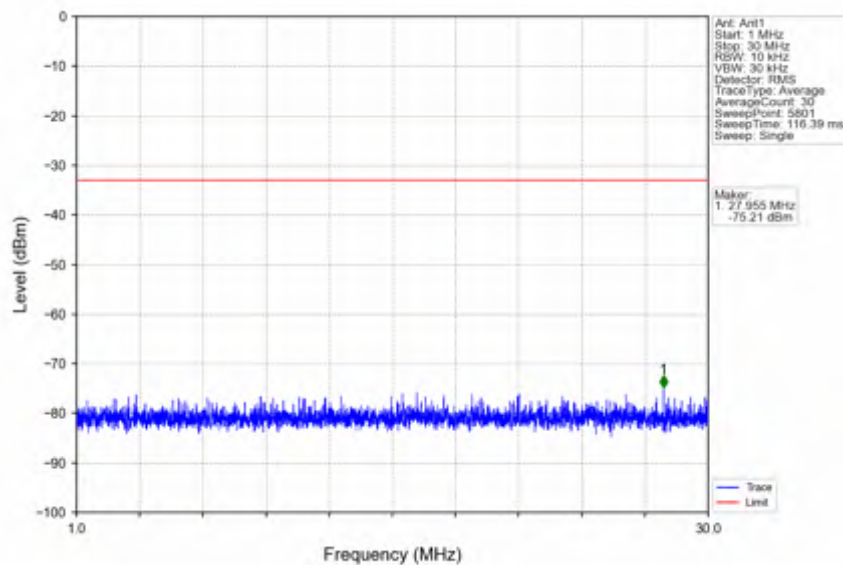
n66_15kHz_SISO_NTNV_15MHz_DFT-s-OFDM QPSK_1717.5MHz_Inner_1RB_Left
