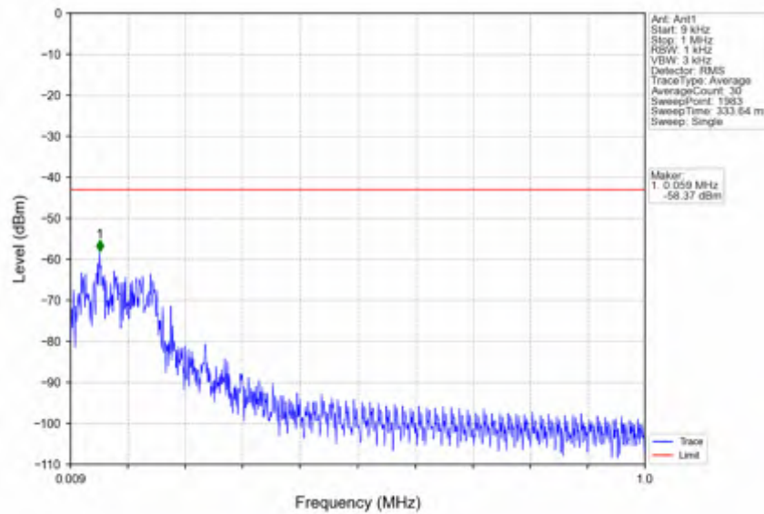
n66_15kHz_SISO_NTV_20MHz_DFT-s-OFDM_QPSK_1770MHz_Inner_1RB_Right
