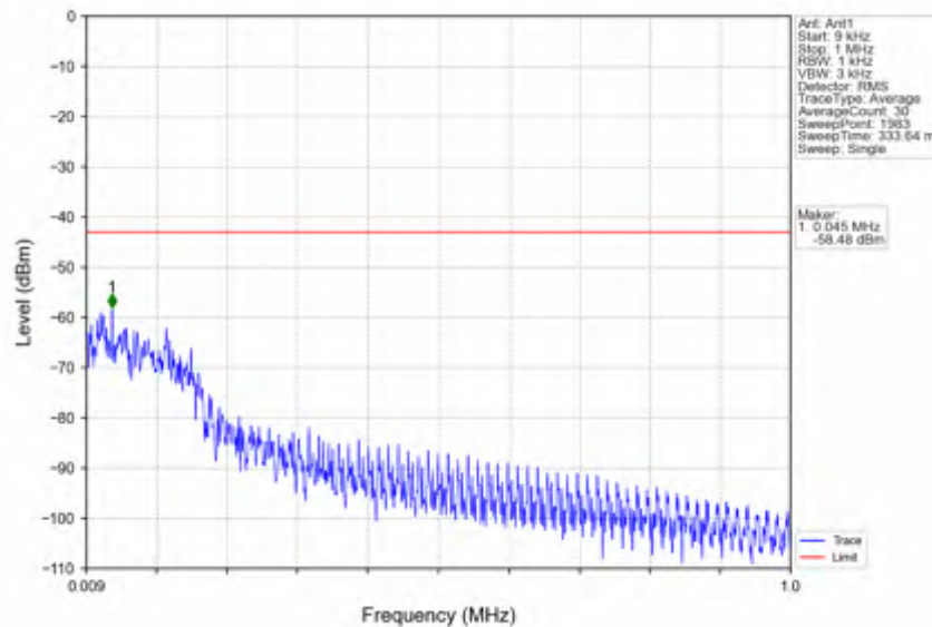
n66_15kHz_SISO_NTV_15MHz_CP-OFDM QPSK_1717.5MHz_Inner_1RB_Left
