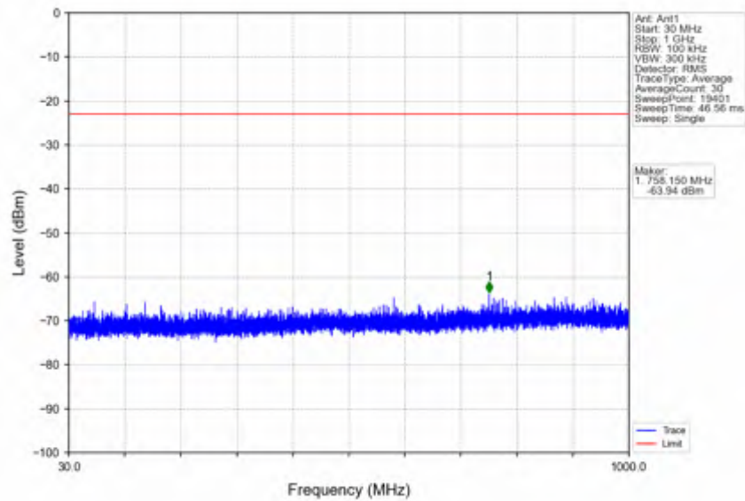
n66_15kHz_SISO_NTNV_15MHz_DFT-s-OFDM QPSK_1717.5MHz_Inner_1RB_Left
