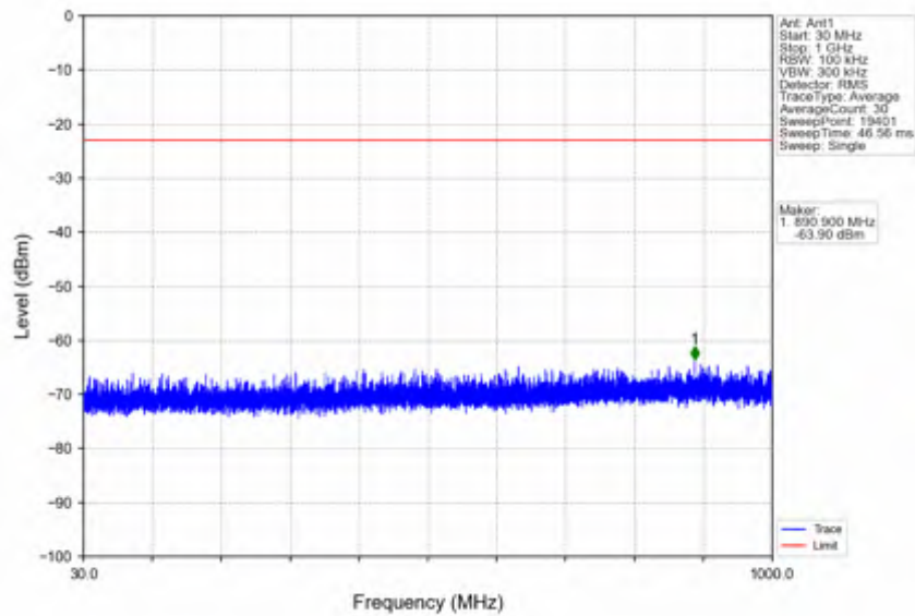
n66_15kHz_SISO_NTNV_20MHz_DFT-s-OFDM QPSK_1720MHz_Edge_1RB_Left
