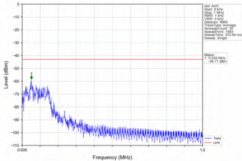
n66_15kHz_SISO_NTNV_20MHz_DFT-s-OFDM QPSK_1720MHz_Inner_1RB_Left
