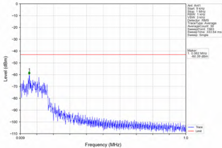
n66_15kHz_SISO_NTNV_20MHz_DFT-s-OFDM QPSK_1720MHz_Edge_1RB_Left
