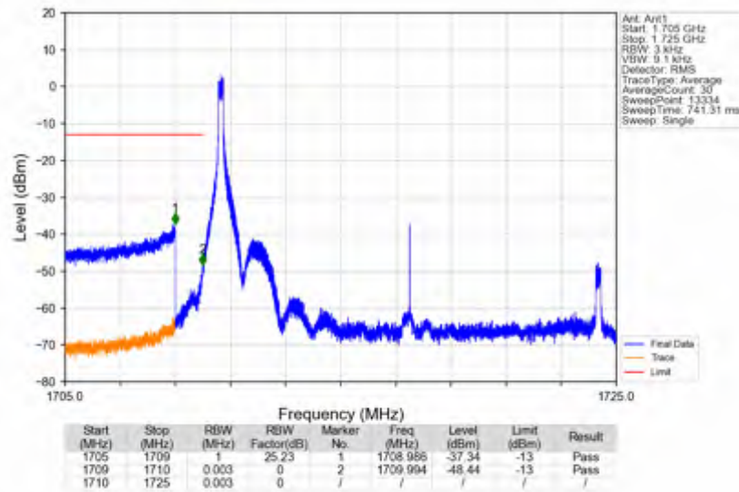
n66_15kHz_SISO_NTV_15MHz_CP-OFDM QPSK_1717.5MHz_Inner_1RB_Left
