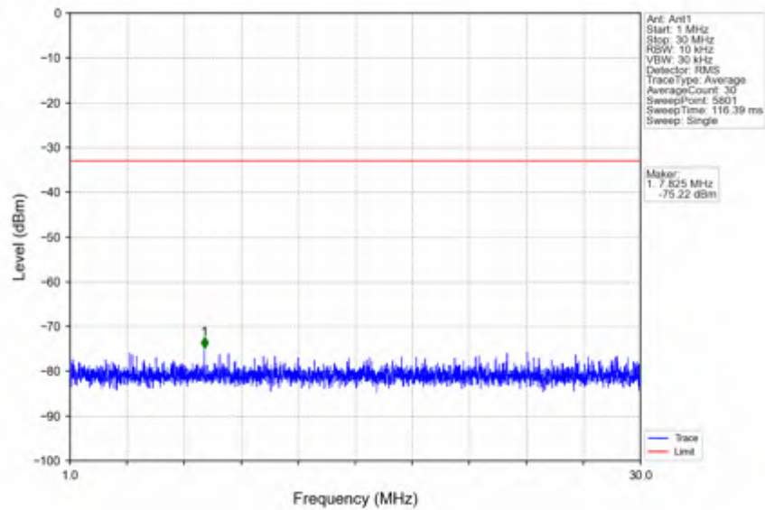
n66_15kHz_SISO_NTNV_20MHz_CP-OFDM QPSK_1770MHz_Inner_1RB_Right
