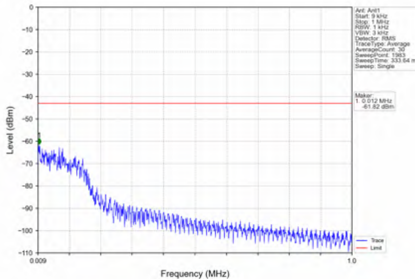
n66_15kHz_SISO_NTNV_20MHz_CP-OFDM QPSK_1720MHz_Edge_1RB_Left
