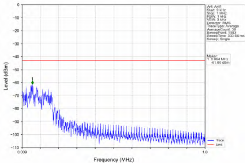
n66_15kHz_SISO_NTNV_20MHz_DFT-s-OFDM_PI/2_BPSK_1720MHz_Edge_1RB_Left
