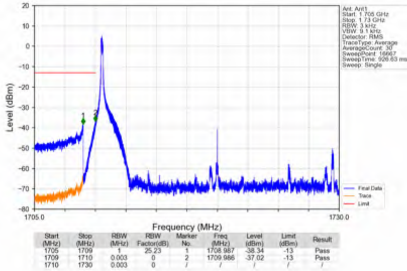
n66_15kHz_SISO_NTNV_20MHz_DFT-s-OFDM_PI/2_BPSK_1720MHz_Edge_1RB_Left
