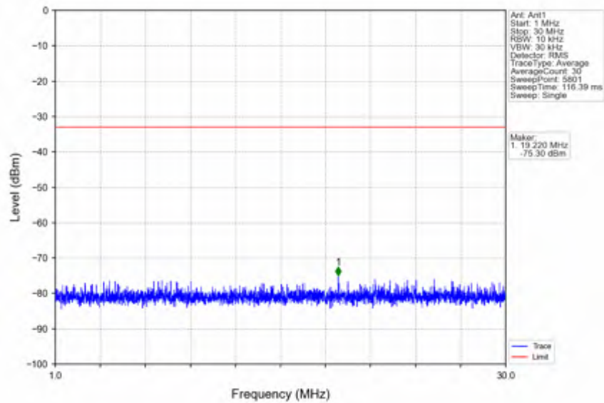
n66_15kHz_SISO_NTNV_20MHz_CP-OFDM QPSK_1720MHz_Inner_1RB_Left
