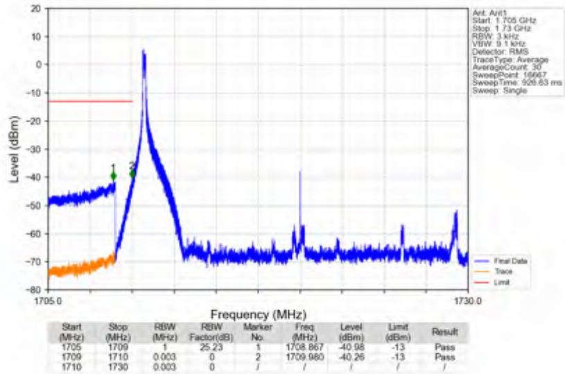
n66_15kHz_SISO_NTNV_20MHz_DFT-s-OFDM QPSK_1720MHz_Inner_1RB_Left
