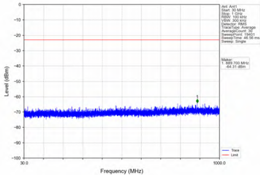
n66_15kHz_SISO_NTNV_20MHz_DFT-s-OFDM QPSK_1720MHz_Inner_1RB_Left
