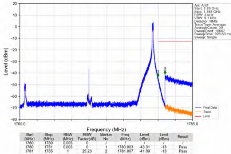
n66_15kHz_SISO_NTNV_20MHz_CP-OFDM QPSK_1770MHz_Inner_1RB_Right
