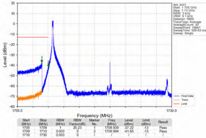
n66_15kHz_SISO_NTNV_20MHz_CP-OFDM QPSK_1720MHz_Inner_1RB_Left
