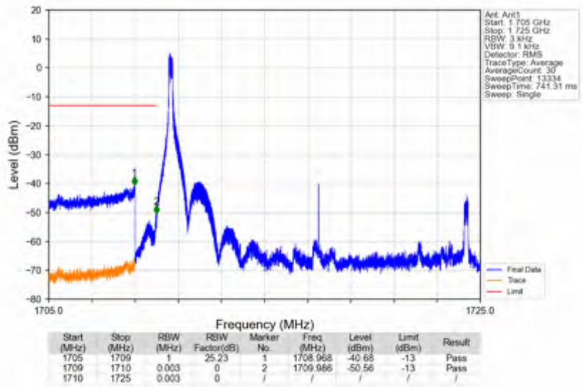
n66_15kHz_SISO_NTNV_15MHz_DFT-s-OFDM QPSK_1717.5MHz_Inner_1RB_Left
