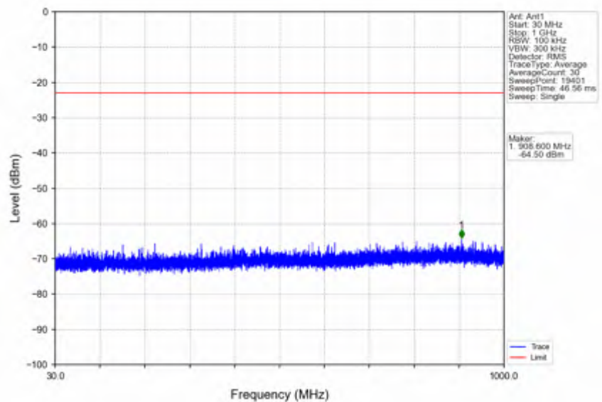
n66_15kHz_SISO_NTNV_15MHz_CP-OFDM QPSK_1717.5MHz_Inner_1RB_Left
