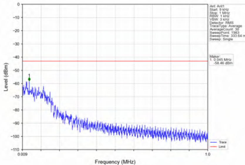
n66_15kHz_SISO_NTNV_20MHz_CP-OFDM QPSK_1720MHz_Inner_1RB_Left
