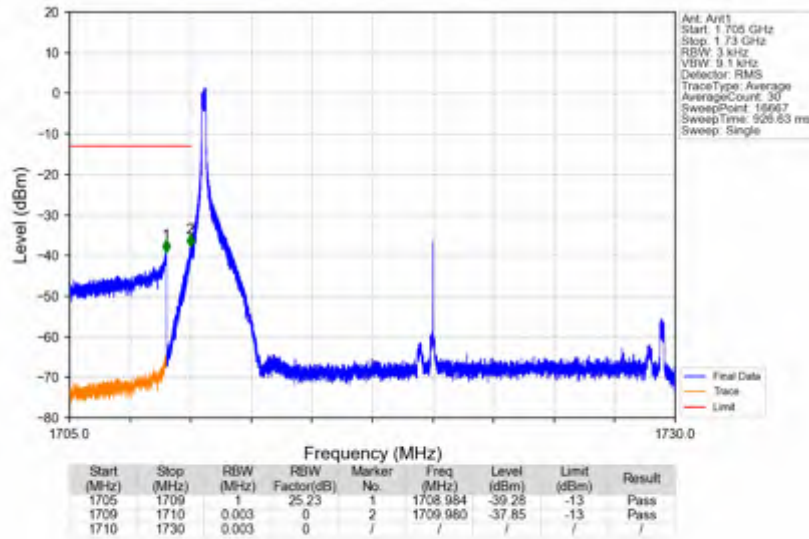
n66_15kHz_SISO_NTNV_20MHz_CP-OFDM QPSK_1720MHz_Edge_1RB_Left
