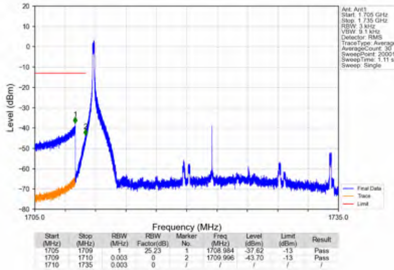
n66_15kHz_SISO_NTV_25MHz_CP-OFDM QPSK_1722.5MHz_Inner_1RB_Left
