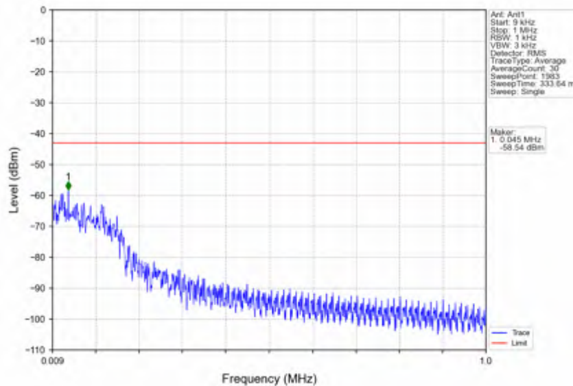
n66_15kHz_SISO_NTV_25MHz_CP-OFDM QPSK_1722.5MHz_Inner_1RB_Left
