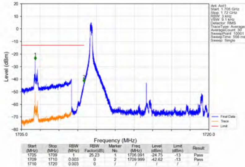
n66_15kHz_SISO_NTNV_10MHz_DFT-s-OFDM PI/2 BPSK_1715MHz_Inner_1RB_Left
