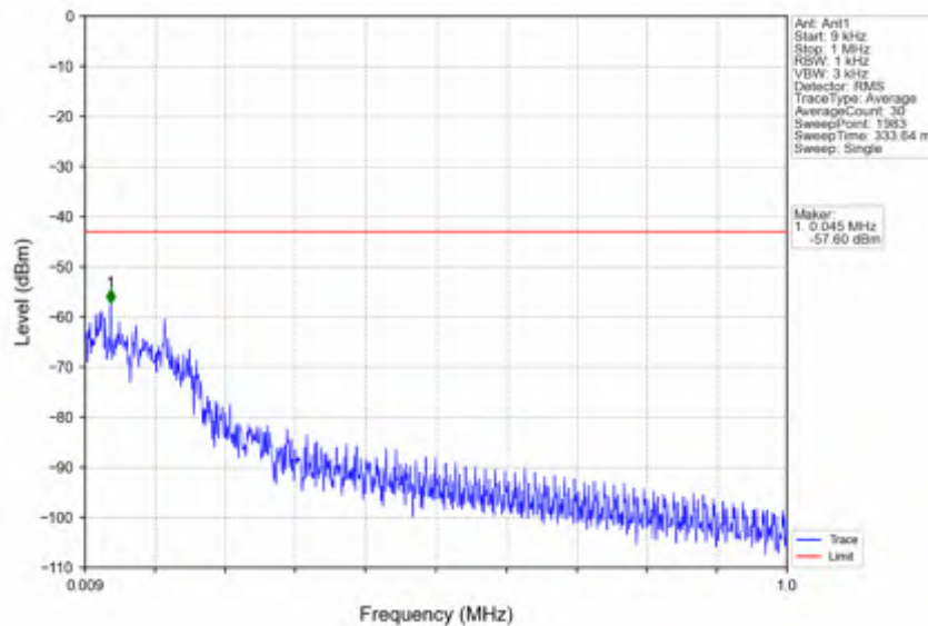
n66_15kHz_SISO_NTV_10MHz_CP-OFDM QPSK_1775MHz_Inner_1RB_Right
