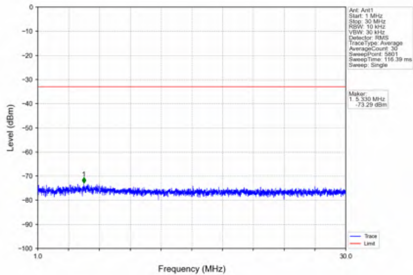
n41_30kHz_SISO_NTV_100MHz_CP-OFDM QPSK_2546.01MHz_Inner_1RB_Left
