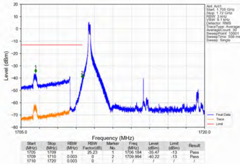
n66_15kHz_SISO_NTNV_10MHz_DFT-s-OFDM QPSK_1715MHz_Inner_1RB_Left
