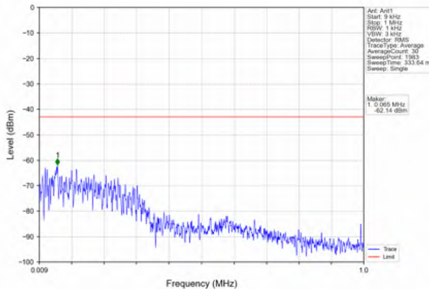
n41_30kHz_SISO_NTV_100MHz_CP-OFDM QPSK_2546.01MHz_Inner_1RB_Left
