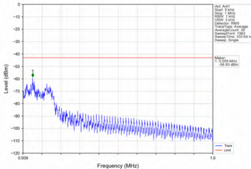
n66_15kHz_SISO_NTNV_10MHz_DFT-s-OFDM PI/2 BPSK_1715MHz_Inner_1RB_Left
