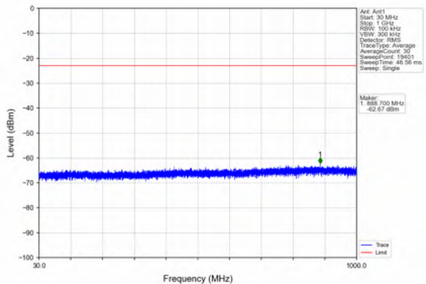
n41_30kHz_SISO_NTNV_90MHz_CP-OFDM QPSK_2541MHz_Inner_1RB_Left
