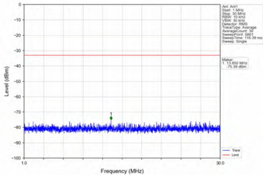
n66_15kHz_SISO_NTNV_10MHz_CP-OFDM QPSK_1775MHz_Inner_1RB_Right
