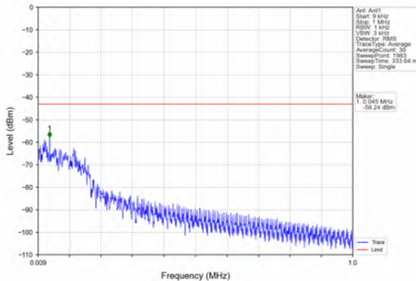
n66_15kHz_SISO_NTNV_10MHz_CP-OFDM QPSK_1715MHz_Inner_1RB_Left
