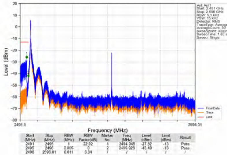
n41_30kHz_SISO_NTV_100MHz_CP-OFDM QPSK_2546.01MHz_Inner_1RB_Left
