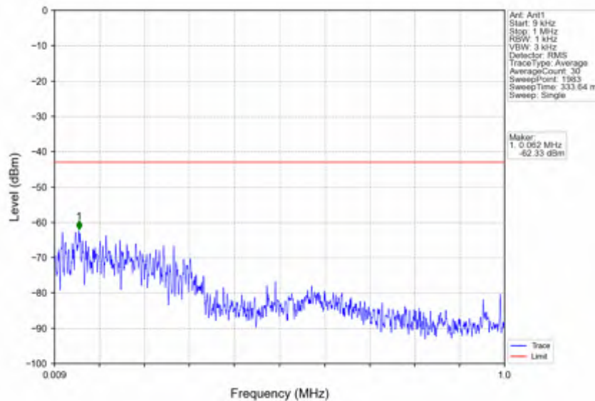
n41_30kHz_SISO_NTNV_90MHz_CP-OFDM QPSK_2541MHz_Inner_1RB_Left
