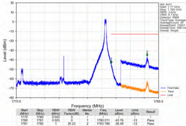
n66_15kHz_SISO_NTV_10MHz_CP-OFDM QPSK_1775MHz_Inner_1RB_Right
