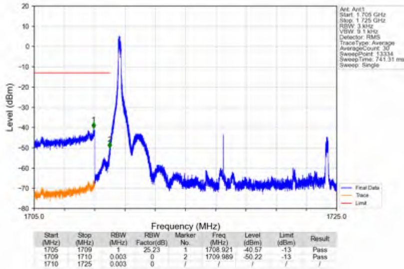
n66_15kHz_SISO_NTNV_15MHz_DFT-s-OFDM PI/2 BPSK_1717.5MHz_Inner_1RB_Left
