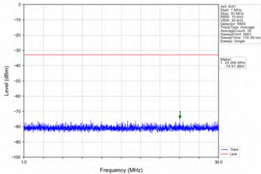
n66_15kHz_SISO_NTNV_10MHz_CP-OFDM QPSK_1715MHz_Inner_1RB_Left
