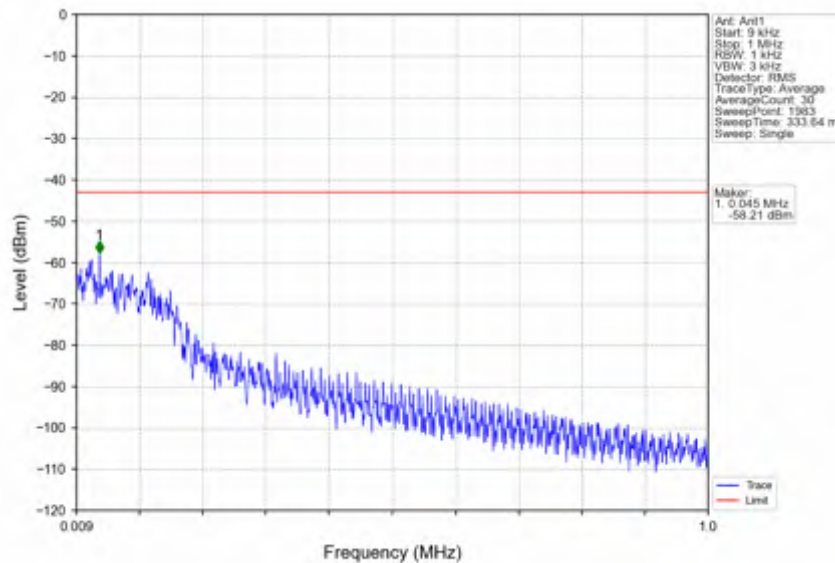
n66_15kHz_SISO_NTNV_5MHz_CP-OFDM QPSK_1712.5MHz_Inner_1RB_Left
