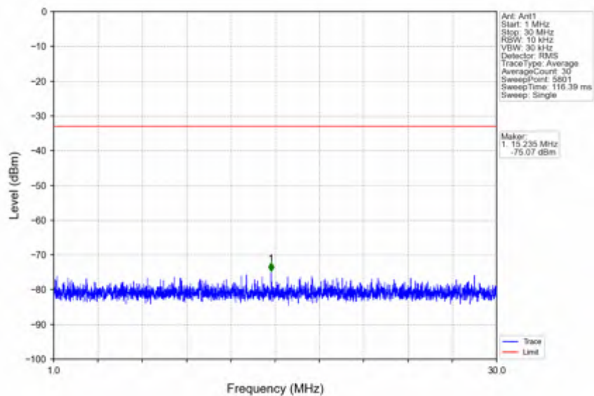
n66_15kHz_SISO_NTNV_10MHz_DFT-s-OFDM QPSK_1715MHz_Inner_1RB_Left
