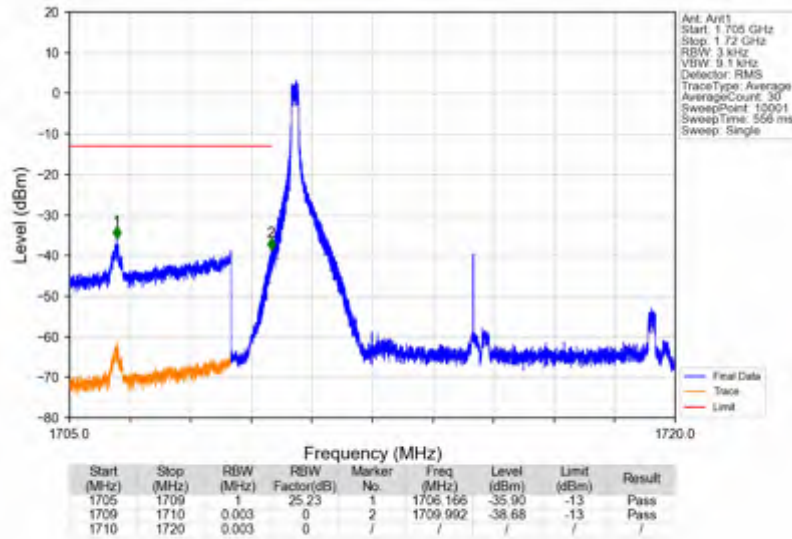
n66_15kHz_SISO_NTNV_10MHz_CP-OFDM QPSK_1715MHz_Inner_1RB_Left
