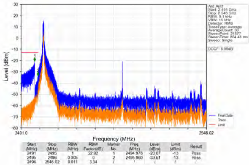
n41_30kHz_SISO_NTNV_50MHz_DFT-s-OFDM QPSK_2521.02MHz_Inner_1RB_Left
