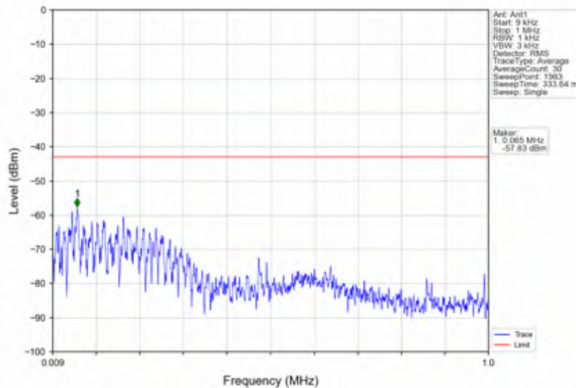
n41_30kHz_SISO_NTV_80MHz_CP-OFDM QPSK_2649.99MHz_Inner_1RB_Right
