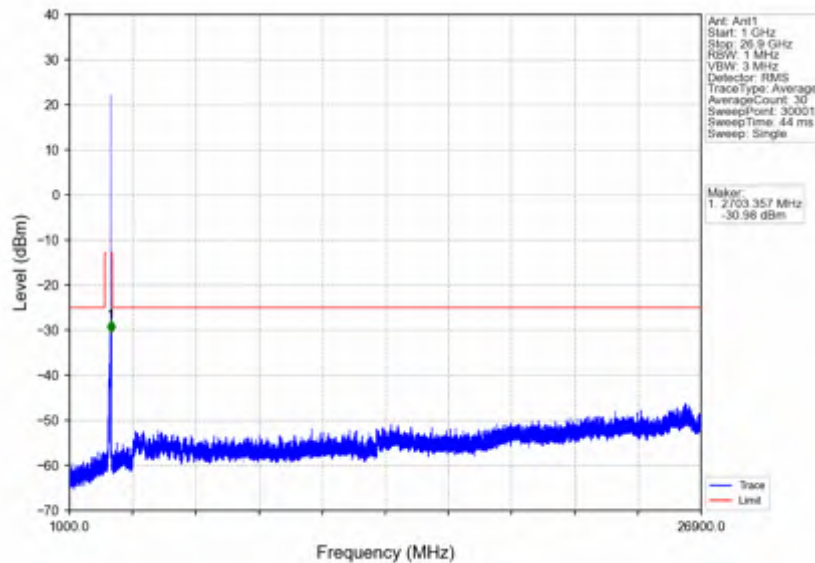
n41_30kHz_SISO_NTV_60MHz_DFT-s-OFDM_QPSK_2659.98MHz_Inner_1RB_Right
