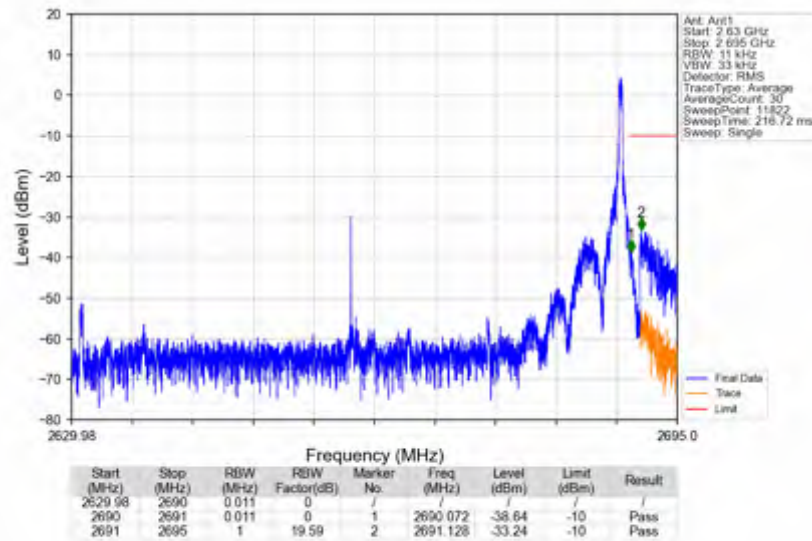
n41_30kHz_SISO_NTV_60MHz_CP-OFDM QPSK_2659.98MHz_Edge_1RB_Right
