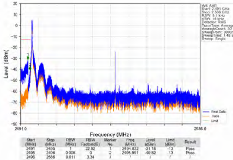
n41_30kHz_SISO_NTNV_90MHz_CP-OFDM QPSK_2541MHz_Edge_1RB_Left
