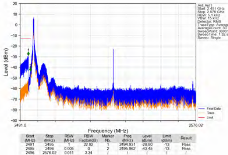
n41_30kHz_SISO_NTNV_80MHz_CP-OFDM QPSK_2536.02MHz_Inner_1RB_Left
