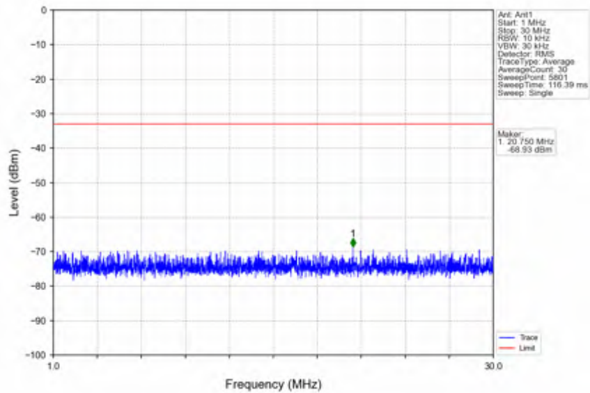
n41_30kHz_SISO_NTNV_60MHz_CP-OFDM QPSK_2526MHz_Edge_1RB_Left
