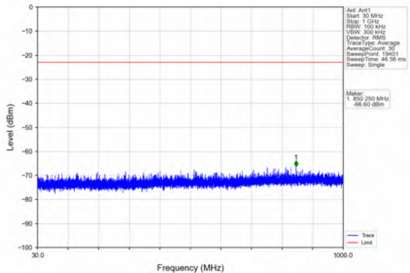
n41_30kHz_SISO_NTNV_60MHz_CP-OFDM QPSK_2526MHz_Inner_1RB_Left
