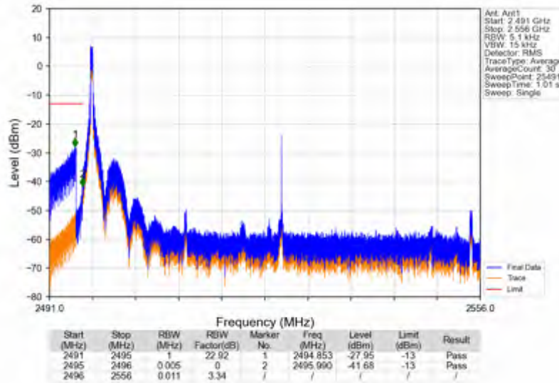
n41_30kHz_SISO_NTNV_60MHz_CP-OFDM QPSK_2526MHz_Inner_1RB_Left
