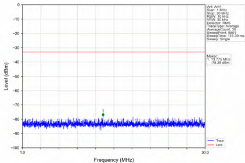
n41_30kHz_SISO_NTNV_50MHz_DFT-s-OFDM QPSK_2521.02MHz_Inner_1RB_Left
