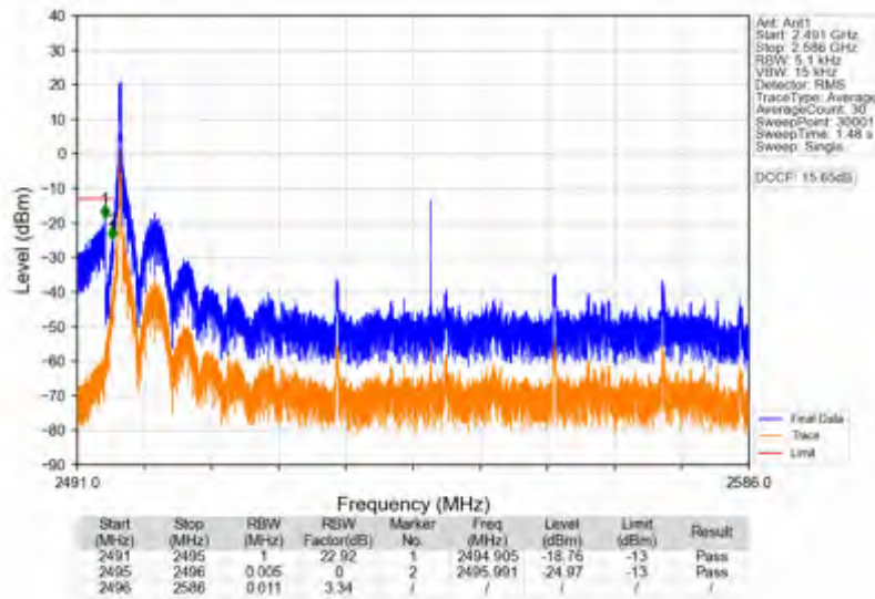
n41_30kHz_SISO_NTNV_90MHz_DFT-s-OFDM QPSK_2541MHz_Edge_1RB_Left
