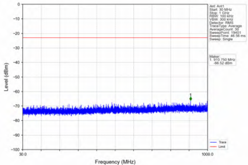
n41_30kHz_SISO_NTNV_80MHz_CP-OFDM QPSK_2536.02MHz_Inner_1RB_Left
