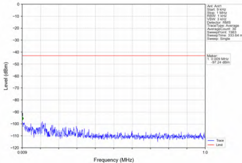
n41_30kHz_SISO_NTNV_80MHz_DFT-s-OFDM PI/2 BPSK_2536.02MHz_Inner_1RB_Left
