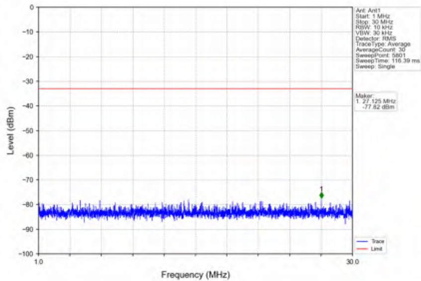
n41_30kHz_SISO_NTNV_60MHz_DFT-s-OFDM PI/2 BPSK_2526MHz_Inner_1RB_Left
