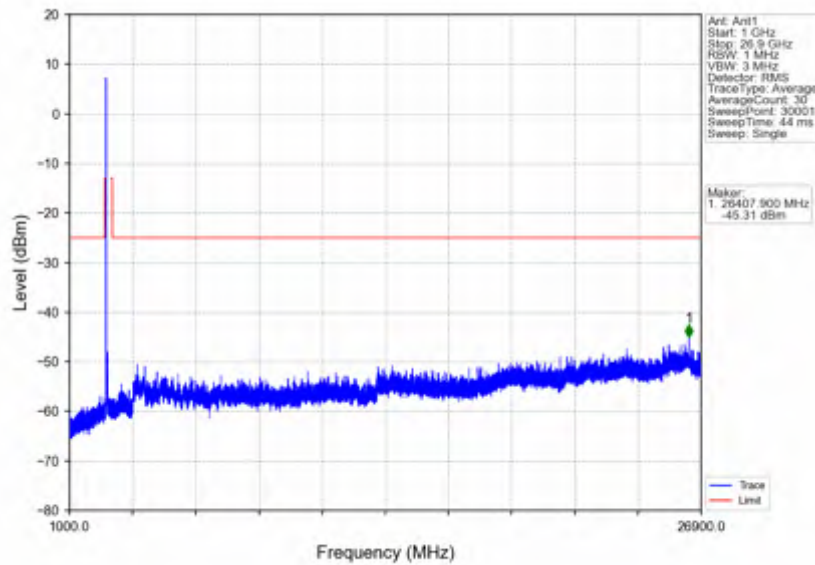
n41_30kHz_SISO_NTNV_60MHz_DFT-s-OFDM PI/2 BPSK_2592.99MHz_Edge_1RB_Left
