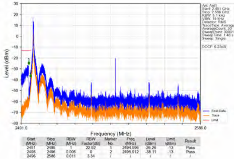
n41_30kHz_SISO_NTNV_90MHz_DFT-s-OFDM PI/2 BPSK_2541MHz_Inner_1RB_Left
