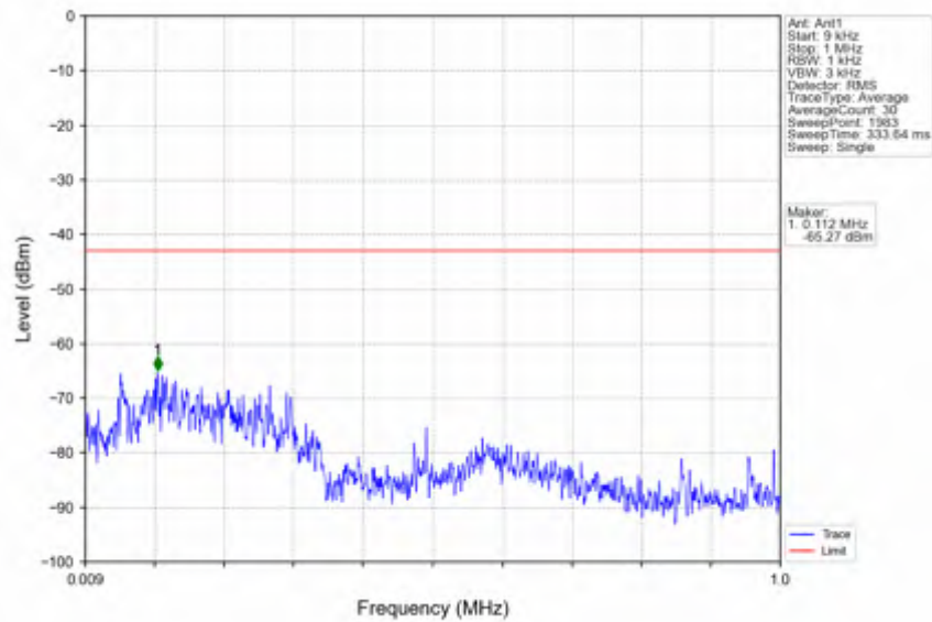
n41_30kHz_SISO_NTNV_90MHz_DFT-s-OFDM_QPSK_2541MHz_Inner_1RB_Left
