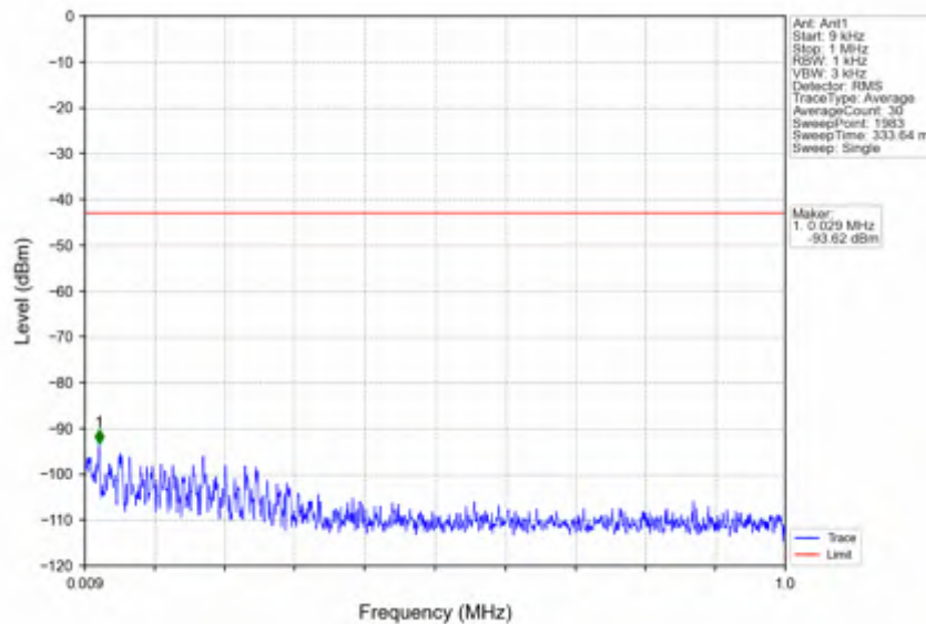
n41_30kHz_SISO_NTNV_60MHz_CP-OFDM QPSK_2526MHz_Inner_1RB_Left
