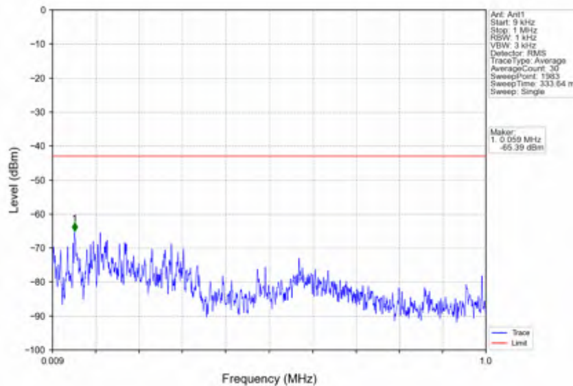
n41_30kHz_SISO_NTNV_90MHz_DFT-s-OFDM PI/2 BPSK_2541MHz_Inner_1RB_Left
