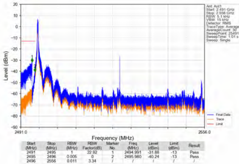
n41_30kHz_SISO_NTNV_60MHz_DFT-s-OFDM QPSK_2526MHz_Edge_1RB_Left
