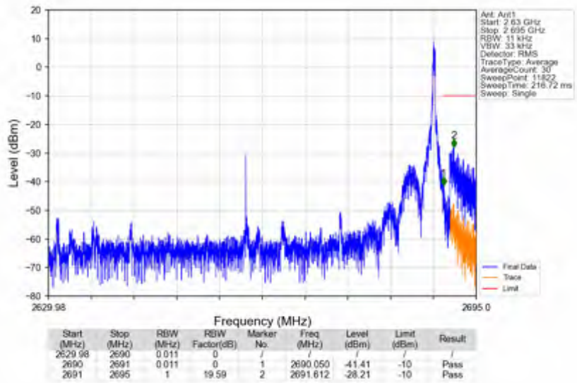
n41_30kHz_SISO_NTNV_60MHz_DFT-s-OFDM QPSK_2659.98MHz_Inner_1RB_Right
