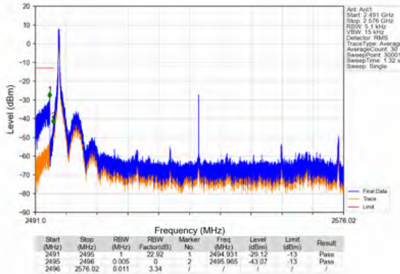
n41_30kHz_SISO_NTNV_80MHz_DFT-s-OFDM PI/2 BPSK_2536.02MHz_Inner_1RB_Left
