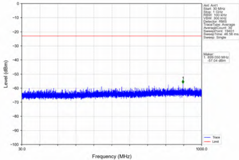
n41_30kHz_SISO_NTNV_60MHz_CP-OFDM QPSK_2592.99MHz_Edge_1RB_Left
