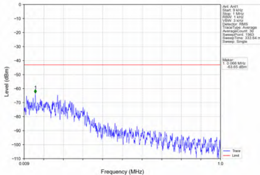
n41_30kHz_SISO_NTV_60MHz_CP-OFDM QPSK_2659.98MHz_Edge_1RB_Right
