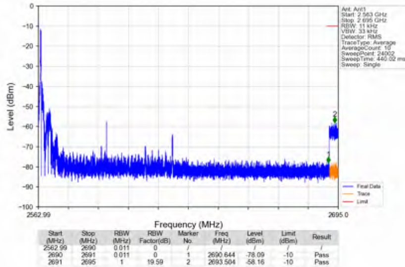
n41_30kHz_SISO_NTNV_60MHz_DFT-s-OFDM QPSK_2592.99MHz_Edge_1RB_Left
