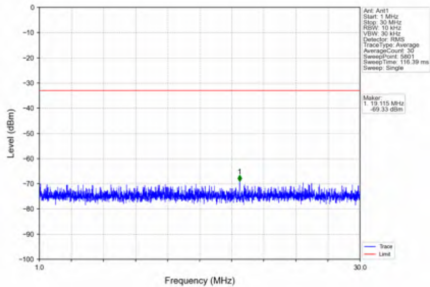
n41_30kHz_SISO_NTV_60MHz_CP-OFDM QPSK_2659.98MHz_Edge_1RB_Right
