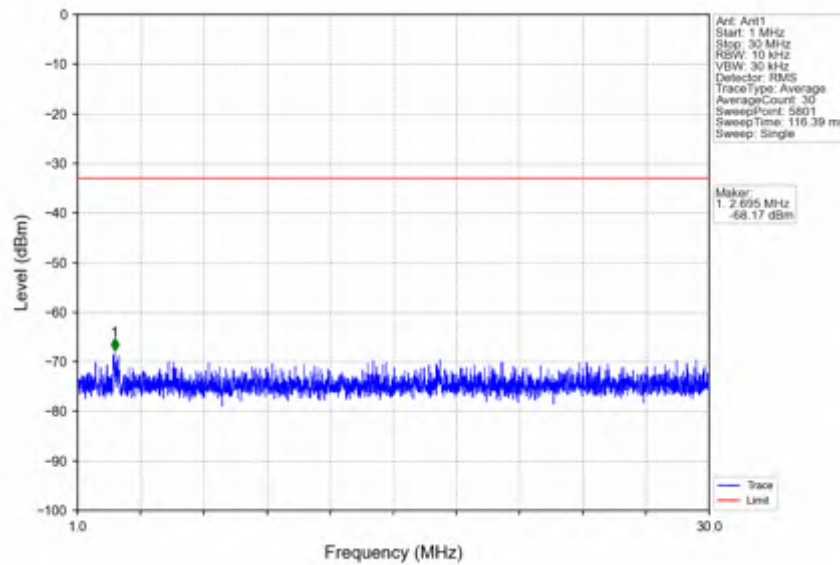
n41_30kHz_SISO_NTNV_60MHz_DFT-s-OFDM QPSK_2592.99MHz_Edge_1RB_Left
