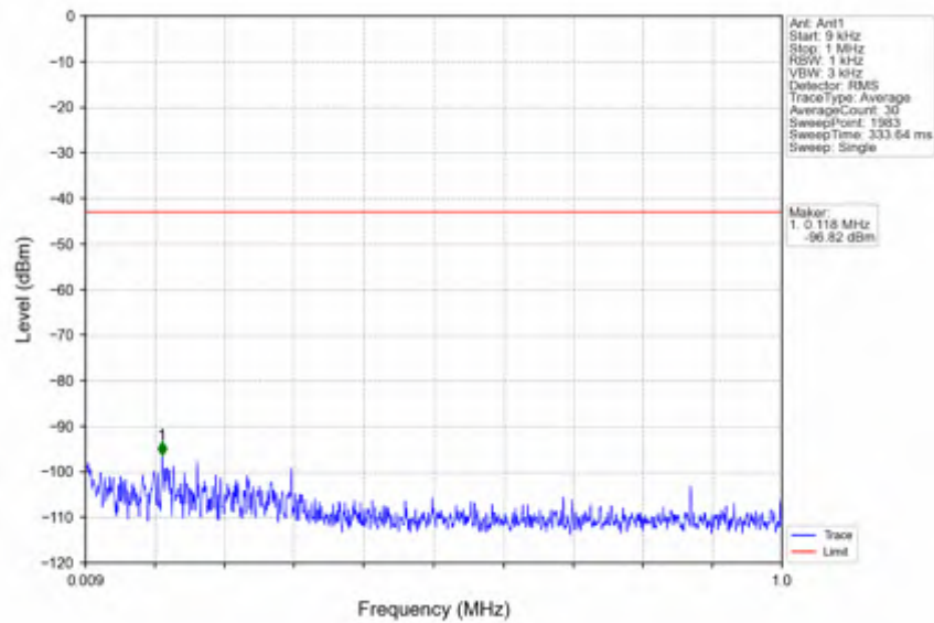
n41_30kHz_SISO_NTNV_80MHz_DFT-s-OFDM QPSK_2536.02MHz_Inner_1RB_Left
