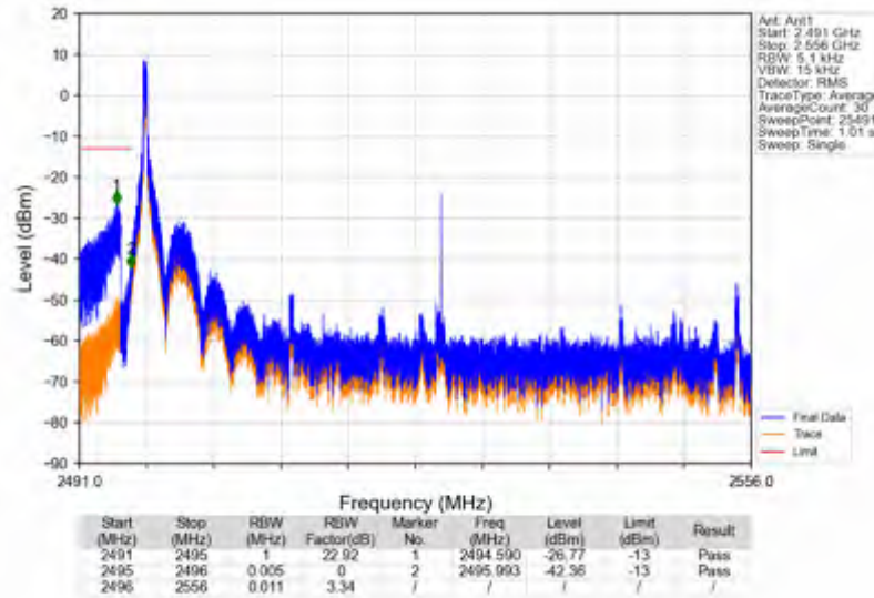
n41_30kHz_SISO_NTNV_60MHz_DFT-s-OFDM_PI/2_BPSK_2526MHz_Inner_1RB_Left
