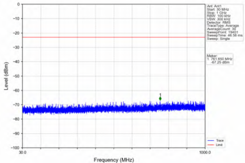
n41_30kHz_SISO_NTNV_50MHz_CP-OFDM QPSK_2521.02MHz_Inner_1RB_Left
