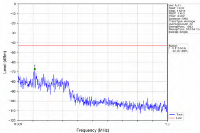
n41_30kHz_SISO_NTNV_60MHz_DFT-s-OFDM_PI/2_BPSK_2526MHz_Edge_1RB_Left
