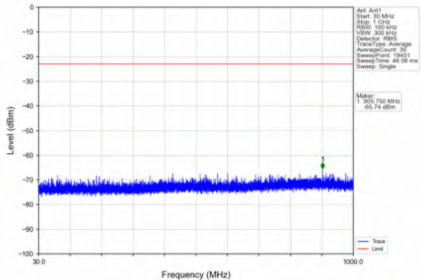
n41_30kHz_SISO_NTV_60MHz_CP-OFDM QPSK_2659.98MHz_Inner_1RB_Right
