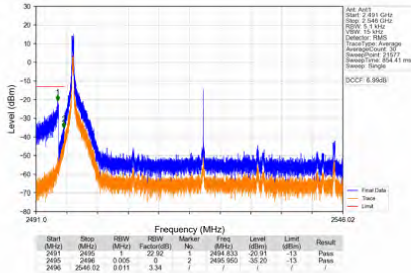
n41_30kHz_SISO_NTNV_50MHz_CP-OFDM QPSK_2521.02MHz_Inner_1RB_Left
