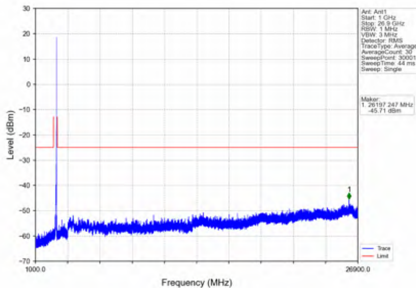
n41_30kHz_SISO_NTV_60MHz_DFT-s-OFDM QPSK_2659.98MHz_Edge_1RB_Right
