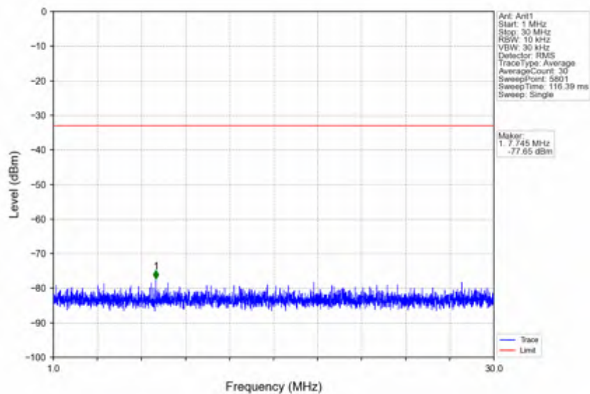
n41_30kHz_SISO_NTV_60MHz_DFT-s-OFDM_QPSK_2659.98MHz_Inner_1RB_Right
