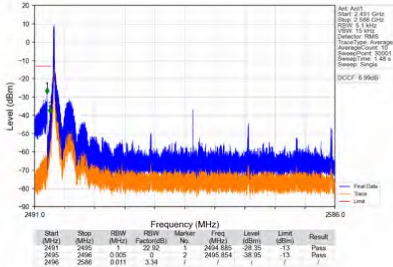
n41_30kHz_SISO_NTNV_90MHz_DFT-s-OFDM_PI/2_BPSK_2541MHz_Edge_1RB_Left
