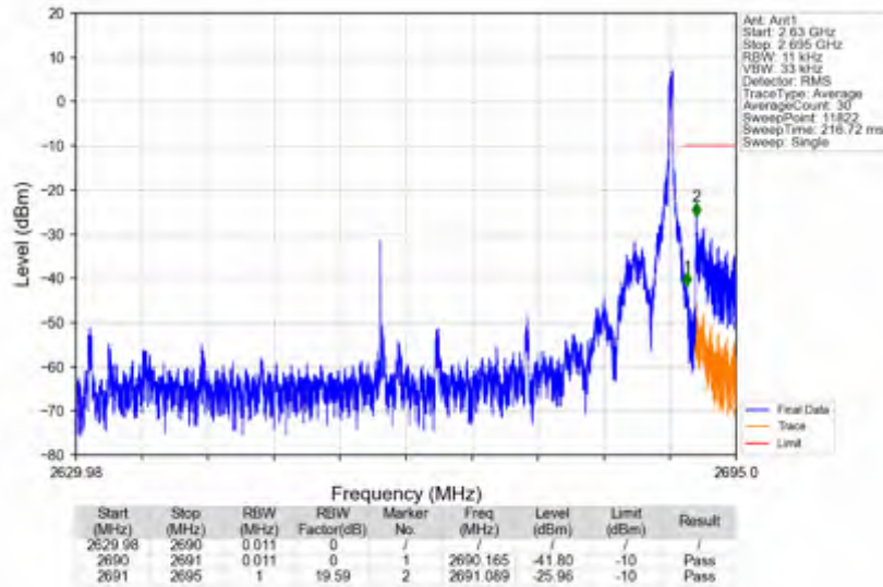
n41_30kHz_SISO_NTNV_60MHz_DFT-s-OFDM PI/2 BPSK_2659.98MHz_Inner_1RB_Right
