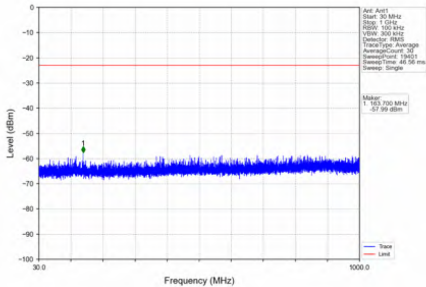
n41_30kHz_SISO_NTNV_60MHz_DFT-s-OFDM PI/2 BPSK_2592.99MHz_Edge_1RB_Left
