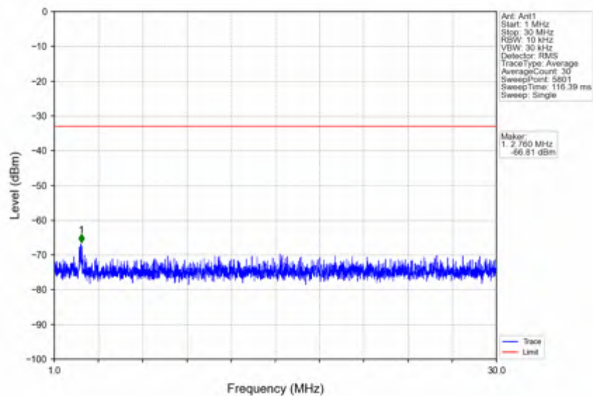
n41_30kHz_SISO_NTNV_60MHz_CP-OFDM QPSK_2592.99MHz_Edge_1RB_Left
