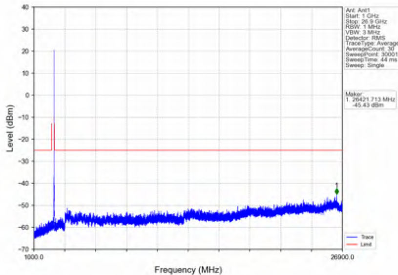
n41_30kHz_SISO_NTV_20MHz_DFT-s-OFDM QPSK_2679.99MHz_Inner_1RB_Right
