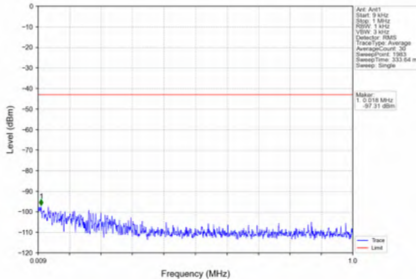
n41_30kHz_SISO_NTNV_40MHz_CP-OFDM_QPSK_2670MHz_Inner_1RB_Right
