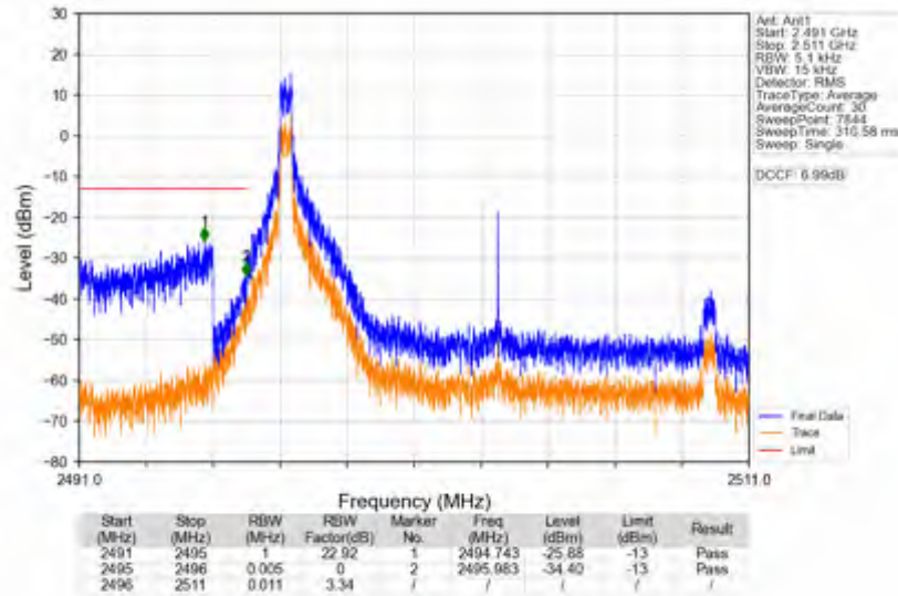
n41_30kHz_SISO_NTNV_15MHz_CP-OFDM QPSK_2503.5MHz_Inner_1RB_Left
