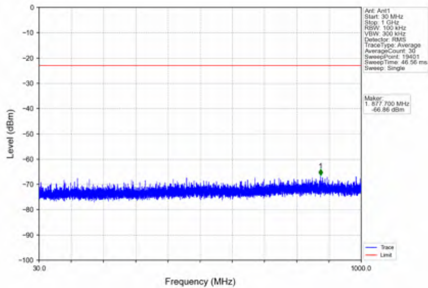
n41_30kHz_SISO_NTNV_40MHz_DFT-s-OFDM QPSK_2516.01MHz_Inner_1RB_Left
