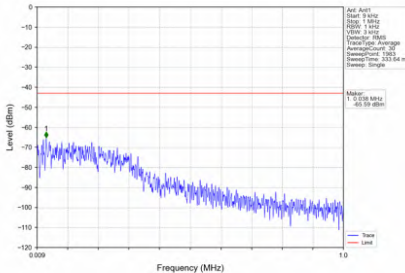
n41_30kHz_SISO_NTV_40MHz_CP-OFDM QPSK_2670MHz_Edge_1RB_Right
