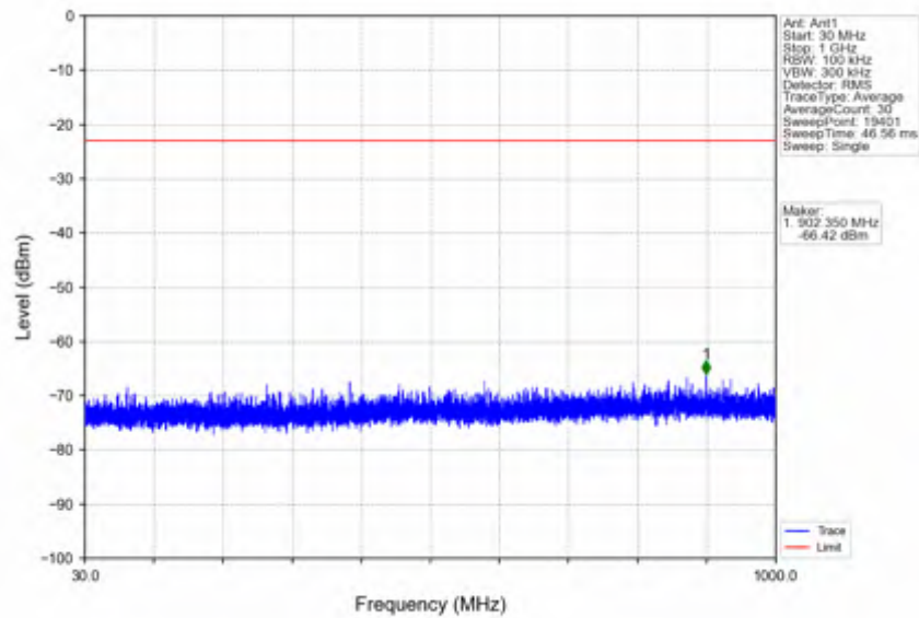
n41_30kHz_SISO_NTNV_20MHz_DFT-s-OFDM QPSK_2506.02MHz_Inner_1RB_Left
