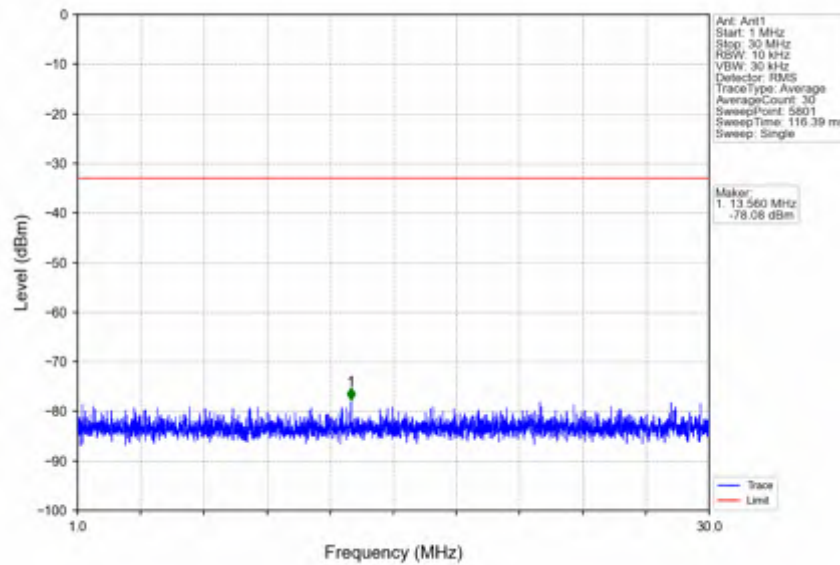
n41_30kHz_SISO_NTV_20MHz_CP-OFDM QPSK_2679.99MHz_Inner_1RB_Right
