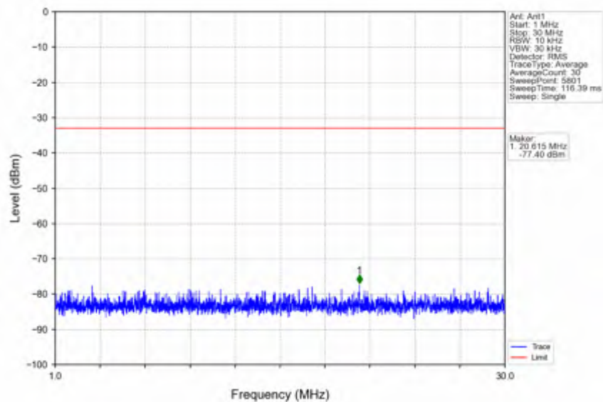
n41_30kHz_SISO_NTV_20MHz_DFT-s-OFDM_QPSK_2679.99MHz_Inner_1RB_Right
