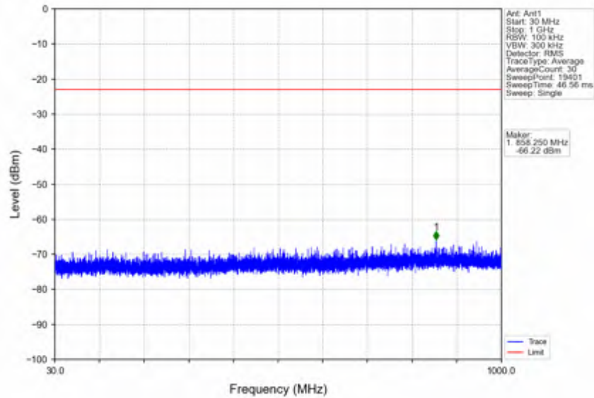
n41_30kHz_SISO_NTNV_40MHz_DFT-s-OFDM QPSK_2670MHz_Inner_1RB_Right
