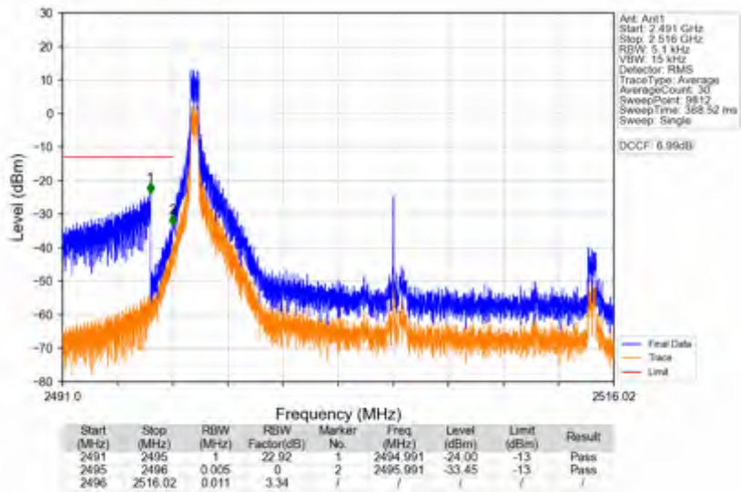
n41_30kHz_SISO_NTNV_20MHz_DFT-s-OFDM QPSK_2506.02MHz_Edge_1RB_Left
