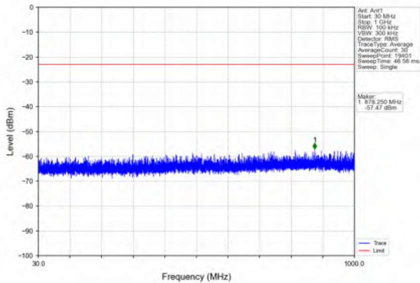
n41_30kHz_SISO_NTNV_20MHz_DFT-s-OFDM QPSK_2506.02MHz_Edge_1RB_Left
