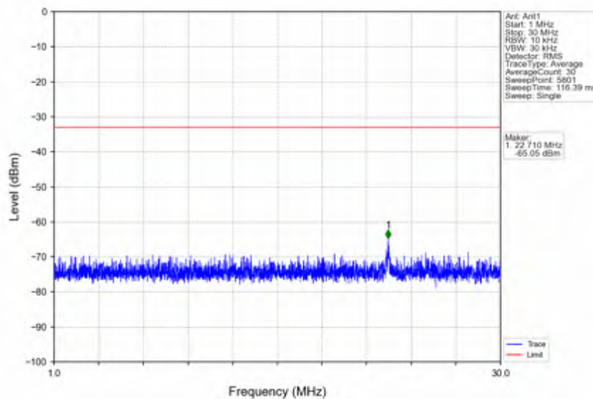
n41_30kHz_SISO_NTNV_20MHz_CP-OFDM QPSK_2592.99MHz_Edge_1RB_Left
