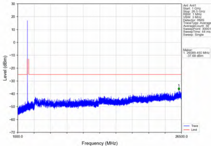
n41_30kHz_SISO_NTNV_20MHz_DFT-s-OFDM QPSK_2506.02MHz_Edge_1RB_Left
