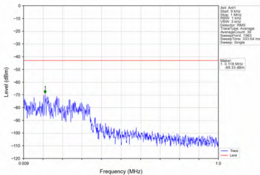
n41_30kHz_SISO_NTNV_30MHz_DFT-s-OFDM_PI/2_BPSK_2511MHz_Edge_1RB_Left
