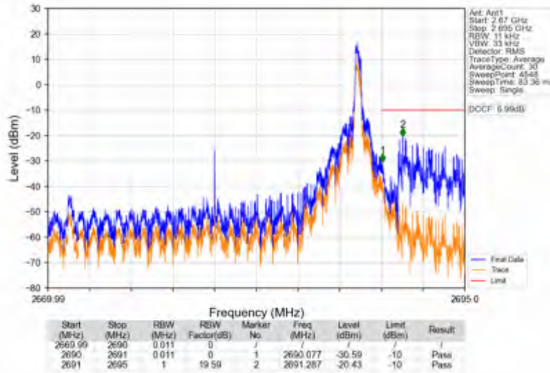
n41_30kHz_SISO_NTV_20MHz_CP-OFDM QPSK_2679.99MHz_Inner_1RB_Right
