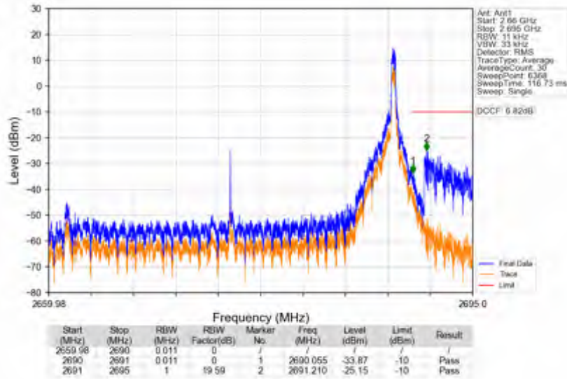
n41_30kHz_SISO_NTV_30MHz_CP-OFDM QPSK_2674.98MHz_Inner_1RB_Right
