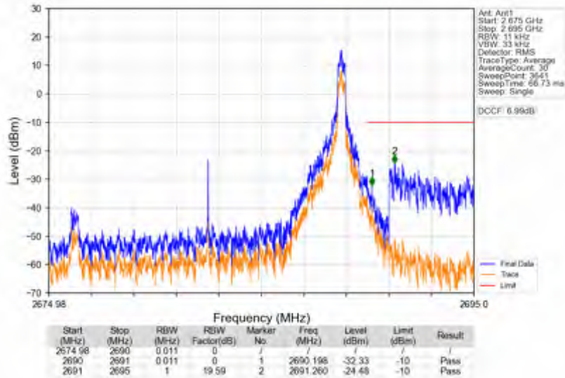
n41_30kHz_SISO_NTV_15MHz_CP-OFDM QPSK_2682.48MHz_Inner_1RB_Right
