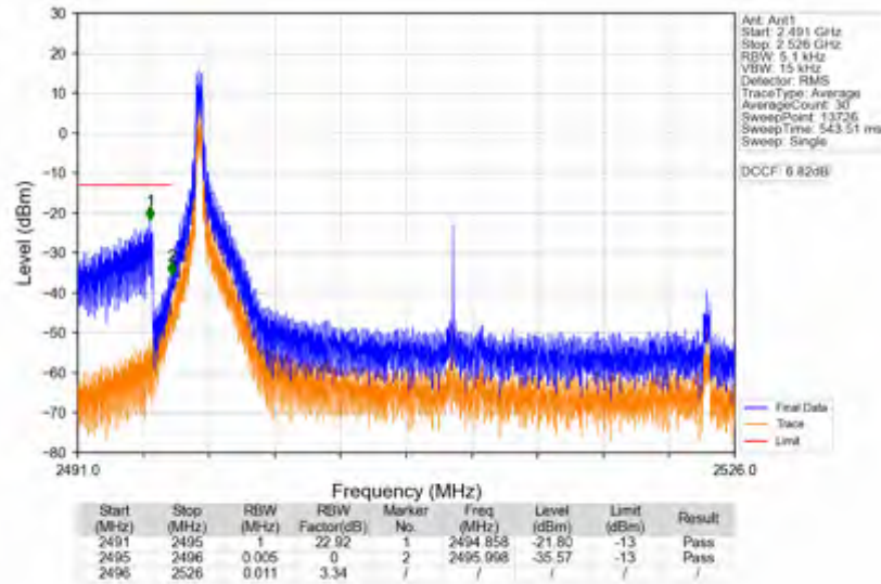
n41_30kHz_SISO_NTNV_30MHz_CP-OFDM QPSK_2511MHz_Inner_1RB_Left
