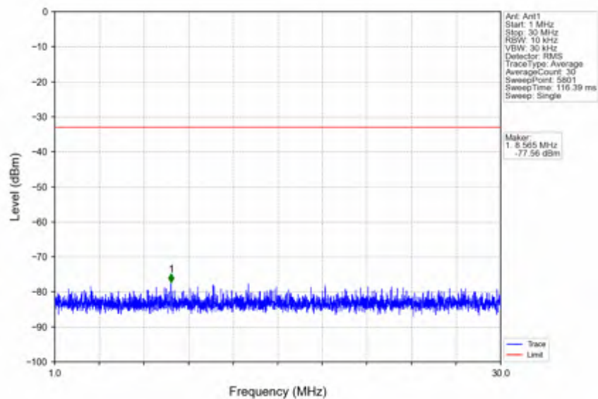
n41_30kHz_SISO_NTNV_30MHz_DFT-s-OFDM_QPSK_2511MHz_Inner_1RB_Left
