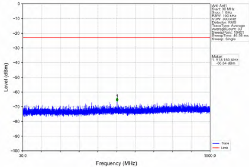
n41_30kHz_SISO_NTV_20MHz_DFT-s-OFDM QPSK_2679.99MHz_Inner_1RB_Right
