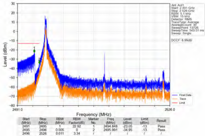
n41_30kHz_SISO_NTNV_30MHz_DFT-s-OFDM QPSK_2511MHz_Inner_1RB_Left
