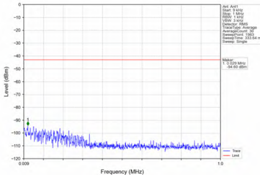
n41_30kHz_SISO_NTNV_20MHz_CP-OFDM QPSK_2506.02MHz_Inner_1RB_Left
