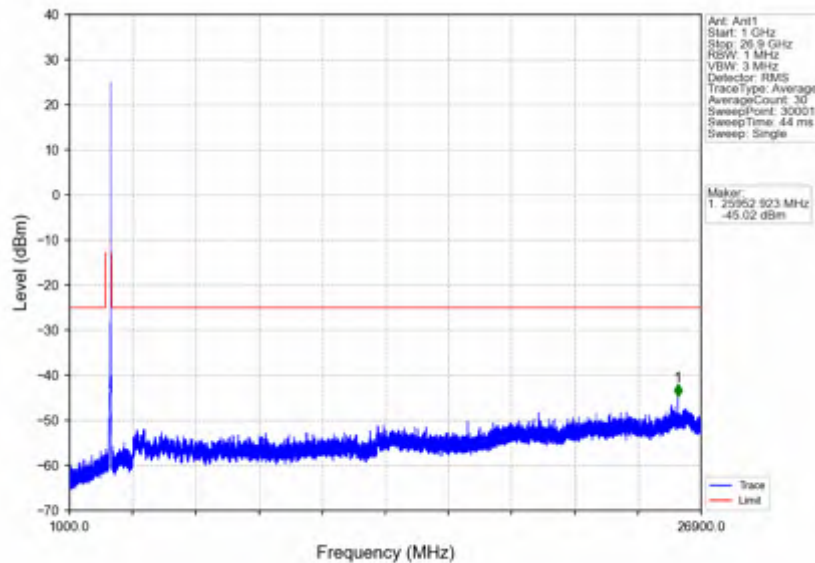
n41_30kHz_SISO_NTV_30MHz_DFT-s-OFDM QPSK_2674.98MHz_Inner_1RB_Right
