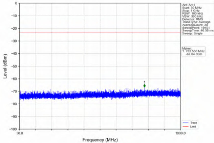
n41_30kHz_SISO_NTV_30MHz_DFT-s-OFDM QPSK_2674.98MHz_Inner_1RB_Right
