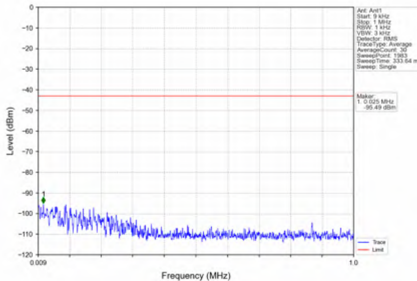
n41_30kHz_SISO_NTNV_40MHz_CP-OFDM QPSK_2516.01MHz_Inner_1RB_Left
