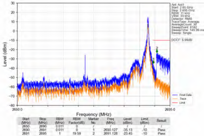
n41_30kHz_SISO_NTNV_40MHz_DFT-s-OFDM QPSK_2670MHz_Inner_1RB_Right
