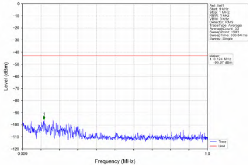
n41_30kHz_SISO_NTNV_20MHz_DFT-s-OFDM QPSK_2506.02MHz_Inner_1RB_Left
