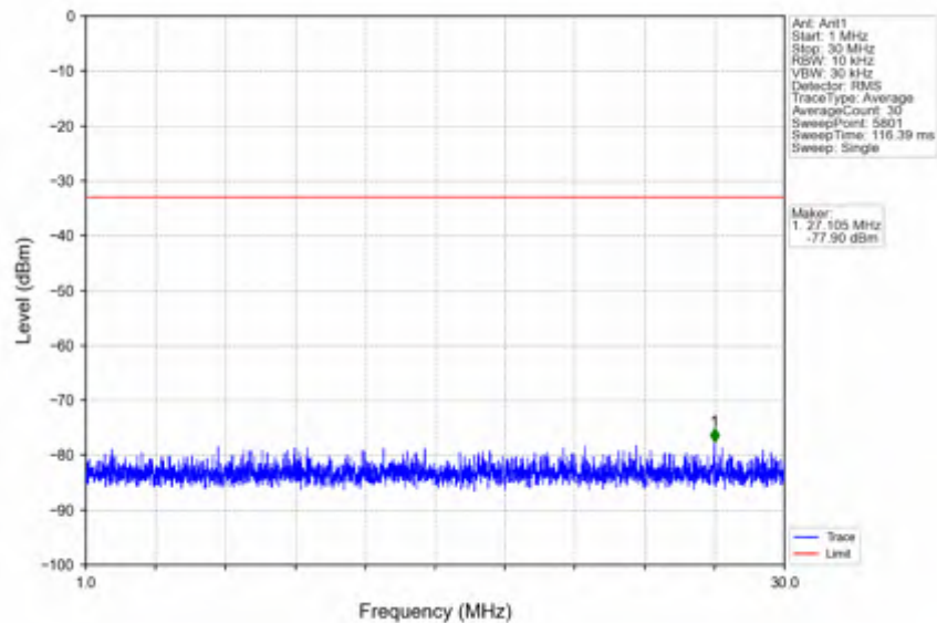
n41_30kHz_SISO_NTNV_40MHz_DFT-s-OFDM_QPSK_2670MHz_Inner_1RB_Right
