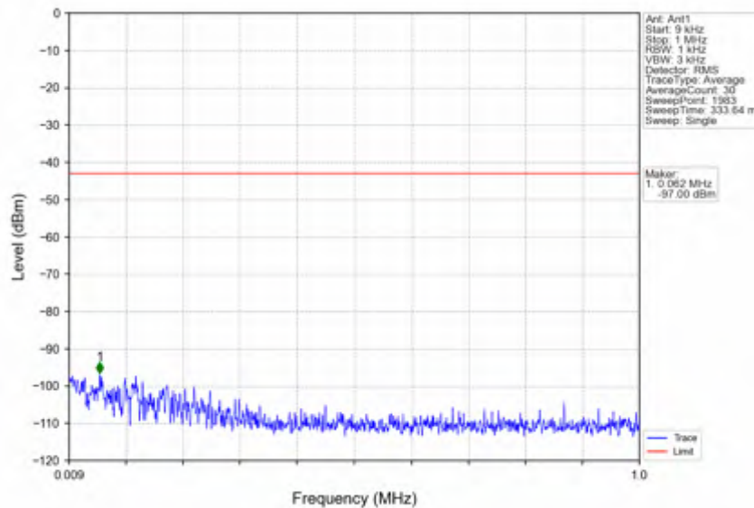
n41_30kHz_SISO_NTV_15MHz_CP-OFDM QPSK_2682.48MHz_Inner_1RB_Right
