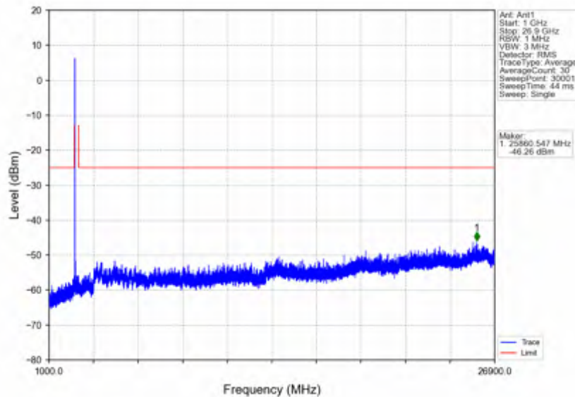
n41_30kHz_SISO_NTNV_30MHz_DFT-s-OFDM_QPSK_2511MHz_Inner_1RB_Left
