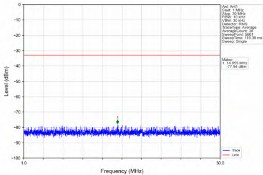
n41_30kHz_SISO_NTV_15MHz_CP-OFDM QPSK_2682.48MHz_Inner_1RB_Right
