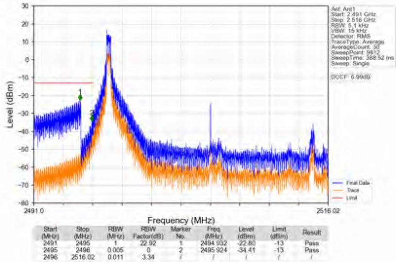
n41_30kHz_SISO_NTNV_20MHz_DFT-s-OFDM QPSK_2506.02MHz_Inner_1RB_Left
