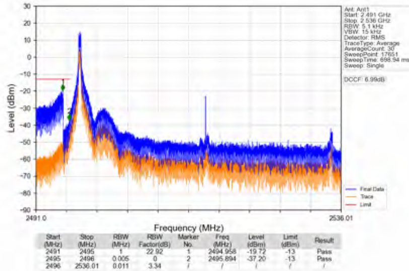
n41_30kHz_SISO_NTNV_40MHz_CP-OFDM QPSK_2516.01MHz_Inner_1RB_Left
