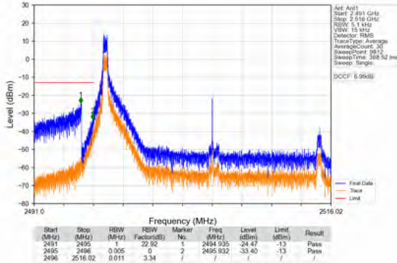
n41_30kHz_SISO_NTNV_20MHz_CP-OFDM QPSK_2506.02MHz_Edge_1RB_Left
