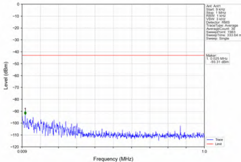
n41_30kHz_SISO_NTNV_30MHz_CP-OFDM QPSK_2511MHz_Inner_1RB_Left
