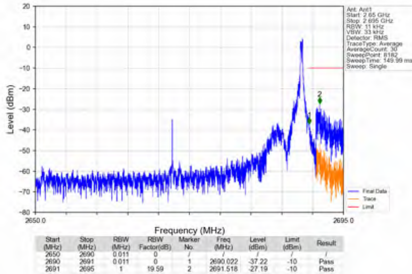
n41_30kHz_SISO_NTV_40MHz_CP-OFDM QPSK_2670MHz_Edge_1RB_Right
