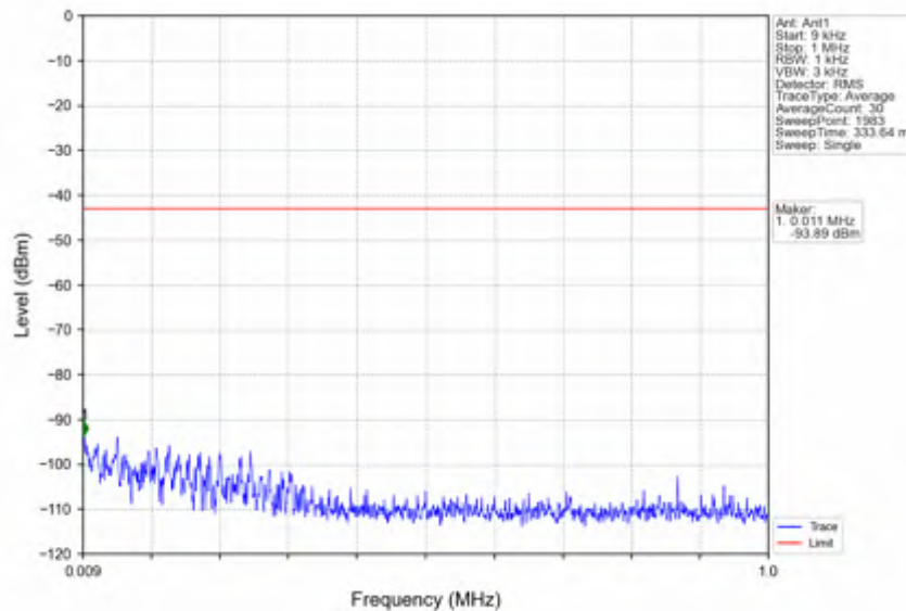
n41_30kHz_SISO_NTNV_15MHz_CP-OFDM QPSK_2503.5MHz_Inner_1RB_Left
