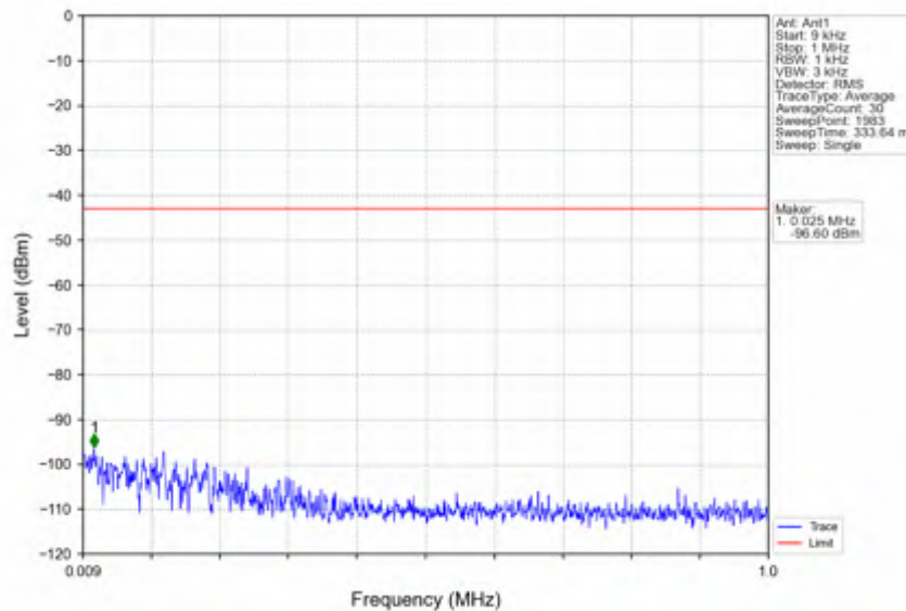
n41_30kHz_SISO_NTV_30MHz_CP-OFDM QPSK_2674.98MHz_Inner_1RB_Right
