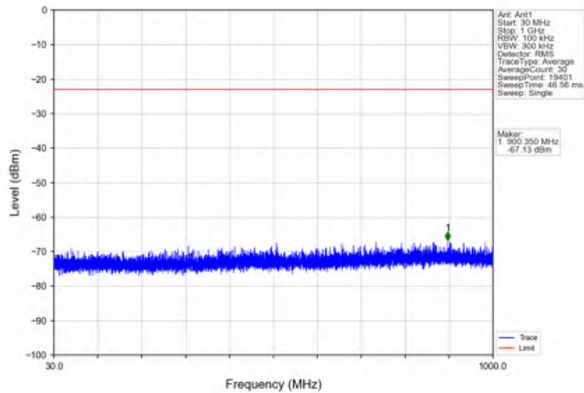
n41_30kHz_SISO_NTNV_30MHz_DFT-s-OFDM_QPSK_2511MHz_Inner_1RB_Left
