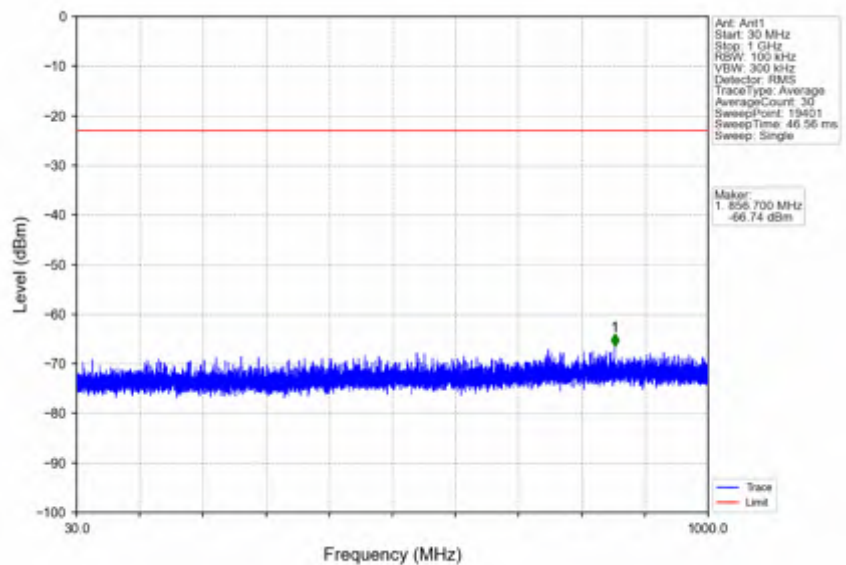
n41_30kHz_SISO_NTNV_40MHz_CP-OFDM QPSK_2670MHz_Inner_1RB_Right
