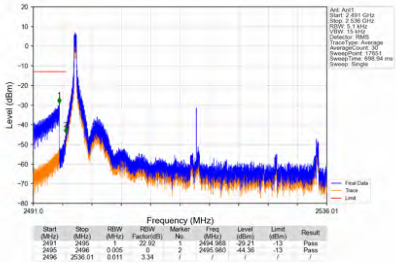
n41_30kHz_SISO_NTNV_40MHz_DFT-s-OFDM QPSK_2516.01MHz_Inner_1RB_Left
