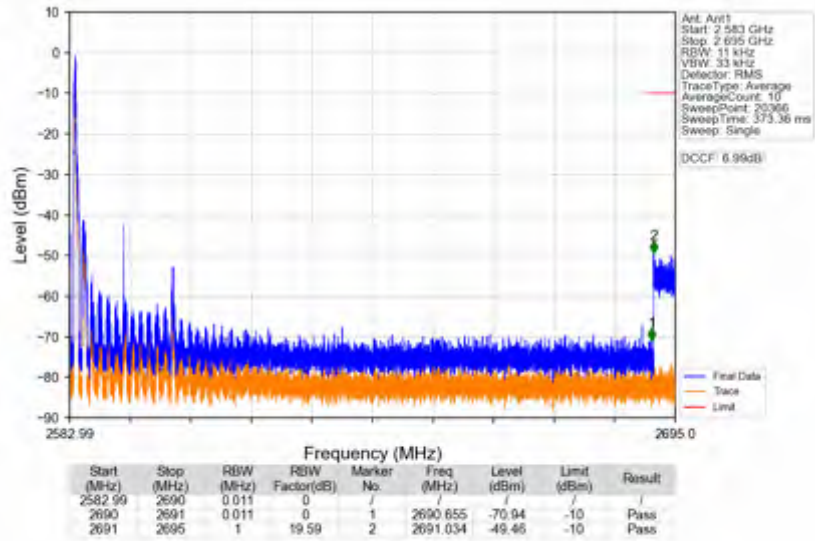
n41_30kHz_SISO_NTNV_20MHz_CP-OFDM QPSK_2592.99MHz_Edge_1RB_Left
