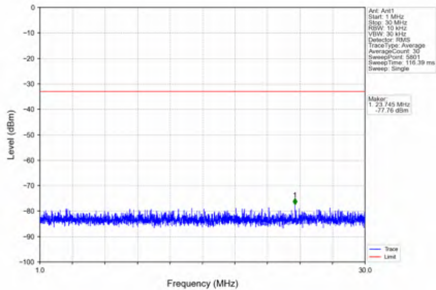
n41_30kHz_SISO_NTNV_40MHz_CP-OFDM QPSK_2516.01MHz_Inner_1RB_Left
