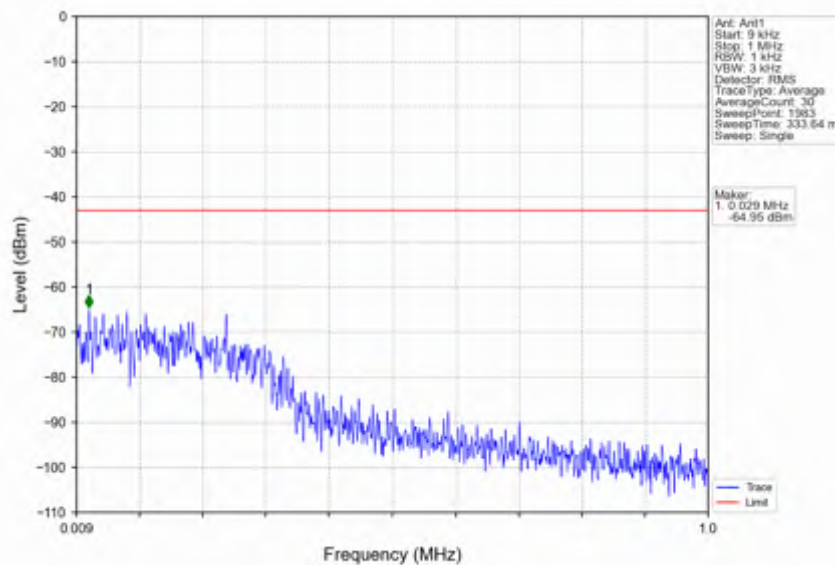
n41_30kHz_SISO_NTNV_20MHz_CP-OFDM QPSK_2506.02MHz_Edge_1RB_Left
