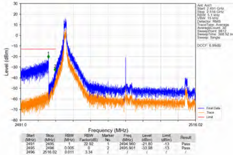
n41_30kHz_SISO_NTNV_20MHz_CP-OFDM QPSK_2506.02MHz_Inner_1RB_Left
