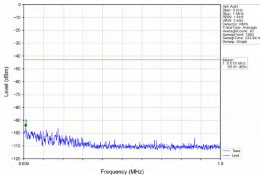
n41_30kHz_SISO_NTV_20MHz_CP-OFDM QPSK_2679.99MHz_Inner_1RB_Right
