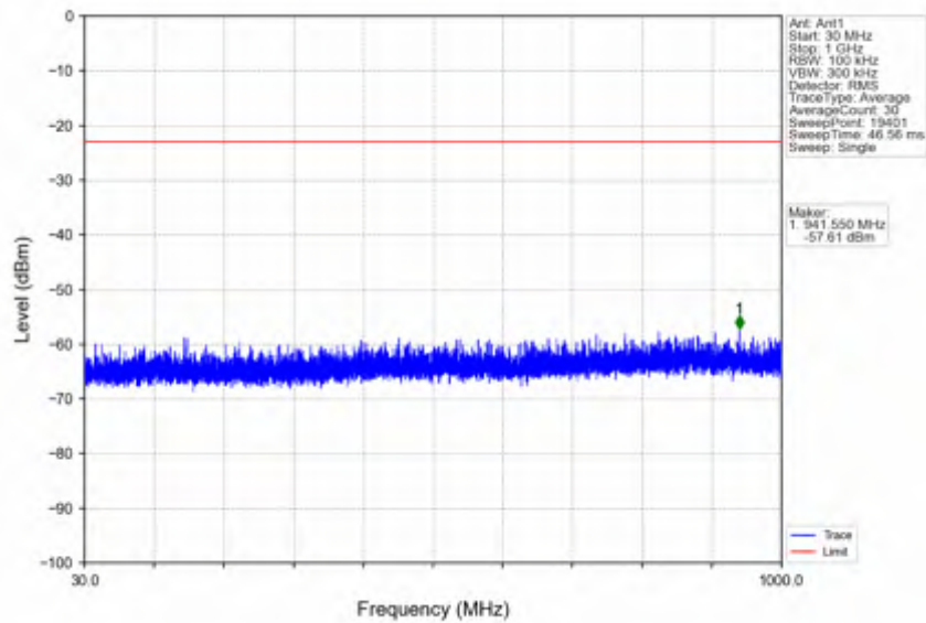
n41_15kHz_SISO_NTV_50MHz_DFT-s-OFDM QPSK_2521.005MHz_Edge_1RB_Left
