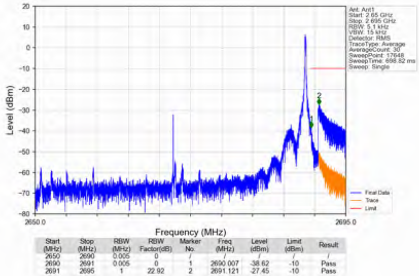
n41_15kHz_SISO_NTNV_40MHz_DFT-s-OFDM QPSK_2670MHz_Inner_1RB_Right
