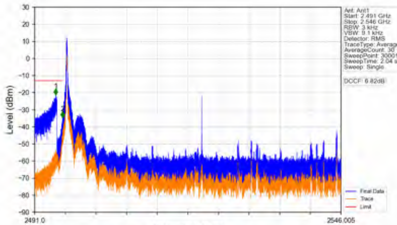
n41_15kHz_SISO_NTNV_50MHz_DFT-s-OFDM QPSK_2521.005MHz_Edge_1RB_Left
