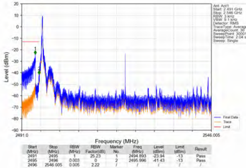
n41_15kHz_SISO_NTNV_50MHz_DFT-s-OFDM PI/2 BPSK_2521.005MHz_Inner_1RB_Left
