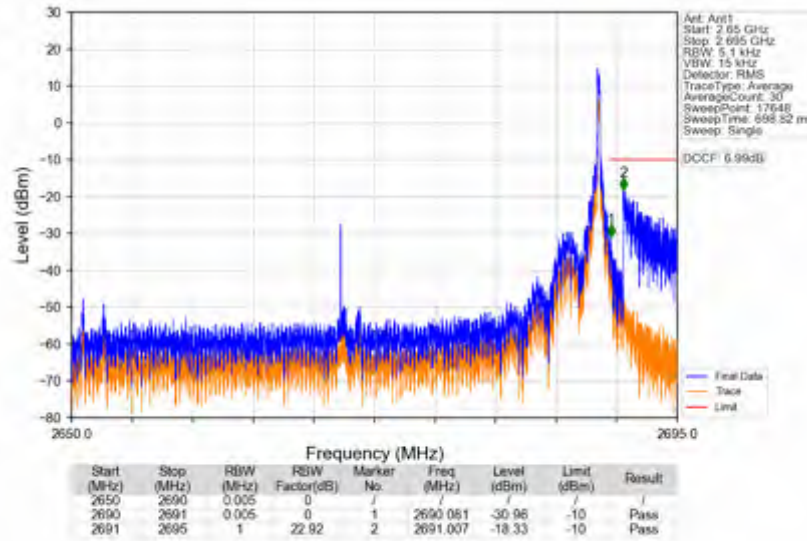
n41_15kHz_SISO_NTNV_40MHz_CP-OFDM QPSK_2670MHz_Inner_1RB_Right
