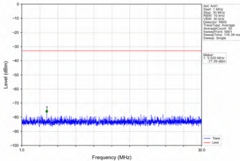
n41_30kHz_SISO_NTNV_10MHz_CP-OFDM QPSK_2501.01MHz_Inner_1RB_Left
