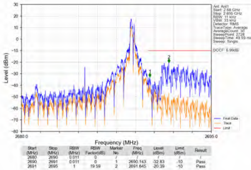
n41_30kHz_SISO_NTNV_10MHz_DFT-s-OFDM QPSK_2685MHz_Inner_1RB_Right
