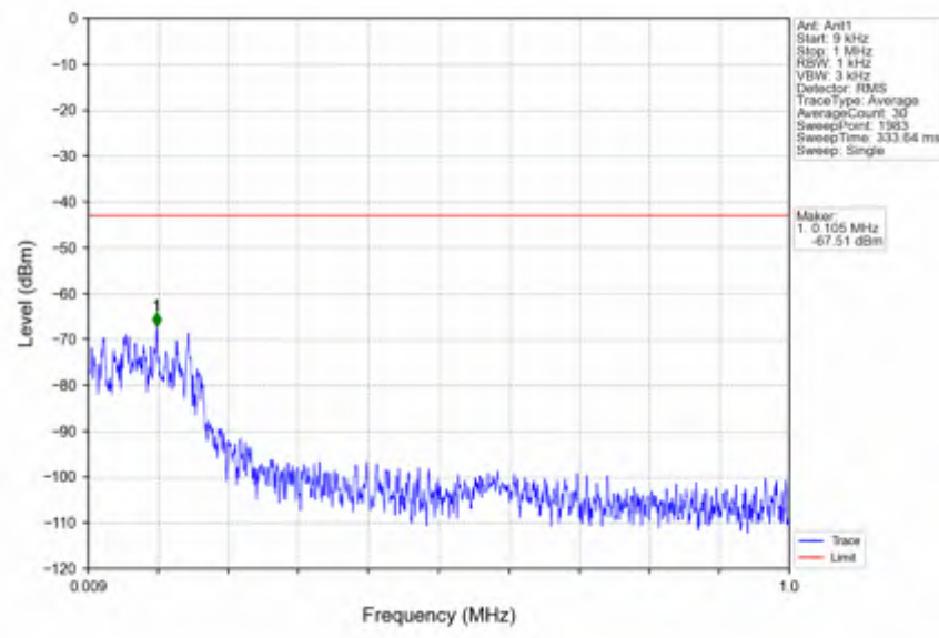
n41_15kHz_SISO_NTV_40MHz_DFT-s-OFDM_QPSK_2593.005MHz_Edge_1RB_Left
