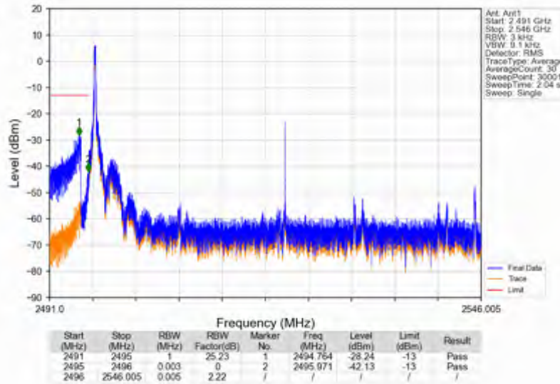
n41_15kHz_SISO_NTV_50MHz_CP-OFDM QPSK_2521.005MHz_Edge_1RB_Left
