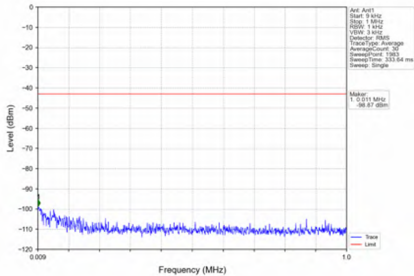
n41_15kHz_SISO_NTNV_40MHz_DFT-s-OFDM QPSK_2670MHz_Inner_1RB_Right
