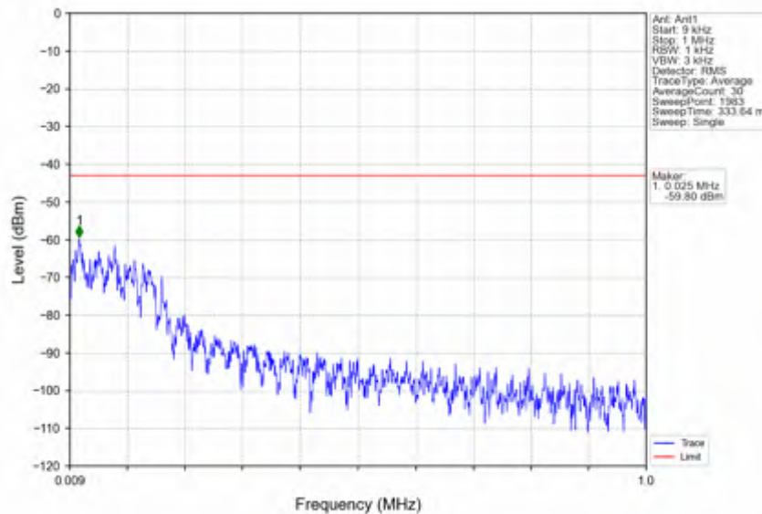
n41_15kHz_SISO_NTV_50MHz_CP-OFDM QPSK_2521.005MHz_Edge_1RB_Left
