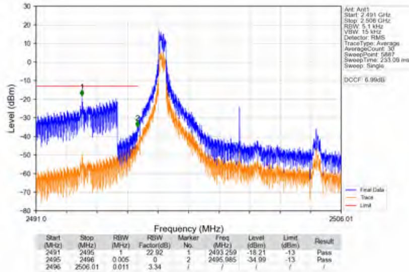
n41_30kHz_SISO_NTNV_10MHz_DFT-s-OFDM PI/2 BPSK_2501.01MHz_Inner_1RB_Left
