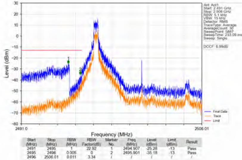
n41_30kHz_SISO_NTNV_10MHz_CP-OFDM QPSK_2501.01MHz_Inner_1RB_Left
