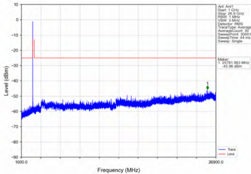
n41_30kHz_SISO_NTNV_10MHz_DFT-s-OFDM QPSK_2501.01MHz_Inner_1RB_Left
