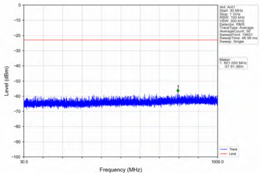
n41_15kHz_SISO_NTV_50MHz_DFT-s-OFDM QPSK_2593.005MHz_Edge_1RB_Left
