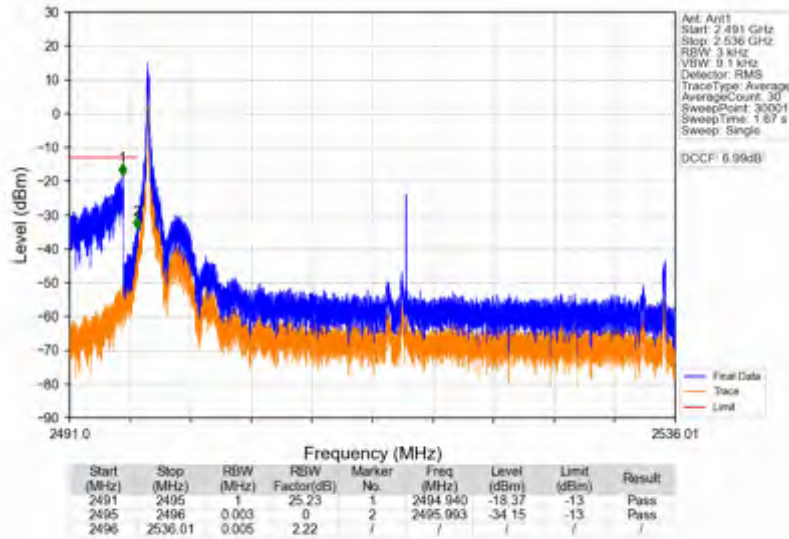
n41_15kHz_SISO_NTNV_40MHz_CP-OFDM QPSK_2516.01MHz_Inner_1RB_Left
