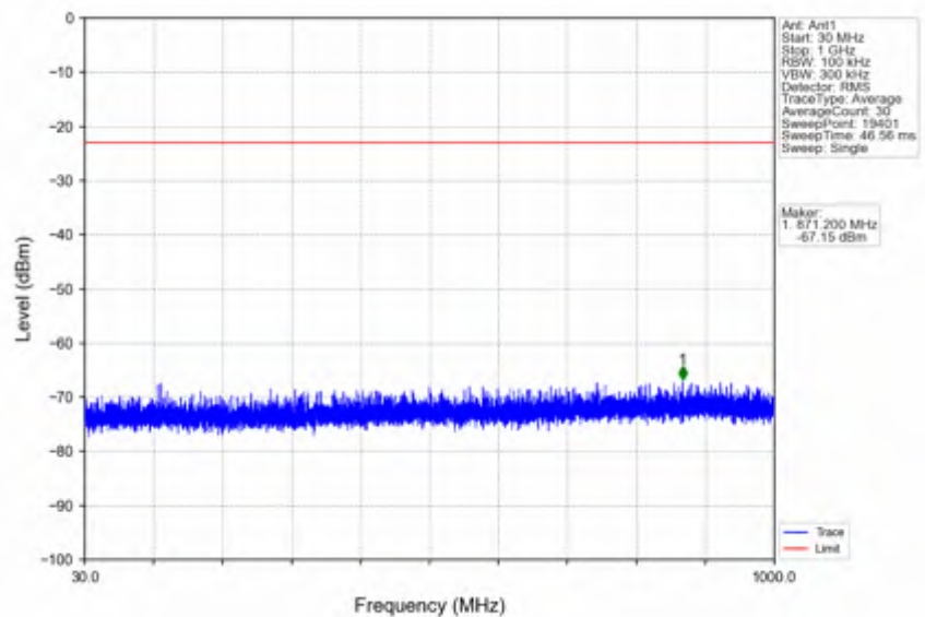
n41_15kHz_SISO_NTNV_40MHz_CP-OFDM QPSK_2670MHz_Inner_1RB_Right
