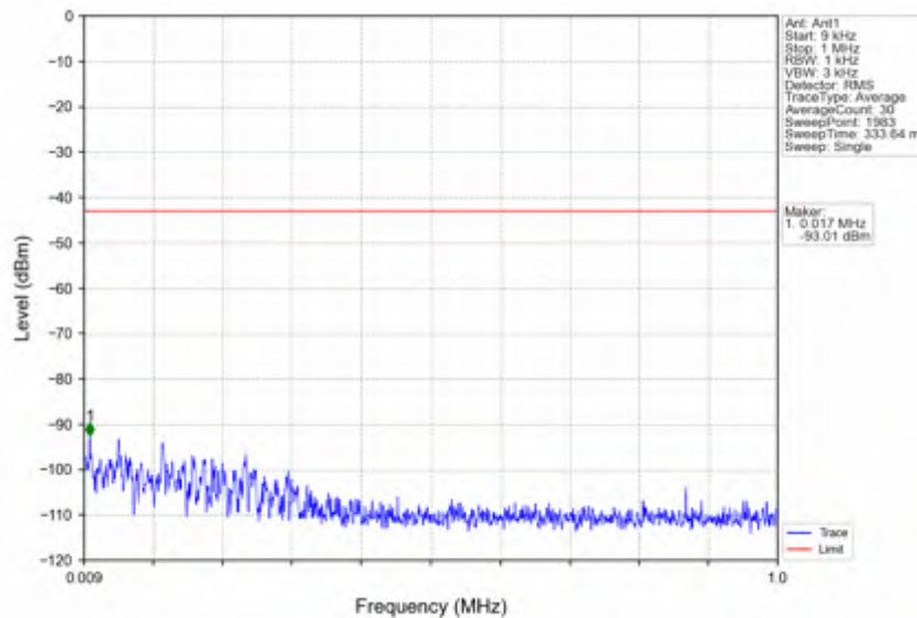
n41_30kHz_SISO_NTNV_10MHz_CP-OFDM QPSK_2501.01MHz_Inner_1RB_Left
