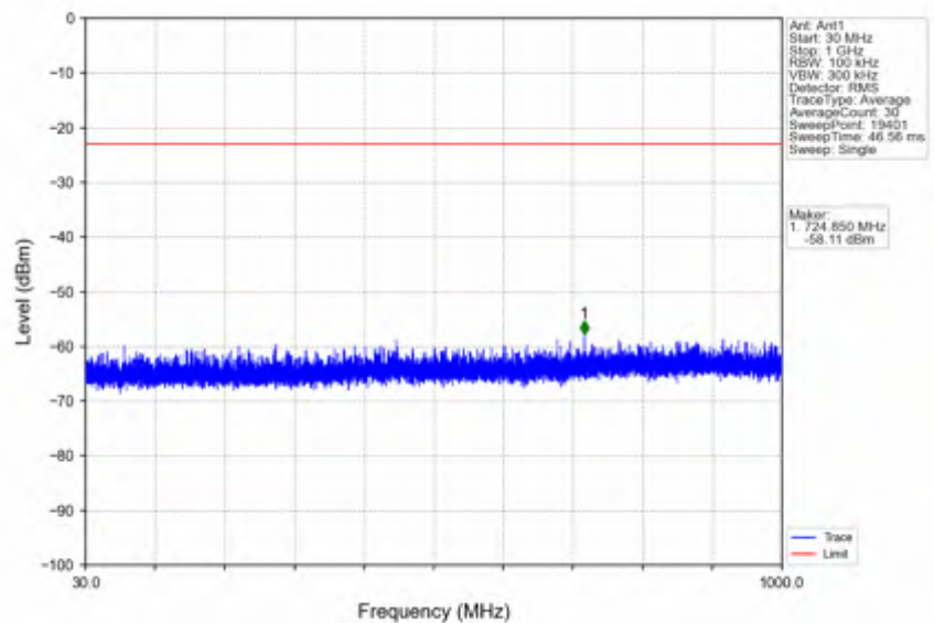
n41_15kHz_SISO_NTV_50MHz_CP-OFDM QPSK_2521.005MHz_Edge_1RB_Left
