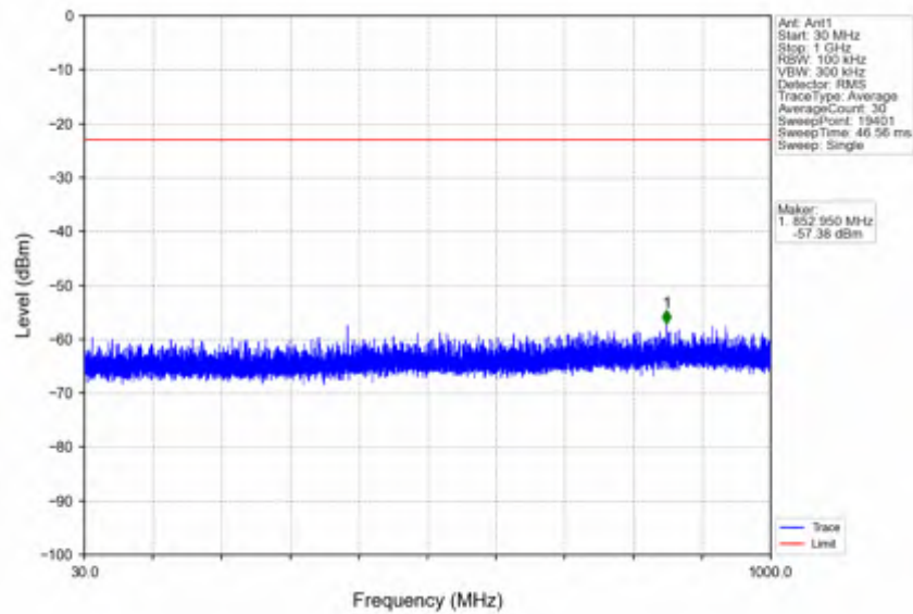
n41_15kHz_SISO_NTV_50MHz_CP-OFDM QPSK_2593.005MHz_Edge_1RB_Left
