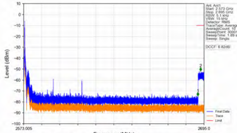
n41_15kHz_SISO_NTV_40MHz_DFT-s-OFDM_QPSK_2593.005MHz_Edge_1RB_Left
