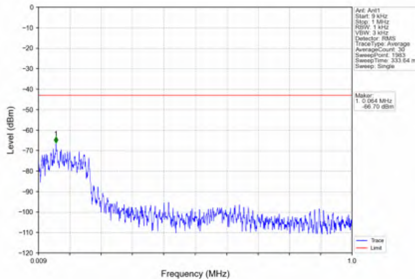
n41_15kHz_SISO_NTNV_50MHz_DFT-s-OFDM_QPSK_2593.005MHz_Edge_1RB_Left
