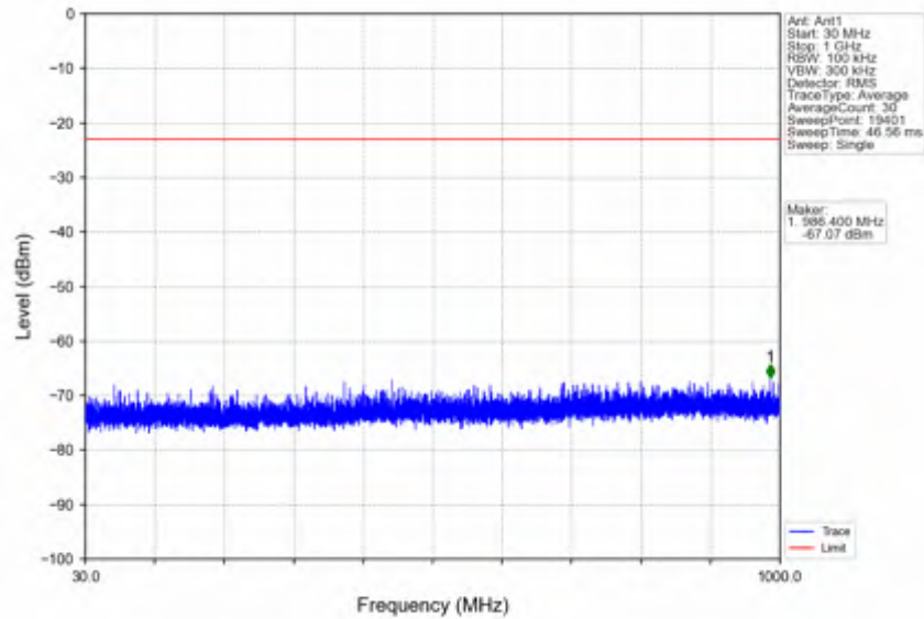
n41_30kHz_SISO_NTNV_10MHz_DFT-s-OFDM QPSK_2501.01MHz_Inner_1RB_Left
