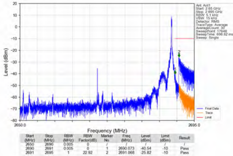
n41_15kHz_SISO_NTNV_40MHz_DFT-s-OFDM PI/2 BPSK_2670MHz_Inner_1RB_Right
