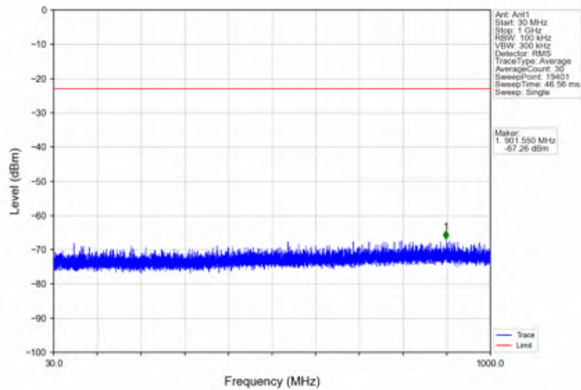
n41_15kHz_SISO_NTNV_40MHz_DFT-s-OFDM QPSK_2516.01MHz_Inner_1RB_Left
