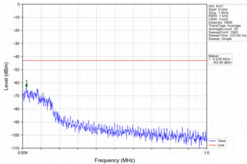
n41_15kHz_SISO_NTV_50MHz_CP-OFDM QPSK_2593.005MHz_Edge_1RB_Left
