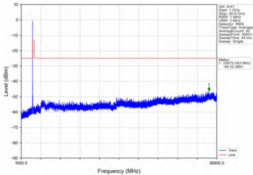
n41_30kHz_SISO_NTNV_15MHz_DFT-s-OFDM QPSK_2503.5MHz_Inner_1RB_Left
