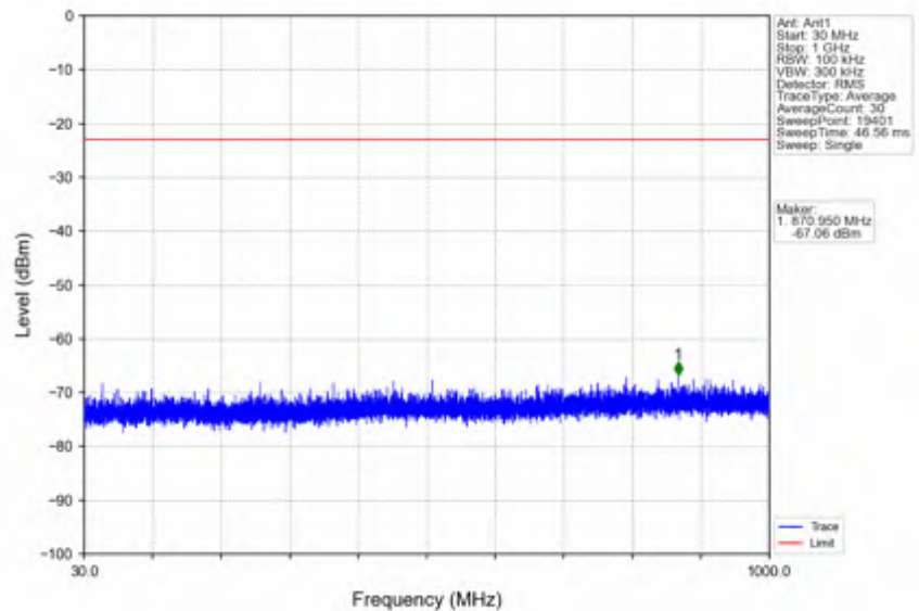
n41_15kHz_SISO_NTNV_40MHz_CP-OFDM QPSK_2516.01MHz_Inner_1RB_Left
