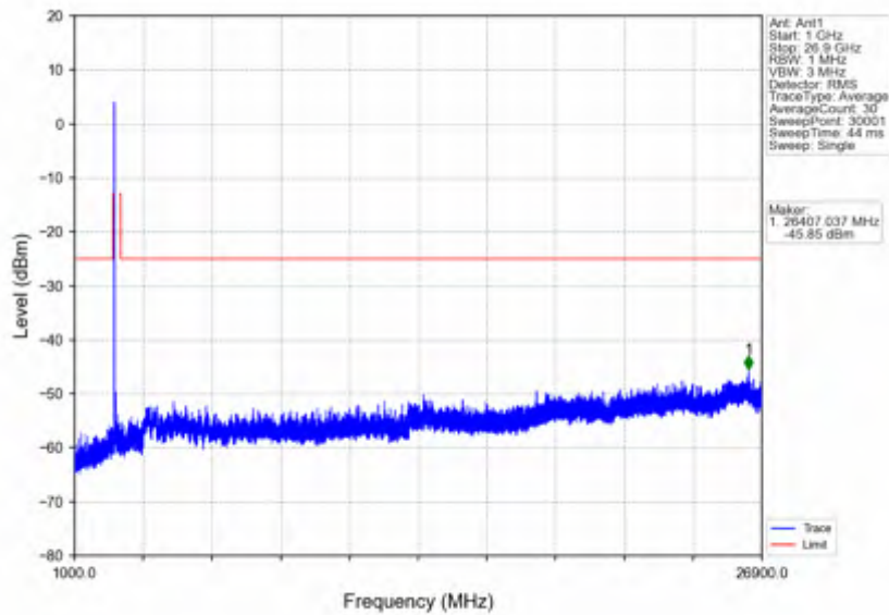
n41_15kHz_SISO_NTV_50MHz_CP-OFDM QPSK_2593.005MHz_Edge_1RB_Left
