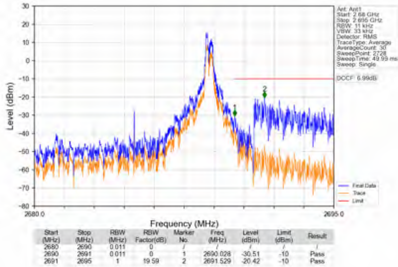
n41_30kHz_SISO_NTNV_10MHz_CP-OFDM QPSK_2685MHz_Inner_1RB_Right
