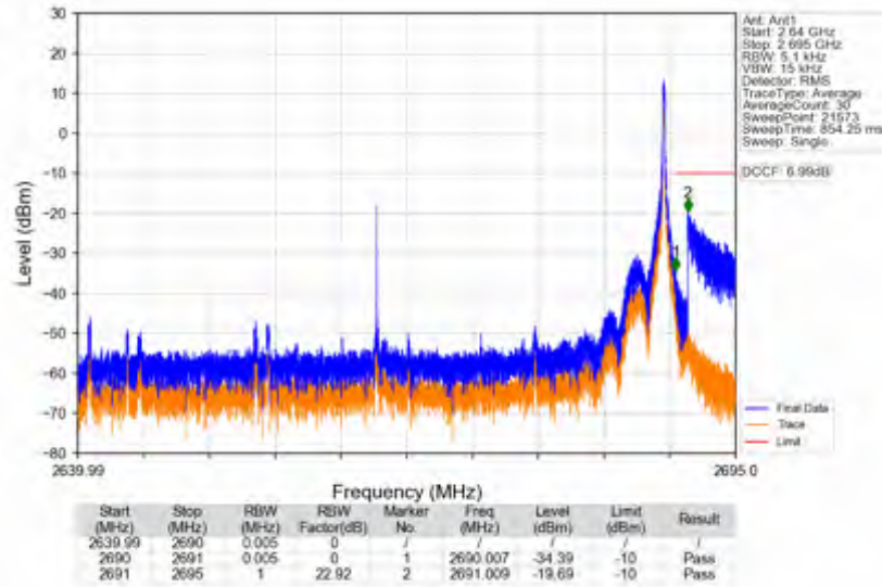
n41_15kHz_SISO_NTV_50MHz_CP-OFDM QPSK_2664.99MHz_Inner_1RB_Right
