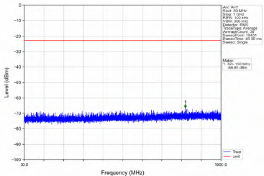
n41_30kHz_SISO_NTNV_10MHz_CP-OFDM QPSK_2685MHz_Inner_1RB_Right
