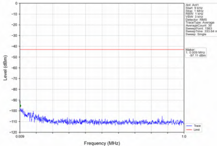
n41_15kHz_SISO_NTNV_40MHz_CP-OFDM QPSK_2670MHz_Inner_1RB_Right
