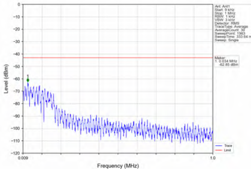
n41_15kHz_SISO_NTNV_40MHz_CP-OFDM QPSK_2516.01MHz_Edge_1RB_Left
