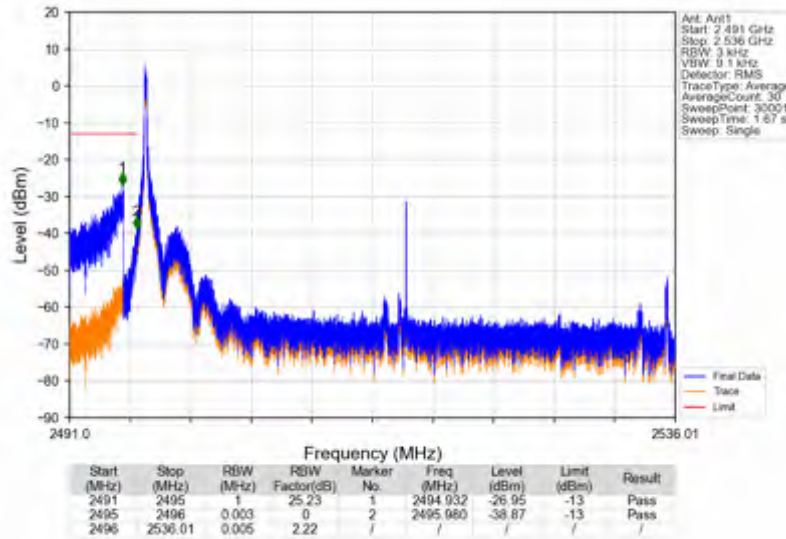
n41_15kHz_SISO_NTNV_40MHz_CP-OFDM QPSK_2516.01MHz_Edge_1RB_Left
