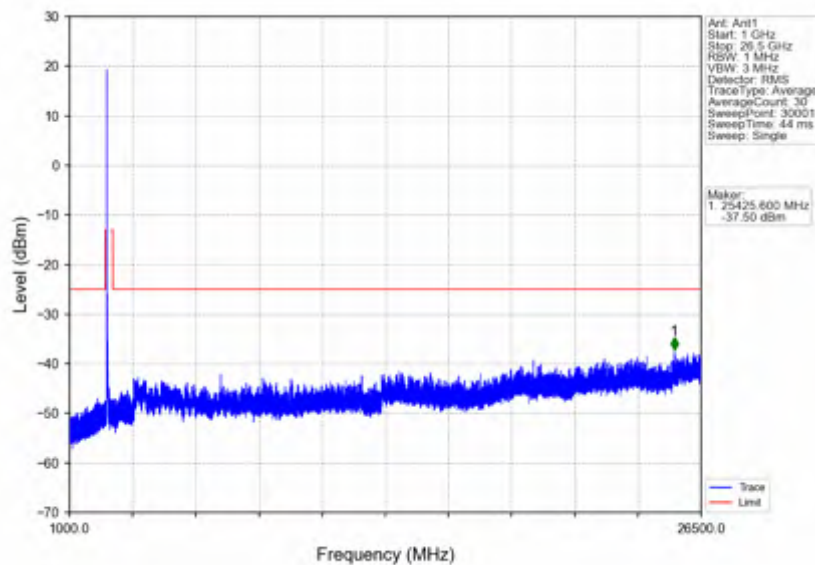
n41_15kHz_SISO_NTV_50MHz_DFT-s-OFDM QPSK_2521.005MHz_Edge_1RB_Left
