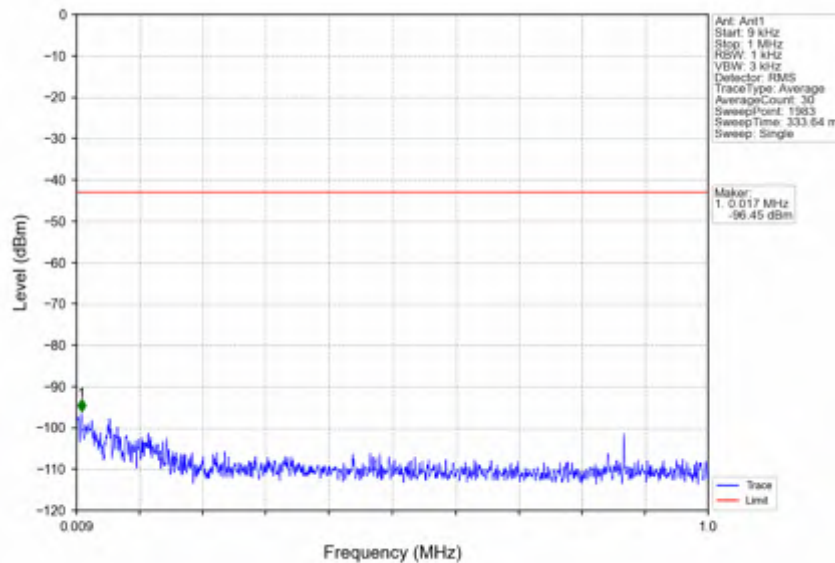
n41_15kHz_SISO_NTNV_50MHz_CP-OFDM QPSK_2521.005MHz_Inner_1RB_Left
