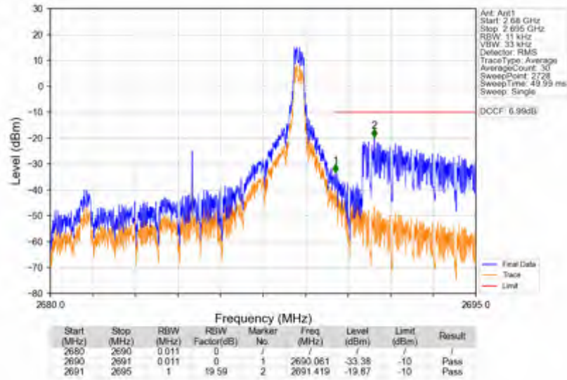
n41_30kHz_SISO_NTNV_10MHz_DFT-s-OFDM PI/2 BPSK_2685MHz_Inner_1RB_Right
