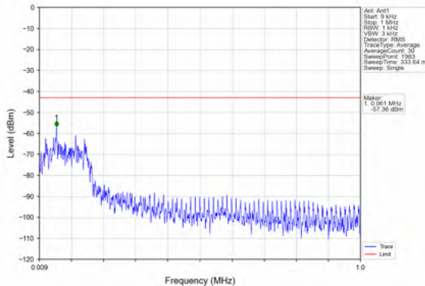
n41_15kHz_SISO_NTNV_50MHz_DFT-s-OFDM PI/2 BPSK_2521.005MHz_Inner_1RB_Left
