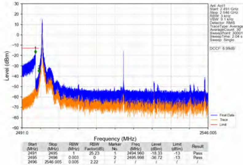
n41_15kHz_SISO_NTNV_50MHz_CP-OFDM QPSK_2521.005MHz_Inner_1RB_Left
