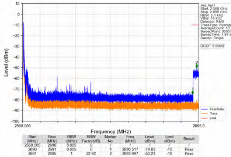
n41_15kHz_SISO_NTNV_50MHz_DFT-s-OFDM_QPSK_2593.005MHz_Edge_1RB_Left
