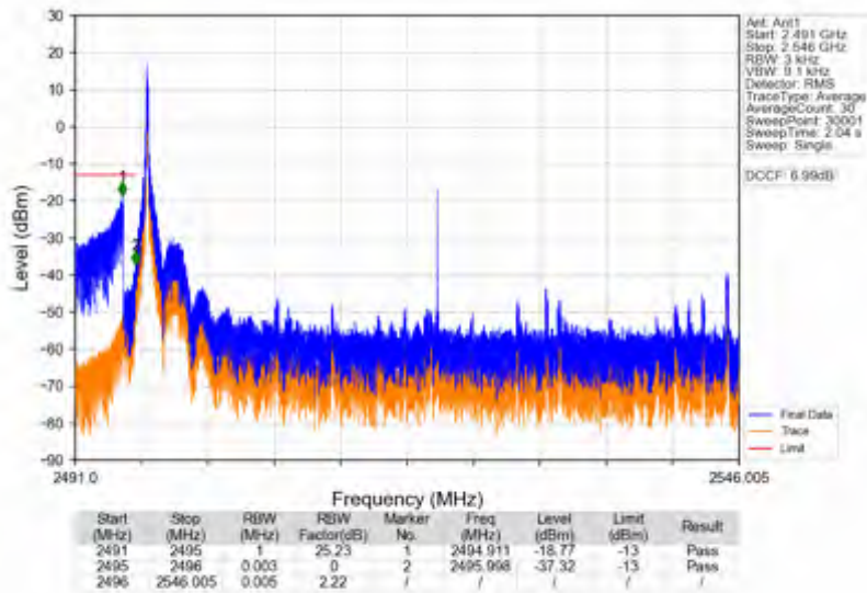
n41_15kHz_SISO_NTNV_50MHz_DFT-s-OFDM QPSK_2521.005MHz_Inner_1RB_Left
