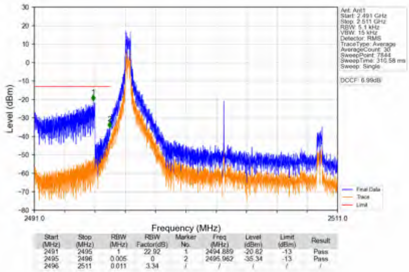
n41_30kHz_SISO_NTNV_15MHz_DFT-s-OFDM QPSK_2503.5MHz_Inner_1RB_Left
