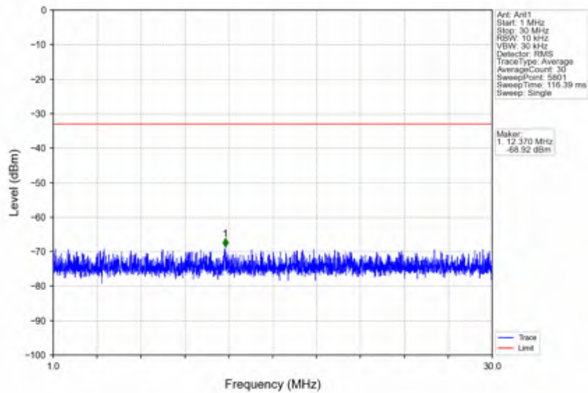
n41_15kHz_SISO_NTV_40MHz_DFT-s-OFDM_QPSK_2593.005MHz_Edge_1RB_Left
