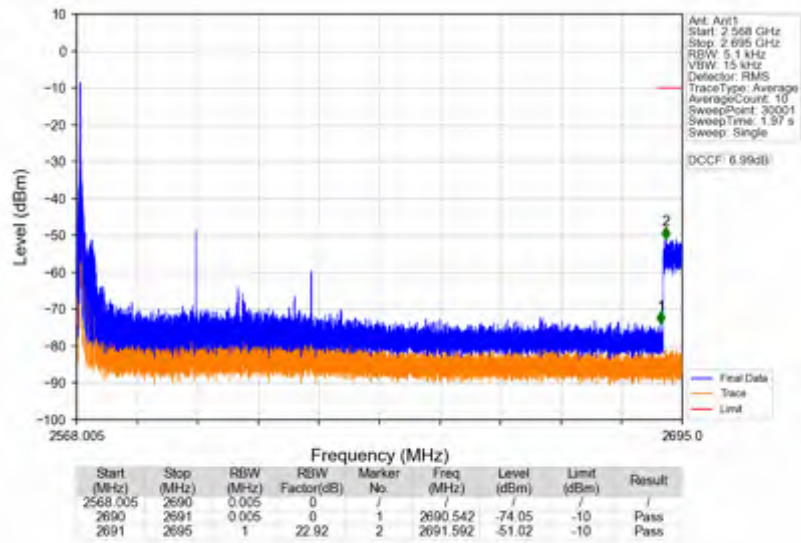
n41_15kHz_SISO_NTV_50MHz_CP-OFDM QPSK_2593.005MHz_Edge_1RB_Left
