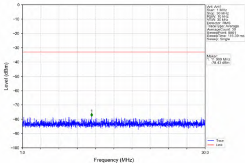
n41_30kHz_SISO_NTNV_10MHz_DFT-s-OFDM QPSK_2501.01MHz_Inner_1RB_Left
