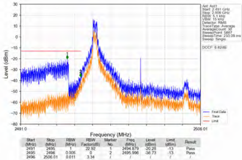
n41_30kHz_SISO_NTNV_10MHz_DFT-s-OFDM QPSK_2501.01MHz_Inner_1RB_Left
