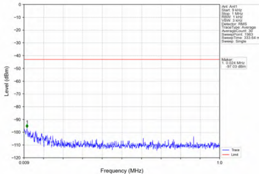
n41_15kHz_SISO_NTV_50MHz_CP-OFDM QPSK_2664.99MHz_Inner_1RB_Right
