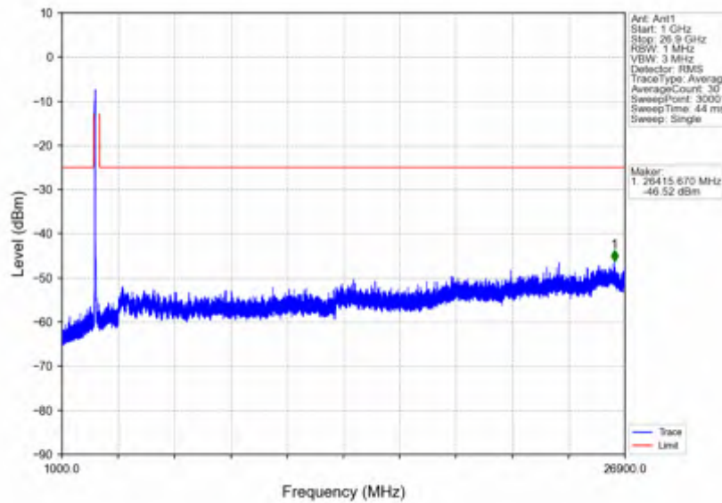
n41_15kHz_SISO_NTNV_40MHz_DFT-s-OFDM QPSK_2516.01MHz_Inner_1RB_Left
