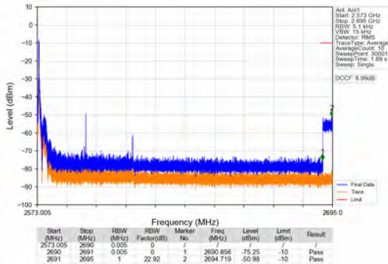
n41_15kHz_SISO_NTNV_40MHz_CP-OFDM QPSK_2593.005MHz_Edge_1RB_Left
