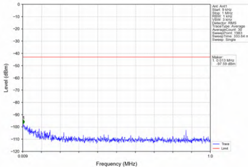
n41_15kHz_SISO_NTV_20MHz_CP-OFDM QPSK_2679.99MHz_Inner_1RB_Right
