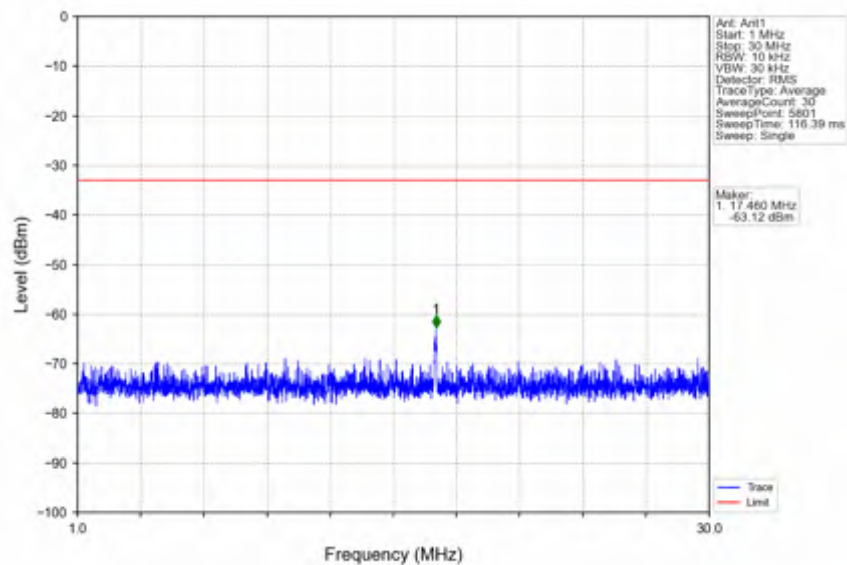
n41_15kHz_SISO_NTV_30MHz_CP-OFDM QPSK_2593.005MHz_Edge_1RB_Left
