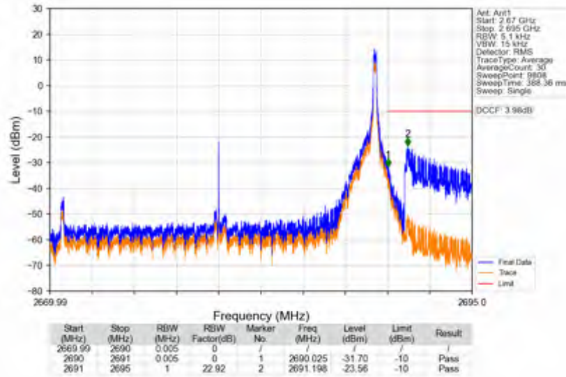
n41_15kHz_SISO_NTV_20MHz_CP-OFDM QPSK_2679.99MHz_Inner_1RB_Right
