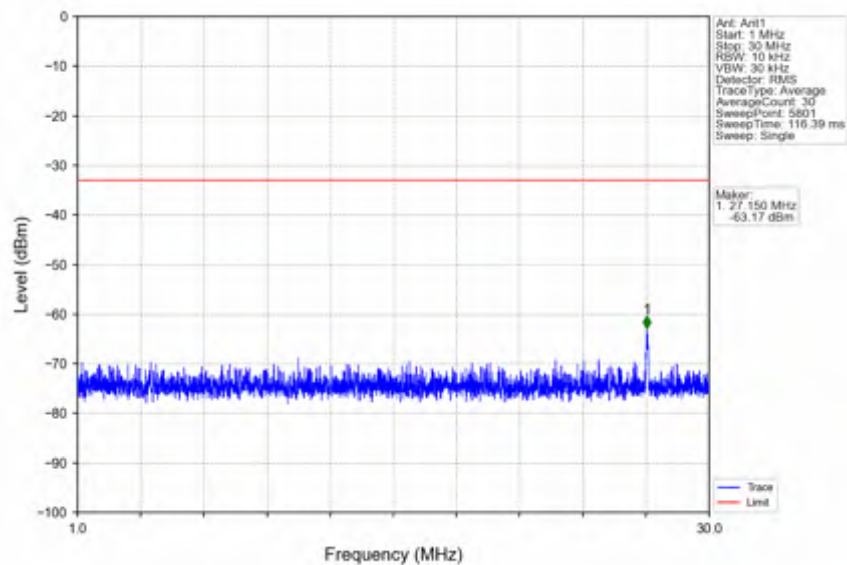
n41_15kHz_SISO_NTV_10MHz_CP-OFDM QPSK_2593.005MHz_Edge_1RB_Left
