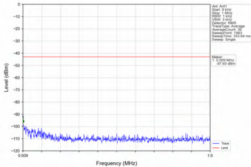
n41_15kHz_SISO_NTV_20MHz_DFT-s-OFDM QPSK_2679.99MHz_Inner_1RB_Right
