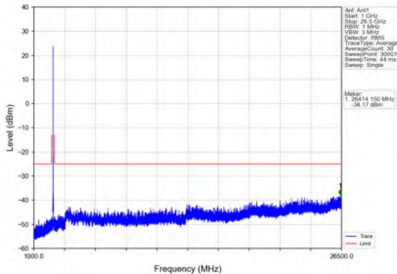
n41_15kHz_SISO_NTV_20MHz_CP-OFDM QPSK_2593.005MHz_Edge_1RB_Left
