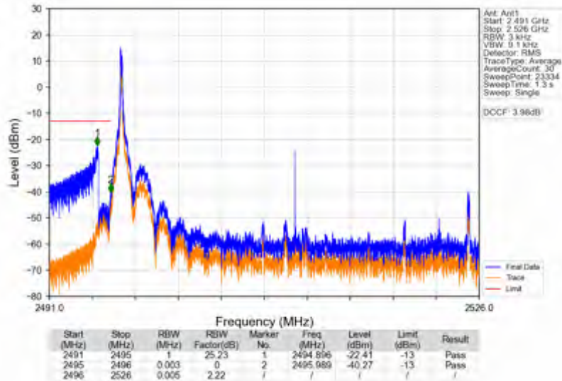
n41_15kHz_SISO_NTNV_30MHz_DFT-s-OFDM PI/2 BPSK_2511MHz_Inner_1RB_Left
