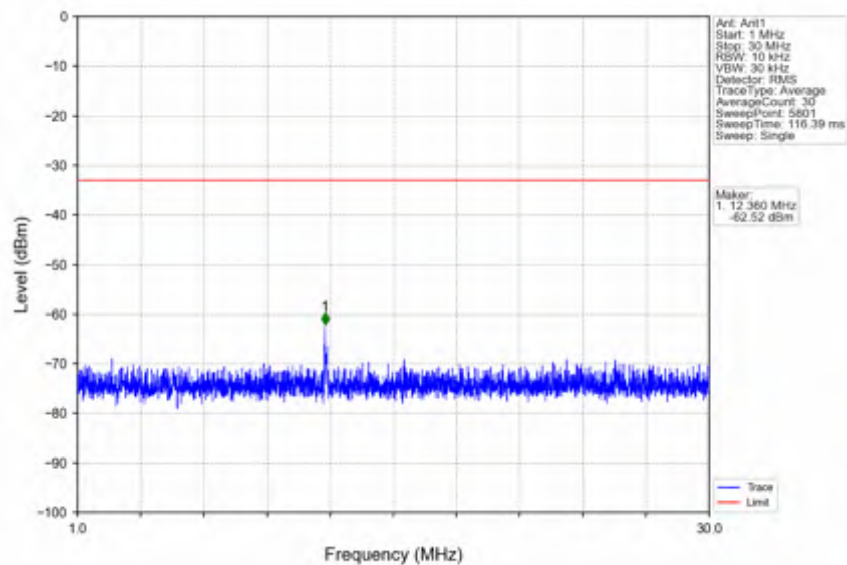
n41_15kHz_SISO_NTNV_40MHz_DFT-s-OFDM PI/2 BPSK_2593.005MHz_Edge_1RB_Left
