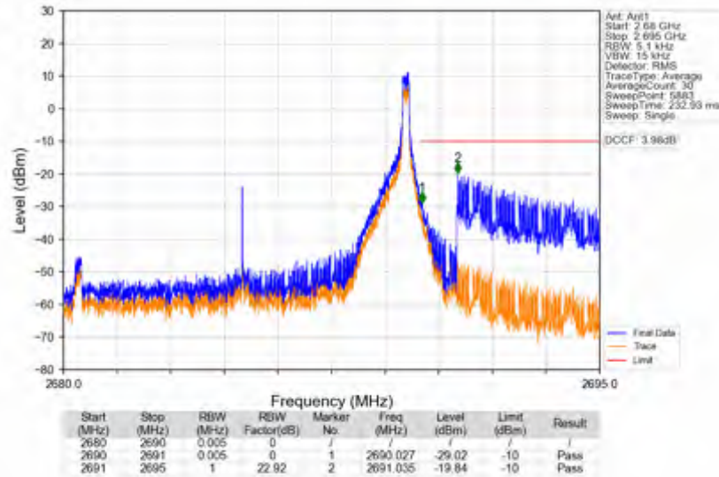
n41_15kHz_SISO_NTV_10MHz_CP-OFDM QPSK_2685MHz_Edge_1RB_Right
