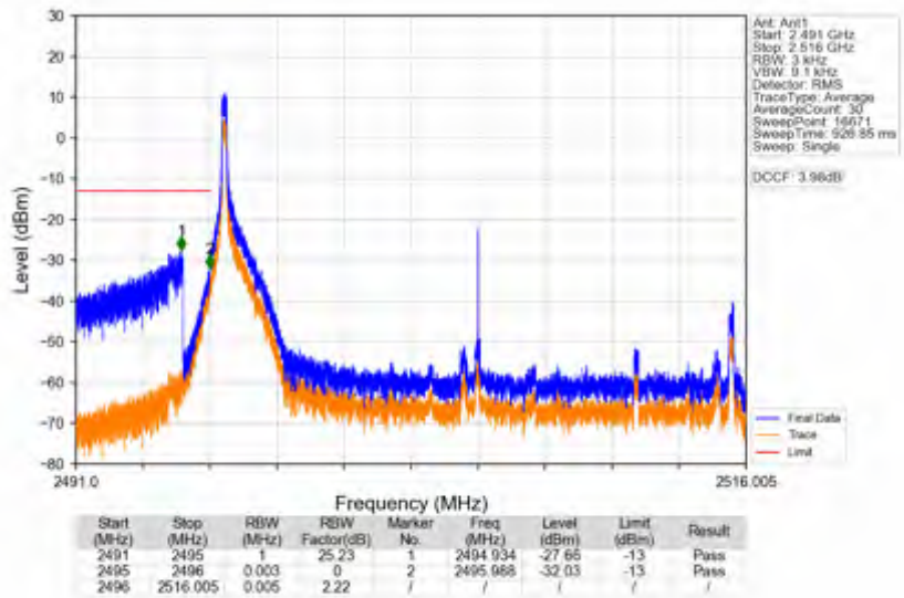
n41_15kHz_SISO_NTNV_20MHz_DFT-s-OFDM QPSK_2506.005MHz_Edge_1RB_Left
