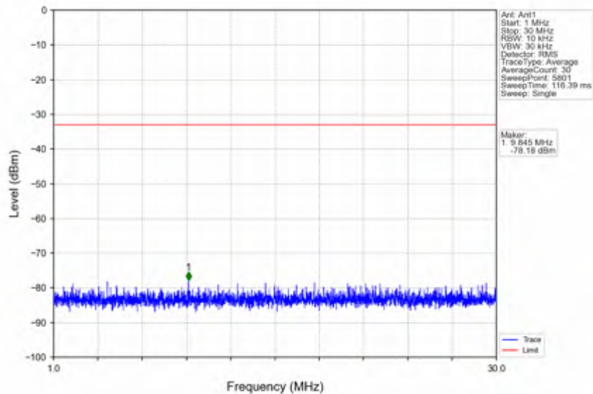
n41_15kHz_SISO_NTNV_15MHz_DFT-s-OFDM QPSK_2503.5MHz_Inner_1RB_Left
