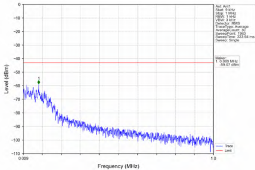
n41_15kHz_SISO_NTV_20MHz_CP-OFDM QPSK_2593.005MHz_Edge_1RB_Left
