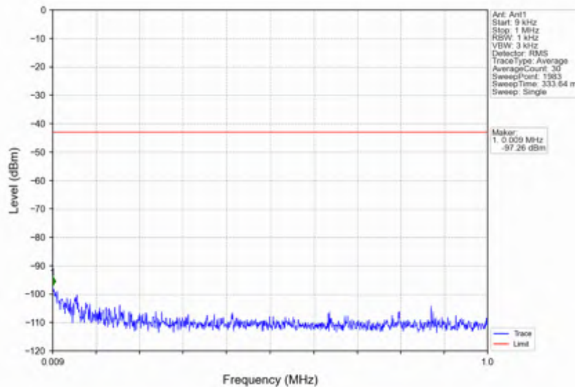
n41_15kHz_SISO_NTNV_30MHz_DFT-s-OFDM PI/2 BPSK_2511MHz_Inner_1RB_Left
