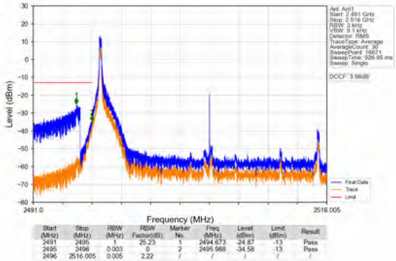
n41_15kHz_SISO_NTNV_20MHz_DFT-s-OFDM QPSK_2506.005MHz_Inner_1RB_Left
