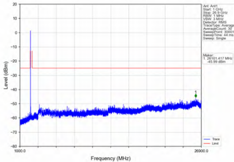
n41_15kHz_SISO_NTNV_40MHz_DFT-s-OFDM PI/2 BPSK_2593.005MHz_Edge_1RB_Left
