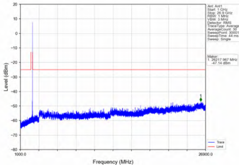
n41_15kHz_SISO_NTV_20MHz_DFT-s-OFDM QPSK_2679.99MHz_Inner_1RB_Right
