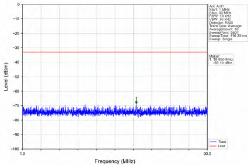
n41_15kHz_SISO_NTVV_15MHz_CP-OFDM QPSK_2503.5MHz_Edge_1RB_Left
