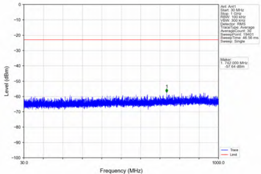
n41_15kHz_SISO_NTNV_10MHz_CP-OFDM QPSK_2501.01MHz_Edge_1RB_Left
