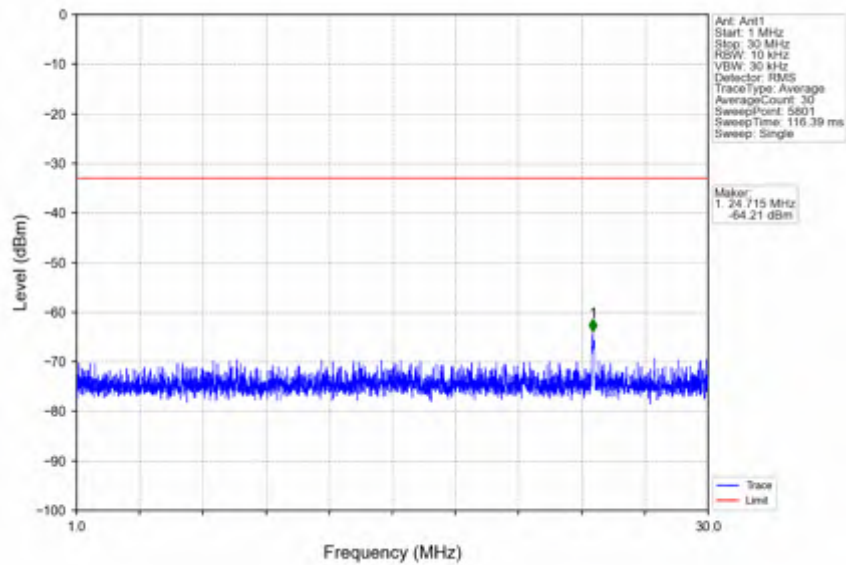
n41_15kHz_SISO_NTV_15MHz_DFT-s-OFDM QPSK_2593.005MHz_Edge_1RB_Left
