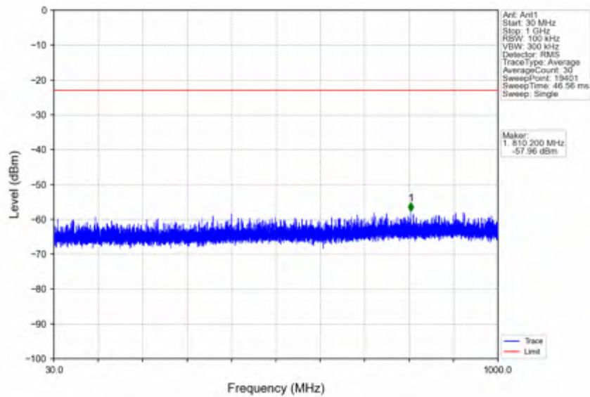
n41_15kHz_SISO_NTV_10MHz_CP-OFDM QPSK_2593.005MHz_Edge_1RB_Left
