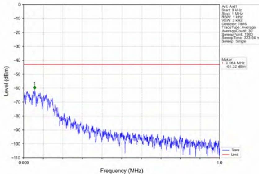
n41_15kHz_SISO_NTV_20MHz_CP-OFDM QPSK_2679.99MHz_Edge_1RB_Right
