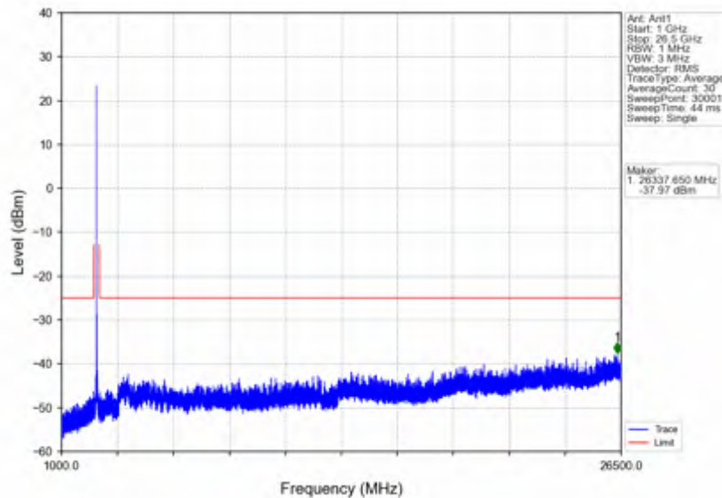
n41_15kHz_SISO_NTV_30MHz_CP-OFDM QPSK_2593.005MHz_Edge_1RB_Left
