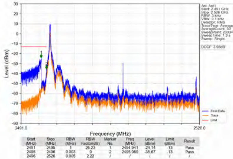
n41_15kHz_SISO_NTNV_30MHz_DFT-s-OFDM_PI/2_BPSK_2511MHz_Edge_1RB_Left
