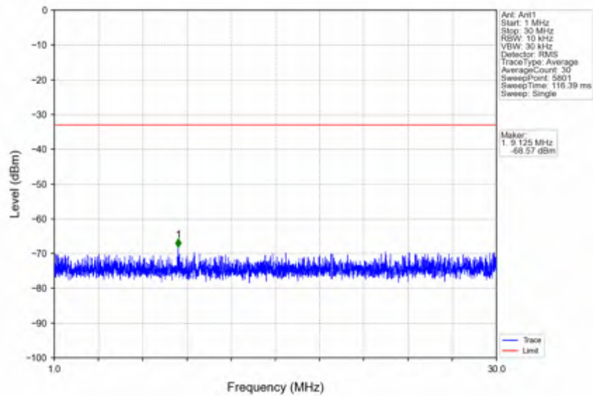
n41_15kHz_SISO_NTV_30MHz_DFT-s-OFDM PI/2 BPSK_2511MHz_Edge_1RB_Left
