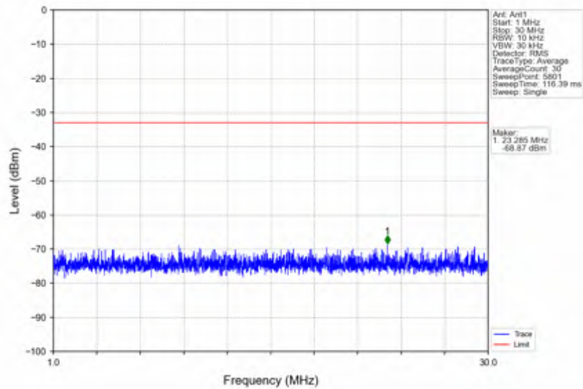
n41_15kHz_SISO_NTNV_20MHz_CP-OFDM QPSK_2506.005MHz_Edge_1RB_Left
