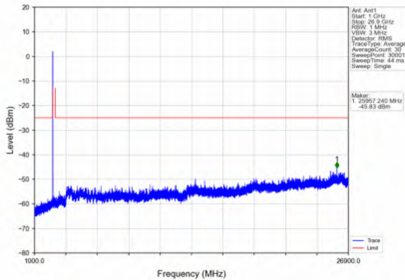
n41_15kHz_SISO_NTV_15MHz_CP-OFDM QPSK_2593.005MHz_Edge_1RB_Left
