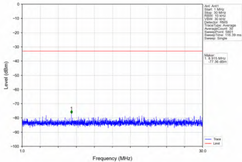
n41_15kHz_SISO_NTNV_10MHz_CP-OFDM QPSK_2501.01MHz_Inner_1RB_Left
