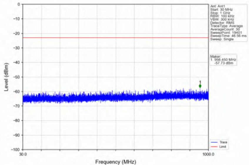
n41_15kHz_SISO_NTNV_30MHz_CP-OFDM QPSK_2511MHz_Edge_1RB_Left
