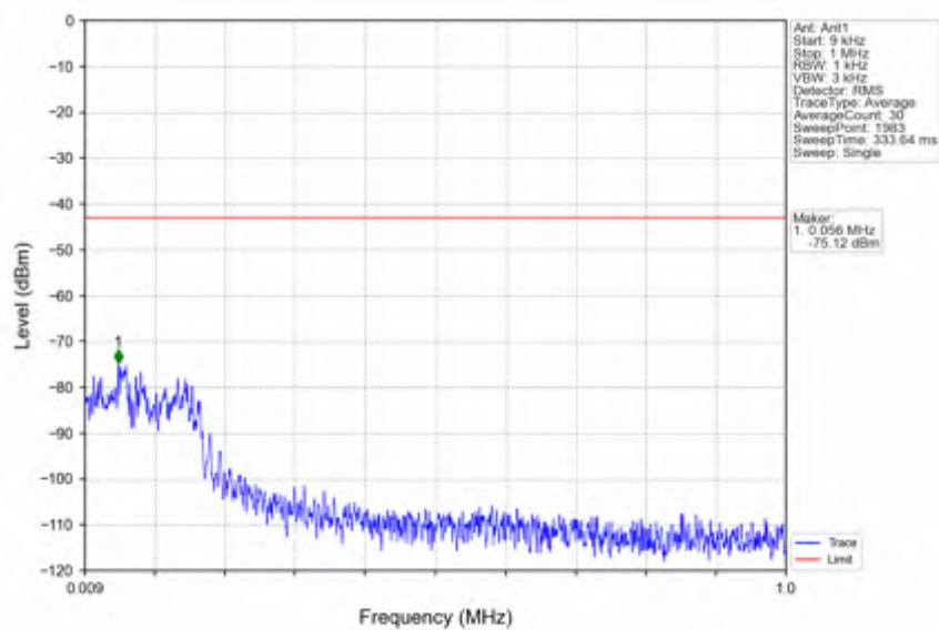
n38_15kHz_SISO_NTNV_20MHz_DFT-s-OFDM PI/2 BPSK_2580MHz_Edge_1RB_Left
