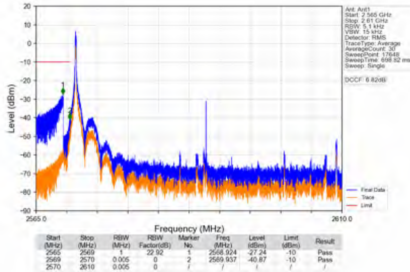
n38_15kHz_SISO_NTNV_40MHz_DFT-s-OFDM PI/2 BPSK_2590MHz_Inner_1RB_Left
