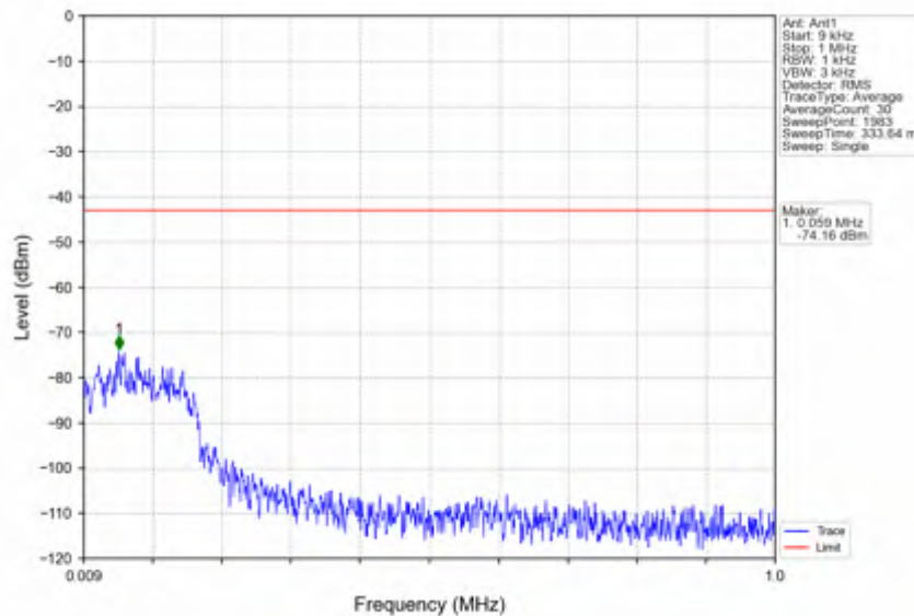
n38_15kHz_SISO_NTNV_20MHz_DFT-s-OFDM QPSK_2580MHz_Edge_1RB_Left
