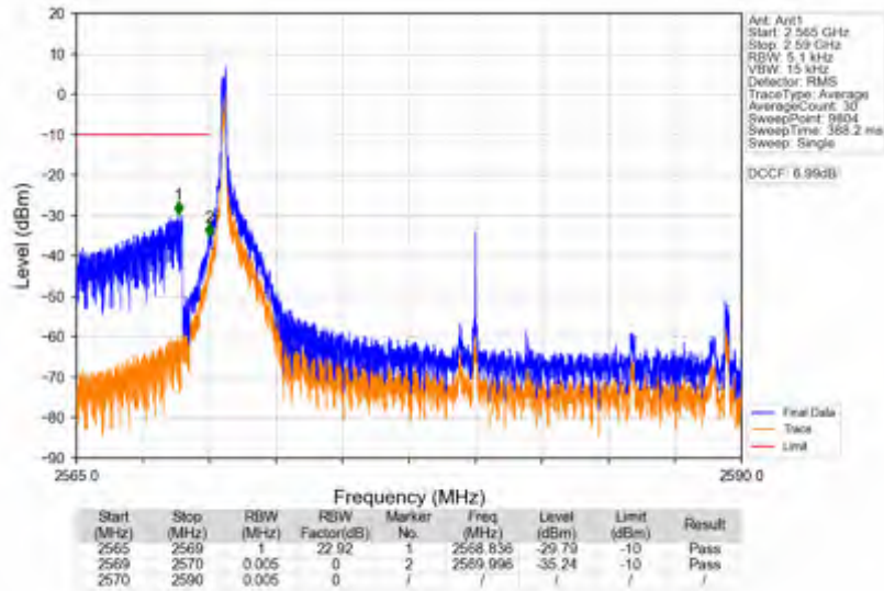
n38_15kHz_SISO_NTNV_20MHz_DFT-s-OFDM QPSK_2580MHz_Edge_1RB_Left
