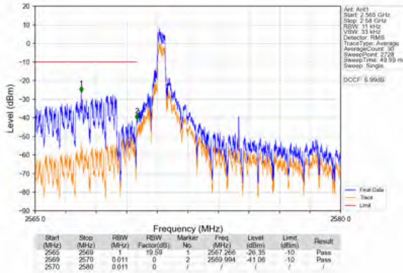
n38_30kHz_SISO_NTNV_10MHz_DFT-s-OFDM PI/2 BPSK_2575MHz_Inner_1RB_Left
