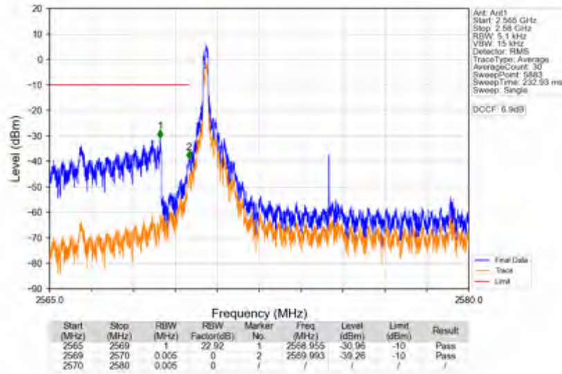
n38_15kHz_SISO_NTNV_10MHz_CP-OFDM QPSK_2575MHz_Inner_1RB_Left
