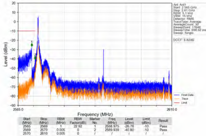
n38_15kHz_SISO_NTNV_40MHz_CP-OFDM QPSK_2590MHz_Inner_1RB_Left
