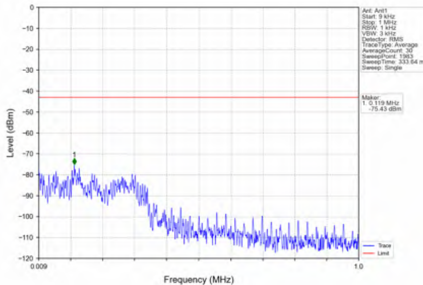
n38_30kHz_SISO_NTNV_10MHz_DFT-s-OFDM PI/2 BPSK_2595MHz_Edge_1RB_Left
