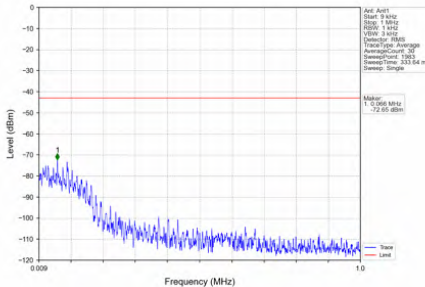
n38_15kHz_SISO_NTNV_10MHz_CP-OFDM QPSK_2595MHz_Edge_1RB_Left
