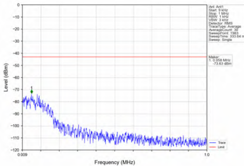
n38_15kHz_SISO_NTNV_20MHz_CP-OFDM QPSK_2595MHz_Edge_1RB_Left
