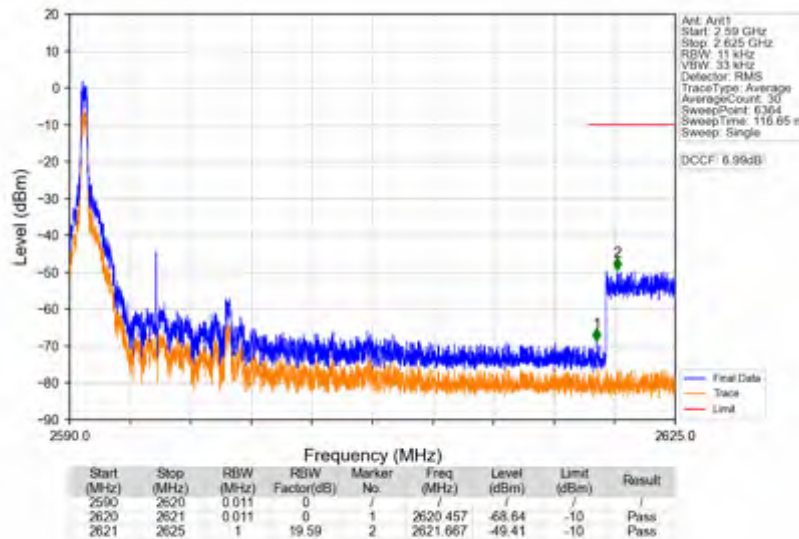
n38_30kHz_SISO_NTNV_10MHz_DFT-s-OFDM QPSK_2595MHz_Edge_1RB_Left
