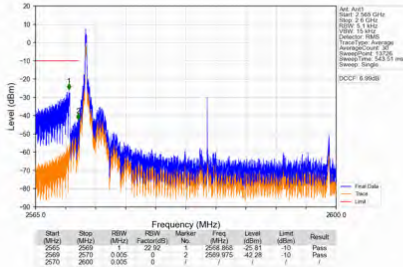
n38_15kHz_SISO_NTNV_30MHz_DFT-s-OFDM PI/2 BPSK_2585MHz_Inner_1RB_Left
