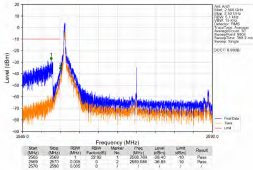
n38_15kHz_SISO_NTNV_20MHz_CP-OFDM QPSK_2580MHz_Edge_1RB_Left
