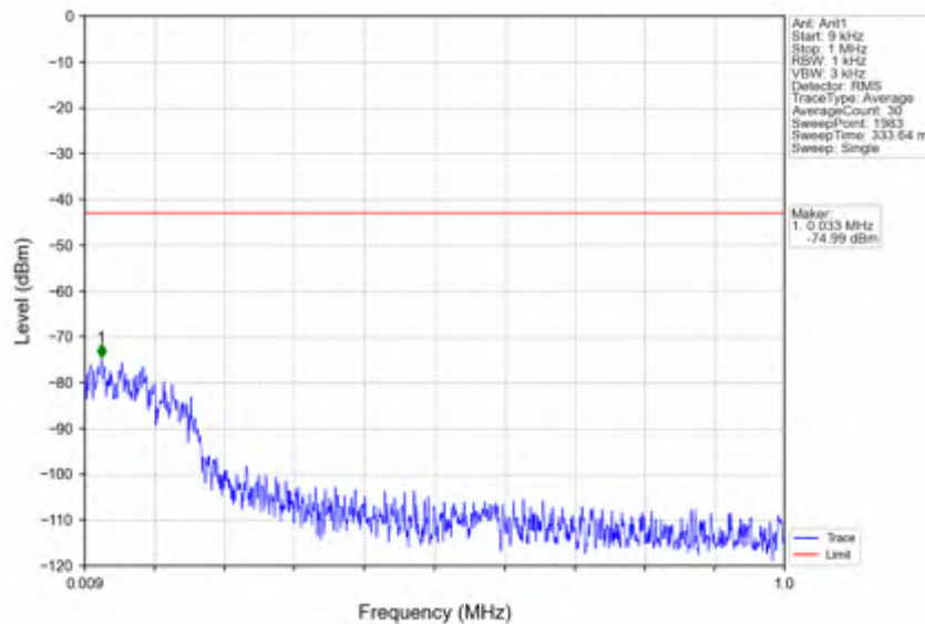
n38_15kHz_SISO_NTNV_40MHz_CP-OFDM QPSK_2595MHz_Edge_1RB_Left
