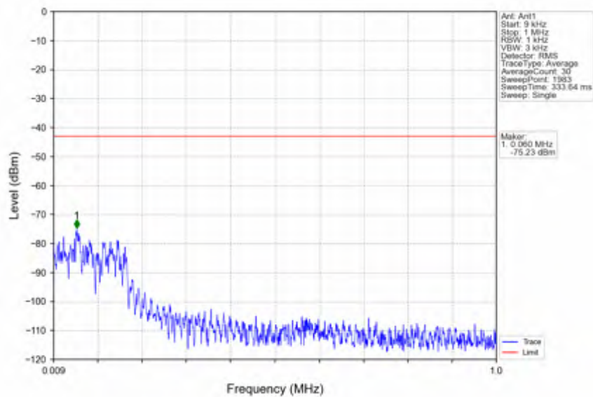
n38_15kHz_SISO_NTNV_40MHz_DFT-s-OFDM_PI/2_BPSK_2590MHz_Edge_1RB_Left
