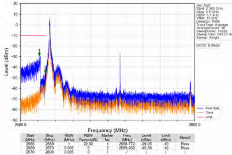
n38_15kHz_SISO_NTNV_30MHz_CP-OFDM QPSK_2585MHz_Inner_1RB_Left
