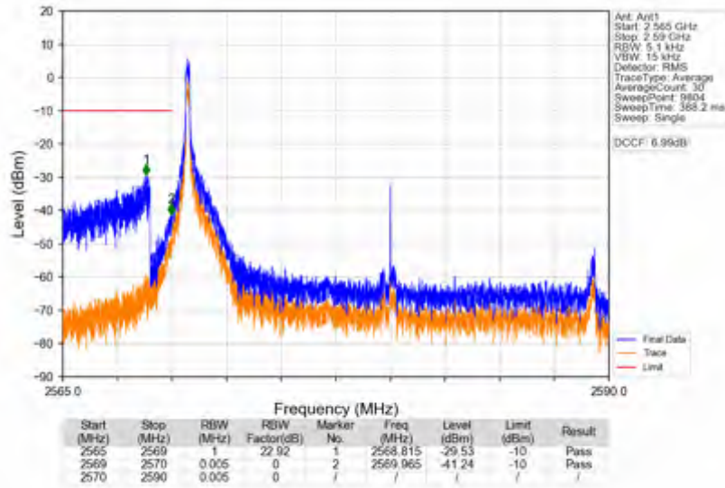
n38_15kHz_SISO_NTNV_20MHz_CP-OFDM QPSK_2580MHz_Inner_1RB_Left
