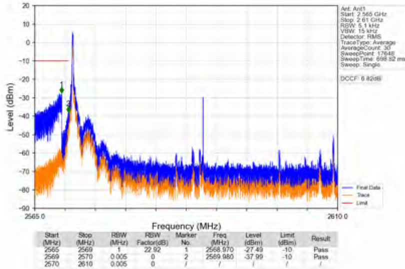
n38_15kHz_SISO_NTNV_40MHz_DFT-s-OFDM_PI/2_BPSK_2590MHz_Edge_1RB_Left
