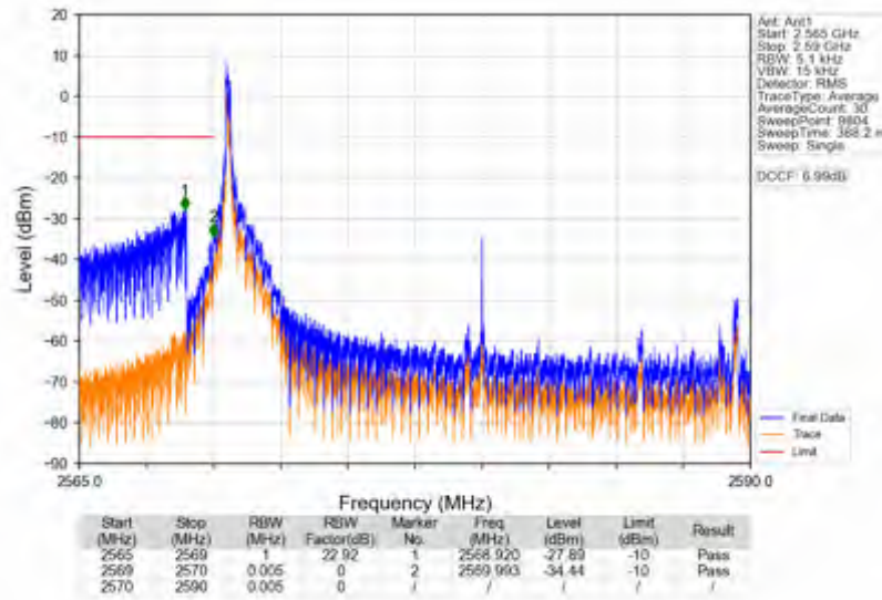
n38_15kHz_SISO_NTNV_20MHz_DFT-s-OFDM PI/2 BPSK_2580MHz_Edge_1RB_Left
