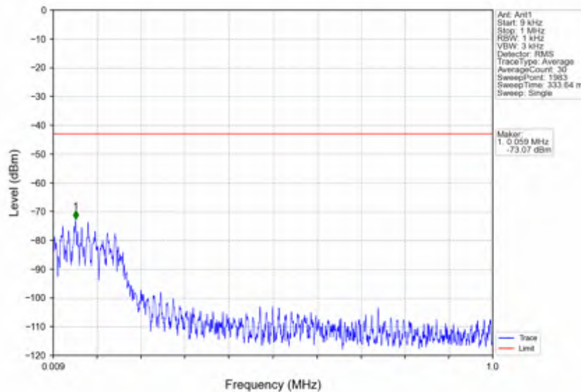
n38_15kHz_SISO_NTNV_40MHz_DFT-s-OFDM QPSK_2590MHz_Edge_1RB_Left
