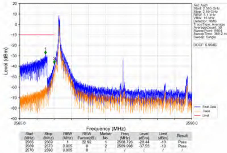
n38_15kHz_SISO_NTNV_20MHz_DFT-s-OFDM QPSK_2580MHz_Inner_1RB_Left
