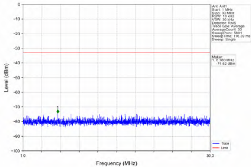
n38_15kHz_SISO_NTNV_40MHz_CP-OFDM QPSK_2590MHz_Edge_1RB_Left
