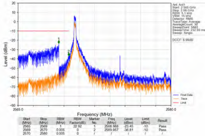
n38_15kHz_SISO_NTNV_10MHz_DFT-s-OFDM QPSK_2575MHz_Inner_1RB_Left
