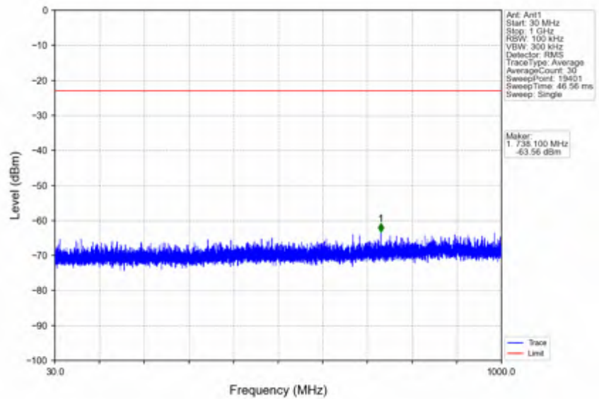
n38_15kHz_SISO_NTNV_20MHz_CP-OFDM QPSK_2580MHz_Edge_1RB_Left
