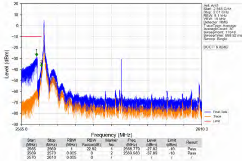
n38_15kHz_SISO_NTNV_40MHz_DFT-s-OFDM QPSK_2590MHz_Edge_1RB_Left
