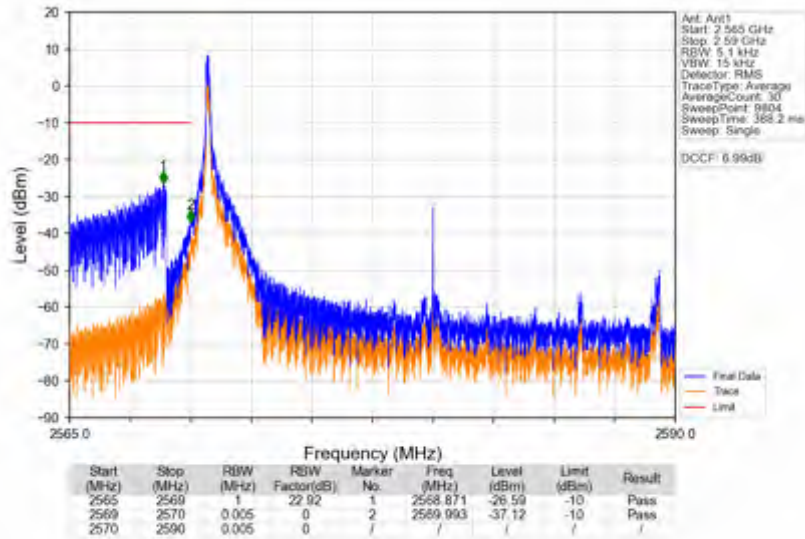
n38_15kHz_SISO_NTNV_20MHz_DFT-s-OFDM PI/2 BPSK_2580MHz_Inner_1RB_Left
