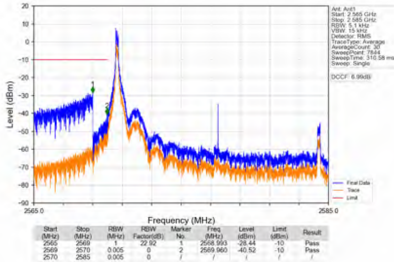
n38_15kHz_SISO_NTNV_15MHz_DFT-s-OFDM PI/2 BPSK_2577.5MHz_Inner_1RB_Left
