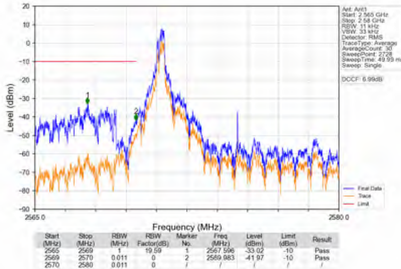
n38_30kHz_SISO_NTNV_10MHz_DFT-s-OFDM QPSK_2575MHz_Inner_1RB_Left
