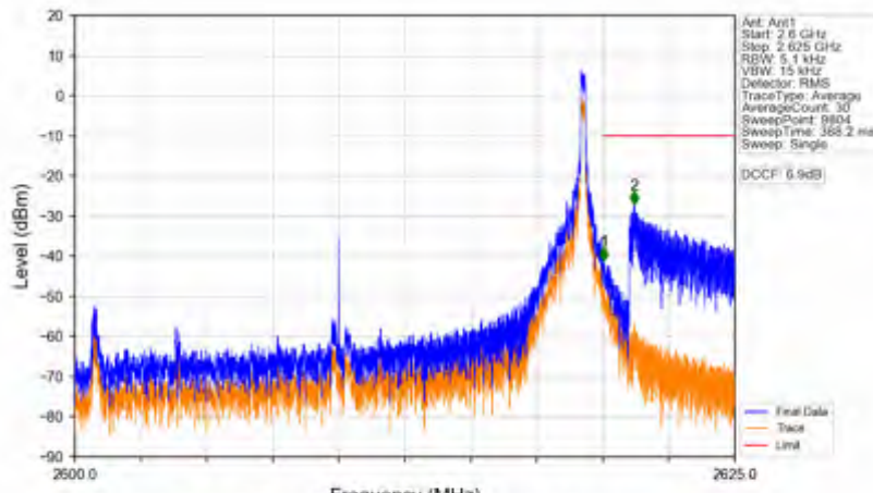
n38_15kHz_SISO_NTNV_20MHz_DFT-s-OFDM PI/2 BPSK_2610MHz_Inner_1RB_Right
