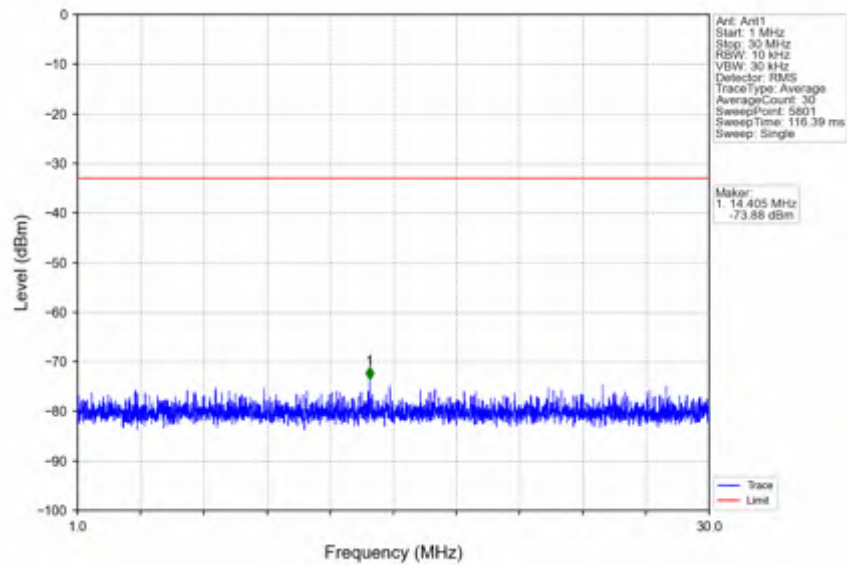
n38_15kHz_SISO_NTNV_40MHz_CP-OFDM QPSK_2595MHz_Edge_1RB_Left
