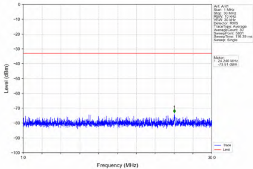
n38_15kHz_SISO_NTNV_20MHz_DFT-s-OFDM QPSK_2595MHz_Edge_1RB_Left
