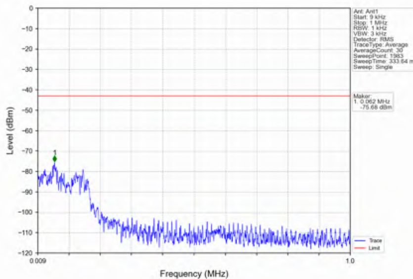
n38_15kHz_SISO_NTNV_40MHz_DFT-s-OFDM PI/2 BPSK_2595MHz_Edge_1RB_Left
