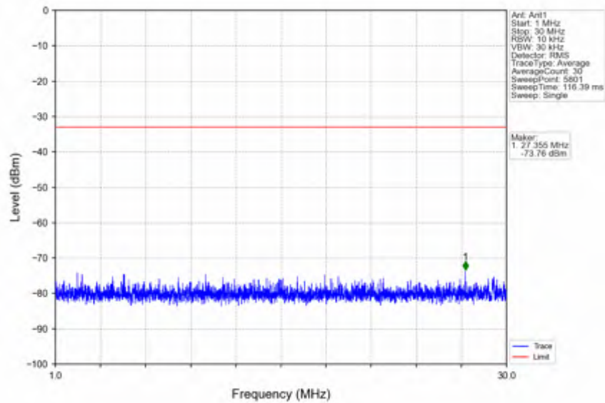
n38_15kHz_SISO_NTNV_10MHz_CP-OFDM QPSK_2595MHz_Edge_1RB_Left
