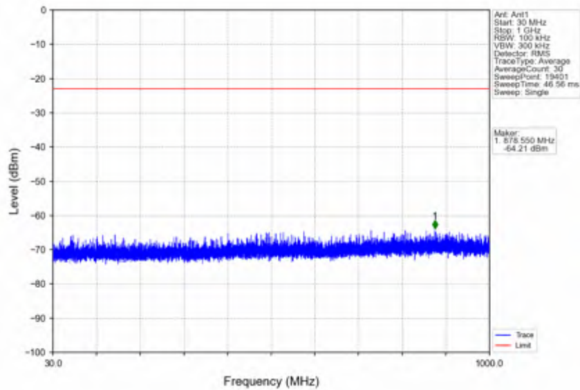
n25_30kHz_SISO_NTNV_30MHz_DFT-s-OFDM QPSK_1865MHz_Inner_1RB_Left
