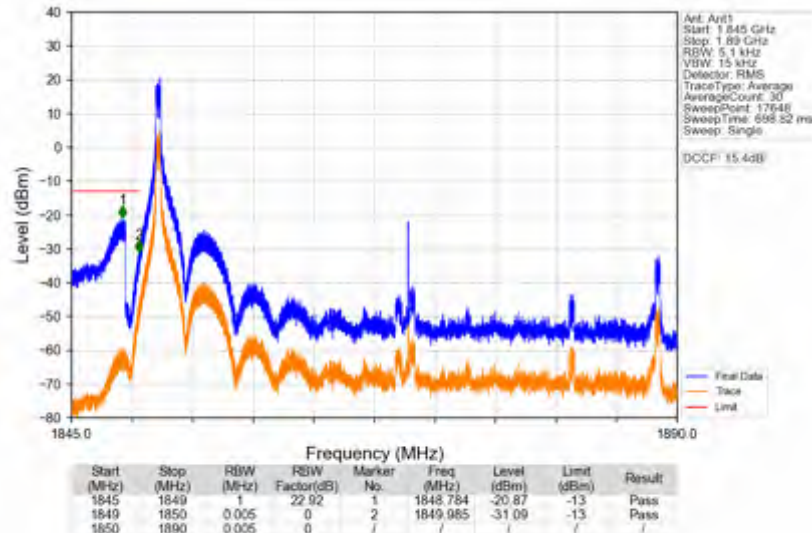
n25_30kHz_SISO_NTNV_40MHz_DFT-s-OFDM PI/2 BPSK_1870MHz_Inner_1RB_Left
