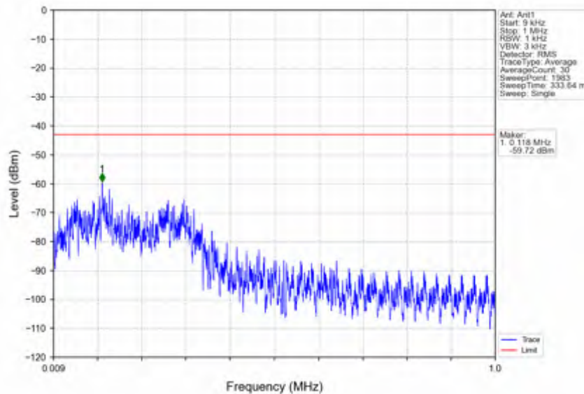
n25_30kHz_SISO_NTNV_40MHz_DFT-s-OFDM PI/2 BPSK_1870MHz_Inner_1RB_Left
