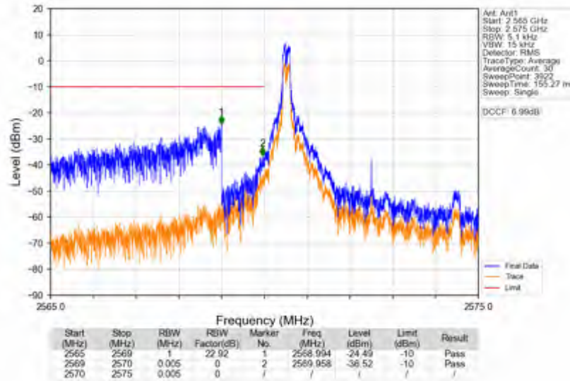
n38_15kHz_SISO_NTNV_5MHz_DFT-s-OFDM PI/2 BPSK_2572.5MHz_Inner_1RB_Left
