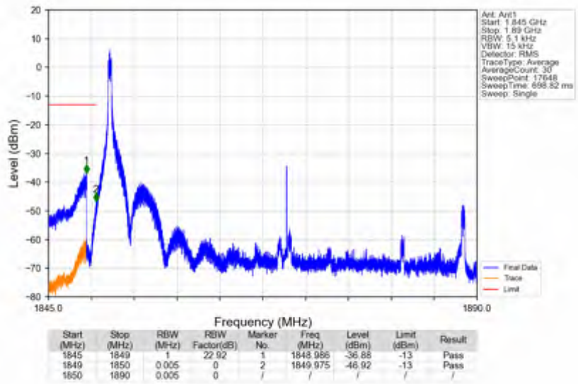
n25_30kHz_SISO_NTNV_40MHz_DFT-s-OFDM QPSK_1870MHz_Inner_1RB_Left
