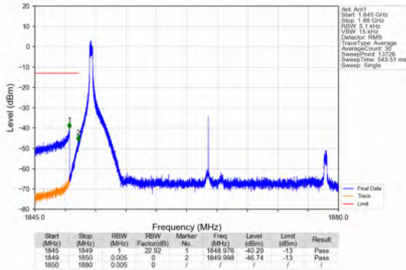
n25_30kHz_SISO_NTNV_30MHz_CP-OFDM QPSK_1865MHz_Inner_1RB_Left
