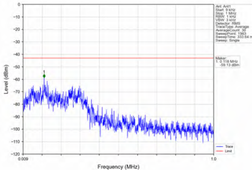
n25_30kHz_SISO_NTNV_30MHz_DFT-s-OFDM PI/2 BPSK_1865MHz_Inner_1RB_Left
