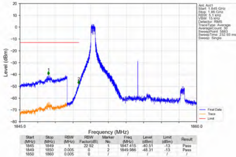
n25_30kHz_SISO_NTNV_10MHz_CP-OFDM QPSK_1855MHz_Inner_1RB_Left
