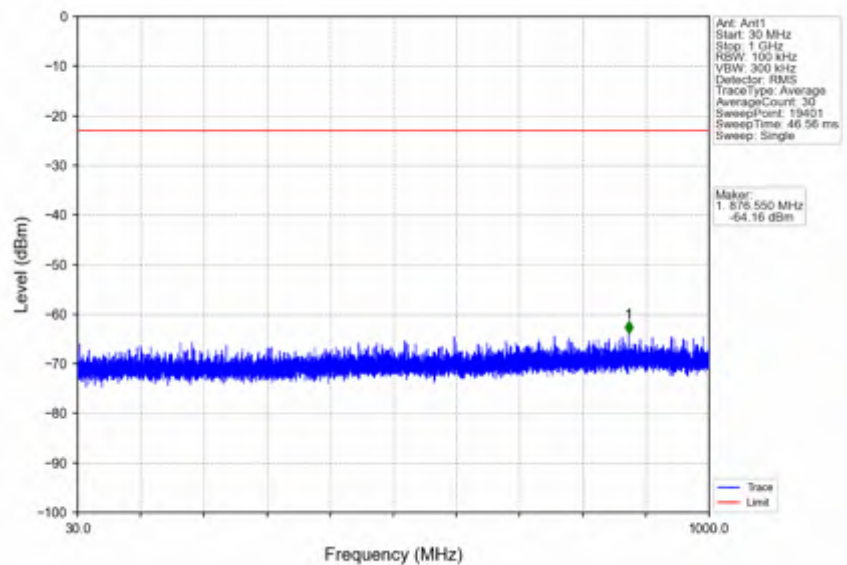
n25_30kHz_SISO_NTNV_10MHz_CP-OFDM QPSK_1855MHz_Inner_1RB_Left
