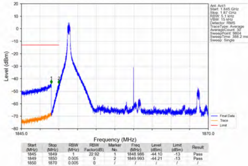
n25_30kHz_SISO_NTNV_20MHz_DFT-s-OFDM QPSK_1860MHz_Inner_1RB_Left
