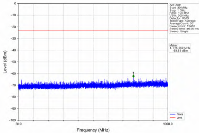
n25_30kHz_SISO_NTNV_20MHz_DFT-s-OFDM QPSK_1860MHz_Inner_1RB_Left
