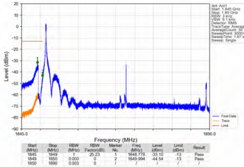
n25_15kHz_SISO_NTNV_40MHz_CP-OFDM QPSK_1870MHz_Inner_1RB_Left
