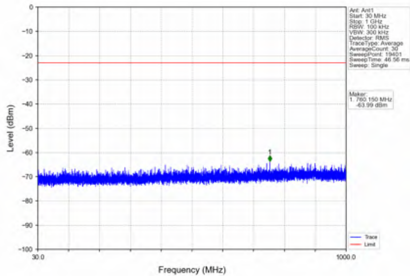
n25_15kHz_SISO_NTNV_40MHz_DFT-s-OFDM QPSK_1870MHz_Inner_1RB_Left
