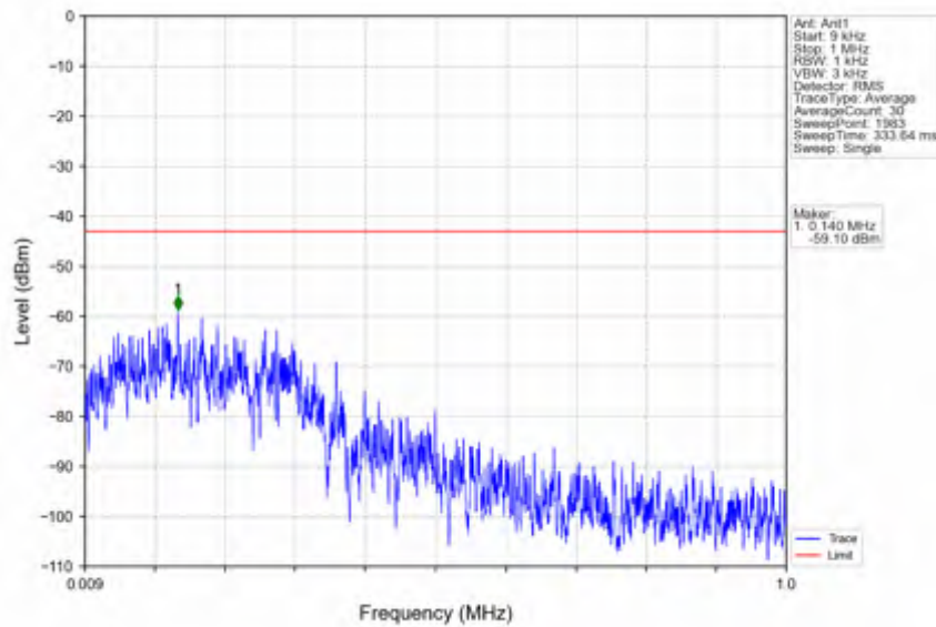
n25_30kHz_SISO_NTNV_20MHz_DFT-s-OFDM QPSK_1860MHz_Inner_1RB_Left
