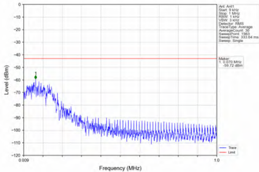
n25_15kHz_SISO_NTNV_40MHz_DFT-s-OFDM QPSK_1870MHz_Inner_1RB_Left
