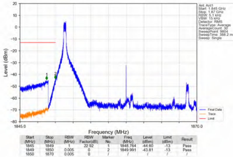
n25_30kHz_SISO_NTNV_20MHz_DFT-s-OFDM PI/2 BPSK_1860MHz_Inner_1RB_Left
