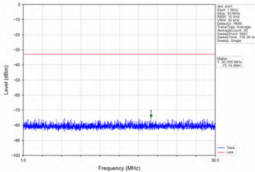
n25_30kHz_SISO_NTNV_10MHz_DFT-s-OFDM_PI/2_BPSK_1855MHz_Inner_1RB_Left
