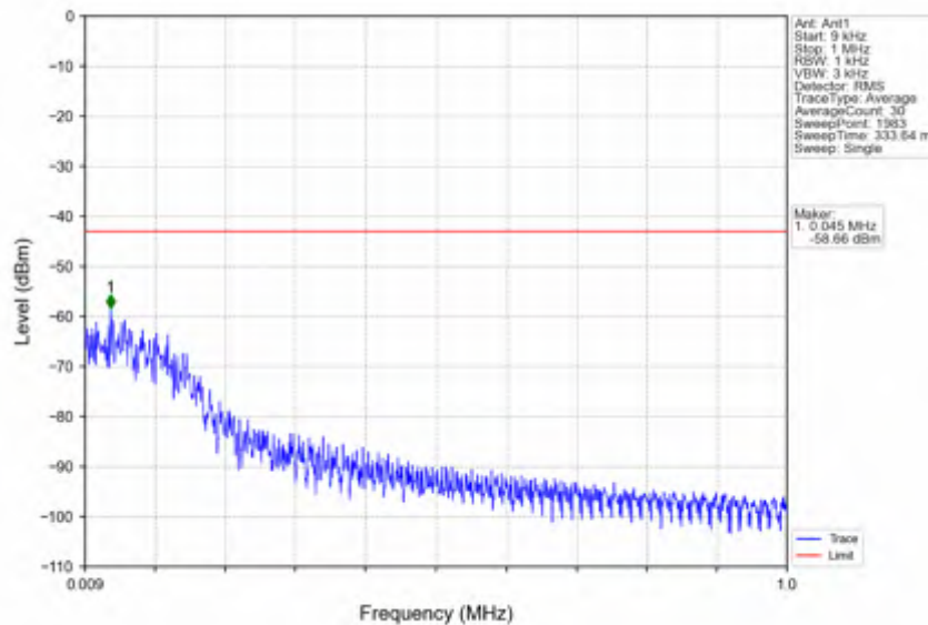
n25_15kHz_SISO_NTNV_40MHz_CP-OFDM QPSK_1870MHz_Inner_1RB_Left
