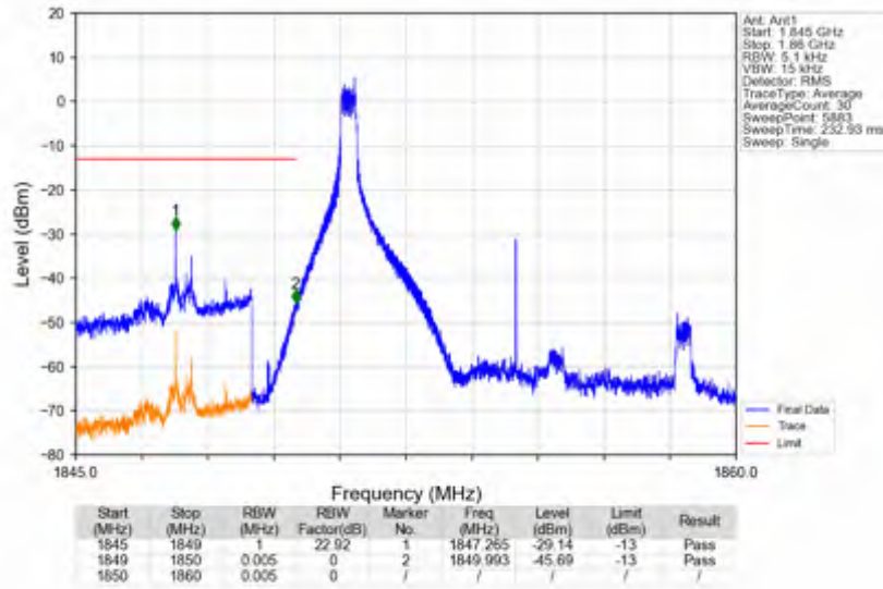
n25_30kHz_SISO_NTNV_10MHz_DFT-s-OFDM PI/2 BPSK_1855MHz_Inner_1RB_Left
