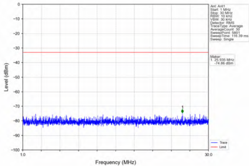
n25_15kHz_SISO_NTNV_40MHz_CP-OFDM QPSK_1870MHz_Inner_1RB_Left
