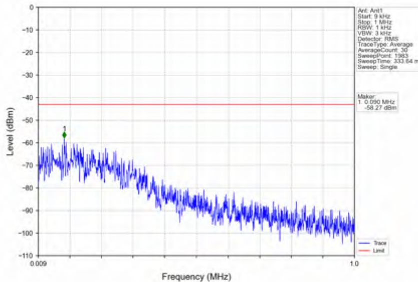
n25_30kHz_SISO_NTNV_10MHz_CP-OFDM QPSK_1855MHz_Inner_1RB_Left
