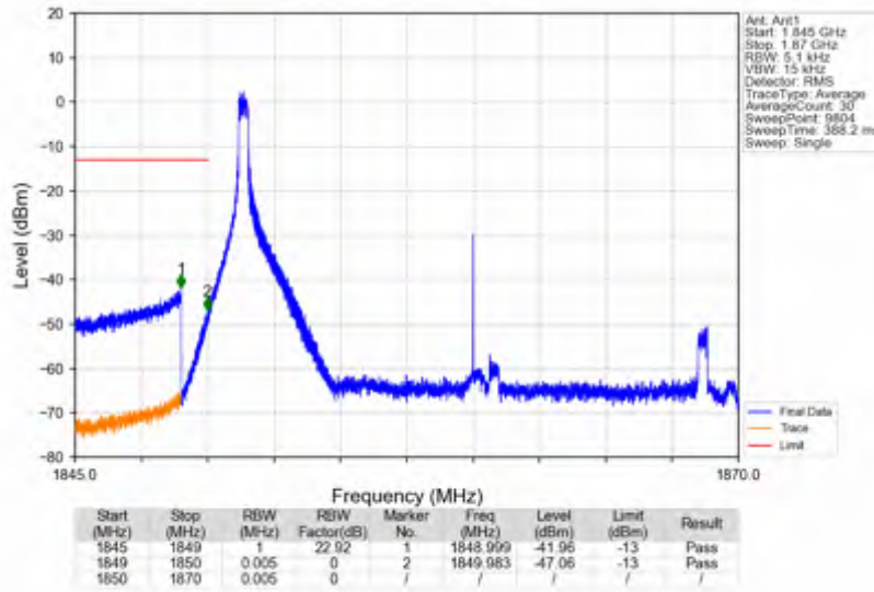
n25_30kHz_SISO_NTNV_20MHz_CP-OFDM QPSK_1860MHz_Inner_1RB_Left
