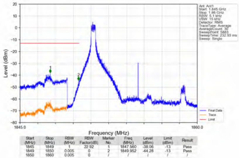
n25_30kHz_SISO_NTNV_10MHz_DFT-s-OFDM QPSK_1855MHz_Inner_1RB_Left
