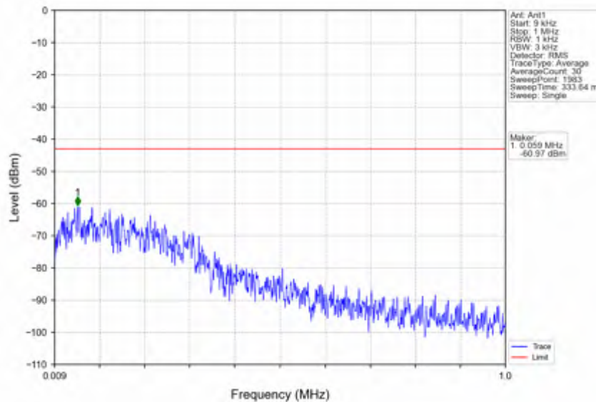
n25_30kHz_SISO_NTNV_20MHz_CP-OFDM QPSK_1860MHz_Inner_1RB_Left
