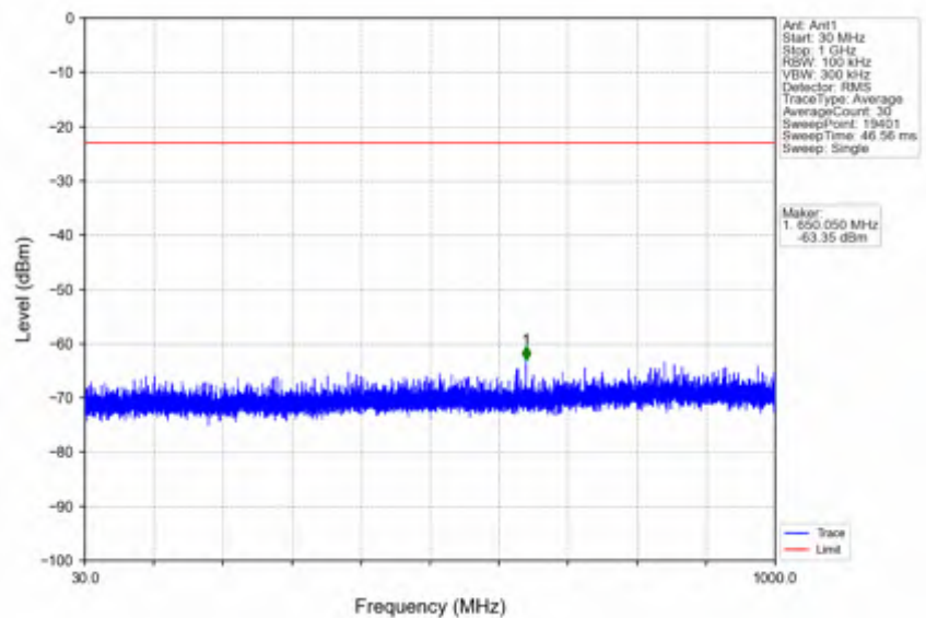
n25_30kHz_SISO_NTNV_20MHz_CP-OFDM QPSK_1860MHz_Inner_1RB_Left
