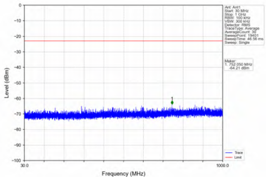
n25_15kHz_SISO_NTNV_30MHz_CP-OFDM QPSK_1865MHz_Inner_1RB_Left
