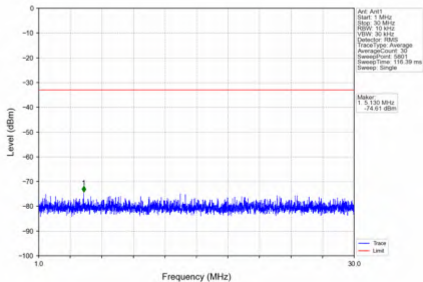
n25_15kHz_SISO_NTNV_20MHz_DFT-s-OFDM QPSK_1860MHz_Inner_1RB_Left
