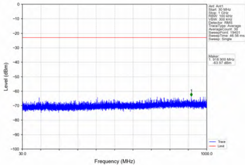
n25_15kHz_SISO_NTNV_20MHz_DFT-s-OFDM QPSK_1860MHz_Inner_1RB_Left
