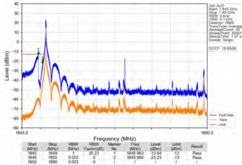
n25_15kHz_SISO_NTNV_40MHz_DFT-s-OFDM PI/2 BPSK_1870MHz_Inner_1RB_Left
