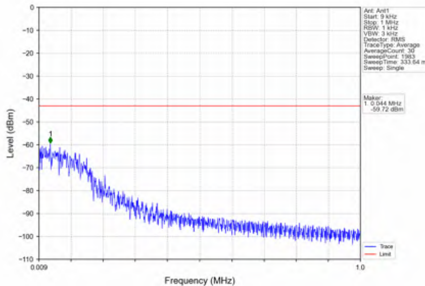
n25_15kHz_SISO_NTNV_20MHz_CP-OFDM QPSK_1860MHz_Inner_1RB_Left
