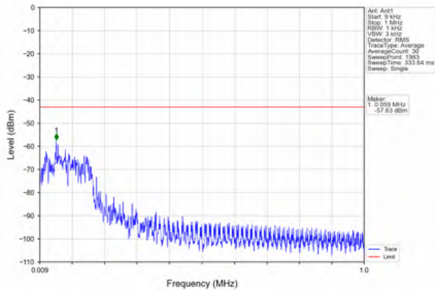
n25_15kHz_SISO_NTV_20MHz_DFT-s-OFDM QPSK_1905MHz_Inner_1RB_Right
