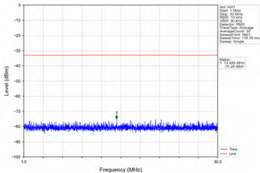
n25_15kHz_SISO_NTNV_30MHz_DFT-s-OFDM QPSK_1865MHz_Inner_1RB_Left
