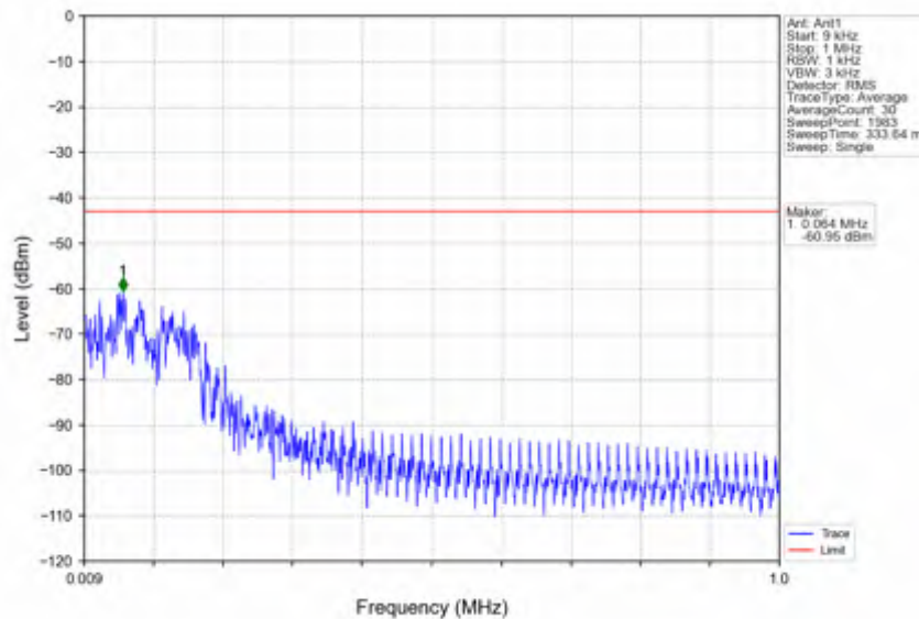
n25_15kHz_SISO_NTNV_20MHz_DFT-s-OFDM PI/2 BPSK_1860MHz_Inner_1RB_Left
