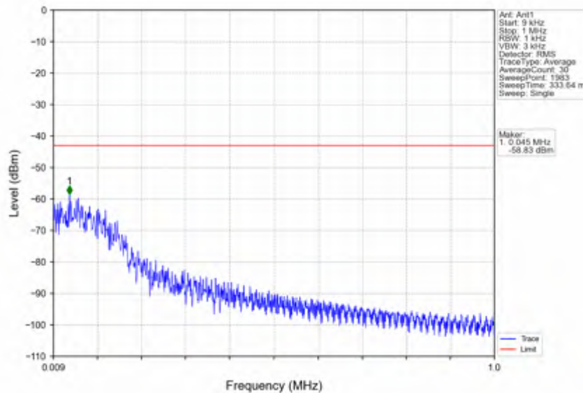
n25_15kHz_SISO_NTNV_30MHz_CP-OFDM QPSK_1865MHz_Inner_1RB_Left
