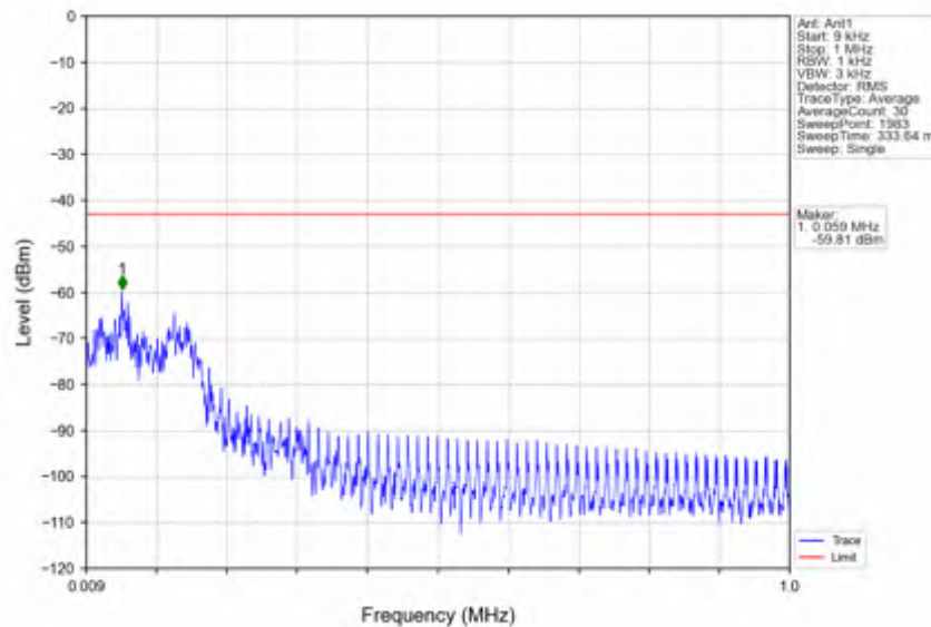
n25_15kHz_SISO_NTNV_40MHz_DFT-s-OFDM PI/2 BPSK_1870MHz_Inner_1RB_Left
