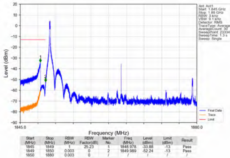
n25_15kHz_SISO_NTNV_30MHz_DFT-s-OFDM QPSK_1865MHz_Inner_1RB_Left
