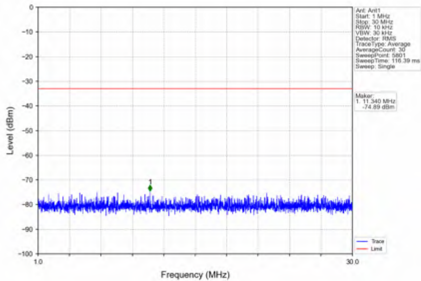
n25_15kHz_SISO_NTNV_20MHz_CP-OFDM QPSK_1860MHz_Inner_1RB_Left
