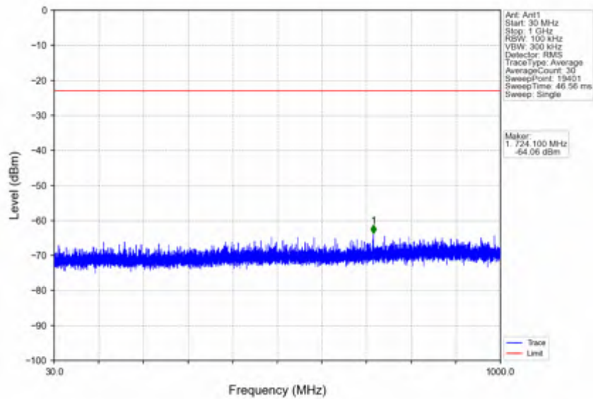
n25_15kHz_SISO_NTNV_30MHz_DFT-s-OFDM QPSK_1865MHz_Inner_1RB_Left
