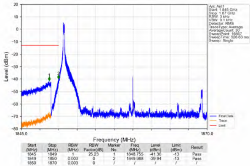
n25_15kHz_SISO_NTNV_20MHz_DFT-s-OFDM QPSK_1860MHz_Inner_1RB_Left
