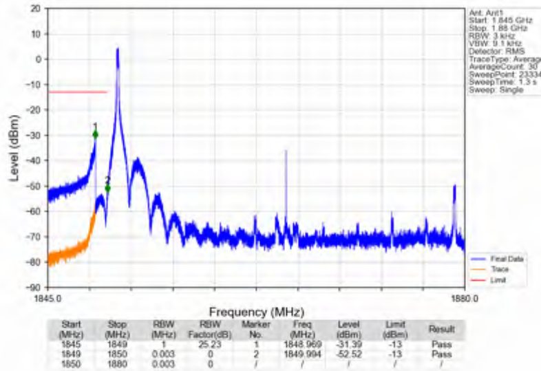
n25_15kHz_SISO_NTNV_30MHz_DFT-s-OFDM PI/2 BPSK_1865MHz_Inner_1RB_Left
