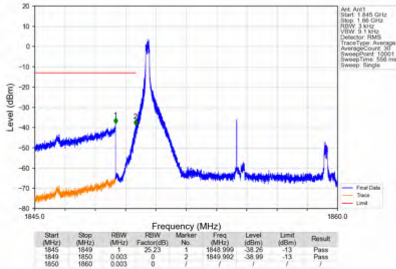
n25_15kHz_SISO_NTNV_10MHz_CP-OFDM QPSK_1855MHz_Inner_1RB_Left
