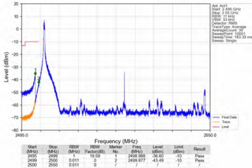
n7_30kHz_SISO_NTNV_50MHz_DFT-s-OFDM PI/2 BPSK_2525MHz_Inner_1RB_Left
