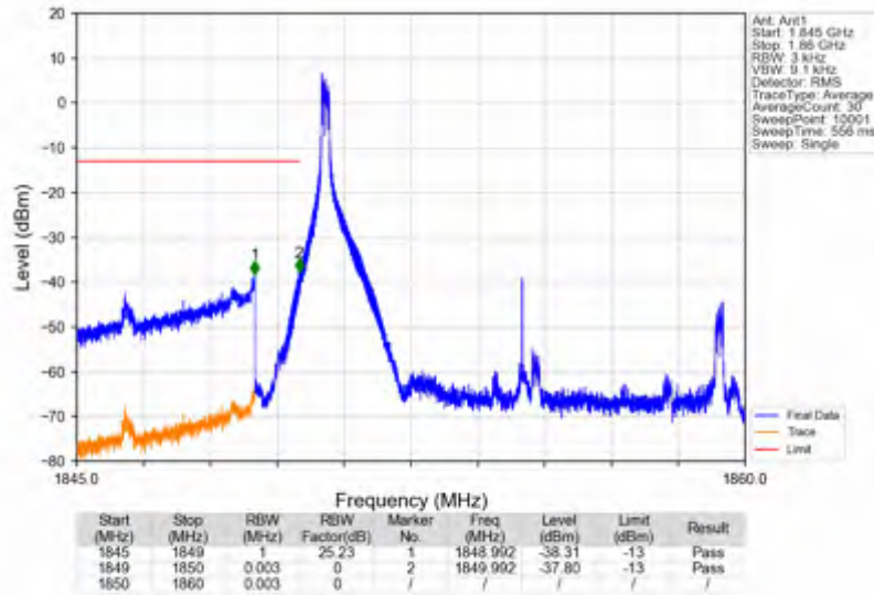
n25_15kHz_SISO_NTNV_10MHz_DFT-s-OFDM PI/2 BPSK_1855MHz_Inner_1RB_Left
