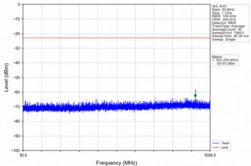
n25_15kHz_SISO_NTNV_10MHz_CP-OFDM QPSK_1855MHz_Inner_1RB_Left
