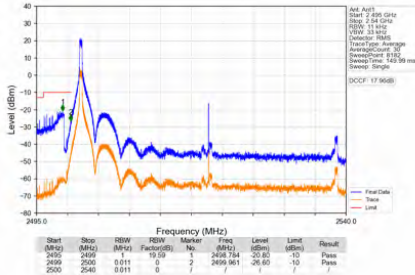
n7_30kHz_SISO_NTNV_40MHz_CP-OFDM QPSK_2520MHz_Inner_1RB_Left
