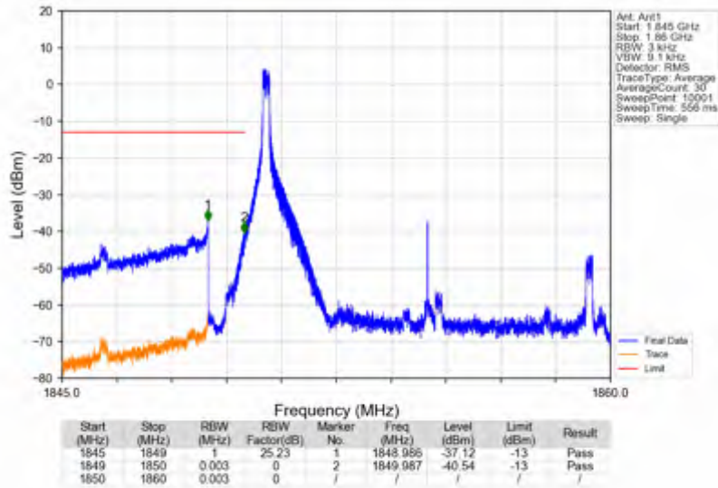
n25_15kHz_SISO_NTNV_10MHz_DFT-s-OFDM QPSK_1855MHz_Inner_1RB_Left
