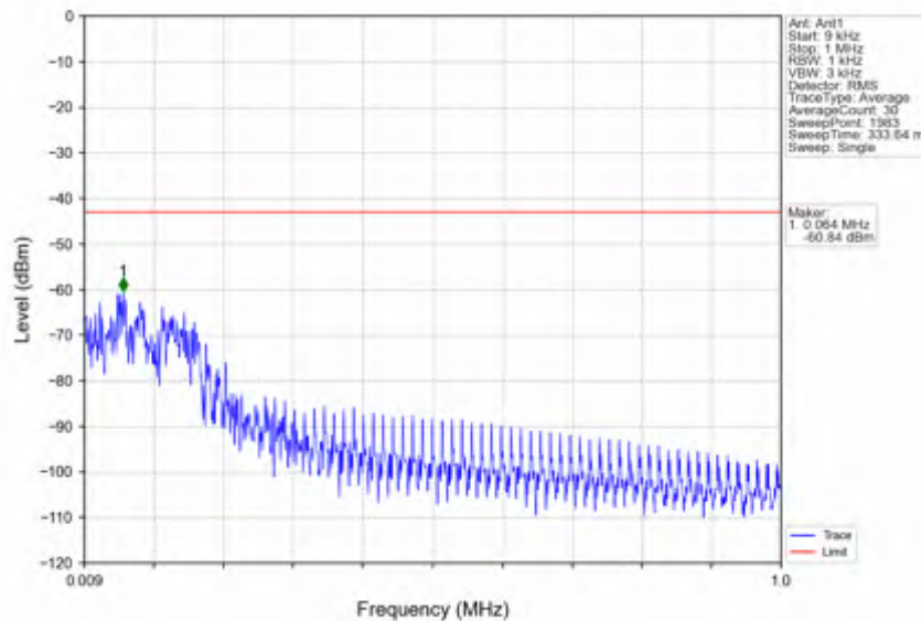
n25_15kHz_SISO_NTNV_10MHz_DFT-s-OFDM PI/2 BPSK_1855MHz_Inner_1RB_Left
