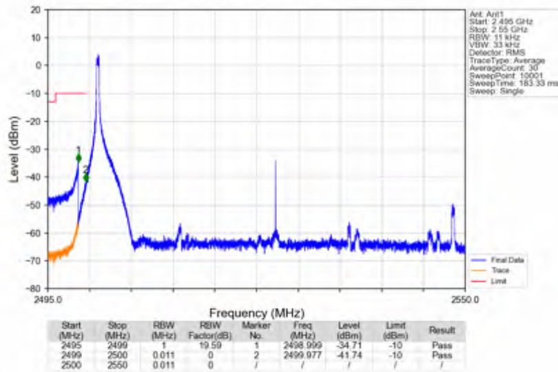
n7_30kHz_SISO_NTNV_50MHz_CP-OFDM QPSK_2525MHz_Inner_1RB_Left
