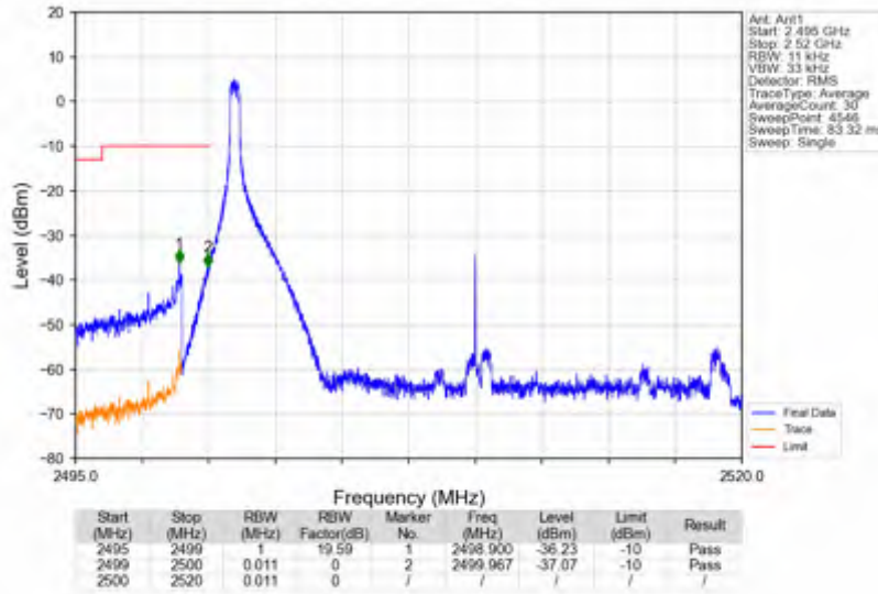
n7_30kHz_SISO_NTNV_20MHz_DFT-s-OFDM_PI/2_BPSK_2510MHz_Edge_1RB_Left
