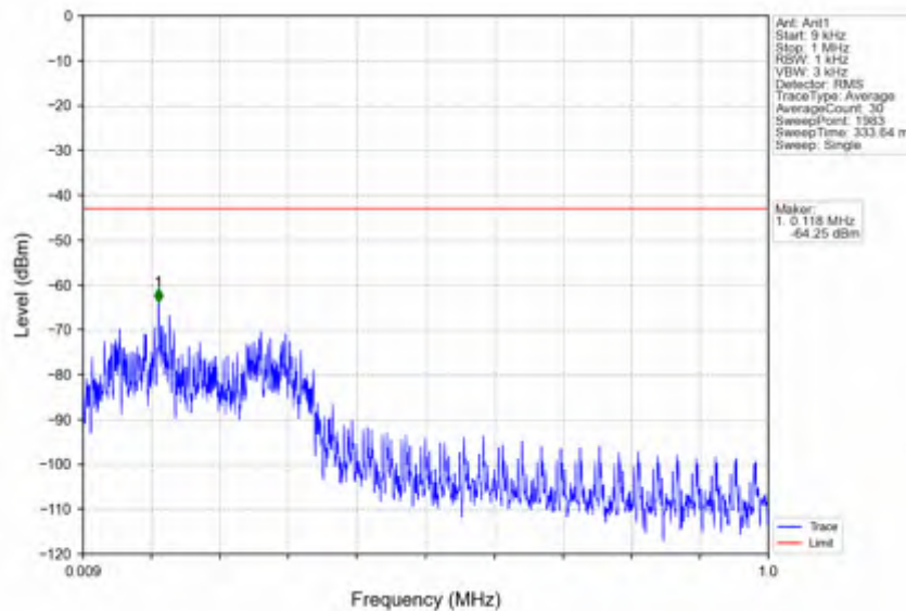
n7_30kHz_SISO_NTNV_20MHz_DFT-s-OFDM PI/2 BPSK_2535MHz_Edge_1RB_Left
