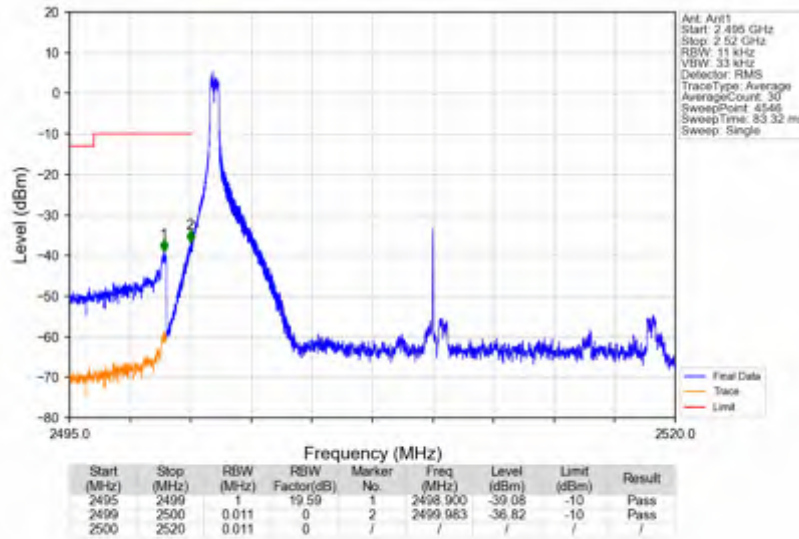
n7_30kHz_SISO_NTV_20MHz_DFT-s-OFDM QPSK_2510MHz_Edge_1RB_Left
