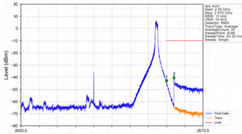
n7_30kHz_SISO_NTNV_20MHz_DFT-s-OFDM PI/2 BPSK_2560MHz_Inner_1RB_Right
