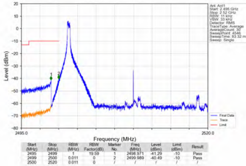
n7_30kHz_SISO_NTNV_20MHz_DFT-s-OFDM QPSK_2510MHz_Inner_1RB_Left
