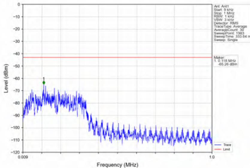
n7_30kHz_SISO_NTV_20MHz_DFT-s-OFDM QPSK_2510MHz_Edge_1RB_Left
