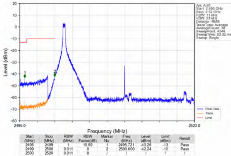
n7_30kHz_SISO_NTNV_20MHz_CP-OFDM QPSK_2510MHz_Inner_1RB_Left
