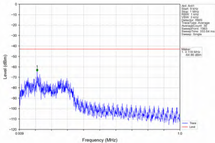
n7_30kHz_SISO_NTNV_20MHz_DFT-s-OFDM_PI/2_BPSK_2510MHz_Edge_1RB_Left
