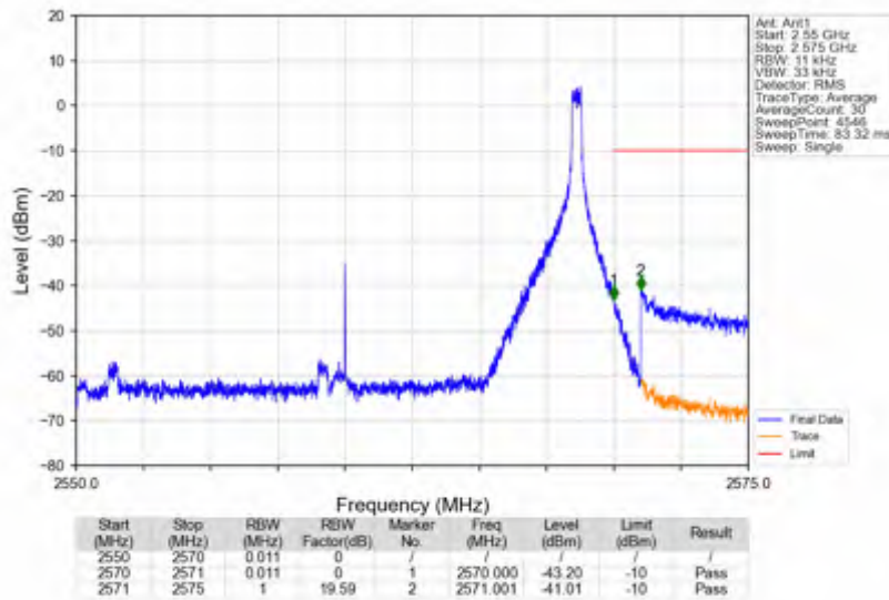
n7_30kHz_SISO_NTNV_20MHz_CP-OFDM QPSK_2560MHz_Inner_1RB_Right
