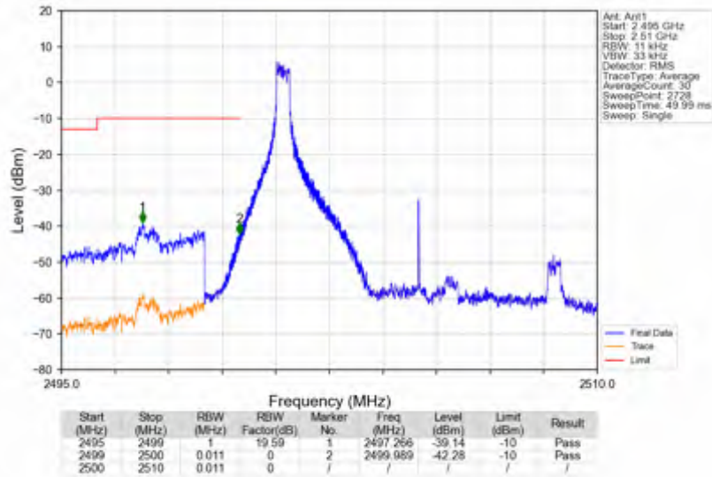
n7_30kHz_SISO_NTV_10MHz_DFT-s-OFDM QPSK_2505MHz_Inner_1RB_Left
