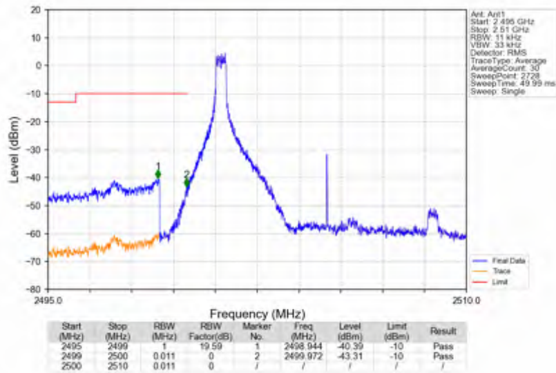
n7_30kHz_SISO_NTNV_10MHz_CP-OFDM QPSK_2505MHz_Inner_1RB_Left
