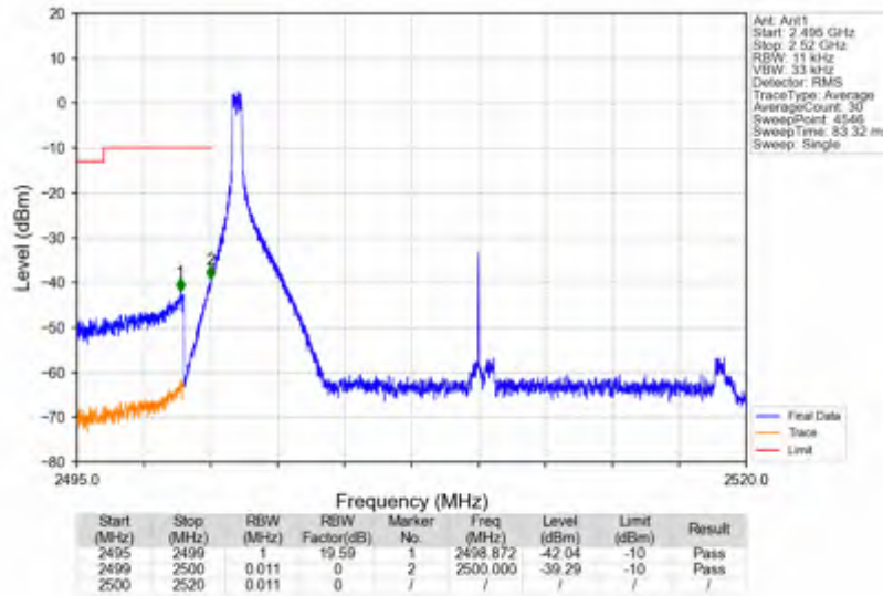
n7_30kHz_SISO_NTNV_20MHz_CP-OFDM QPSK_2510MHz_Edge_1RB_Left
