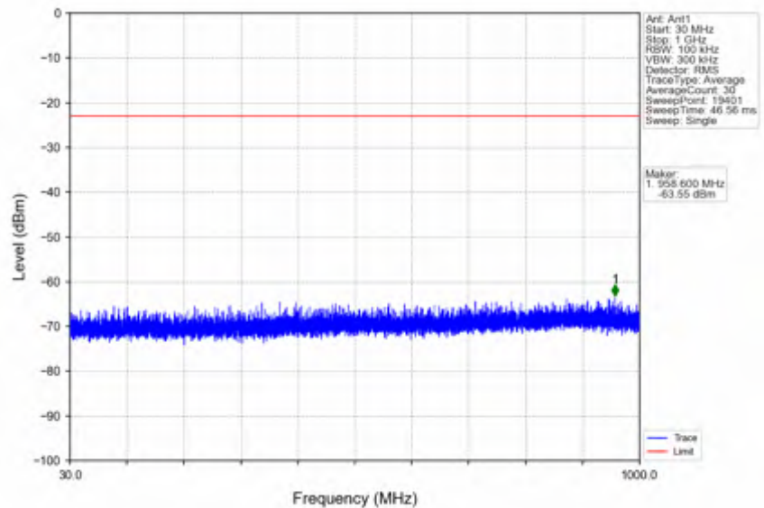
n7_30kHz_SISO_NTNV_20MHz_CP-OFDM QPSK_2510MHz_Edge_1RB_Left
