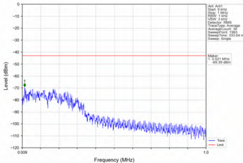
n7_30kHz_SISO_NTNV_20MHz_CP-OFDM QPSK_2510MHz_Edge_1RB_Left
