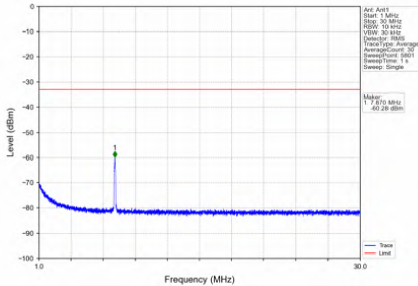
n7_15kHz_SISO_NTNV_30MHz_CP-OFDM QPSK_2555MHz_Inner_1RB_Right
