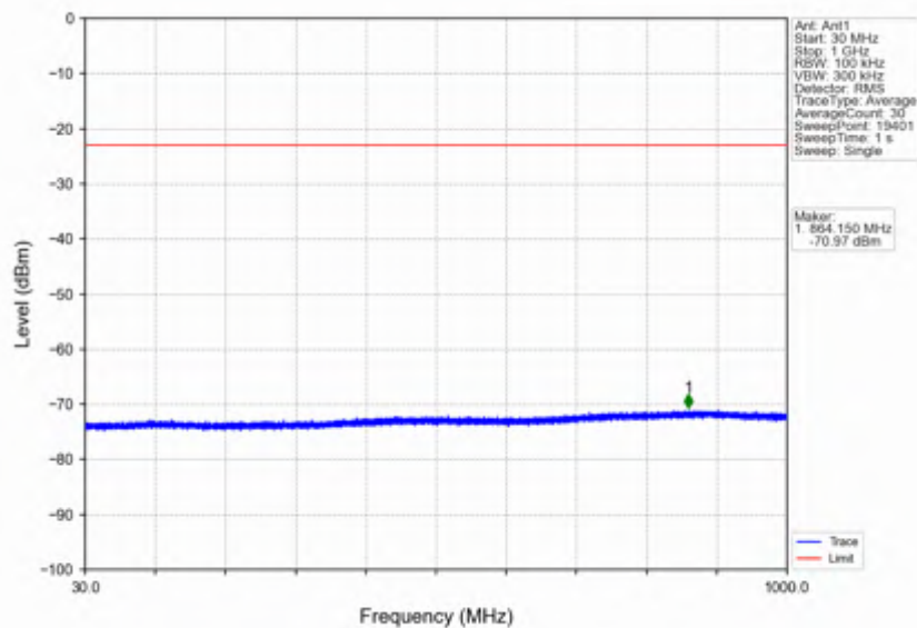
n7_15kHz_SISO_NTNV_20MHz_CP-OFDM QPSK_2560MHz_Inner_1RB_Right
