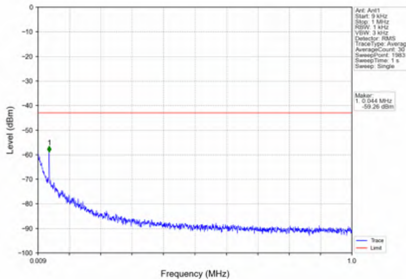
n7_15kHz_SISO_NTNV_30MHz_CP-OFDM QPSK_2515MHz_Inner_1RB_Left
