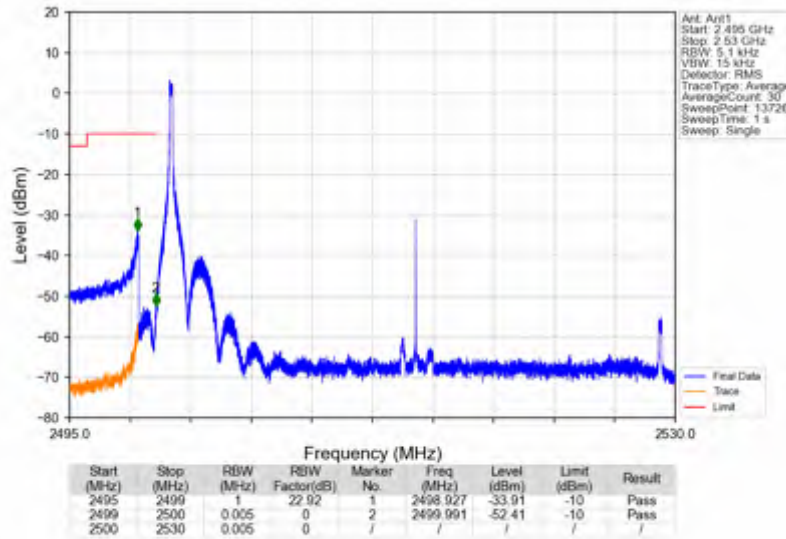
n7_15kHz_SISO_NTNV_30MHz_CP-OFDM QPSK_2515MHz_Inner_1RB_Left
