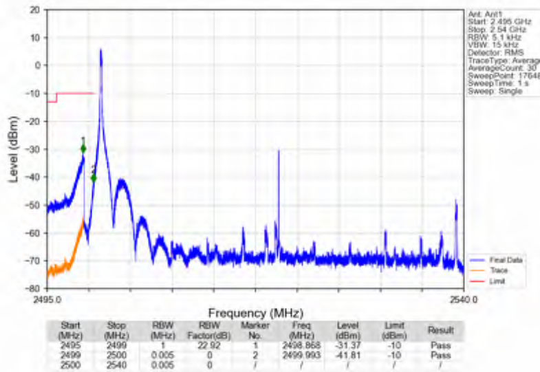
n7_15kHz_SISO_NTNV_40MHz_DFT-s-OFDM_QPSK_2520MHz_Inner_1RB_Left
