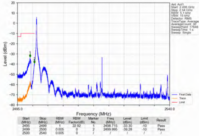
n7_15kHz_SISO_NTNV_40MHz_DFT-s-OFDM_PI/2_BPSK_2520MHz_Edge_1RB_Left
