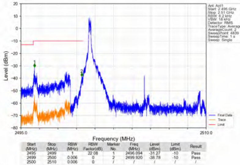
n7_15kHz_SISO_NTNV_10MHz_DFT-s-OFDM PI/2 BPSK_2505MHz_Inner_1RB_Left
