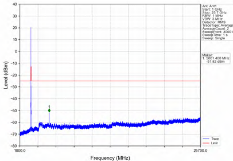
n7_15kHz_SISO_NTNV_20MHz_DFT-s-OFDM QPSK_2510MHz_Edge_1RB_Left
