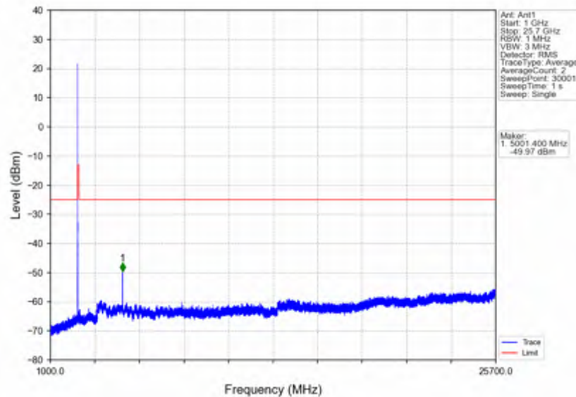
n7_15kHz_SISO_NTNV_10MHz_DFT-s-OFDM QPSK_2505MHz_Inner_1RB_Left
