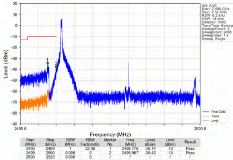
n7_15kHz_SISO_NTNV_20MHz_CP-OFDM QPSK_2510MHz_Inner_1RB_Left
