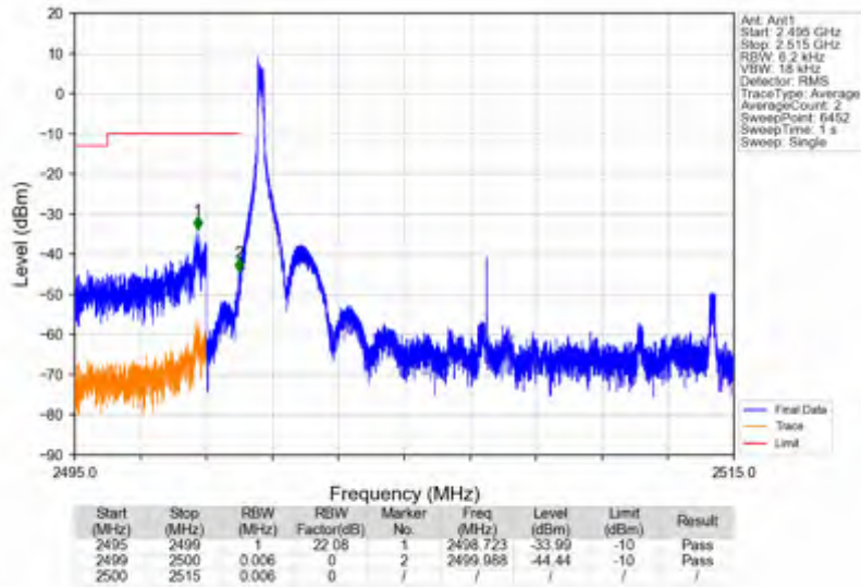
n7_15kHz_SISO_NTV_15MHz_DFT-s-OFDM PI/2 BPSK_2507.5MHz_Inner_1RB_Left
