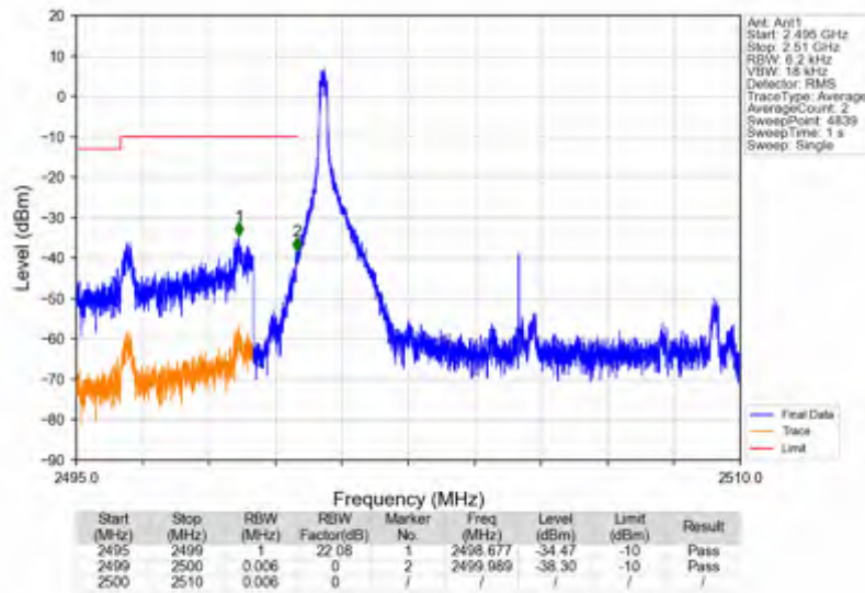
n7_15kHz_SISO_NTV_10MHz_DFT-s-OFDM_QPSK_2505MHz_Inner_1RB_Left
