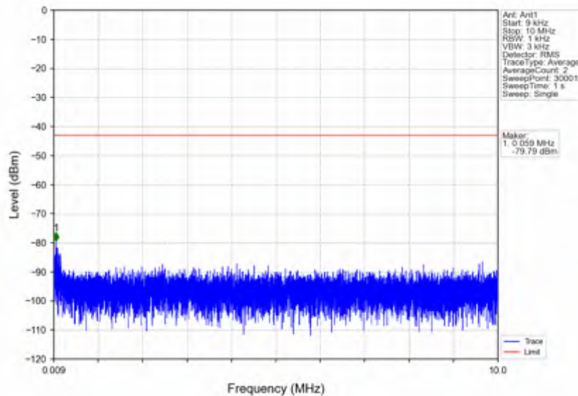
n7_15kHz_SISO_NTV_15MHz_DFT-s-OFDM PI/2 BPSK_2507.5MHz_Inner_1RB_Left
