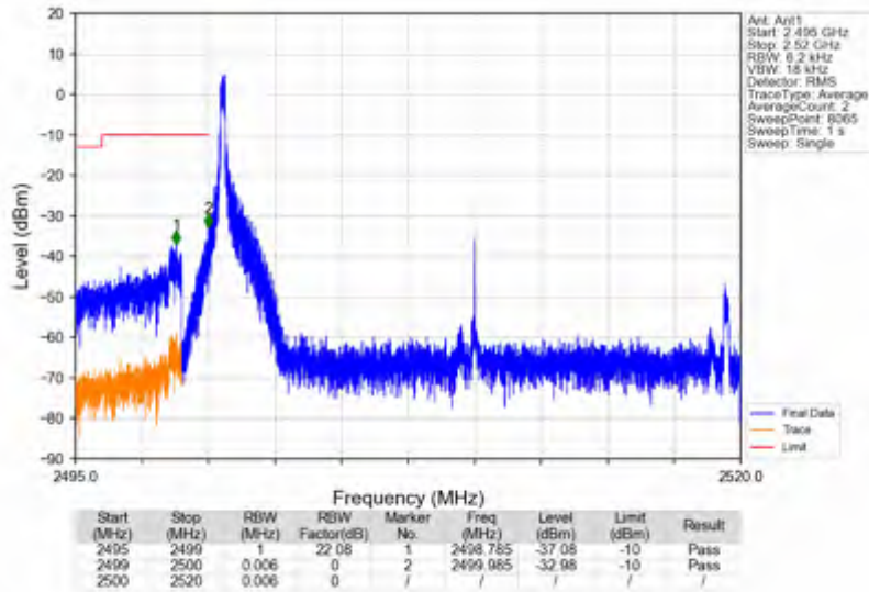
n7_15kHz_SISO_NTNV_20MHz_CP-OFDM QPSK_2510MHz_Edge_1RB_Left
