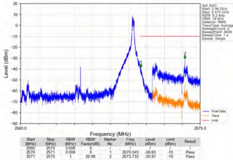
n7_15kHz_SISO_NTNV_10MHz_DFT-s-OFDM PI/2 BPSK_2565MHz_Inner_1RB_Right
