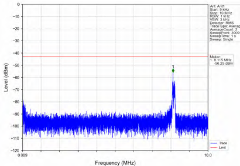
n7_15kHz_SISO_NTNV_10MHz_DFT-s-OFDM PI/2 BPSK_2565MHz_Inner_1RB_Right
