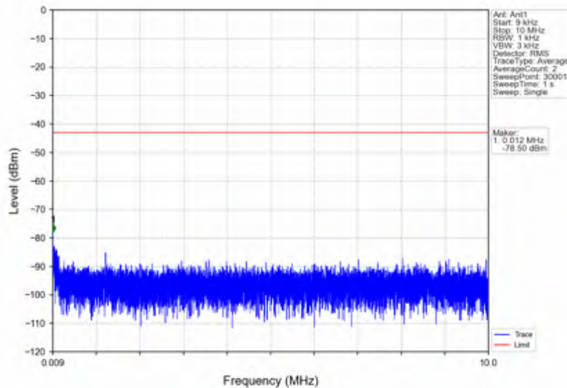
n7_15kHz_SISO_NTNV_20MHz_CP-OFDM QPSK_2510MHz_Edge_1RB_Left
