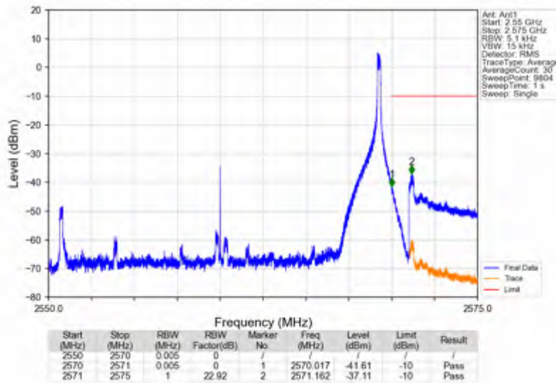
n7_15kHz_SISO_NTNV_20MHz_DFT-s-OFDM QPSK_2560MHz_Inner_1RB_Right
