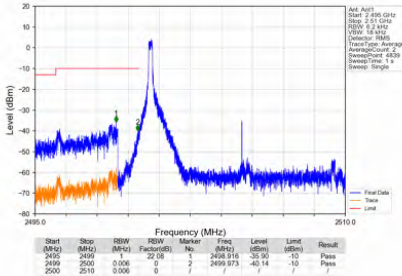
n7_15kHz_SISO_NTNV_10MHz_CP-OFDM QPSK_2505MHz_Inner_1RB_Left
