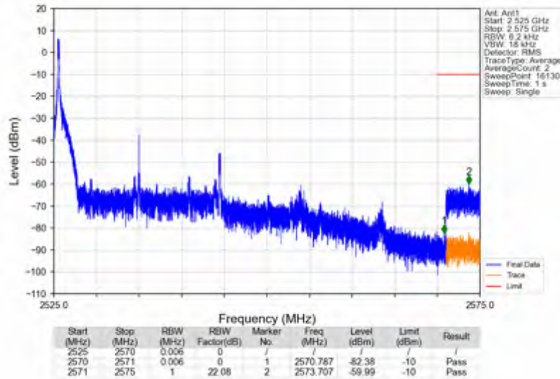
n7_15kHz_SISO_NTNV_20MHz_DFT-s-OFDM PI/2 BPSK_2535MHz_Edge_1RB_Left
