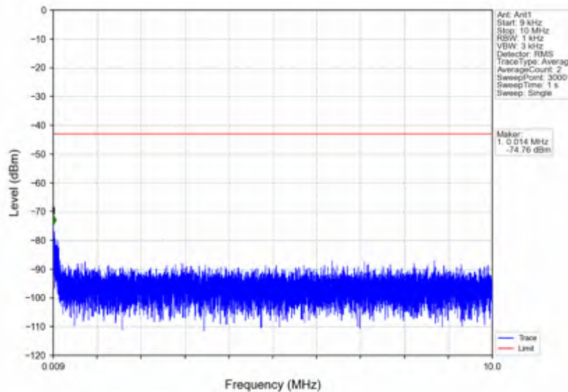
n7_15kHz_SISO_NTNV_10MHz_CP-OFDM QPSK_2505MHz_Inner_1RB_Left
