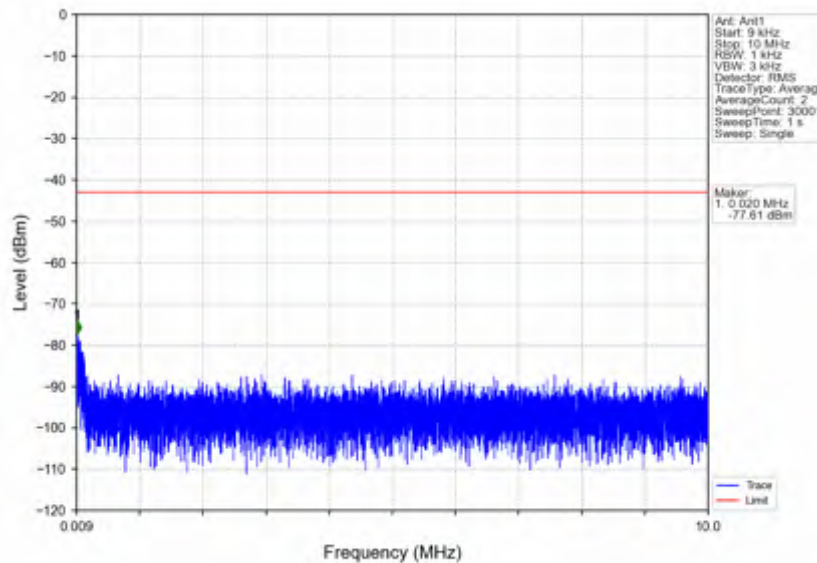
n7_15kHz_SISO_NTNV_20MHz_CP-OFDM QPSK_2510MHz_Inner_1RB_Left
