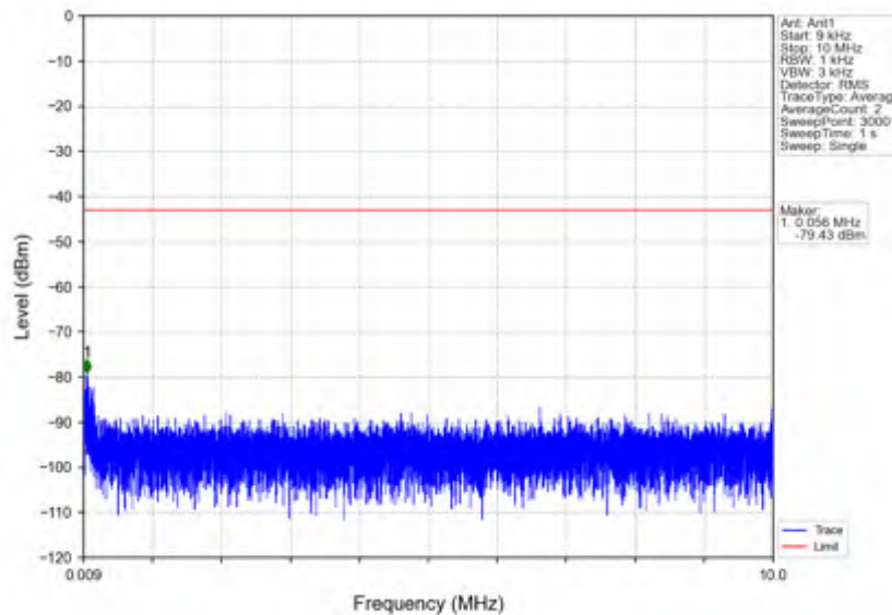
n7_15kHz_SISO_NTNV_10MHz_DFT-s-OFDM PI/2 BPSK_2505MHz_Inner_1RB_Left
