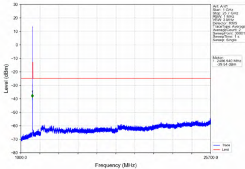
n7_15kHz_SISO_NTV_10MHz_DFT-s-OFDM_QPSK_2505MHz_Inner_1RB_Left
