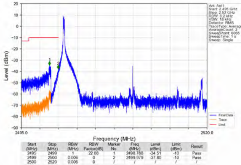
n7_15kHz_SISO_NTNV_20MHz_DFT-s-OFDM PI/2 BPSK_2510MHz_Inner_1RB_Left
