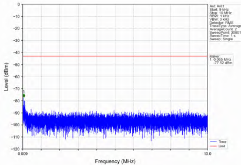
n7_15kHz_SISO_NTV_10MHz_DFT-s-OFDM_QPSK_2505MHz_Inner_1RB_Left
