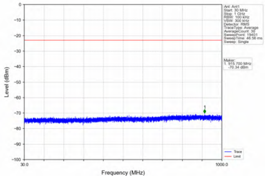
n2_30kHz_SISO_NTNV_20MHz_CP-OFDM QPSK_1900MHz_Inner_1RB_Right
