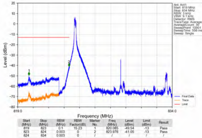
n5_15kHz_SISO_NTNV_10MHz_DFT-s-OFDM PI/2 BPSK_829MHz_Inner_1RB_Left
