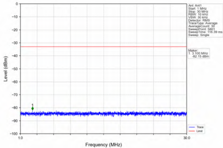
n2_30kHz_SISO_NTV_10MHz_DFT-s-OFDM QPSK_1880MHz_Edge_1RB_Left
