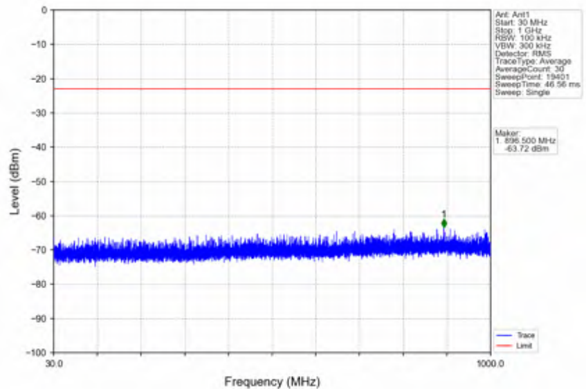
n2_15kHz_SISO_NTNV_10MHz_CP-OFDM QPSK_1855MHz_Edge_1RB_Left
