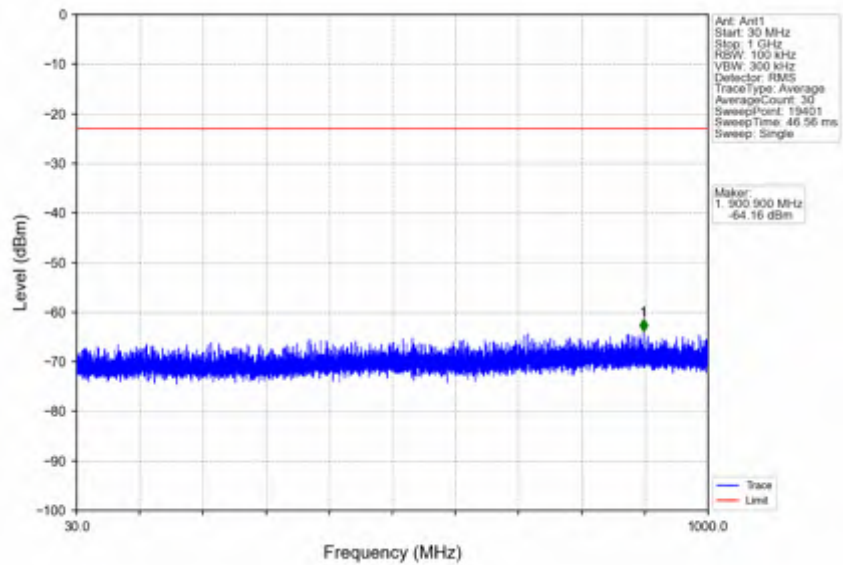
n2_15kHz_SISO_NTV_10MHz_DFT-s-OFDM QPSK_1880MHz_Edge_1RB_Left
