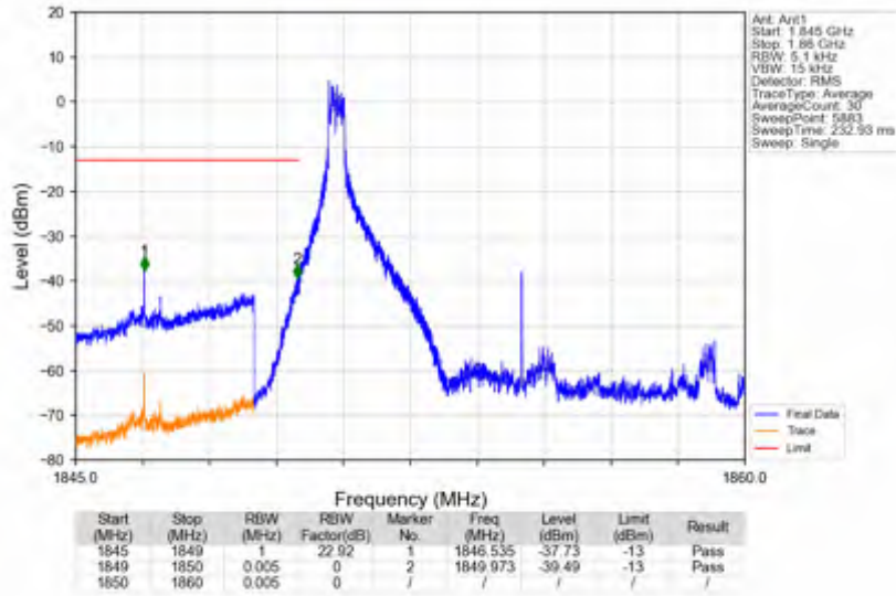
n2_30kHz_SISO_NTNV_10MHz_DFT-s-OFDM_PI/2_BPSK_1855MHz_Edge_1RB_Left
