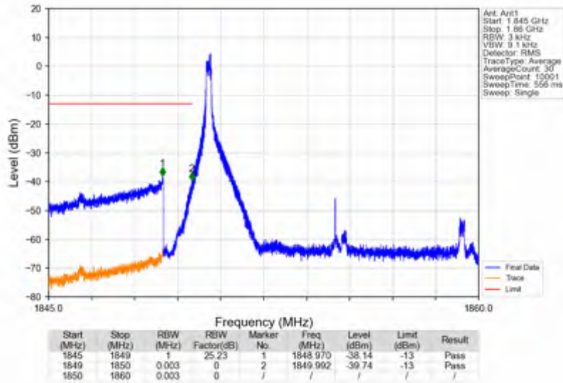
n2_15kHz_SISO_NTNV_10MHz_CP-OFDM QPSK_1855MHz_Inner_1RB_Left
