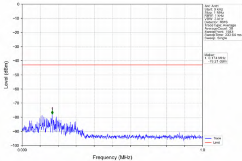
n2_30kHz_SISO_NTV_10MHz_DFT-s-OFDM QPSK_1855MHz_Inner_1RB_Left
