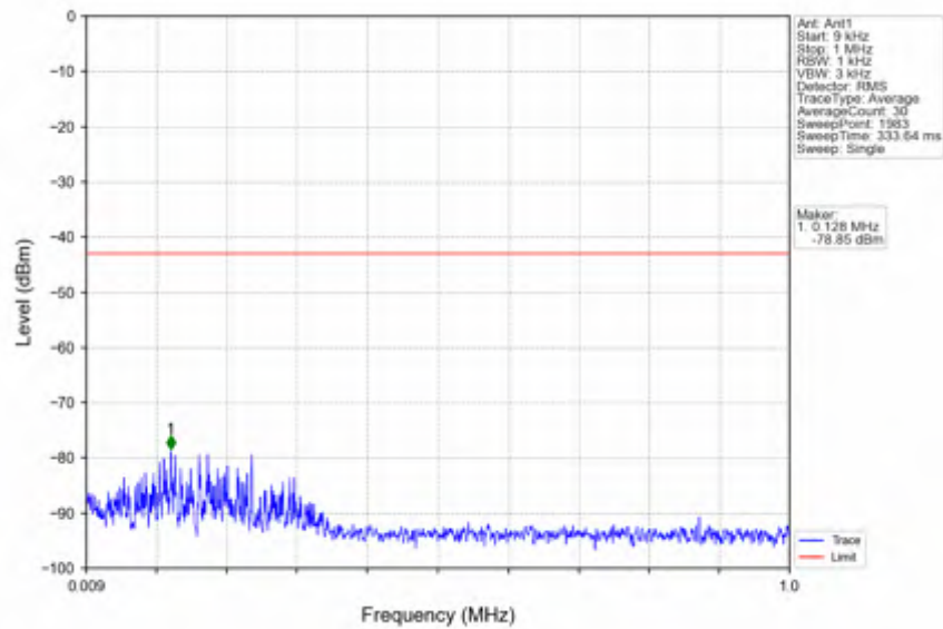
n2_30kHz_SISO_NTV_10MHz_DFT-s-OFDM QPSK_1855MHz_Edge_1RB_Left
