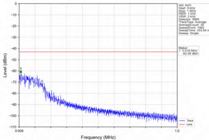
n2_15kHz_SISO_NTNV_20MHz_CP-OFDM QPSK_1880MHz_Edge_1RB_Left
