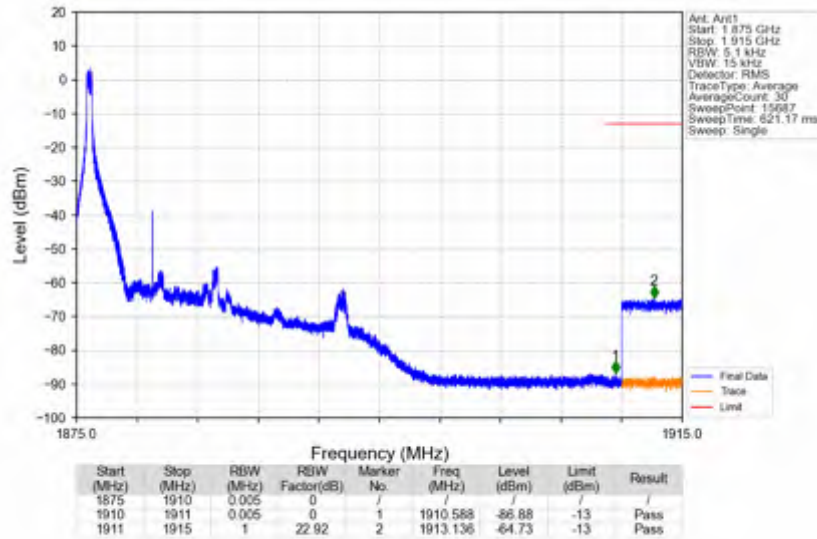
n2_30kHz_SISO_NTV_10MHz_DFT-s-OFDM QPSK_1880MHz_Edge_1RB_Left
