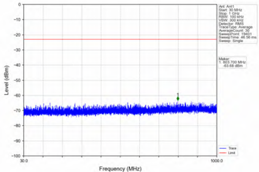
n2_15kHz_SISO_NTV_20MHz_DFT-s-OFDM QPSK_1860MHz_Edge_1RB_Left
