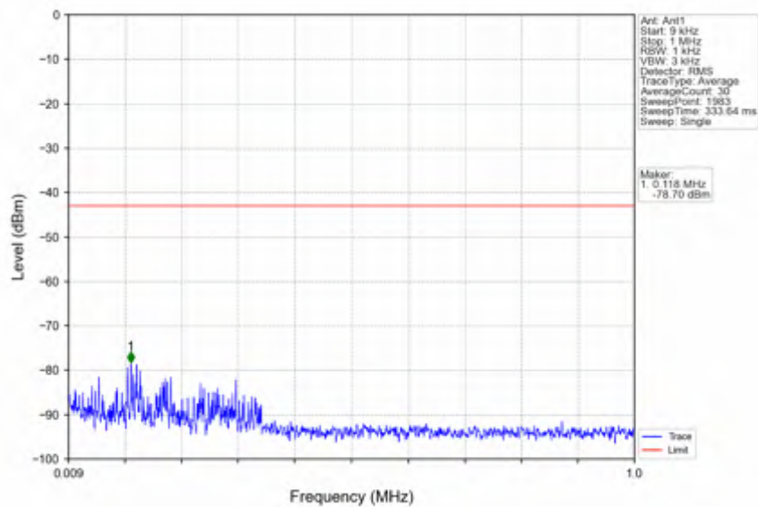
n2_30kHz_SISO_NTNV_10MHz_DFT-s-OFDM_PI/2_BPSK_1855MHz_Edge_1RB_Left
