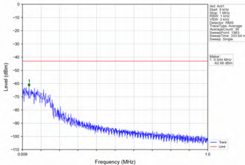
n2_15kHz_SISO_NTNV_20MHz_CP-OFDM QPSK_1860MHz_Edge_1RB_Left
