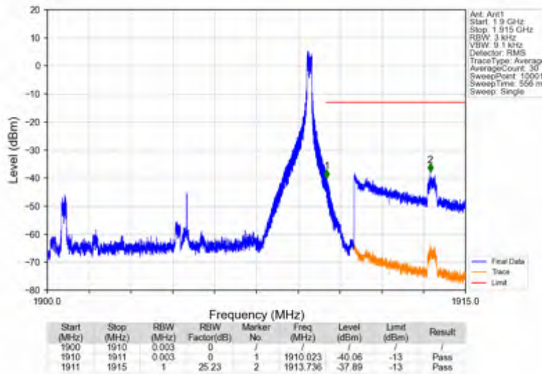
n2_15kHz_SISO_NTNV_10MHz_DFT-s-OFDM QPSK_1905MHz_Inner_1RB_Right
