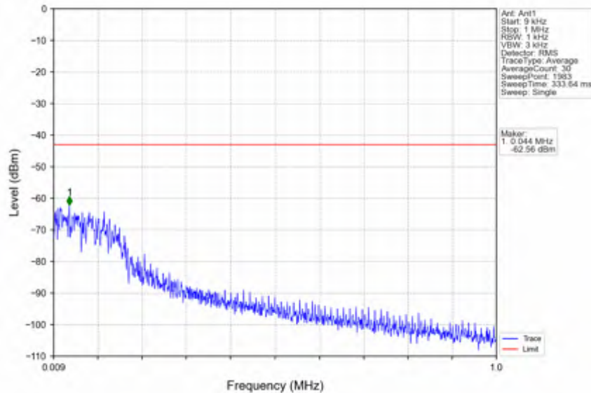
n2_15kHz_SISO_NTNV_10MHz_CP-OFDM QPSK_1880MHz_Edge_1RB_Left
