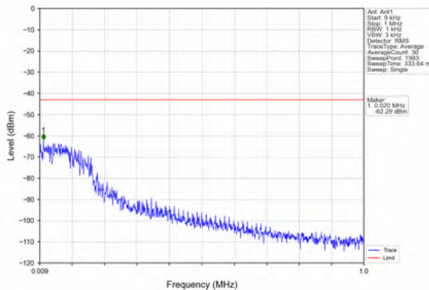
n2_15kHz_SISO_NTNV_5MHz_CP-OFDM QPSK_1880MHz_Edge_1RB_Left
