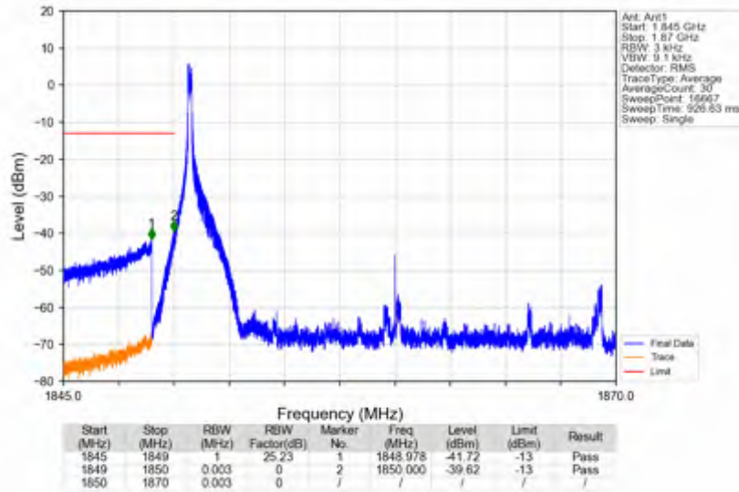
n2_15kHz_SISO_NTV_20MHz_DFT-s-OFDM QPSK_1860MHz_Inner_1RB_Left
