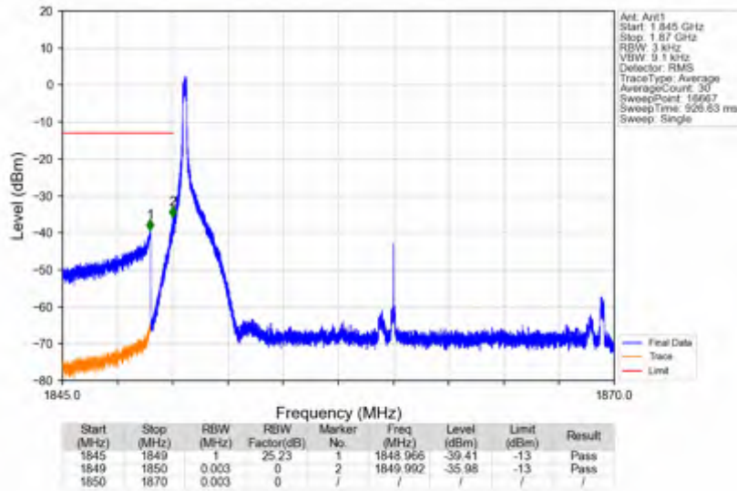
n2_15kHz_SISO_NTNV_20MHz_CP-OFDM QPSK_1860MHz_Edge_1RB_Left
