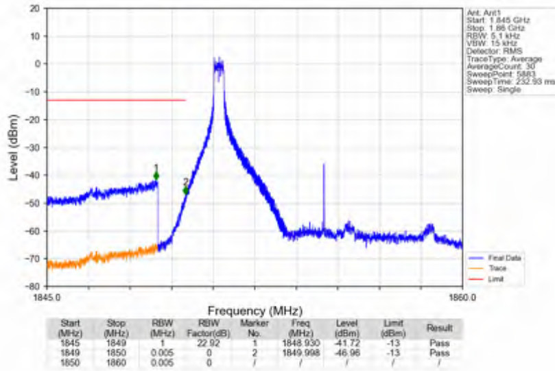
n2_30kHz_SISO_NTNV_10MHz_CP-OFDM QPSK_1855MHz_Inner_1RB_Left
