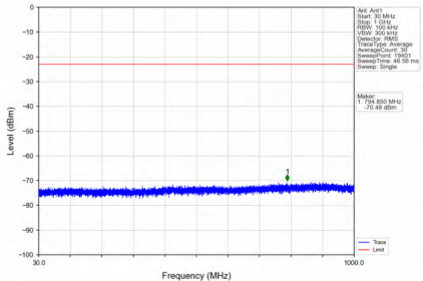
n2_30kHz_SISO_NTNV_10MHz_CP-OFDM QPSK_1855MHz_Inner_1RB_Left
