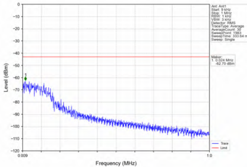
n2_15kHz_SISO_NTNV_10MHz_CP-OFDM QPSK_1855MHz_Edge_1RB_Left
