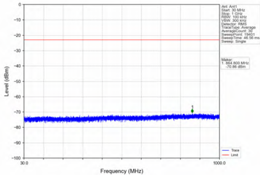
n2_30kHz_SISO_NTNV_10MHz_DFT-s-OFDM QPSK_1855MHz_Inner_1RB_Left
