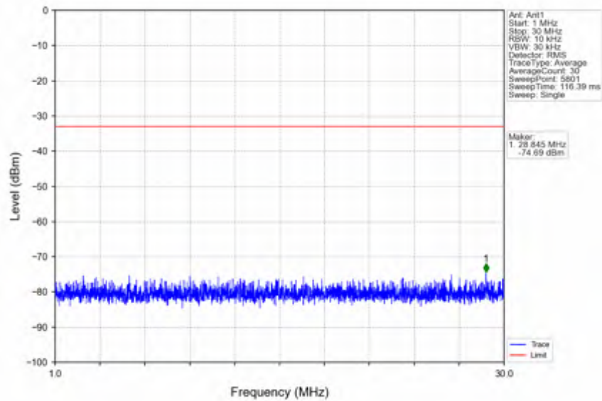
n2_15kHz_SISO_NTNV_10MHz_CP-OFDM QPSK_1880MHz_Edge_1RB_Left
