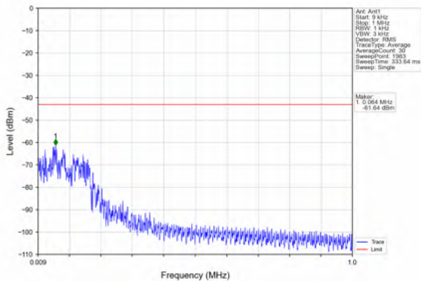
n2_15kHz_SISO_NTNV_20MHz_DFT-s-OFDM_PI/2_BPSK_1860MHz_Edge_1RB_Left
