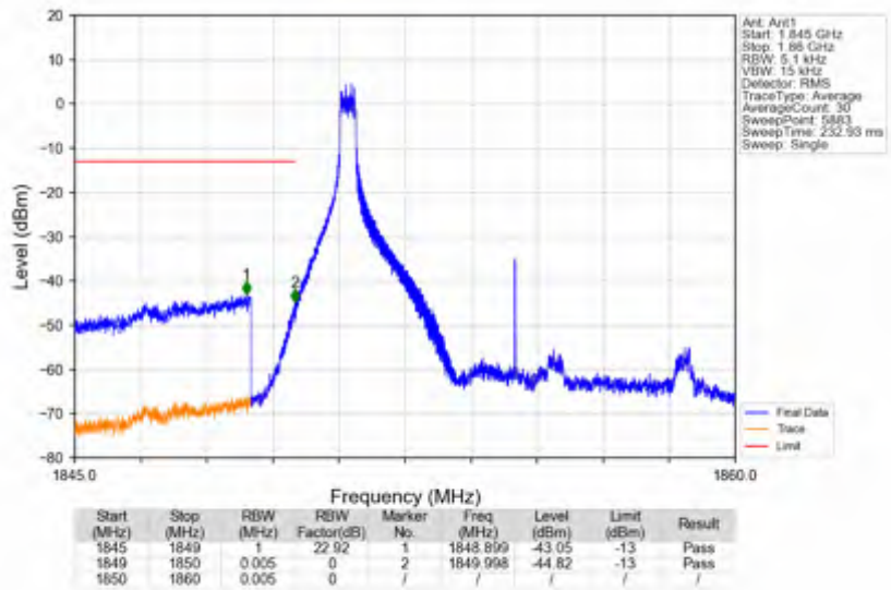
n2_30kHz_SISO_NTV_10MHz_DFT-s-OFDM QPSK_1855MHz_Inner_1RB_Left
