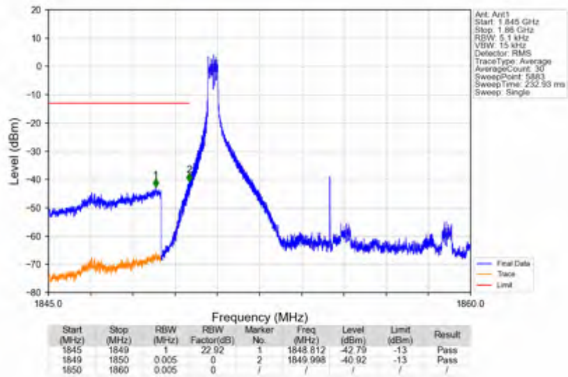
n2_30kHz_SISO_NTNV_10MHz_DFT-s-OFDM QPSK_1855MHz_Edge_1RB_Left
