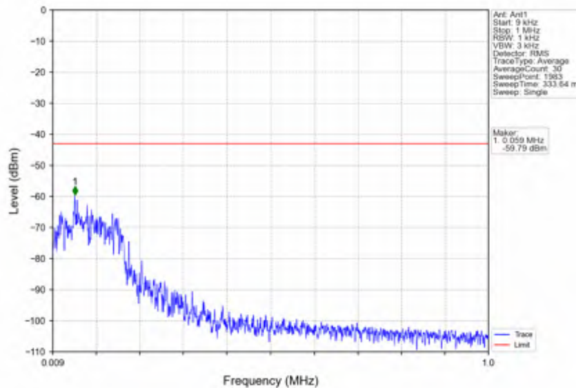
n2_15kHz_SISO_NTV_20MHz_DFT-s-OFDM QPSK_1860MHz_Edge_1RB_Left
