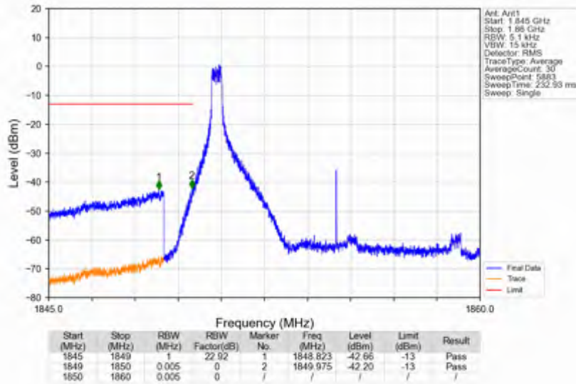
n2_30kHz_SISO_NTNV_10MHz_CP-OFDM QPSK_1855MHz_Edge_1RB_Left
