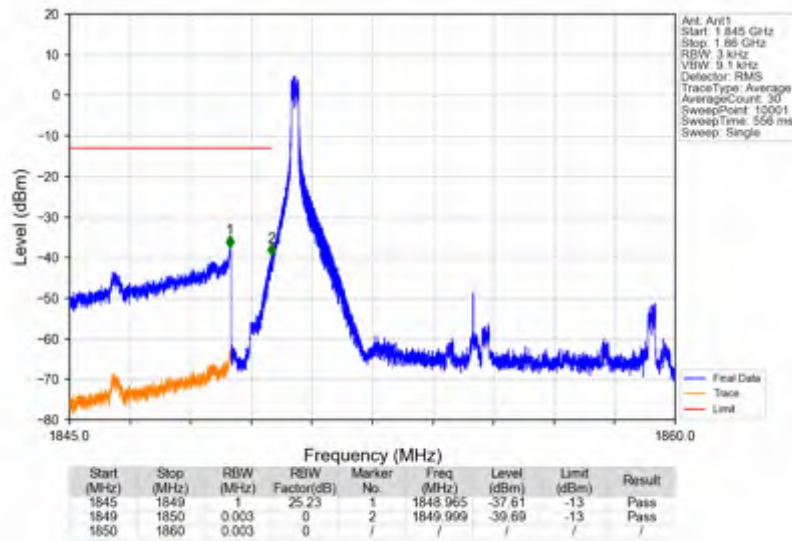
n2_15kHz_SISO_NTNV_10MHz_DFT-s-OFDM QPSK_1855MHz_Inner_1RB_Left
