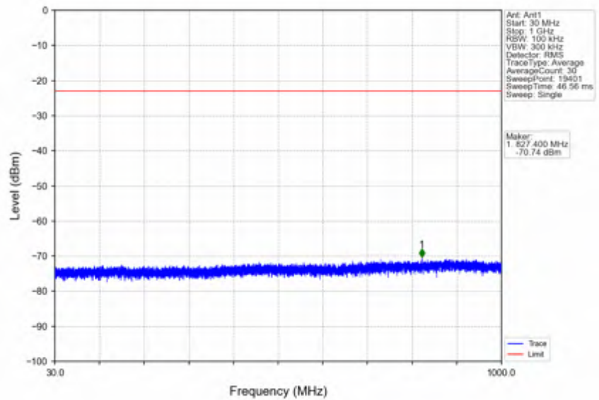
n2_30kHz_SISO_NTNV_10MHz_CP-OFDM QPSK_1855MHz_Edge_1RB_Left
