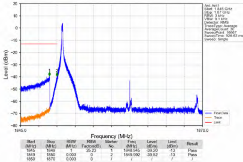
n2_15kHz_SISO_NTNV_20MHz_CP-OFDM QPSK_1860MHz_Inner_1RB_Left
