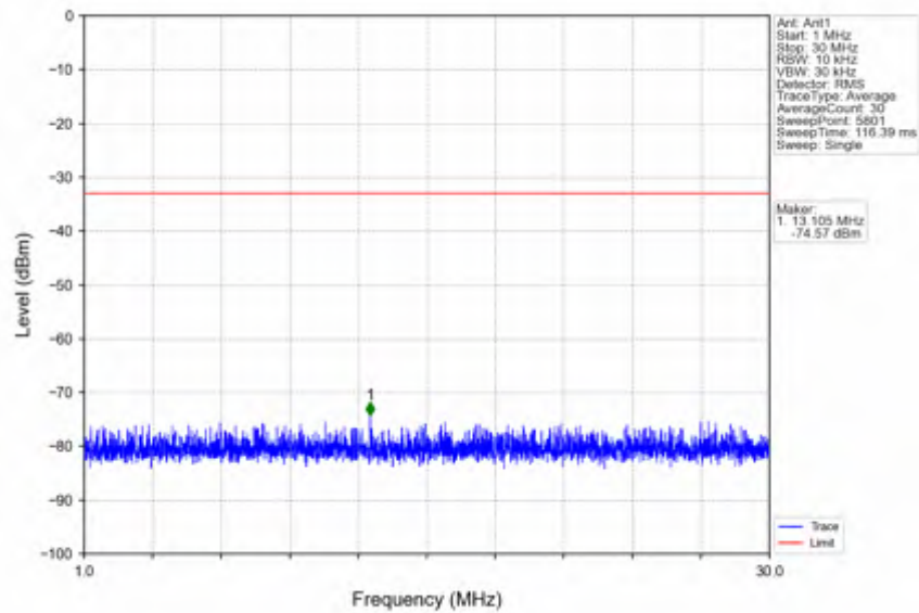
n2_15kHz_SISO_NTNV_20MHz_DFT-s-OFDM_QPSK_1880MHz_Edge_1RB_Left
