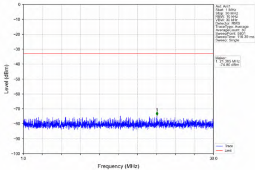
n2_15kHz_SISO_NTV_10MHz_DFT-s-OFDM QPSK_1855MHz_Edge_1RB_Left
