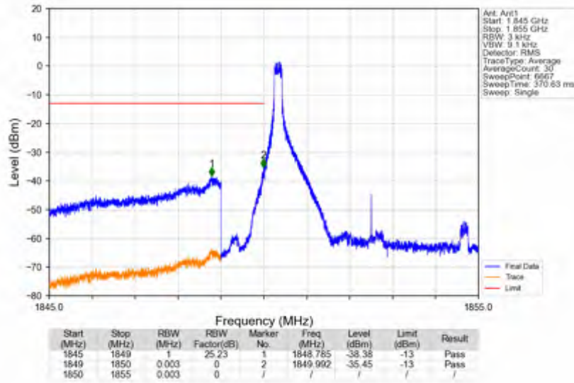
n2_15kHz_SISO_NTV_5MHz_CP-OFDM QPSK_1852.5MHz_Edge_1RB_Left
