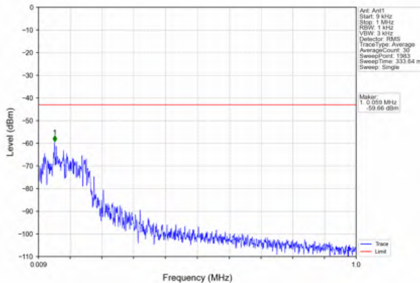
n2_15kHz_SISO_NTV_10MHz_DFT-s-OFDM QPSK_1855MHz_Edge_1RB_Left
