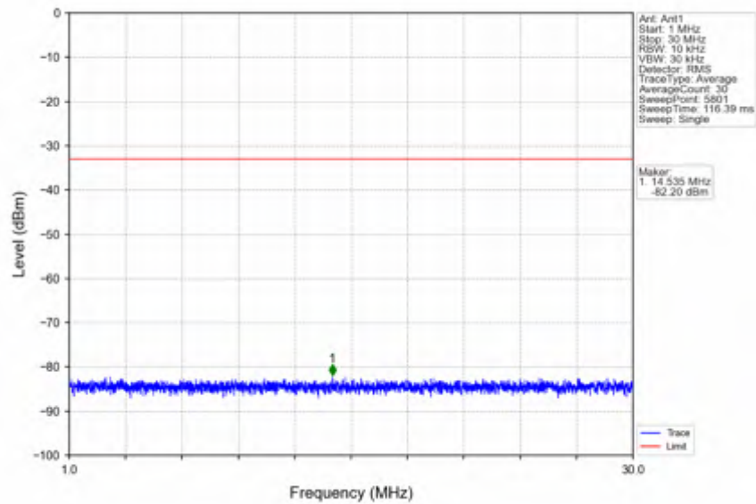
n2_30kHz_SISO_NTNV_10MHz_CP-OFDM QPSK_1905MHz_Inner_1RB_Right
