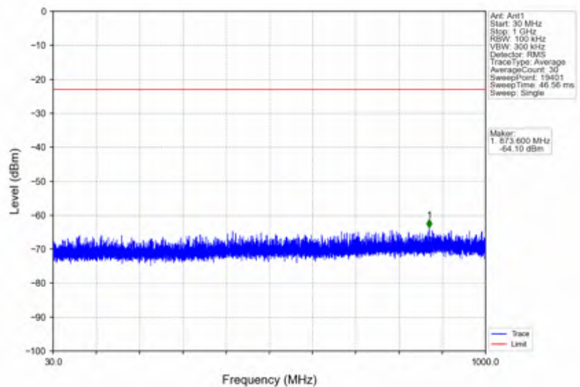
n2_15kHz_SISO_NTNV_20MHz_CP-OFDM QPSK_1860MHz_Edge_1RB_Left
