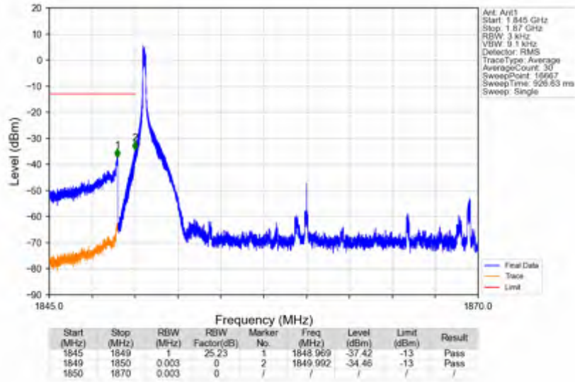
n2_15kHz_SISO_NTNV_20MHz_DFT-s-OFDM_PI/2_BPSK_1860MHz_Edge_1RB_Left
