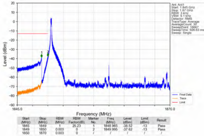
n2_15kHz_SISO_NTV_20MHz_DFT-s-OFDM QPSK_1860MHz_Edge_1RB_Left
