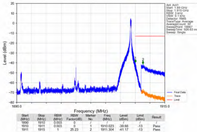
n2_15kHz_SISO_NTNV_20MHz_DFT-s-OFDM QPSK_1900MHz_Inner_1RB_Right
