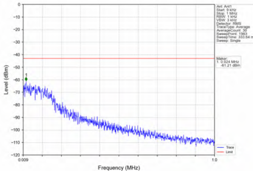
n2_15kHz_SISO_NTV_5MHz_CP-OFDM QPSK_1852.5MHz_Edge_1RB_Left
