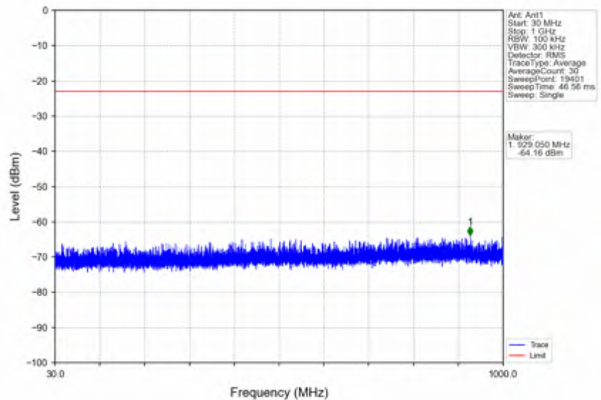
n2_15kHz_SISO_NTNV_20MHz_CP-OFDM QPSK_1880MHz_Edge_1RB_Left
