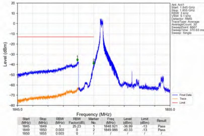
n2_15kHz_SISO_NTNV_5MHz_DFT-s-OFDM QPSK_1852.5MHz_Inner_1RB_Left
