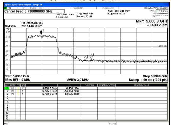
802.11 n40 5670MHz
