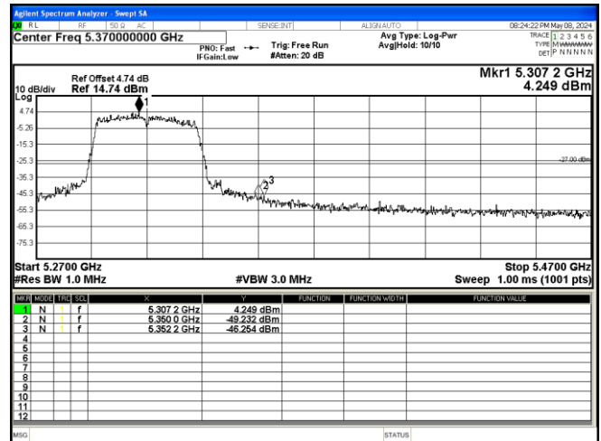
802.11 ac40 5310MHz
