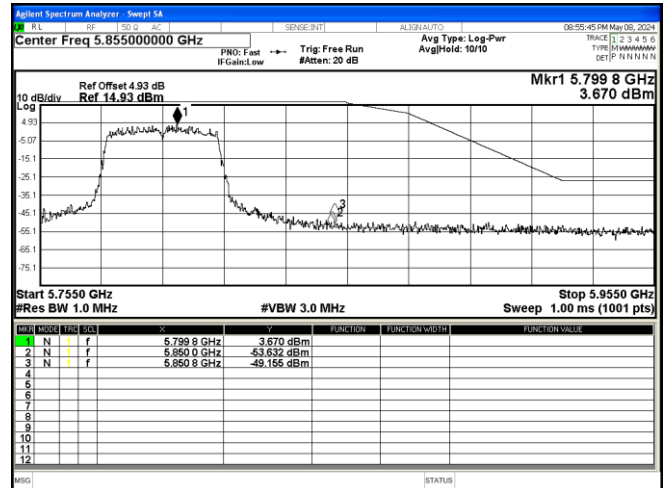
802.11 n40 5795MHz
