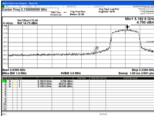
802.11 n40 5190MHz
