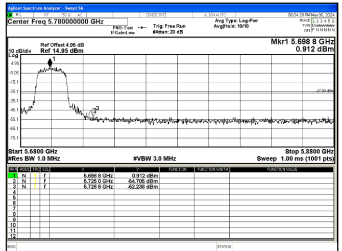
802.11 ac20 5700MHz
