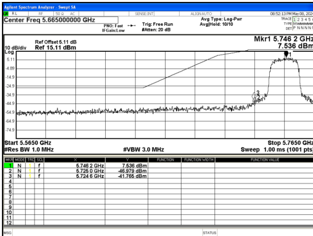
802.11 ac20 5745MHz
