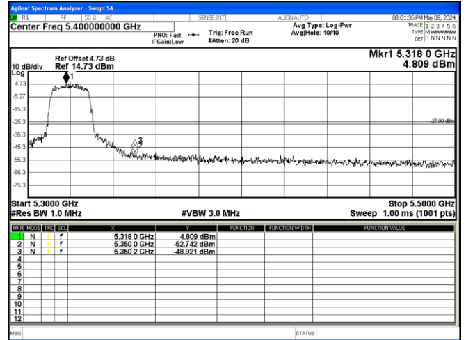
802.11 ac20 5320MHz
