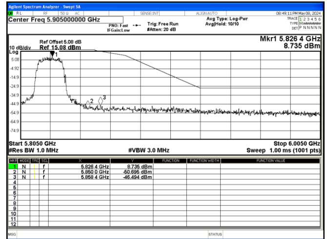
802.11 a 5825MHz
