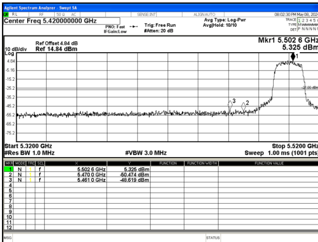
802.11 ac20 5500MHz
