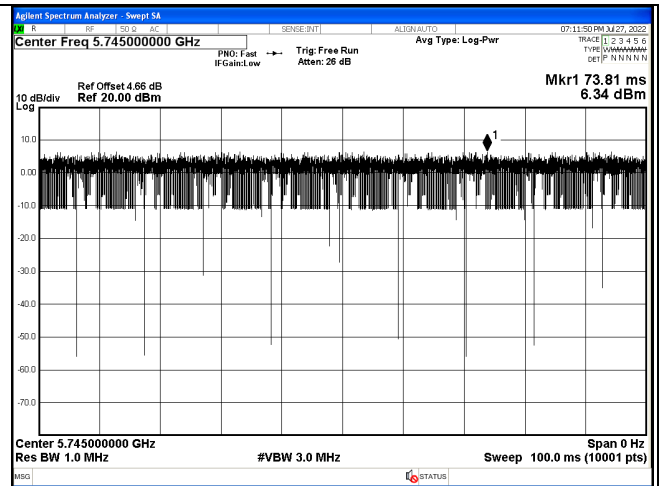
802.11n(HT20) 5745MHz
