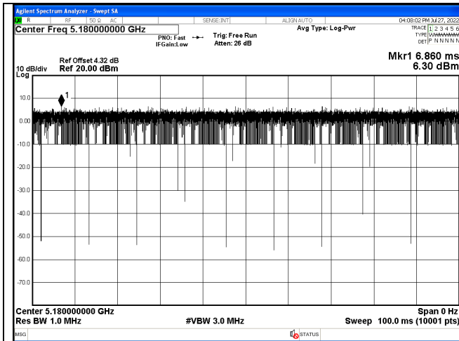
802.11n(HT20) 5180MHz
