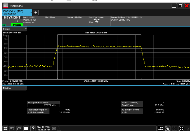
n41_30MHz_30kHz_2674.98MHz_CP-OFDM 64 QAM_RB78@0 27.770MHz
